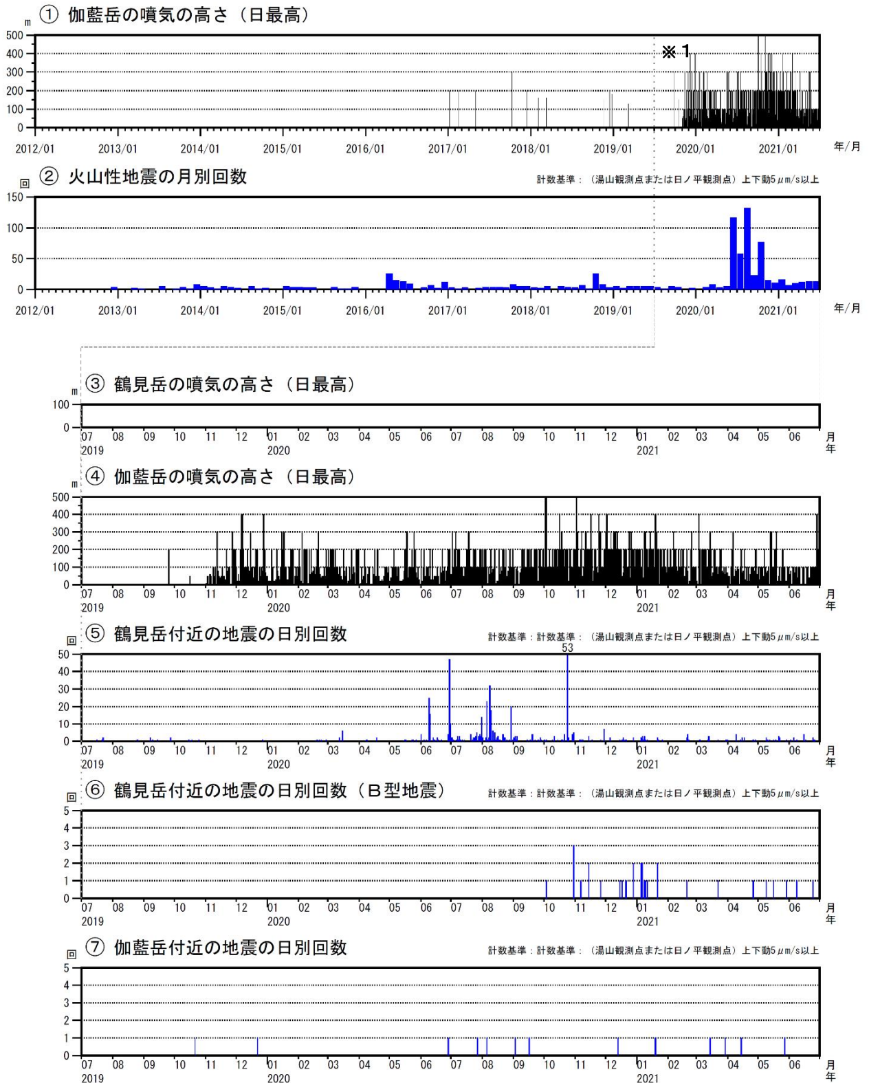
図2 鶴見岳・伽藍岳 火山活動経過図（2012年1月～2021年6月）
