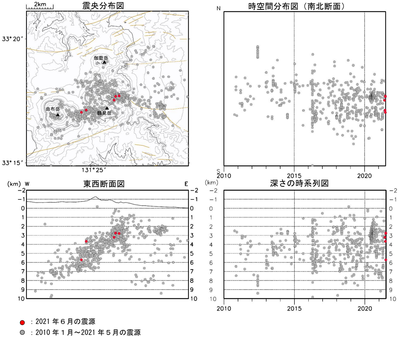
図3 鶴見岳・伽藍岳 震源分布図（2010年1月～2021年6月）
