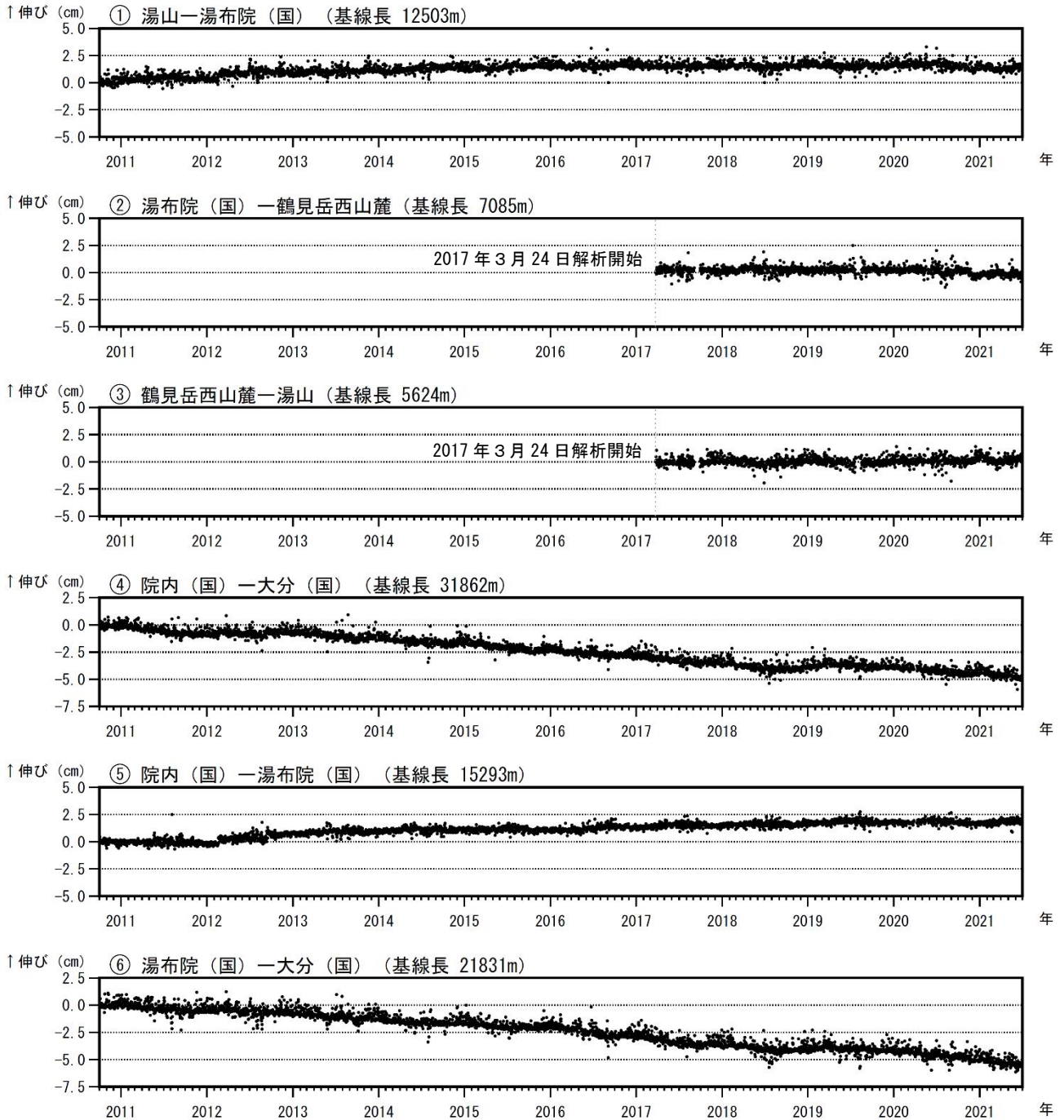
図4 鶴見岳・伽藍岳 GNSS連続観測による基線長変化 (2010年10月～2021年6月)
