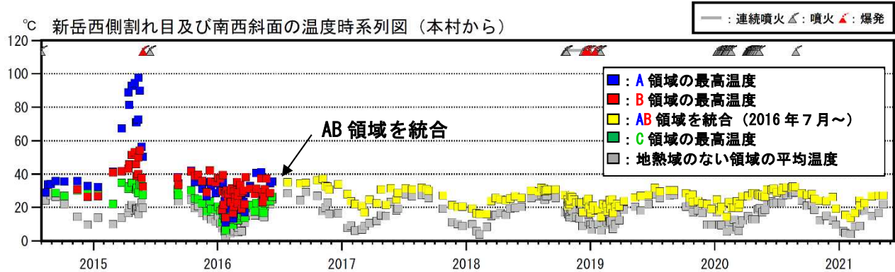
図3 口永良部島 新岳西斜面及び新岳南西側斜面の地熱域の温度時系列(2014年8月～2021年5月)
