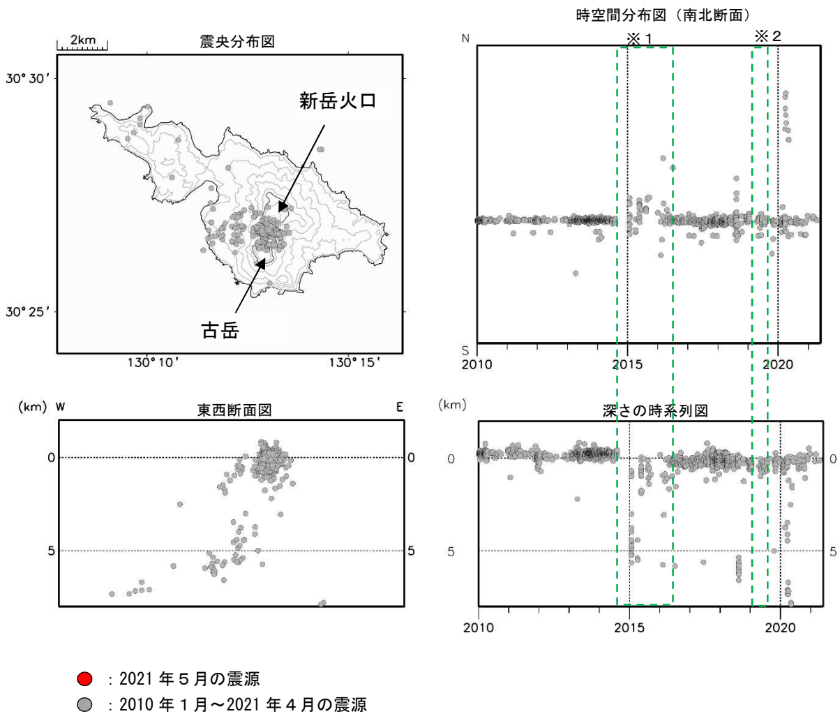
図7 口永良部島 震源分布図（2010年1月～2021年5月）
