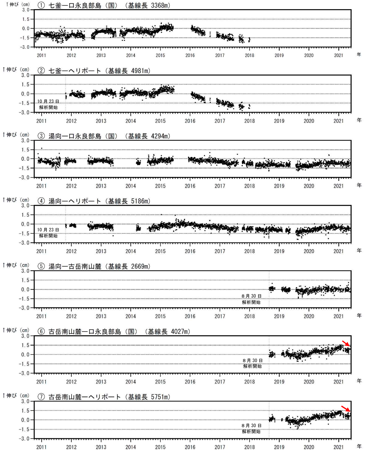
図8 口永良部島 GNSS 連続観測による基線長変化（2010年10月～2021年5月）
