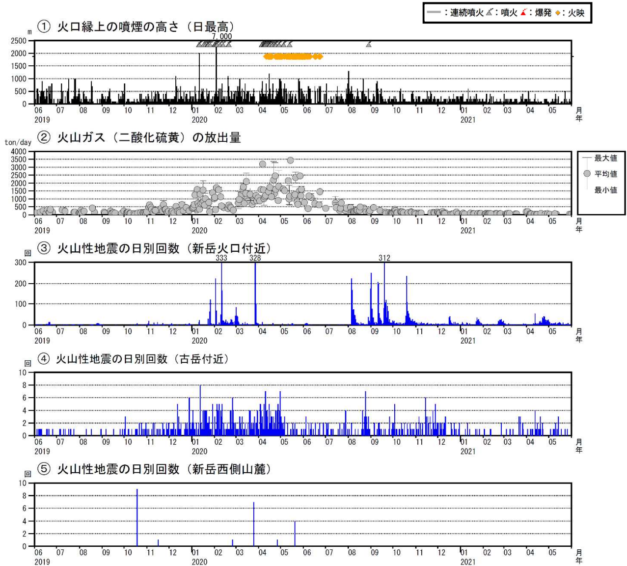
図6 口永良部島 最近の火山活動経過図（2019年6月～2021年5月）
