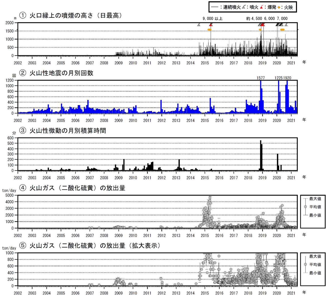
図5 口永良部島 火山活動経過図（2002年1月～2021年5月）
