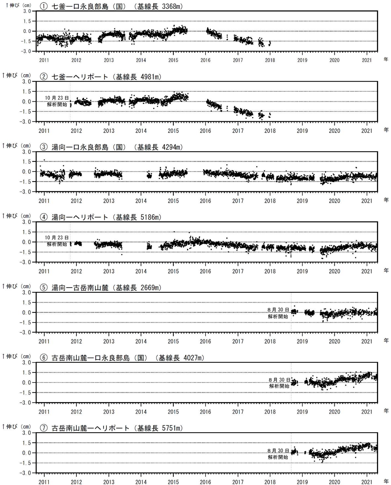
図9 口永良部島 GNSS 連続観測による基線長変化（2010年10月～2021年4月）
