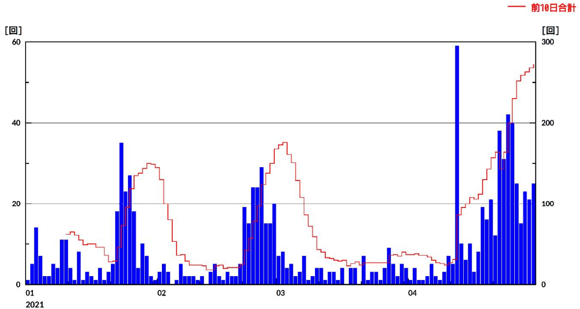
図1 口永良部島 火山性地震の日別地震回数と前10日間の積算回数（2021年1月～4月）
