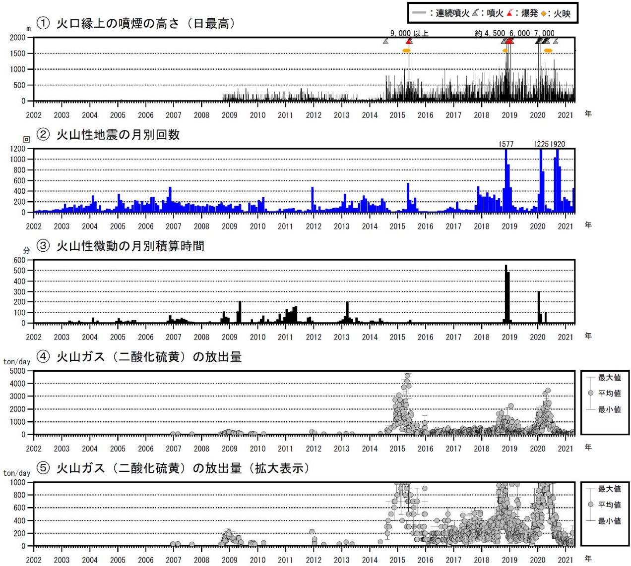
図6 口永良部島 火山活動経過図（2002年1月～2021年4月）
