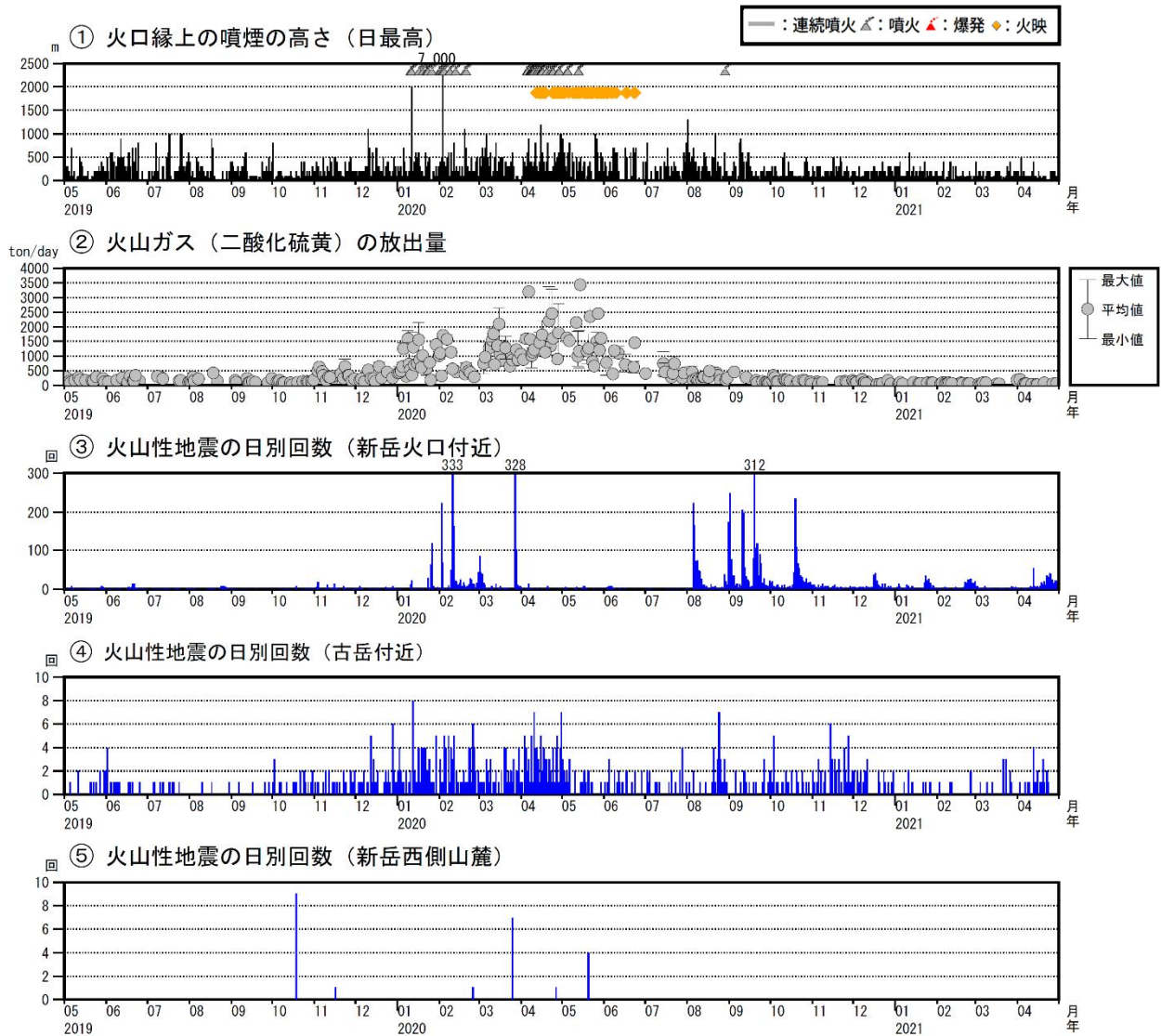
図7 口永良部島 最近の火山活動経過図（2019年5月～2021年4月）
