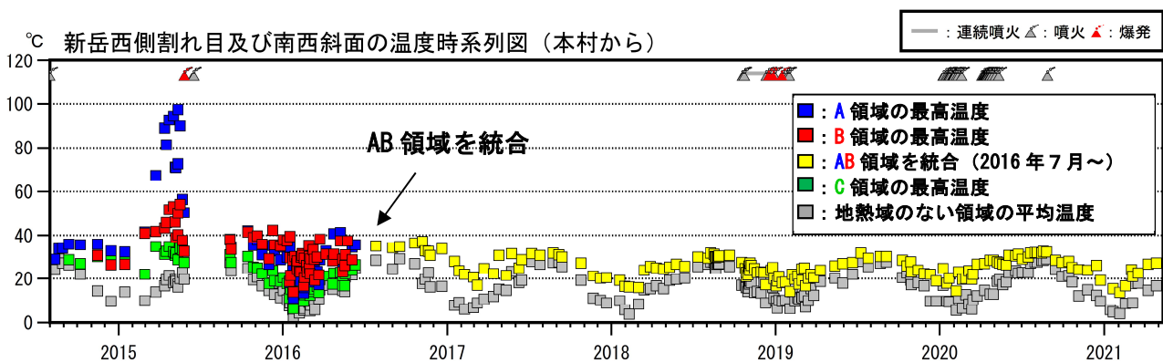
図4 口永良部島 新岳西斜面及び新岳南西側斜面の地熱域の温度時系列(2014年8月～2021年4月)
