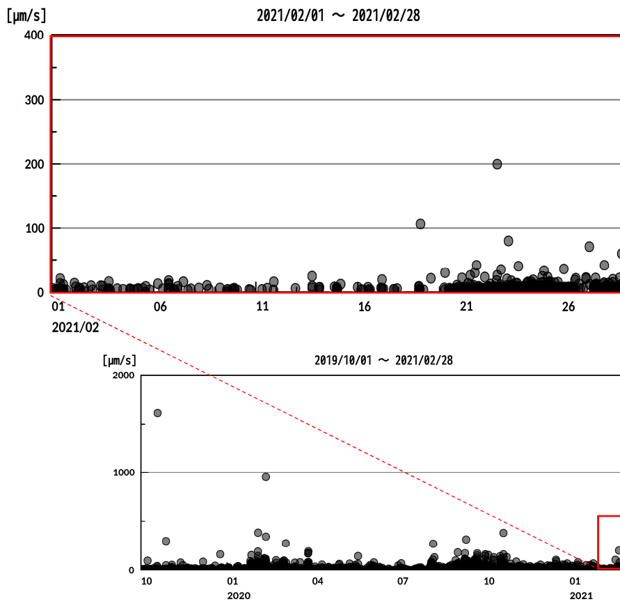
図3 口永良部島 火山性地震の最大振幅（FDKL（京）観測点の上下動、上：2021年2月1日～2月28日、下：2019年10月1日～2021年2月28日） 21日以降、これまでの活動でみられたような規模の大きな火山性地震は観測されませんでした。
