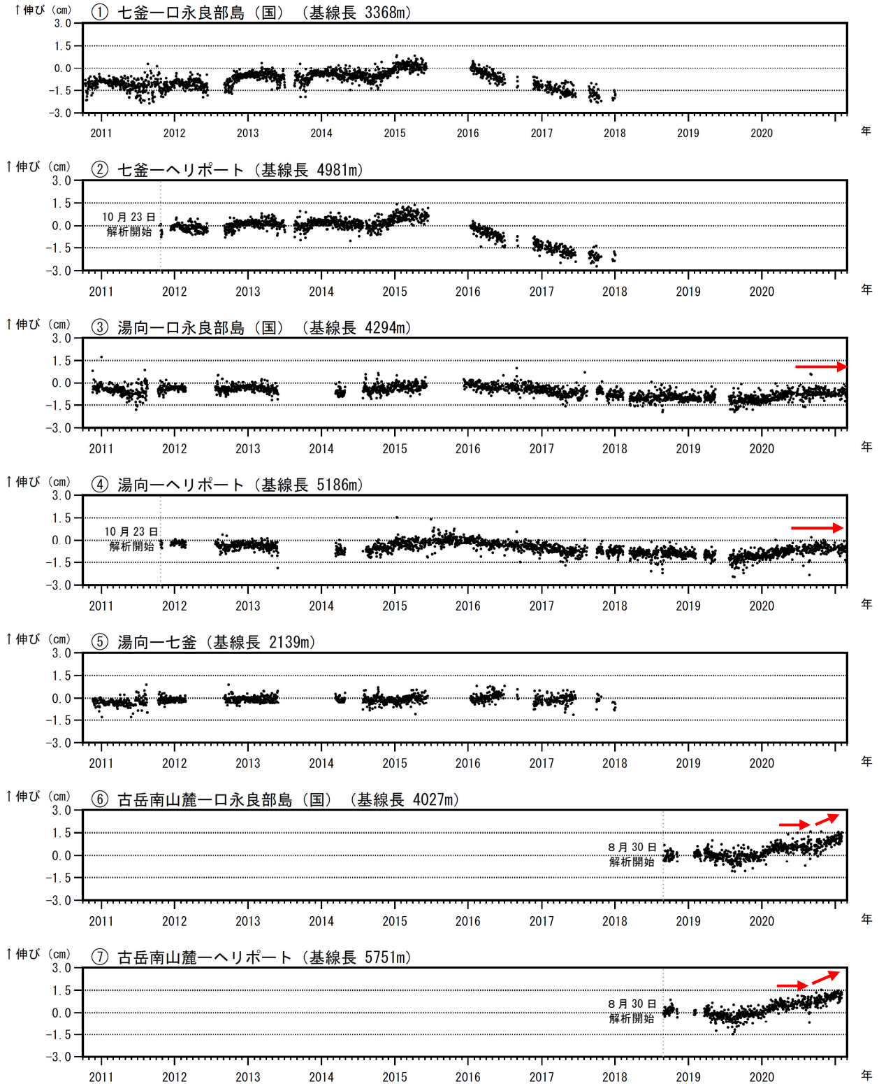
図 10 口永良部島 GNSS 連続観測による基線長変化（2010年10月～2021年2月）
