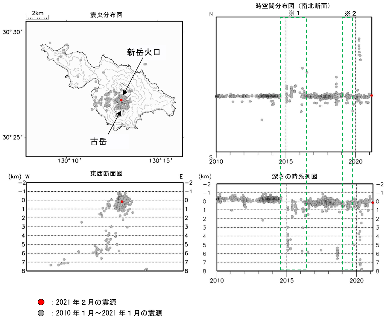
図9 口永良部島 震源分布図（2010年1月～2021年2月）
