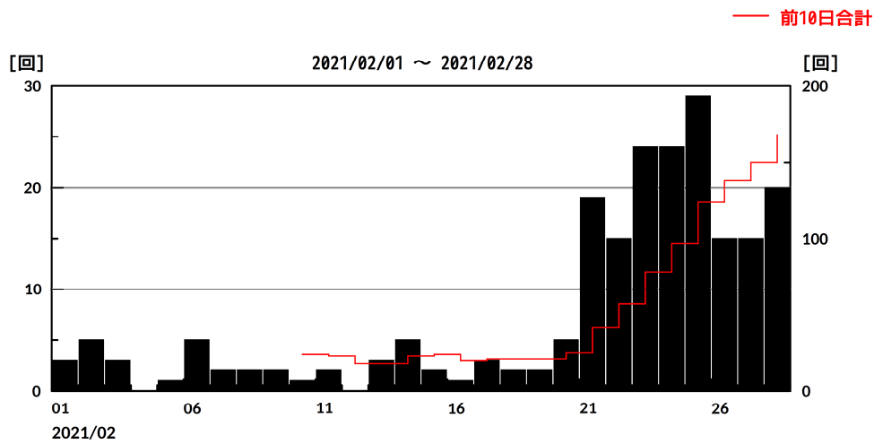
図2 口永良部島 火山性地震の日別地震回数と前10日間の積算回数（2021年2月1日～2月28日） 21日以降、新岳火口付近の浅い所が震源と推定される火山性地震が増加し、多い状態となりました。
