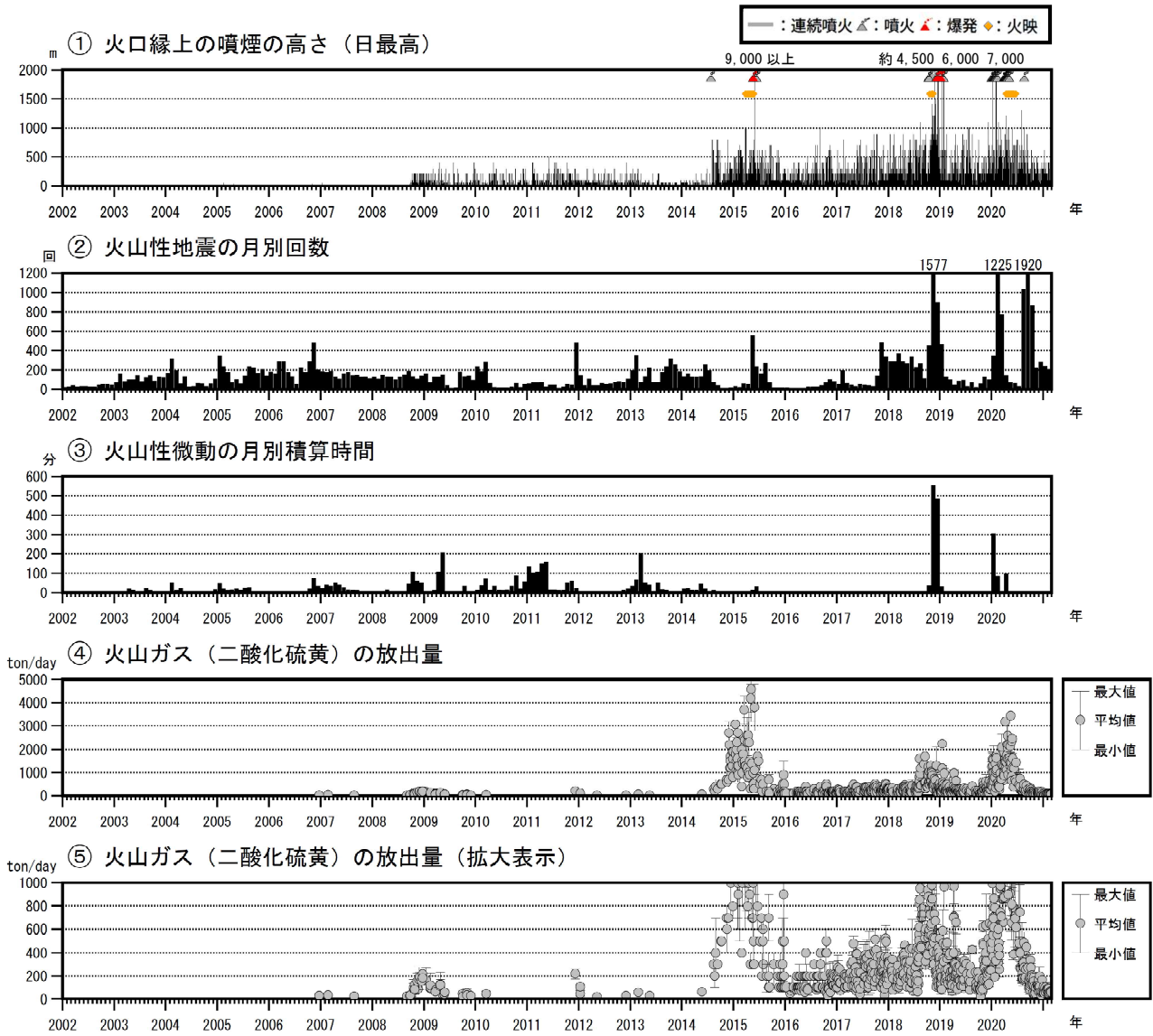
図7 口永良部島 火山活動経過図（2002年1月～2021年2月）
