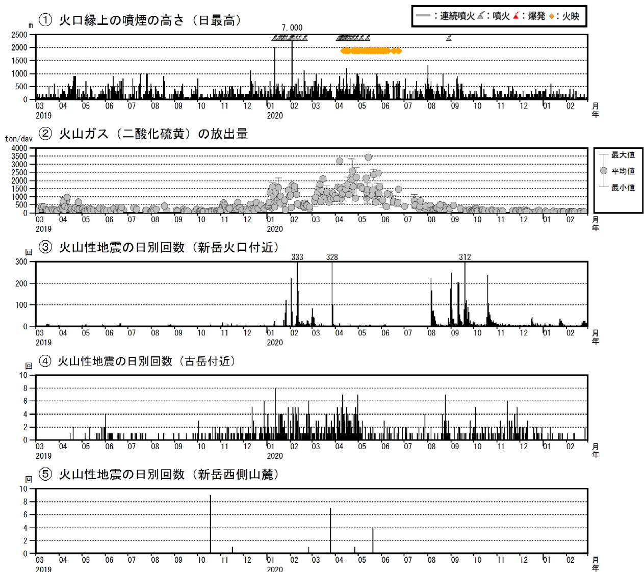
図8 口永良部島 最近の火山活動経過図（2019年3月～2021年2月）
