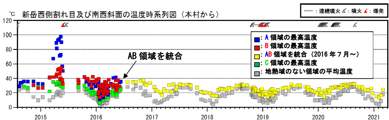
図5 口永良部島 新岳西斜面及び新岳南西側斜面の地熱域の温度時系列（2014年8月～2021年3月1日）
