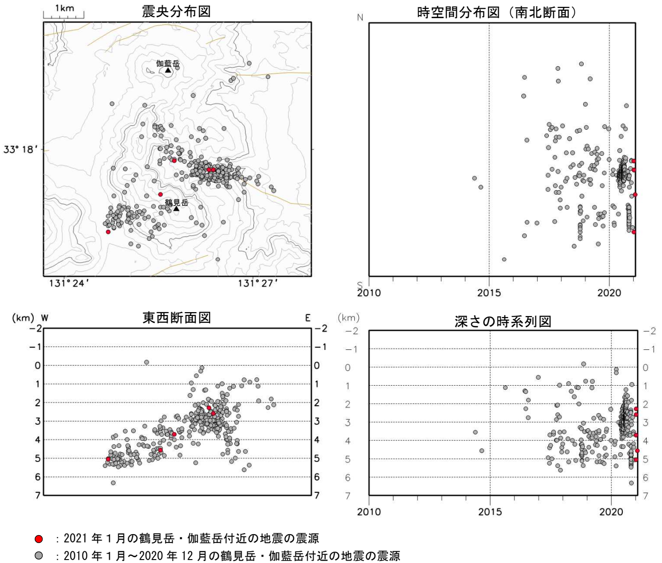
図 3-2 鶴見岳・伽藍岳 震源分布図（鶴見岳・伽藍岳付近の地震）（2010年1月～2021年1月）
