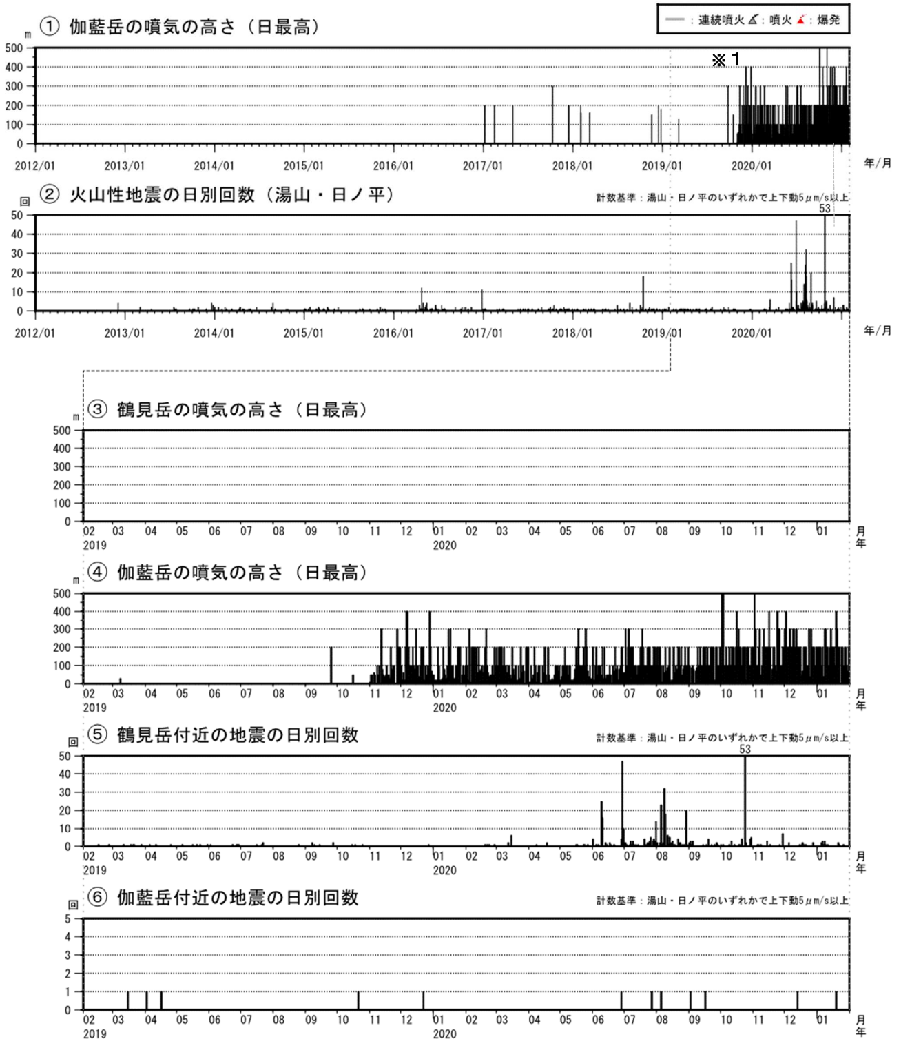
図2 鶴見岳・伽藍岳 火山活動経過図（2012年1月～2021年1月）
