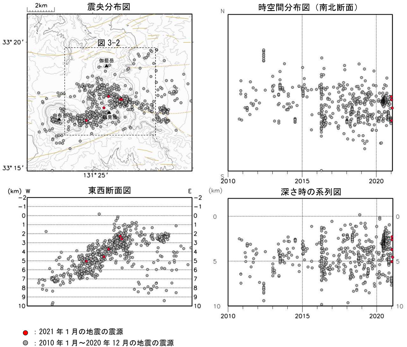
図 3-1 鶴見岳・加藍岳 震源分布図（広域）（2010年1月～2021年1月）
