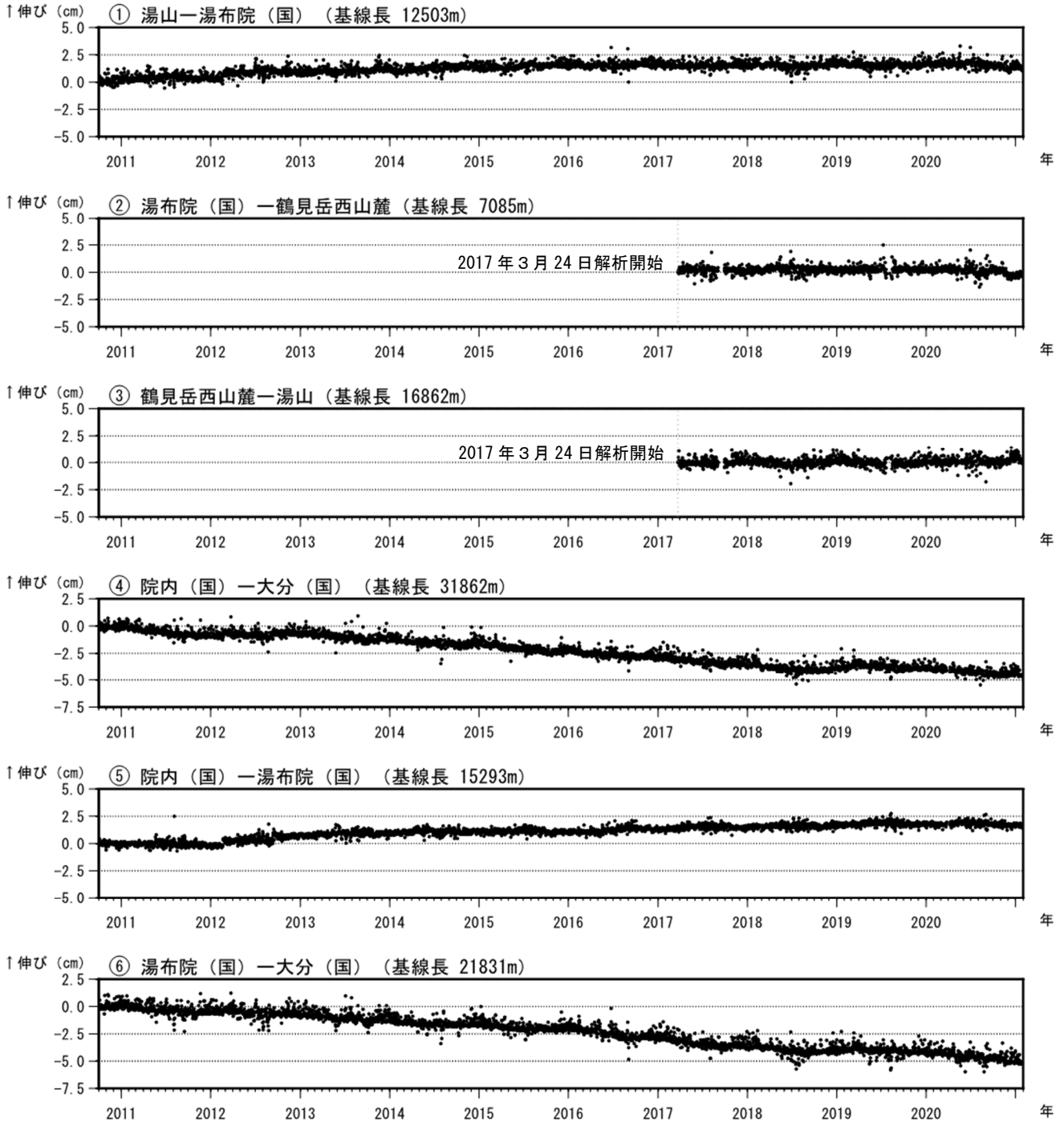
図4 鶴見岳・伽藍岳 GNSS連続観測による基線長変化（2010年10月～2021年1月）
