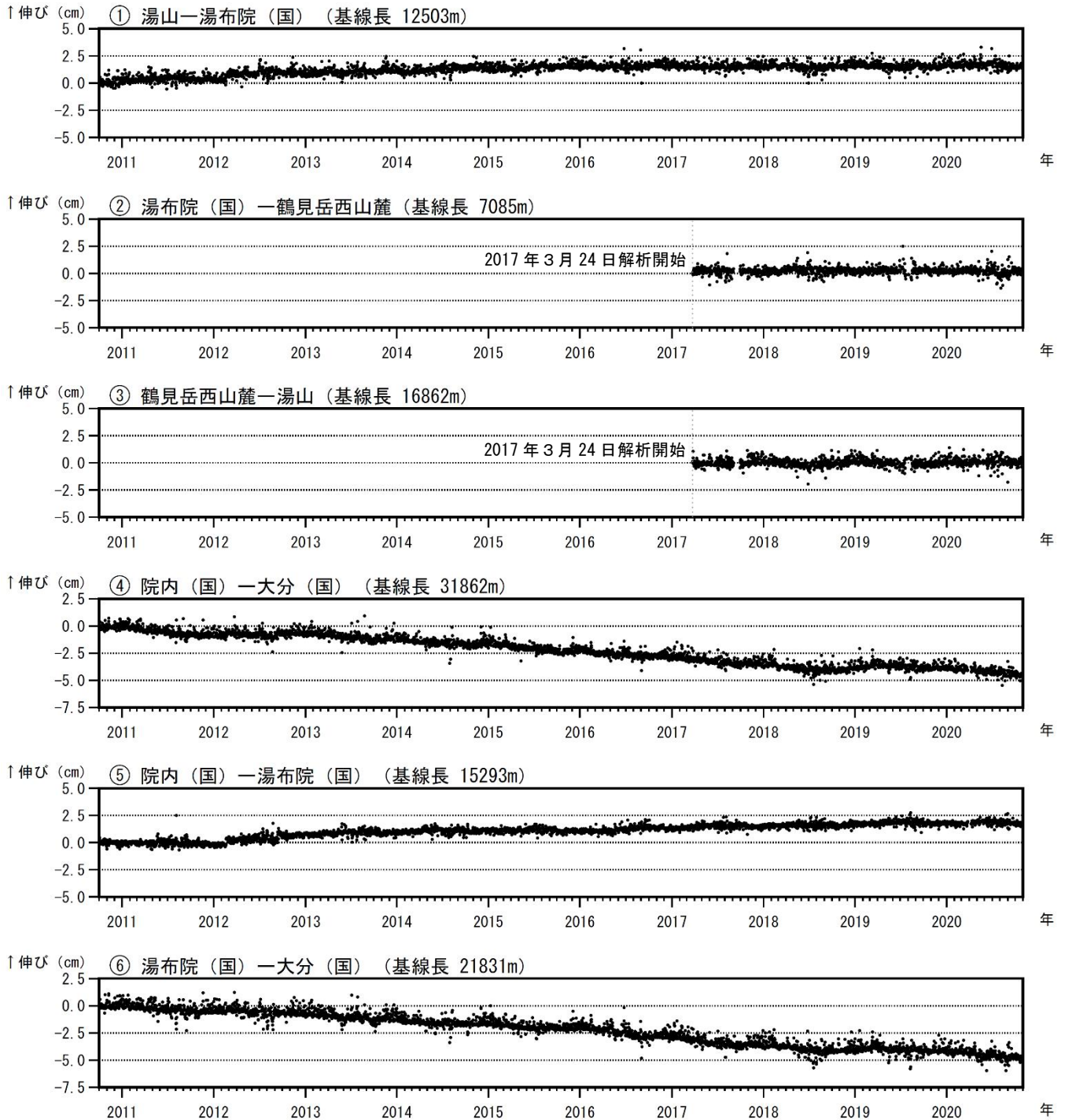
図4 鶴見岳・伽藍岳 GNSS連続観測による基線長変化（2010年10月～2020年10月）
