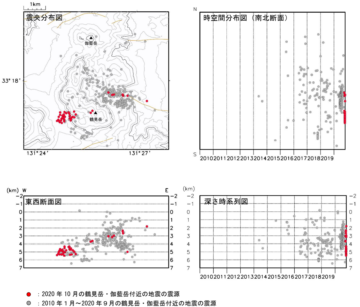
図 3-2 鶴見岳・伽藍岳 震源分布図（鶴見岳・伽藍岳付近の地震）（2010年1月～2020年10月）
