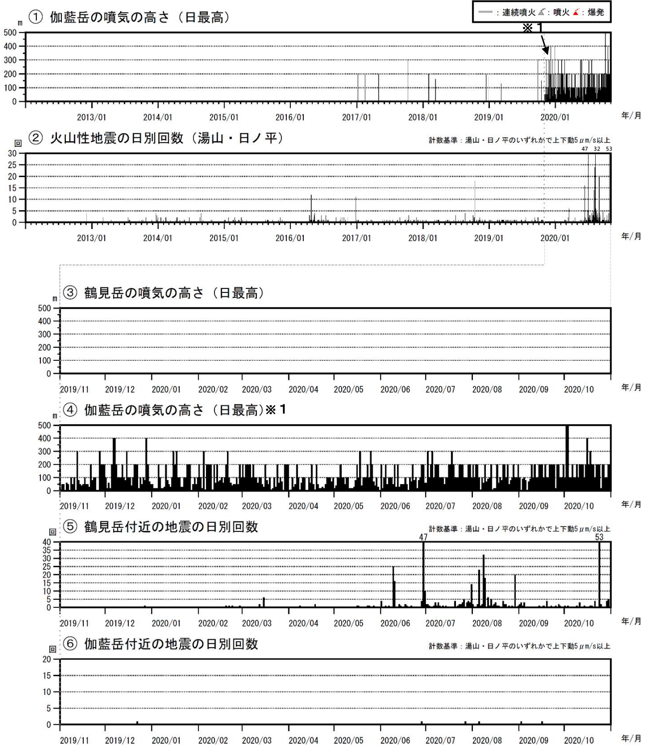
図2 鶴見岳・伽藍岳 火山活動経過図（2012年1月～2020年10月）
