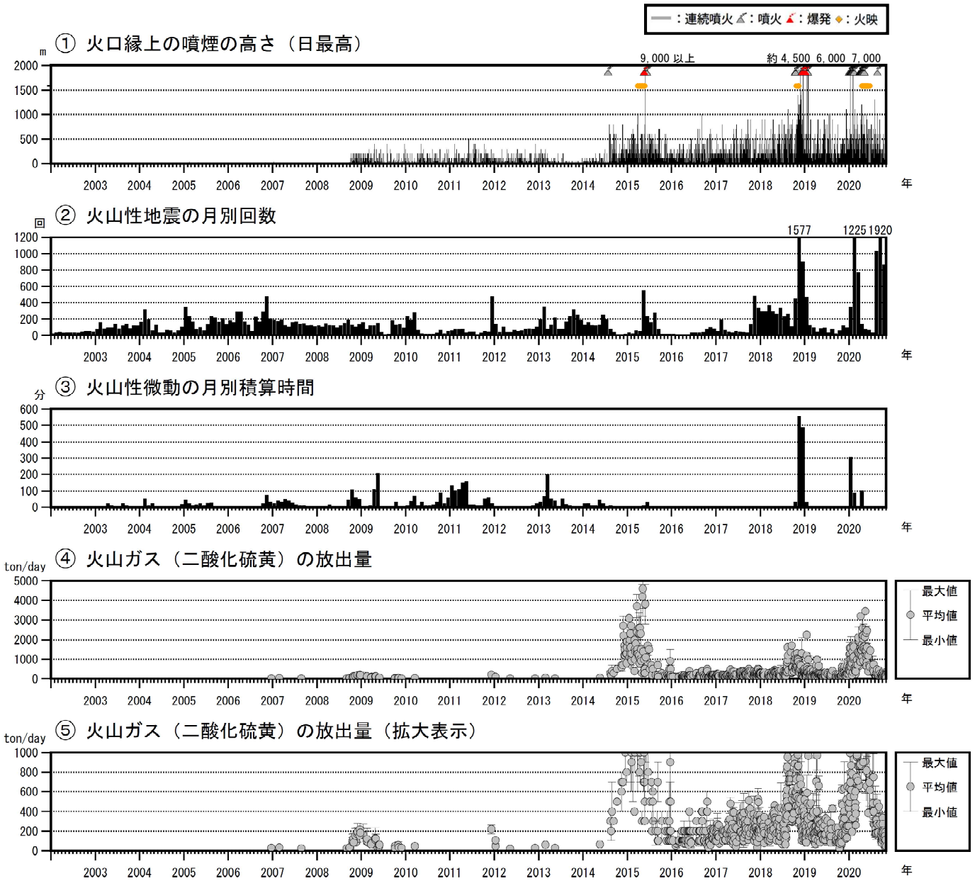
図5 口永良部島 火山活動経過図（2002年1月～2020年10月）
