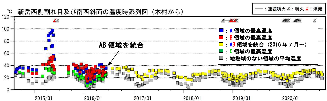
図3 口永良部島 新岳西斜面及び新岳南西側斜面の地熱域の温度時系列（2014年8月～2020年10月）
