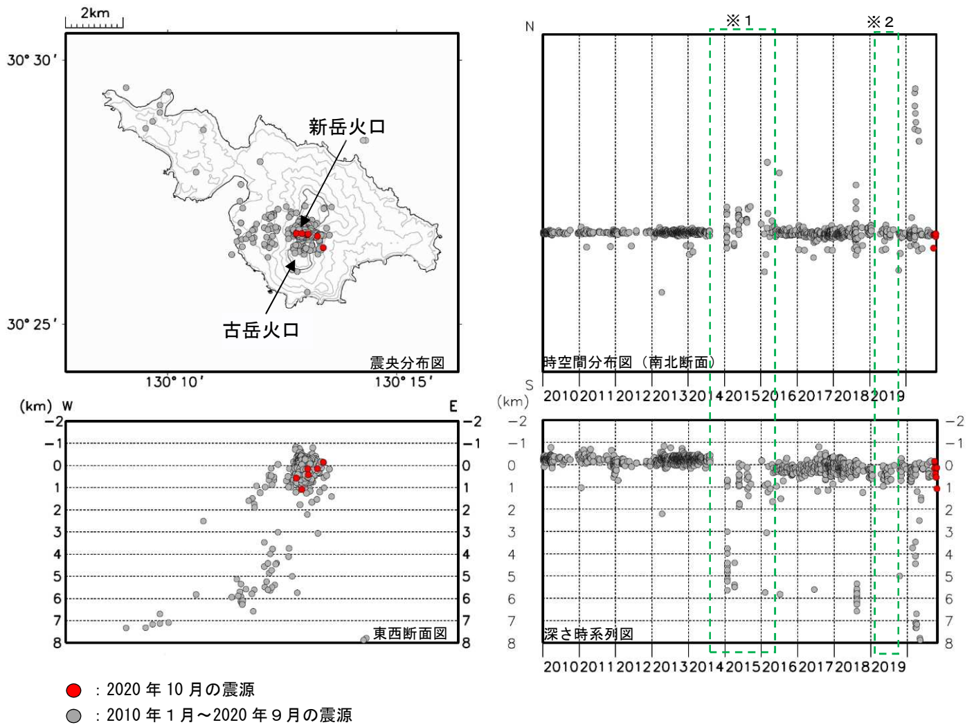
図7 口永良部島 震源分布図（2010年1月～2020年10月）
