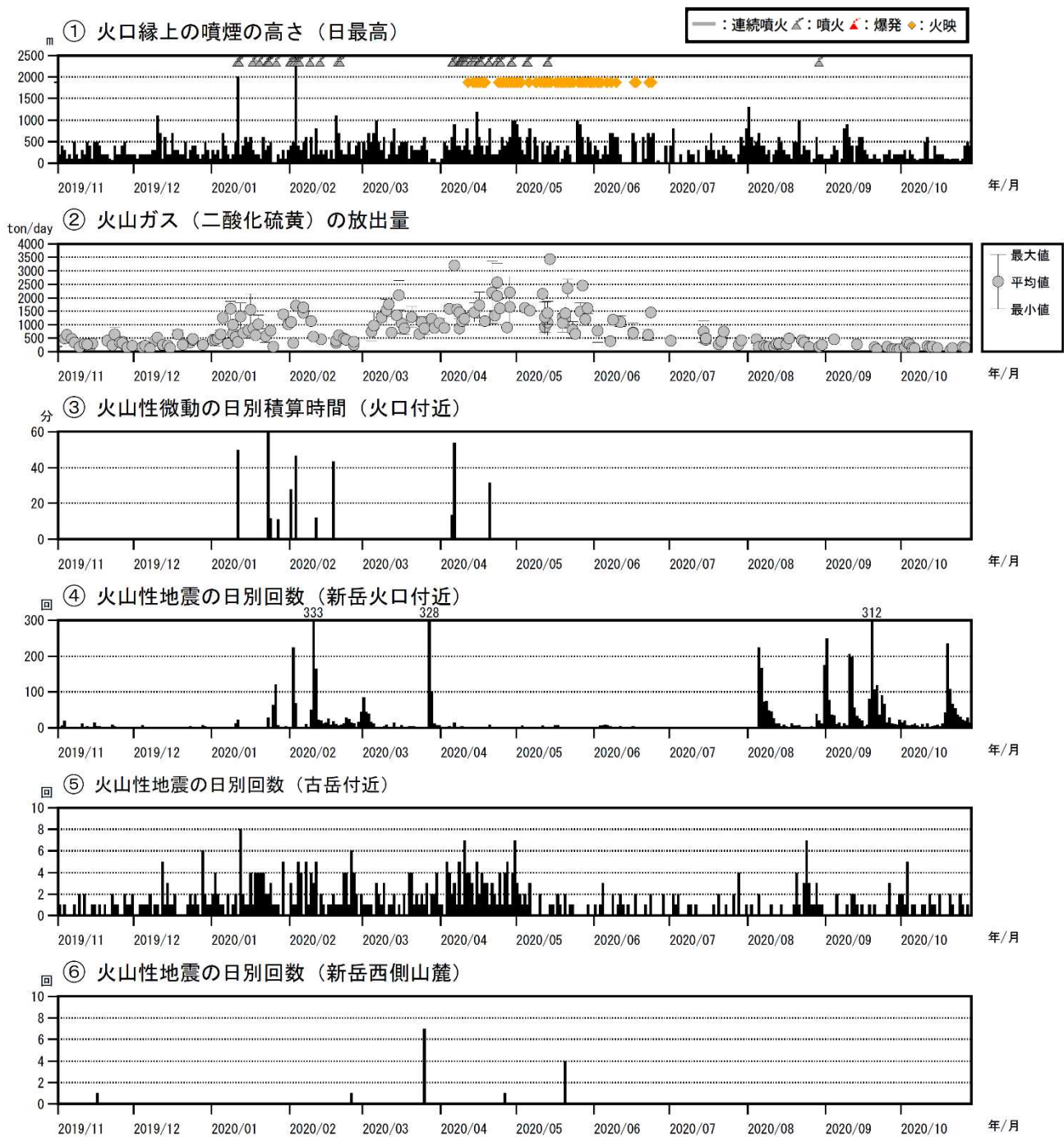
図6 口永良部島 最近の火山活動経過図（2019年11月～2020年10月）
