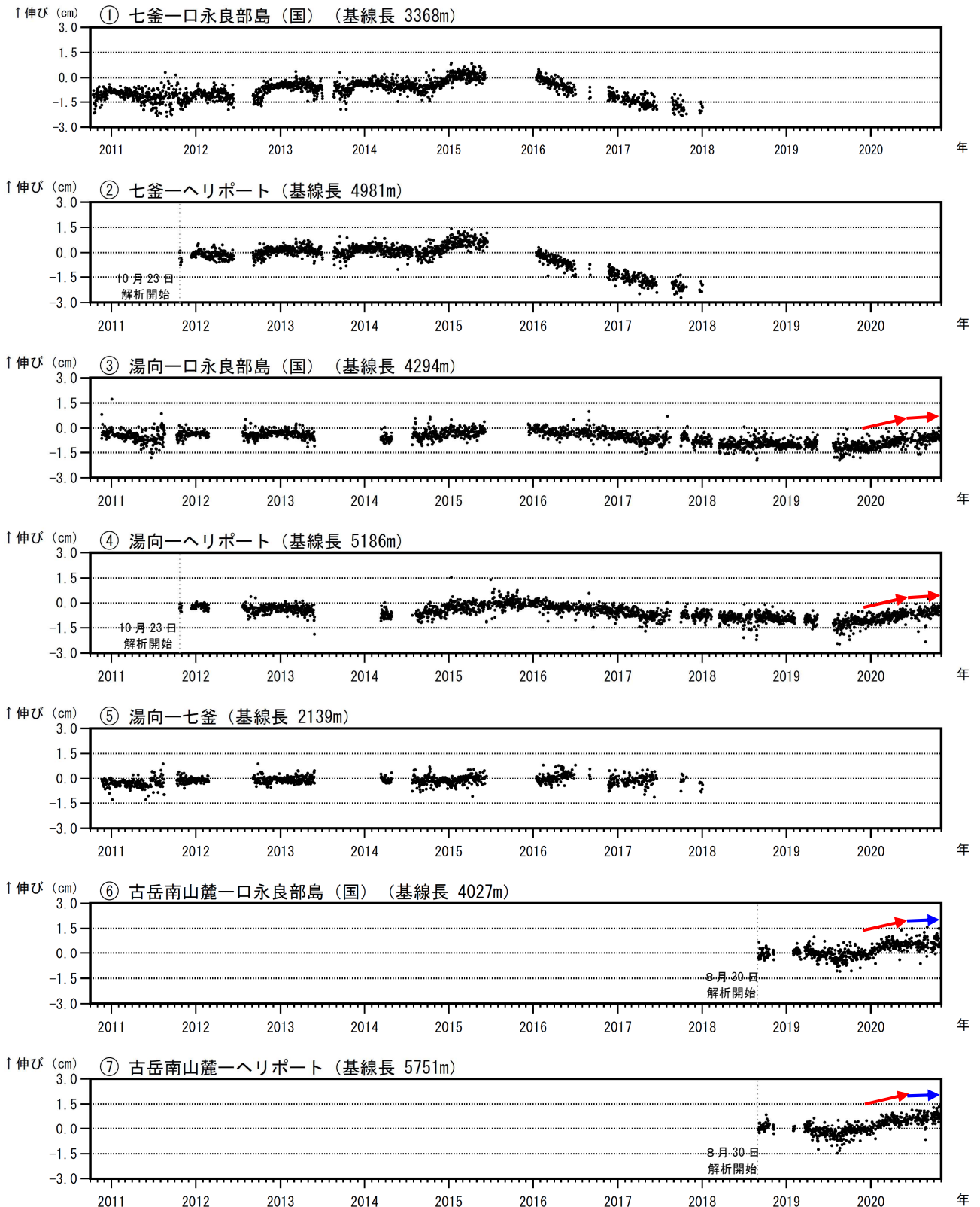
図8 口永良部島 GNSS 連続観測による基線長変化（2010年10月～2020年10月）
