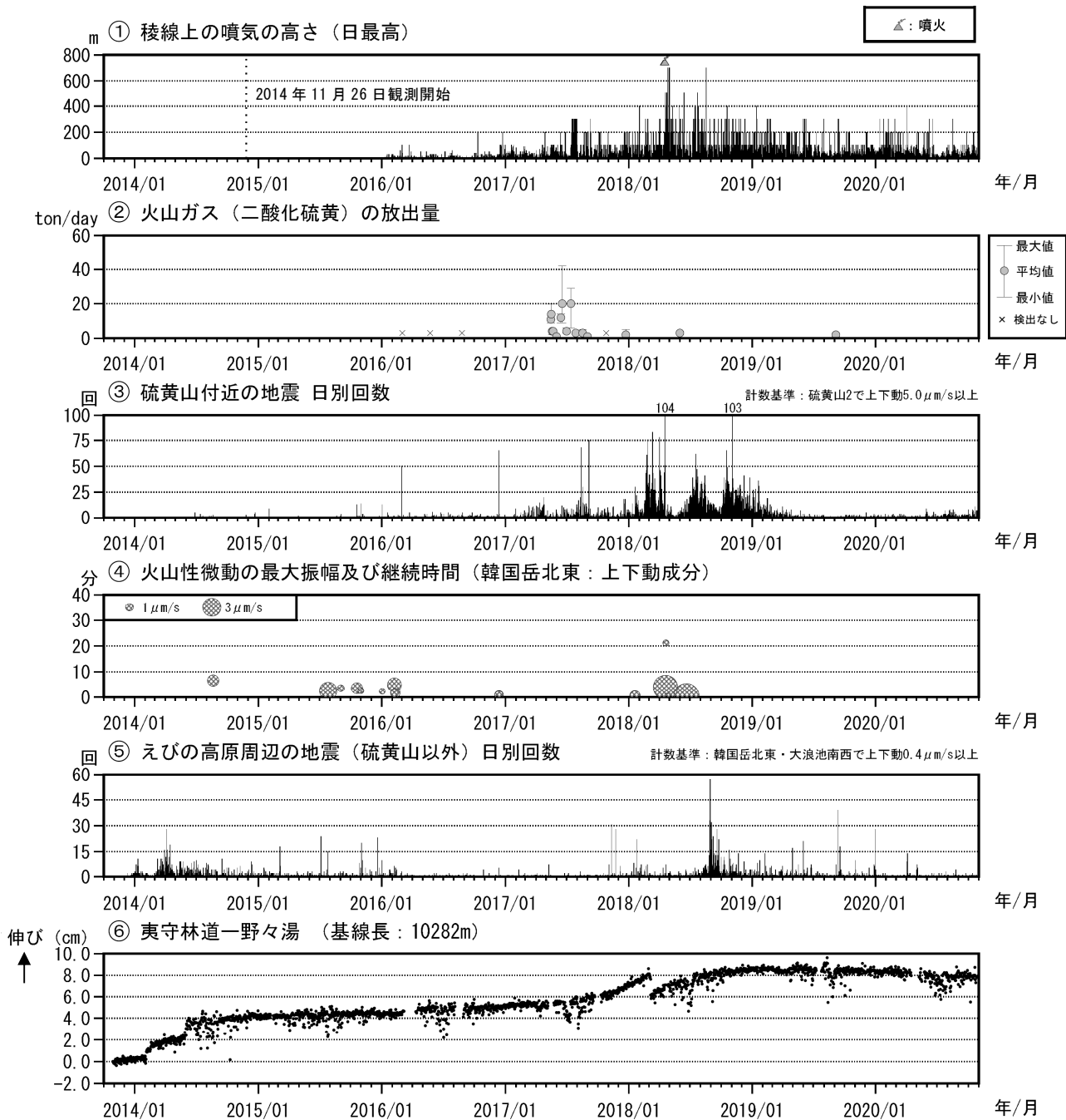
図8 霧島山（えびの高原（硫黄山）周辺） 火山活動経過図（2013年10月～2020年10月）
