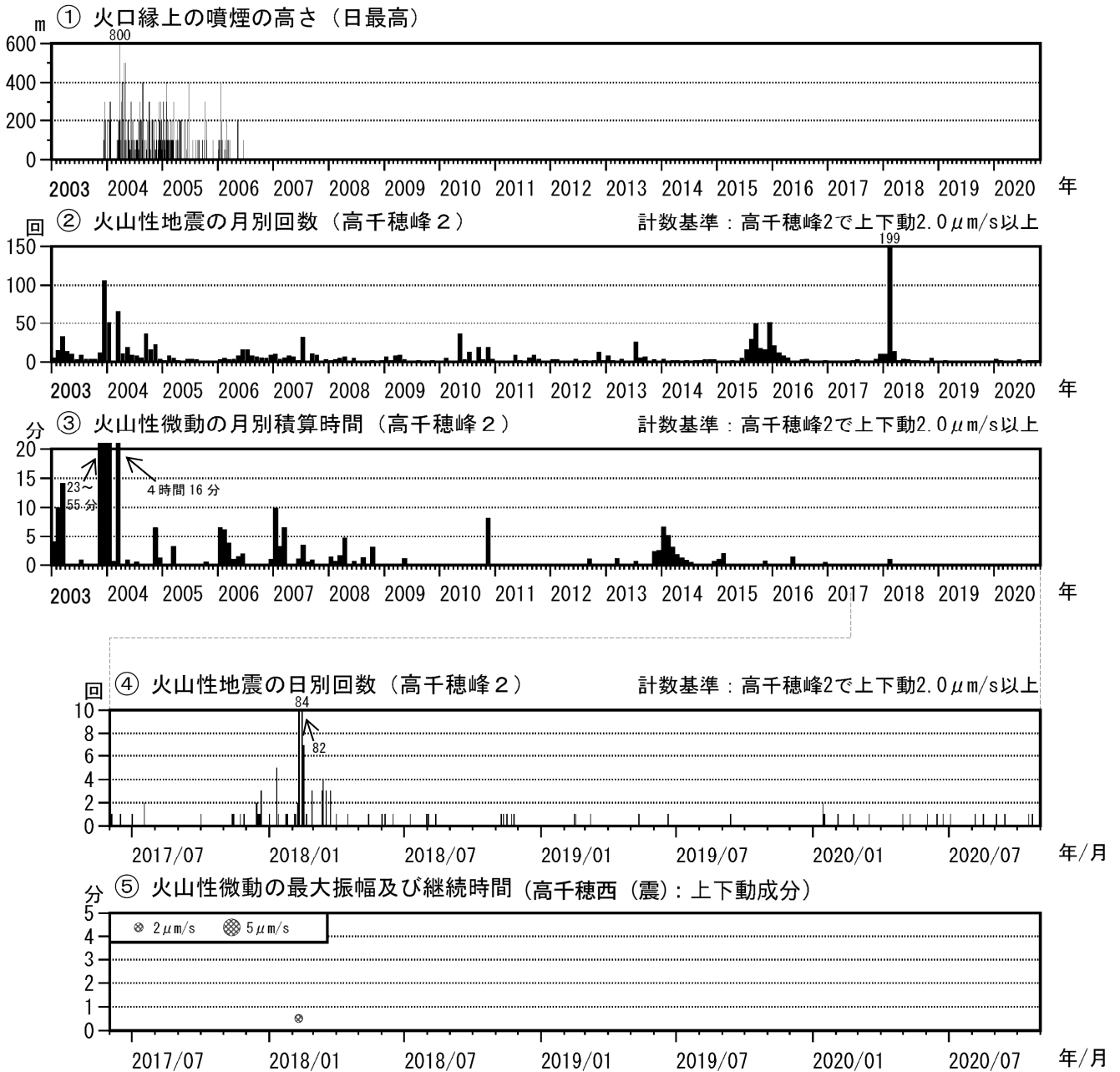
図6 霧島山（御鉢） 火山活動経過図（2003年1月～2020年10月）
