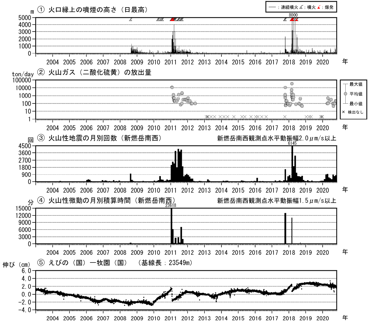
図4 霧島山（新燃岳） 火山活動経過図（2003年1月～2020年10月）
