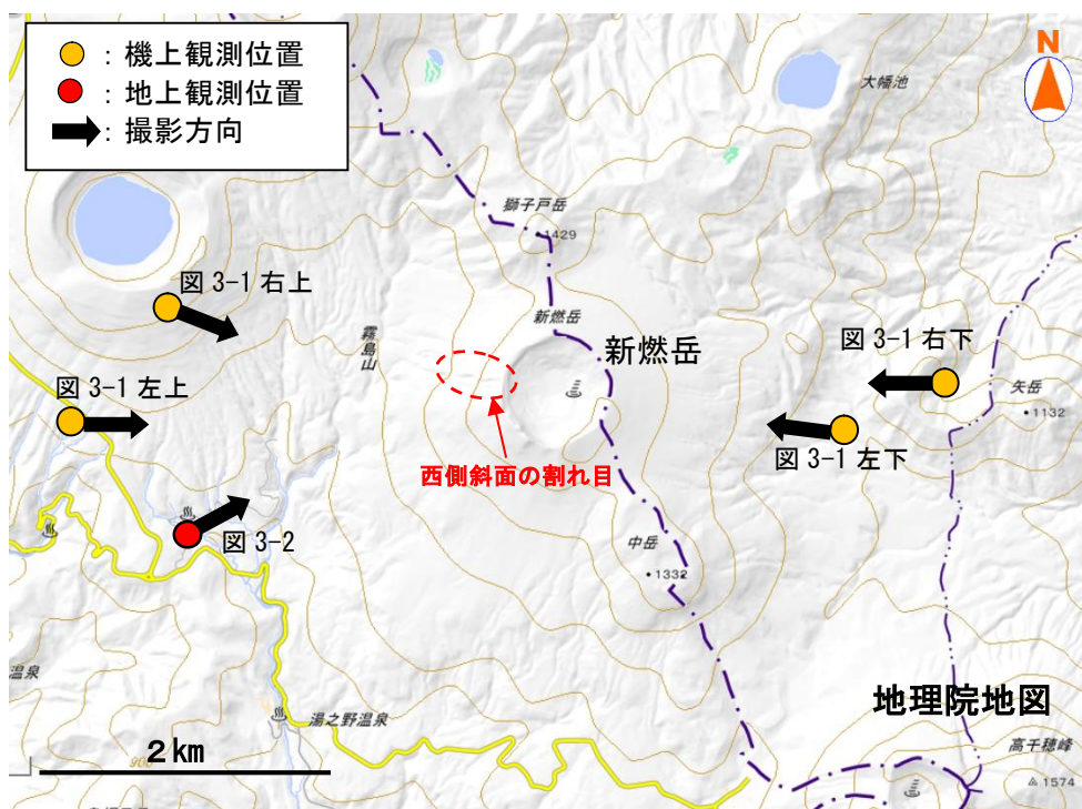
図2 霧島山（新燃岳） 図3の観測位置及び撮影方向
