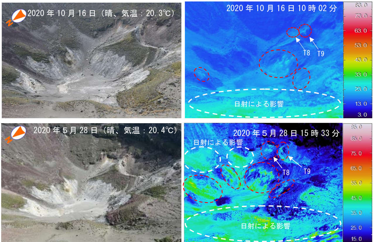
図 2-1 霧島山 (御鉢) 火口内の状況 (定点 1 (火口縁北西側) から観測)
