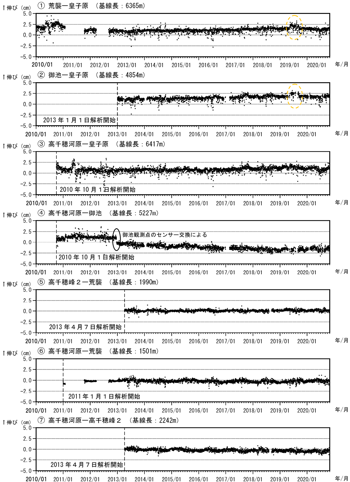
図8 霧島山（御鉢） GNSS 連続観測による基線長変化（2010年1月～2020年10月）
