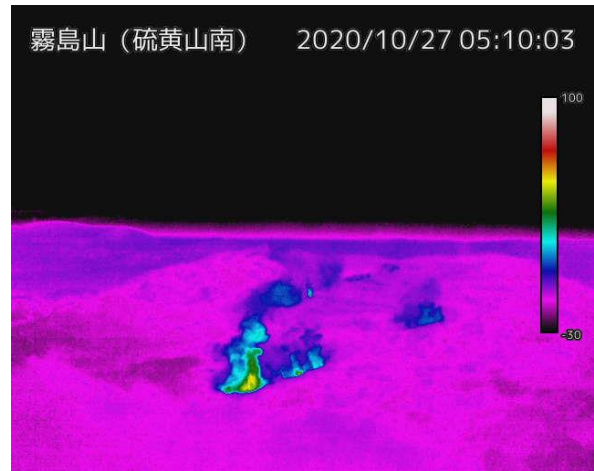
図1-2 霧島山（えびの高原（硫黄山）周辺） 硫黄山南側の状況 （10月27日、硫黄山南監視カメラによる）
