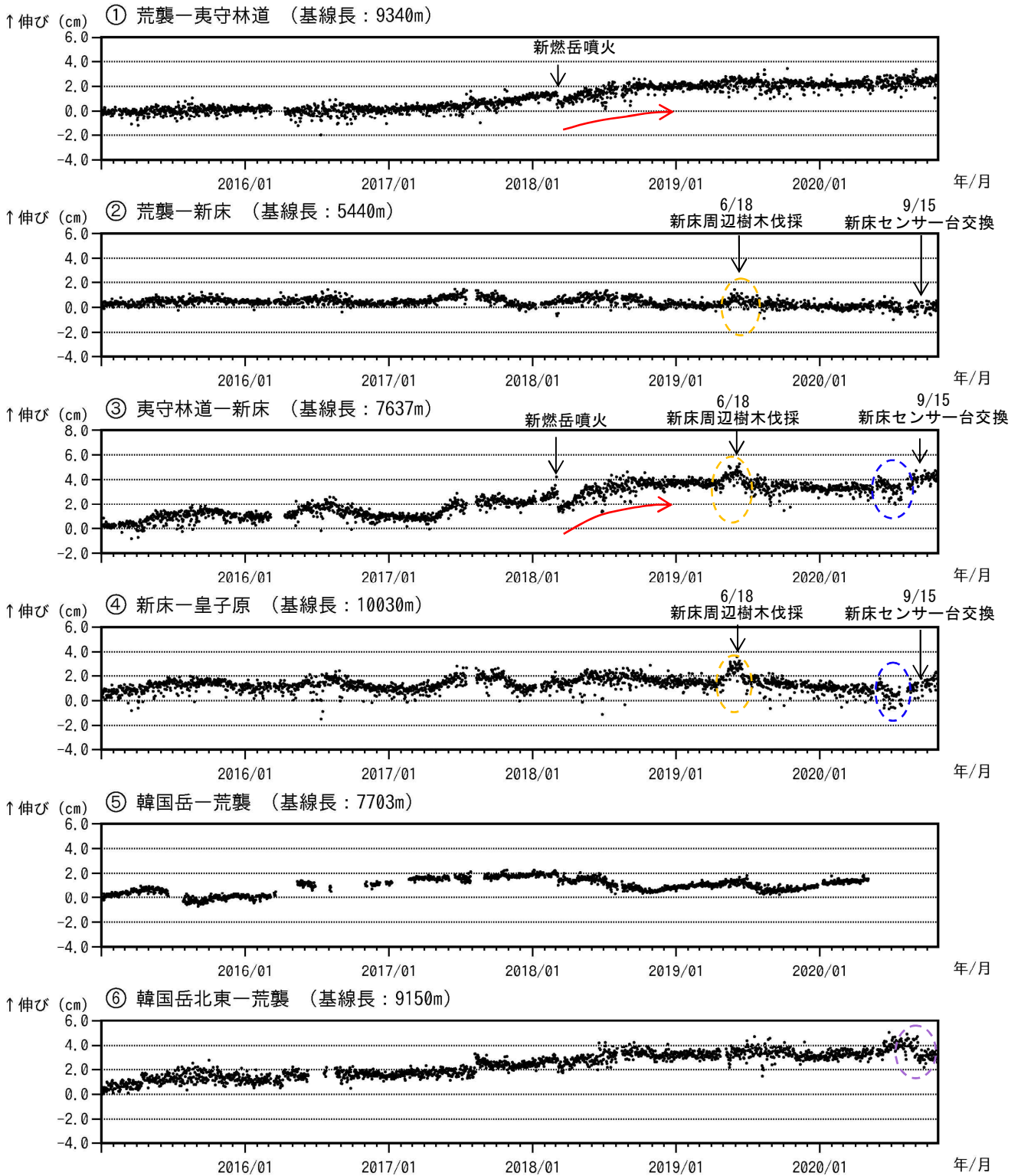
図 9-1 霧島山（新燃岳） GNSS 連続観測による基線長変化（2015 年 1 月～2020 年 10 月）
