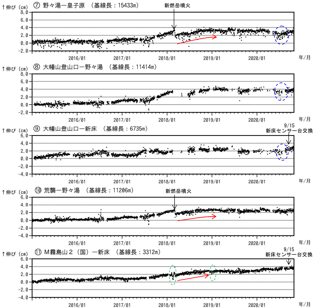
図 9-2 霧島山（新燃岳） GNSS 連続観測による基線長変化（2015 年 1 月～2020 年 10 月）
