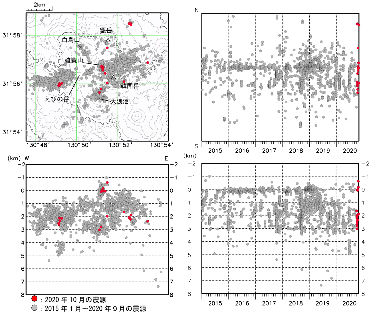
図6 霧島山（えびの高原（硫黄山）周辺） 震源分布図（2015年1月～2020年10月）
