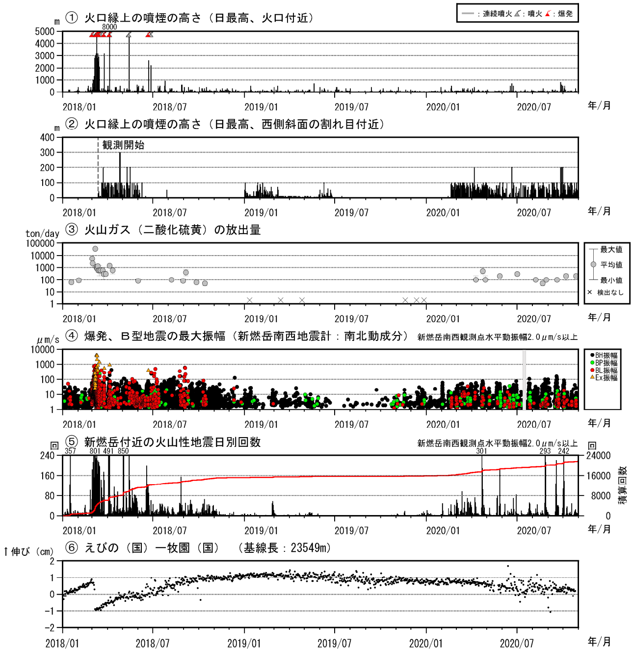
図5 霧島山（新燃岳） 火山活動経過図（2018年1月～2020年10月）
