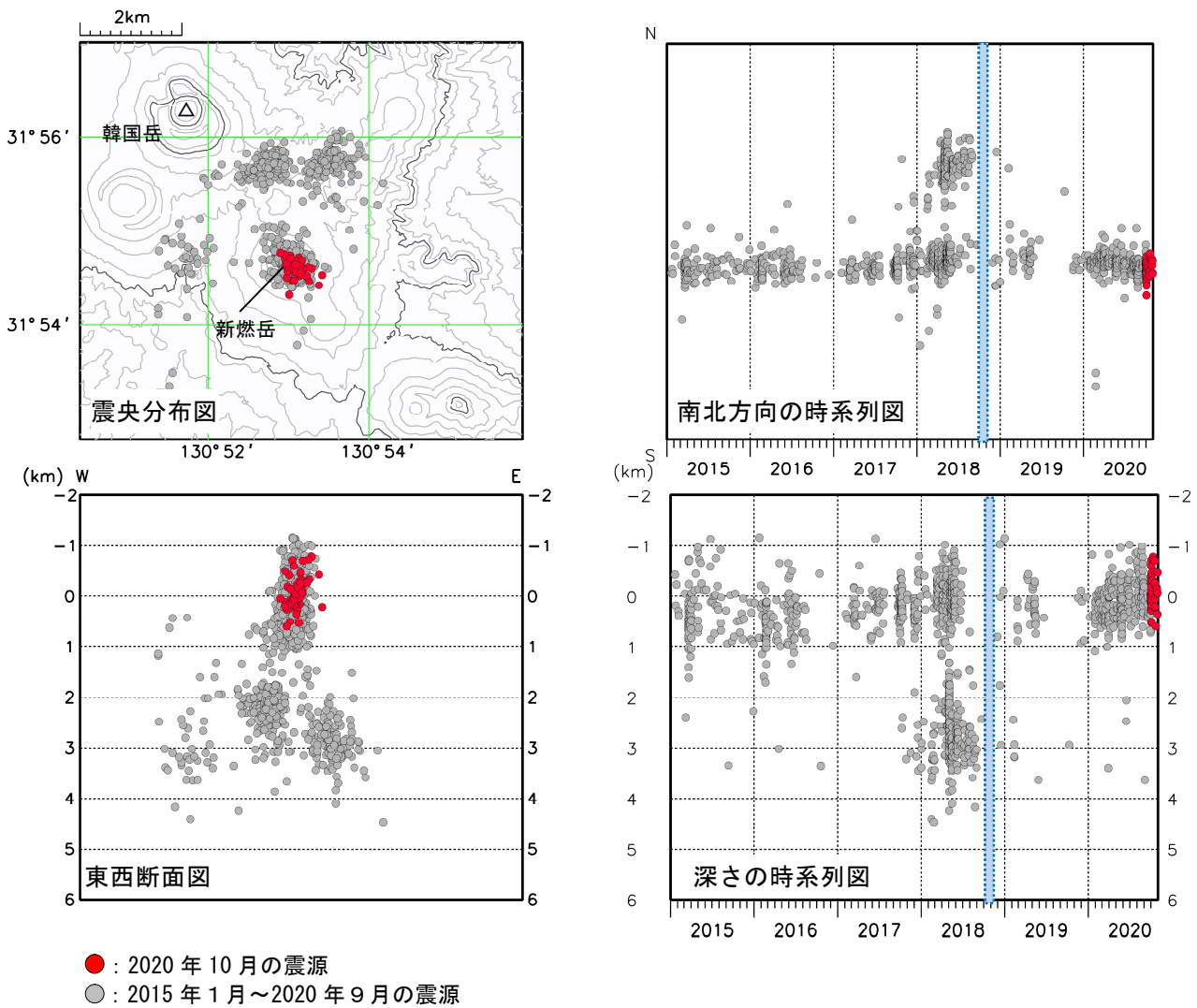
図8 霧島山（新燃岳）震源分布図（2015年1月～2020年10月）
