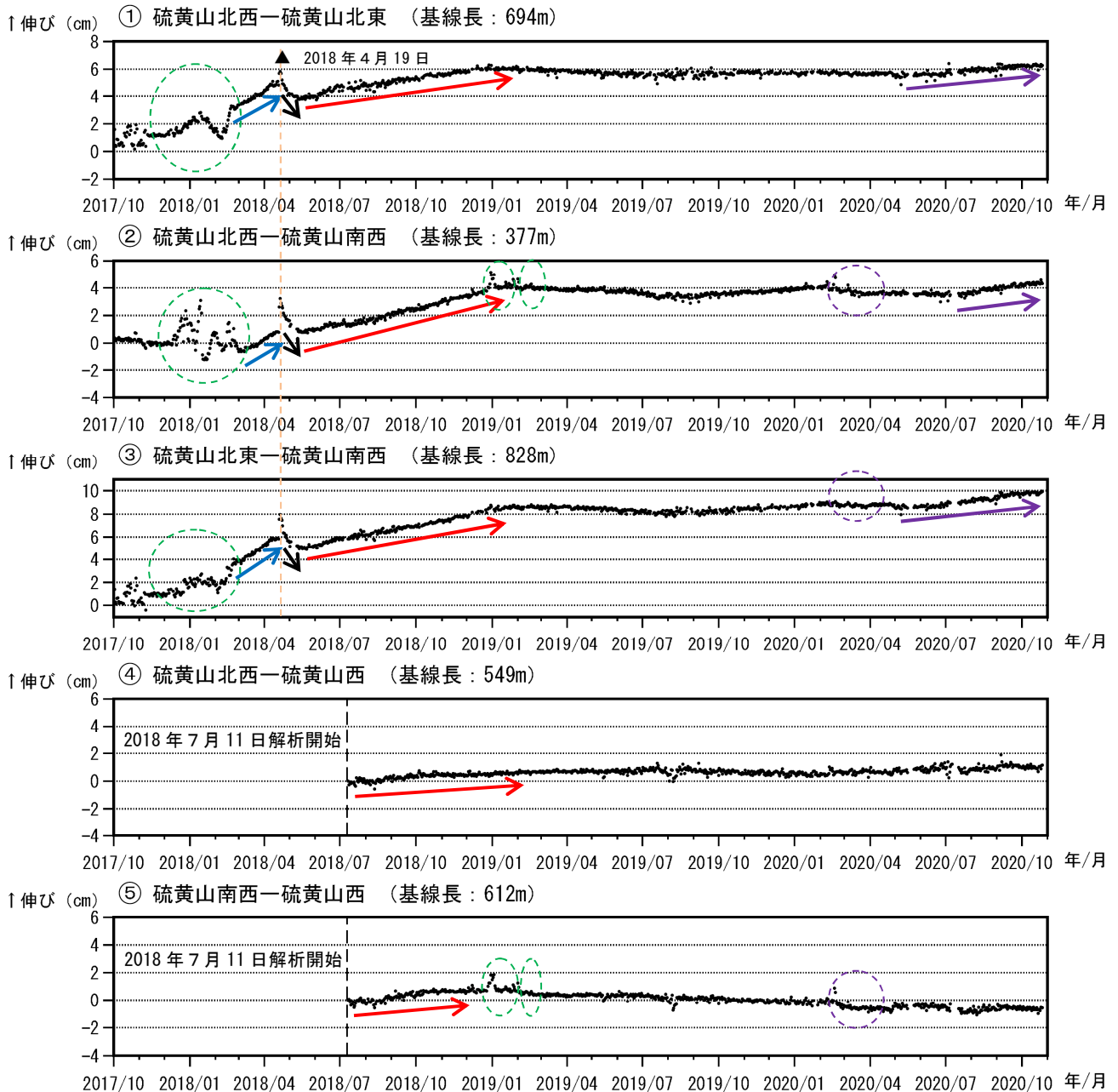
図9 霧島山（えびの高原（硫黄山）周辺） GNSS 連続観測による基線長変化 （2017年10月～2020年10月）
