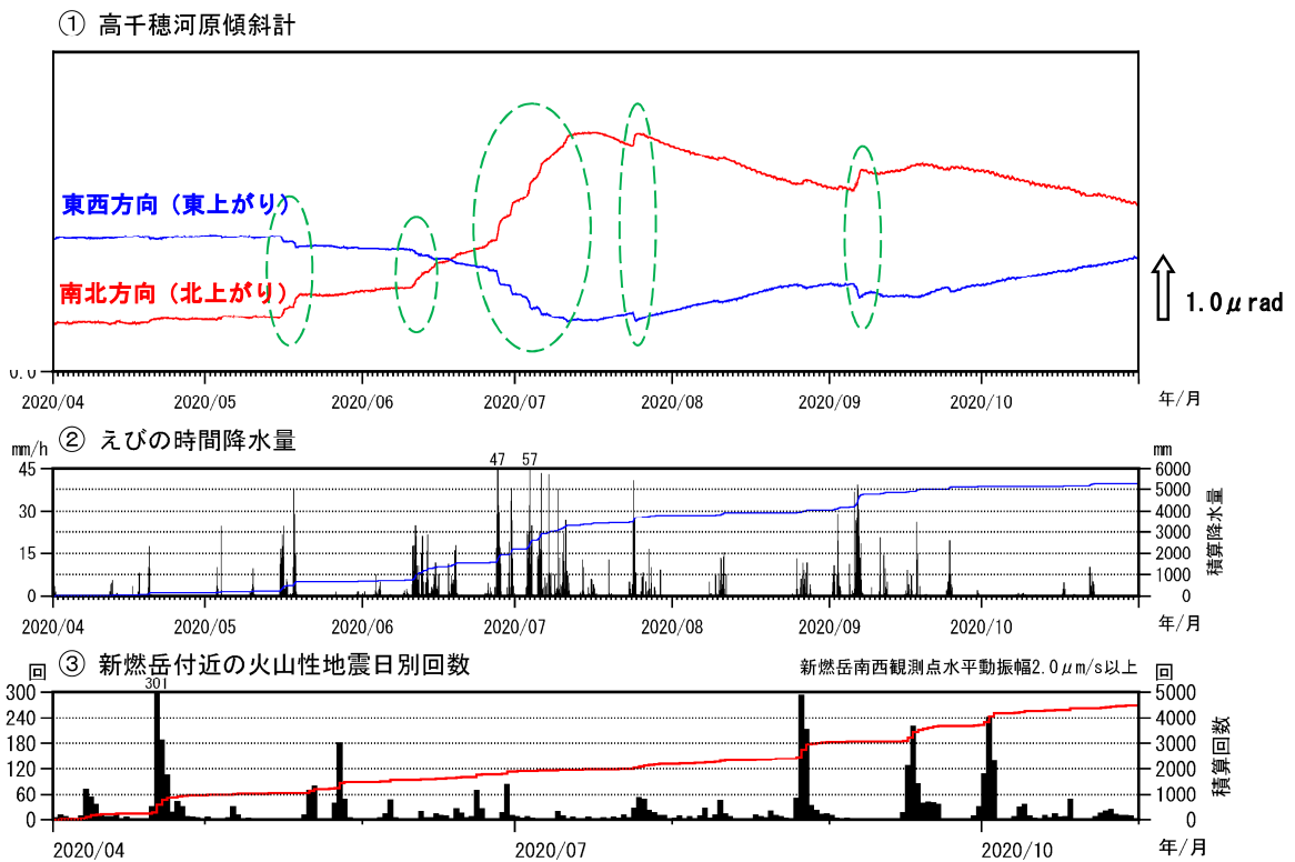
図7 霧島山（新燃岳） 高千穂河原観測点の傾斜変動の状況（2020年4月～2020年10月）
