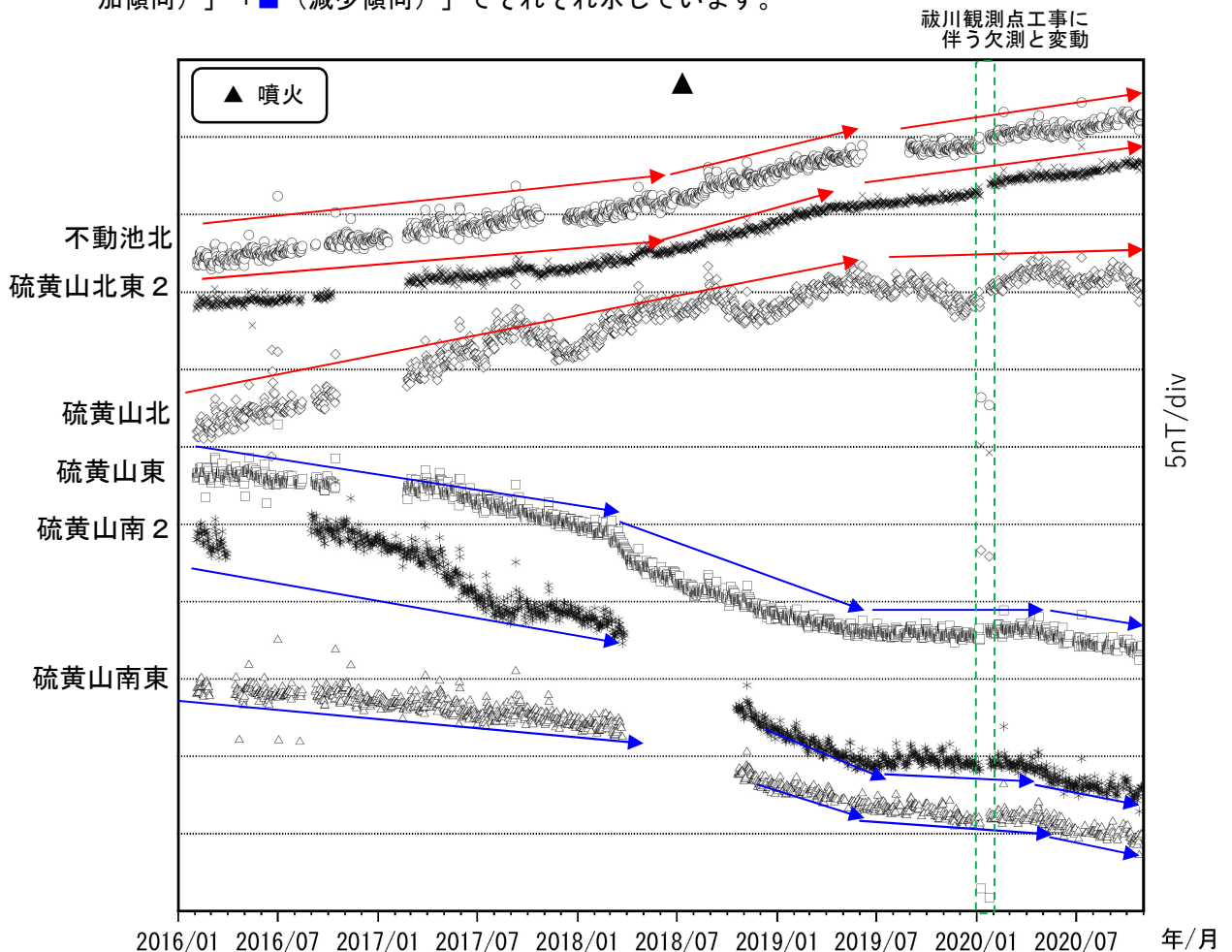
図14 霧島山（えびの高原（硫黄山）周辺） 全磁力観測点で観測された全磁力変動（2016年2月～2020年10月）
