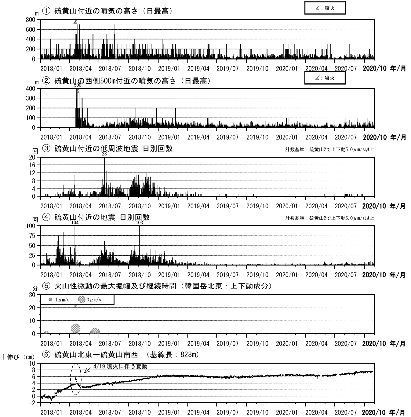
図7 霧島山（えびの高原（硫黄山）周辺） 火山活動経過図（2018年1月～2020年10月）
