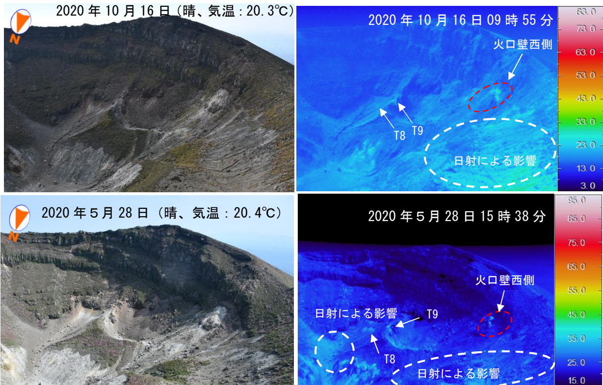
図 2-2 霧島山 (御鉢) 火口内の状況 (定点 1 (火口縁北西側) から観測)
