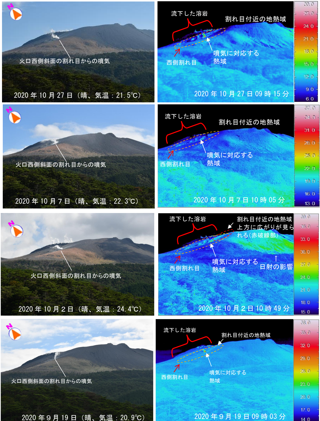
図 3-2 霧島山（新燃岳） 新燃岳南西側斜面の状況（新湯温泉付近から観測）
