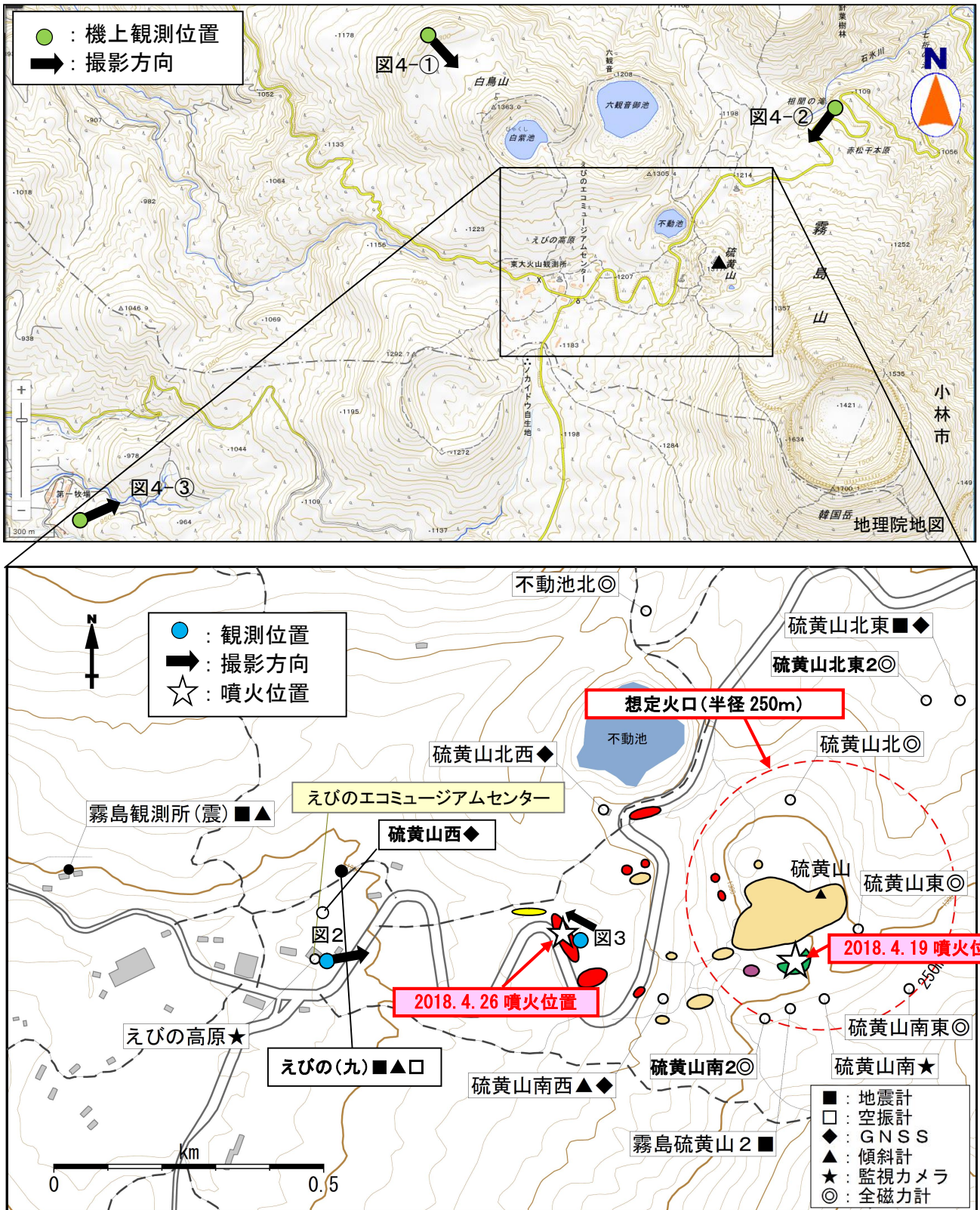
図5 霧島山（えびの高原（硫黄山）周辺） 図2～4の観測位置及び観測方向、噴火位置、主な噴気地帯及び地熱域
