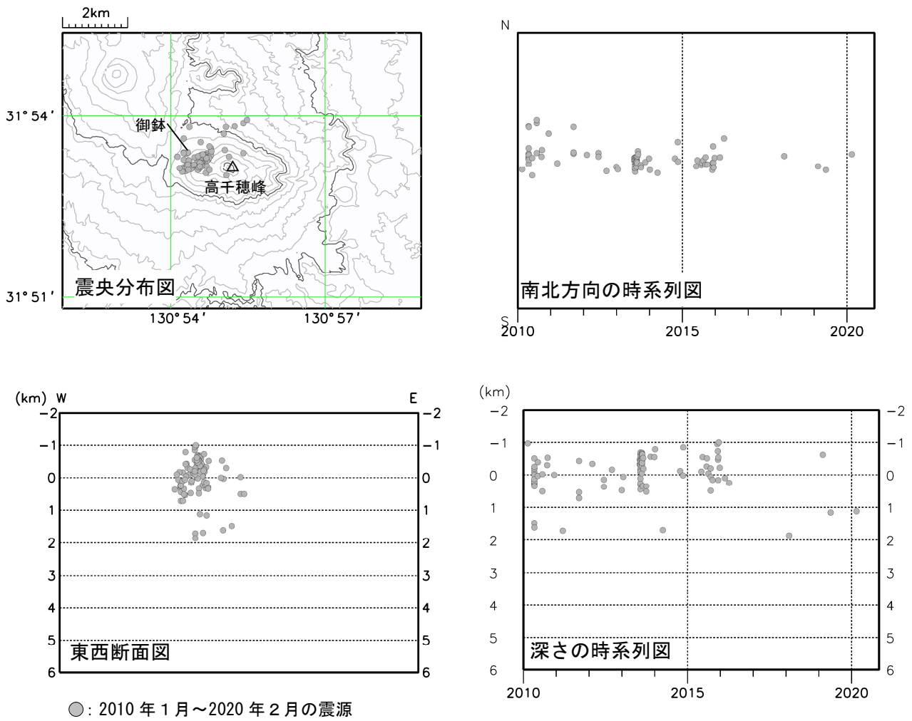
図7 霧島山（御鉢） 震源分布図（2010年1月～2020年10月）
