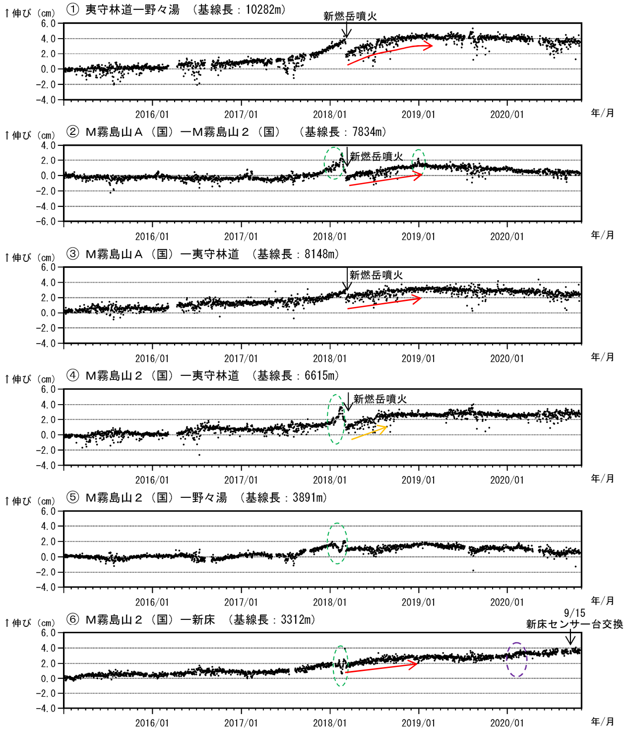
図10 霧島山（えびの高原（硫黄山）周辺） GNSS連続観測による基線長変化 (2015年1月～2020年10月)
