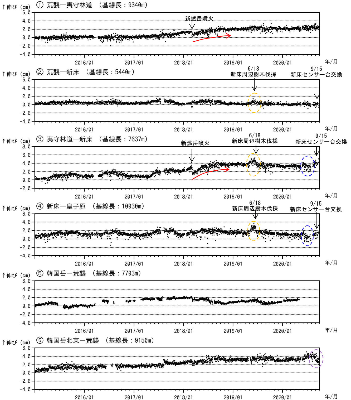
図 9-1 霧島山（新燃岳） GNSS 連続観測による基線長変化（2015 年 1 月～2020 年 9 月）
