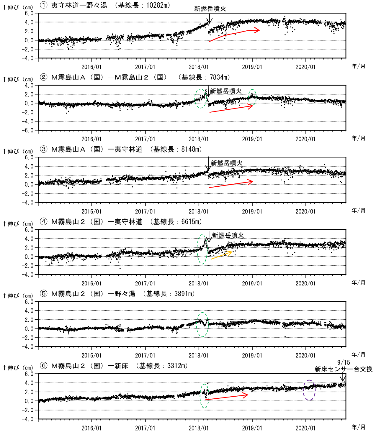
図 10 霧島山（えびの高原（硫黄山）周辺） GNSS 連続観測による基線長変化 (2015年1月～2020年9月)
