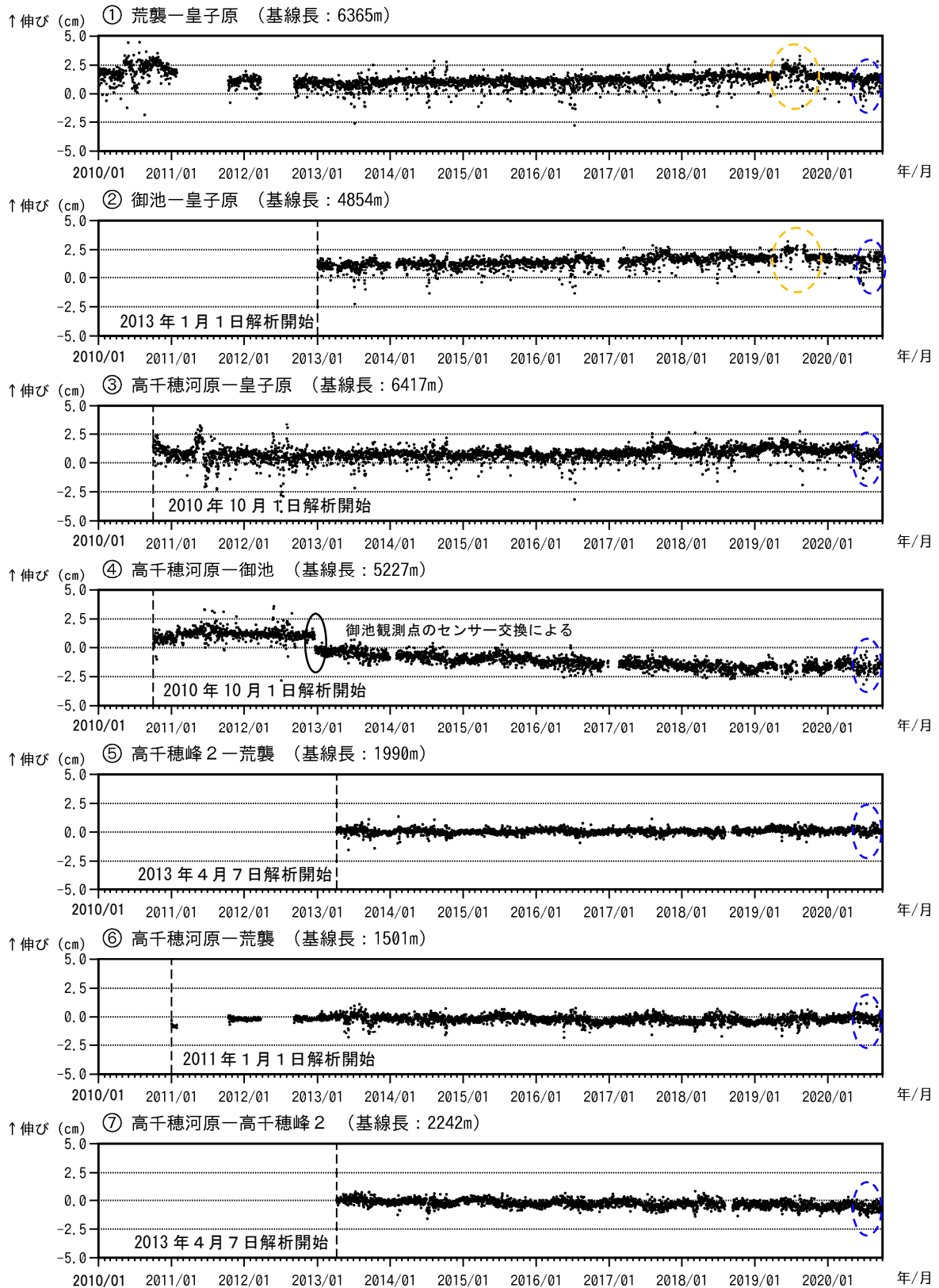
図4 霧島山（御鉢） GNSS 連続観測による基線長変化（2010年1月～2020年9月）
