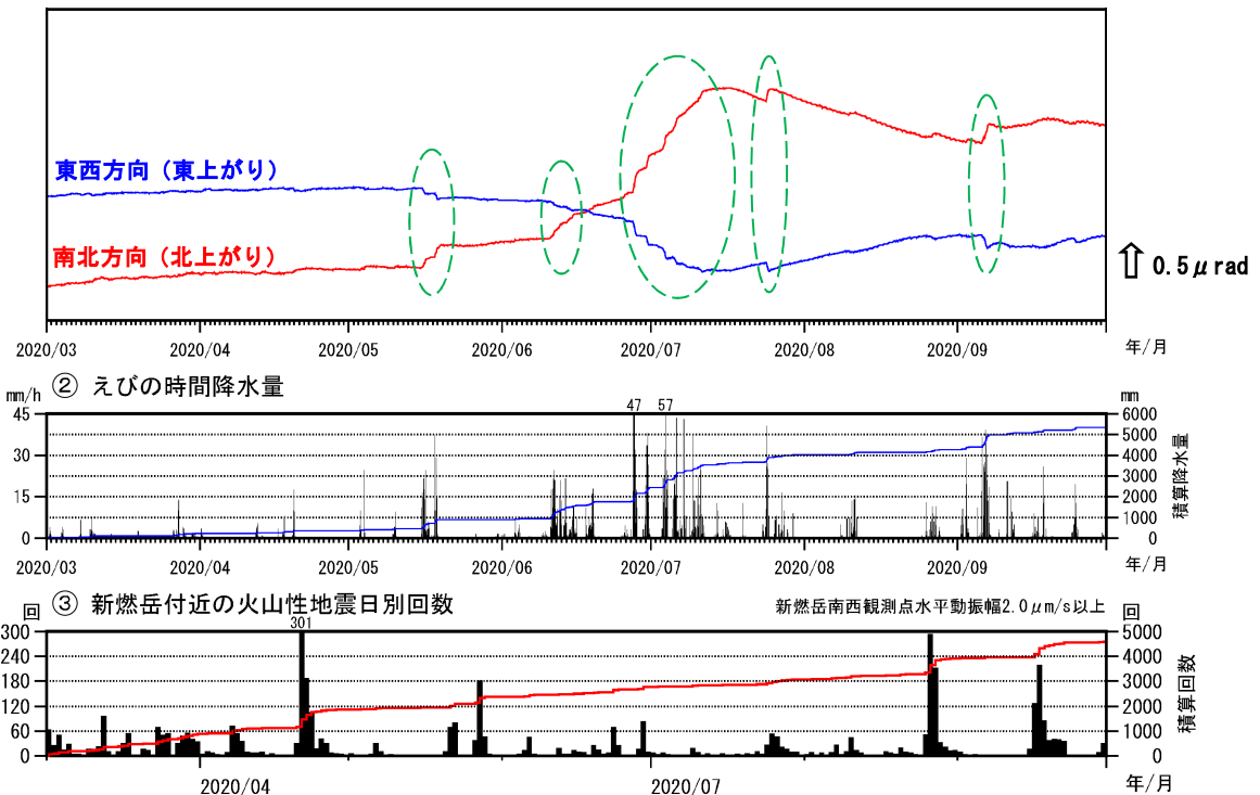
図7 霧島山（新燃岳） 高千穂河原観測点の傾斜変動の状況（2020年3月～2020年9月）
