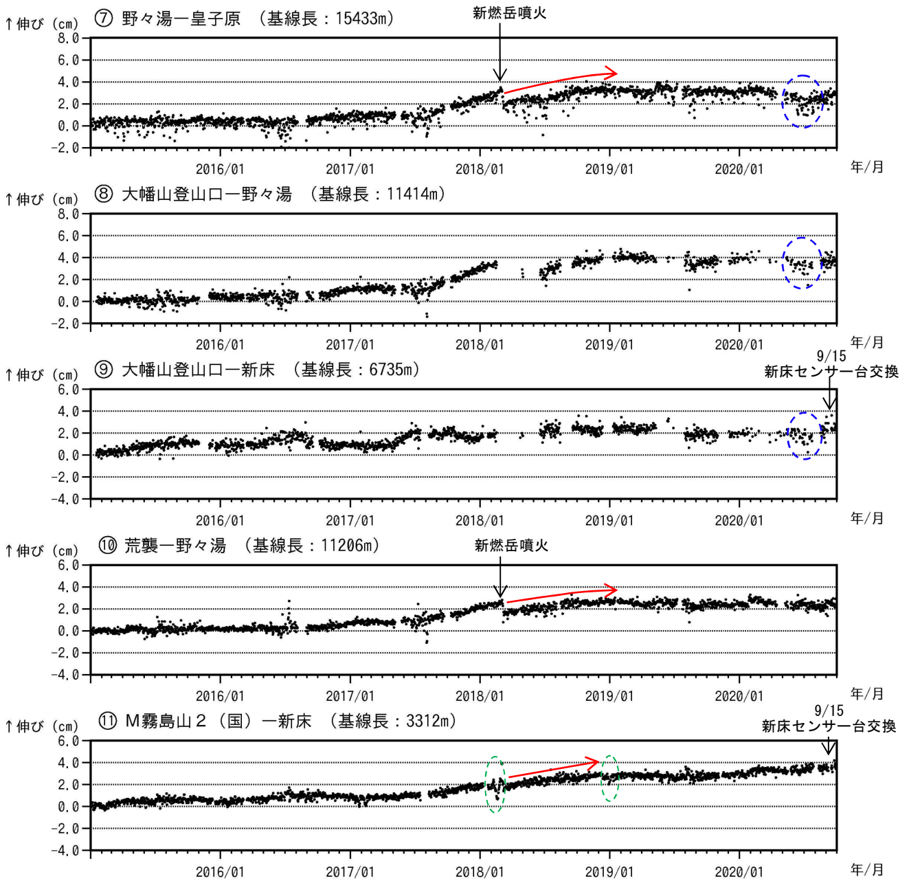
図 9-2 霧島山（新燃岳） GNSS 連続観測による基線長変化（2015 年 1 月～2020 年 9 月）
