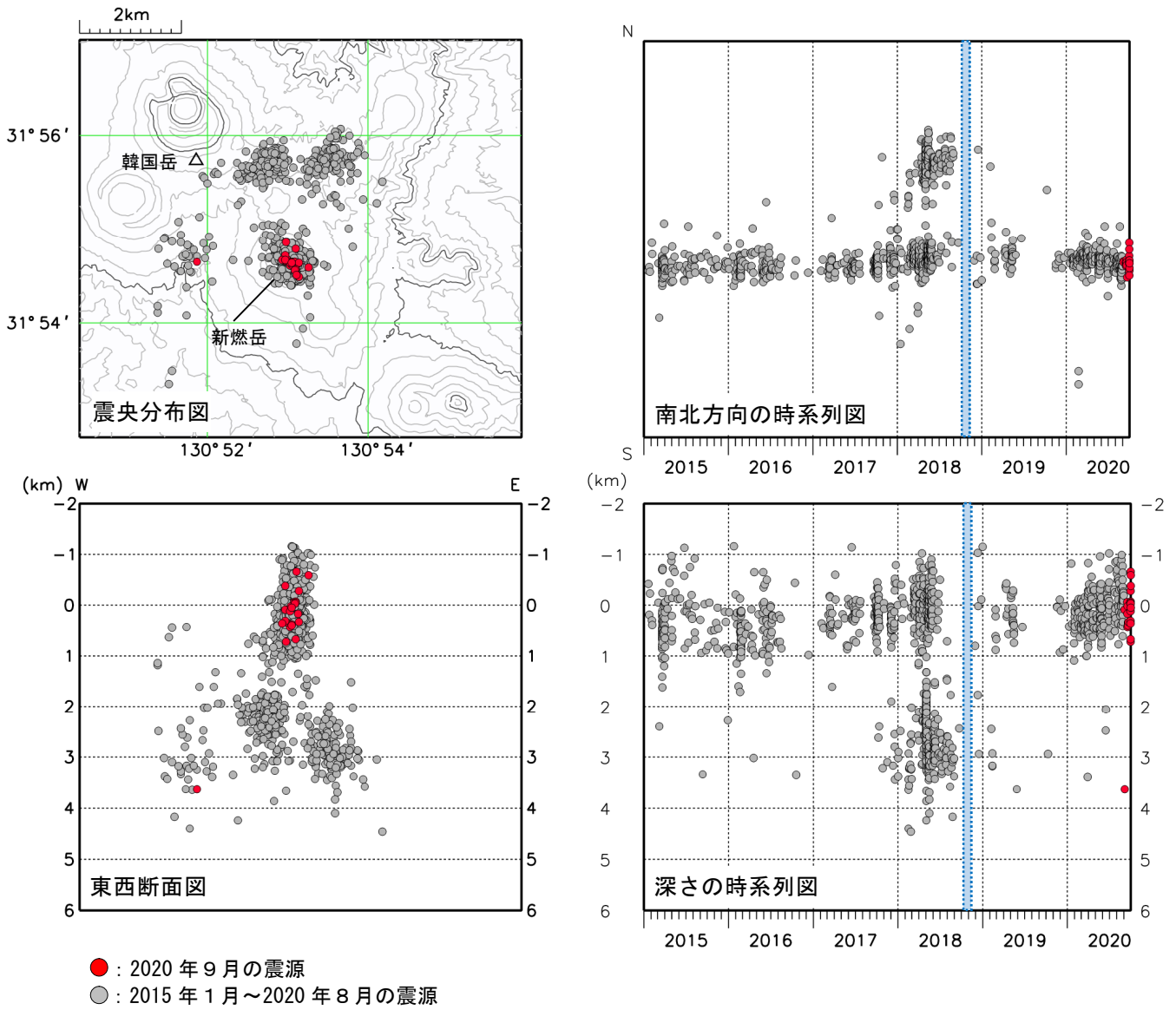
図8 霧島山（新燃岳） 震源分布図（2015年1月～2020年9月）
