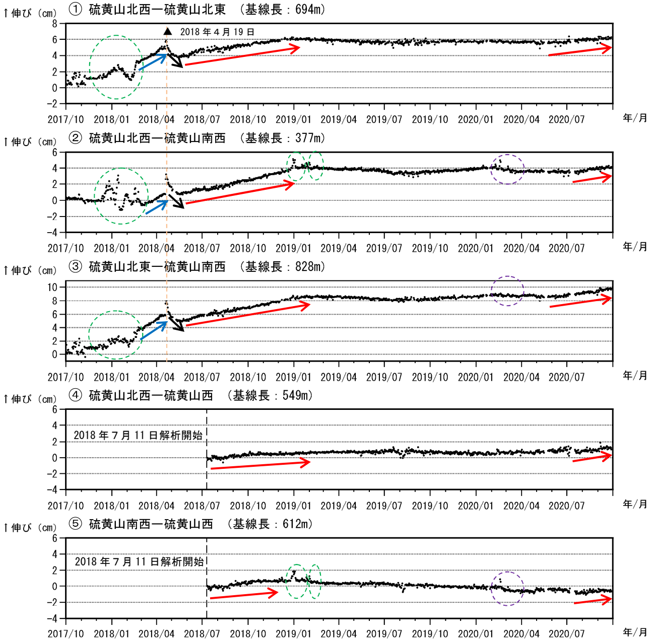
図9 霧島山（えびの高原（硫黄山）周辺） GNSS 連続観測による基線長変化 （2017年10月～2020年9月）
