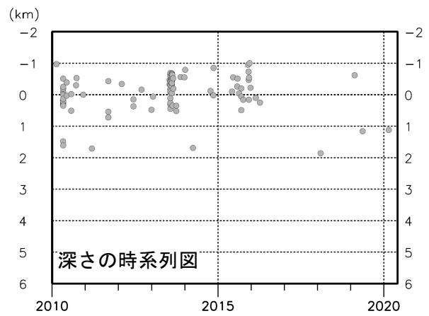
図5 霧島山（御鉢） 震源分布図（2010年1月～2020年5月）
