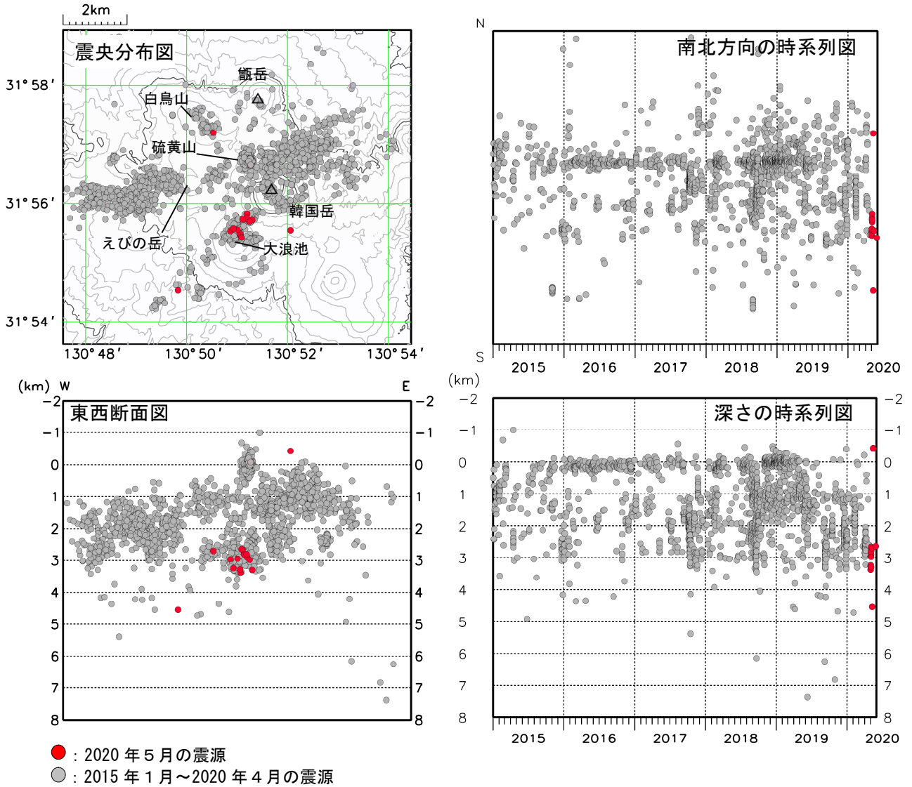
図4 霧島山（えびの高原（硫黄山）周辺） 震源分布図（2015年1月～2020年5月）
