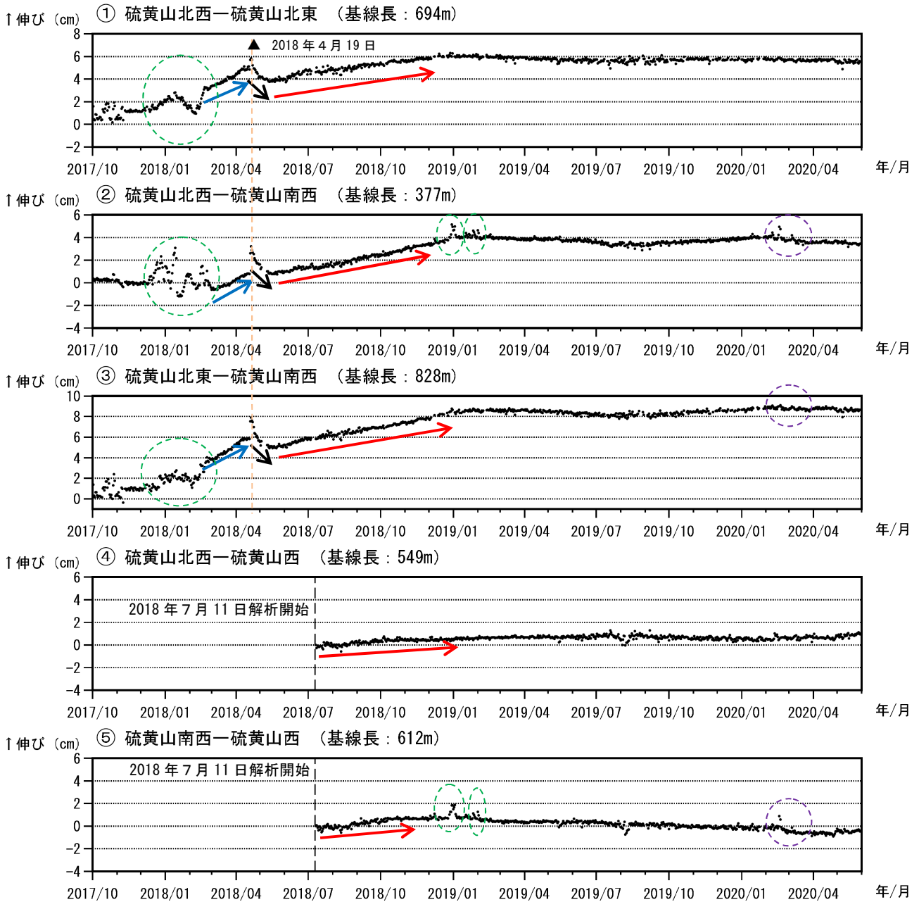
図7 霧島山（えびの高原（硫黄山）周辺） GNSS 連続観測による基線長変化 （2017年10月～2020年5月）
