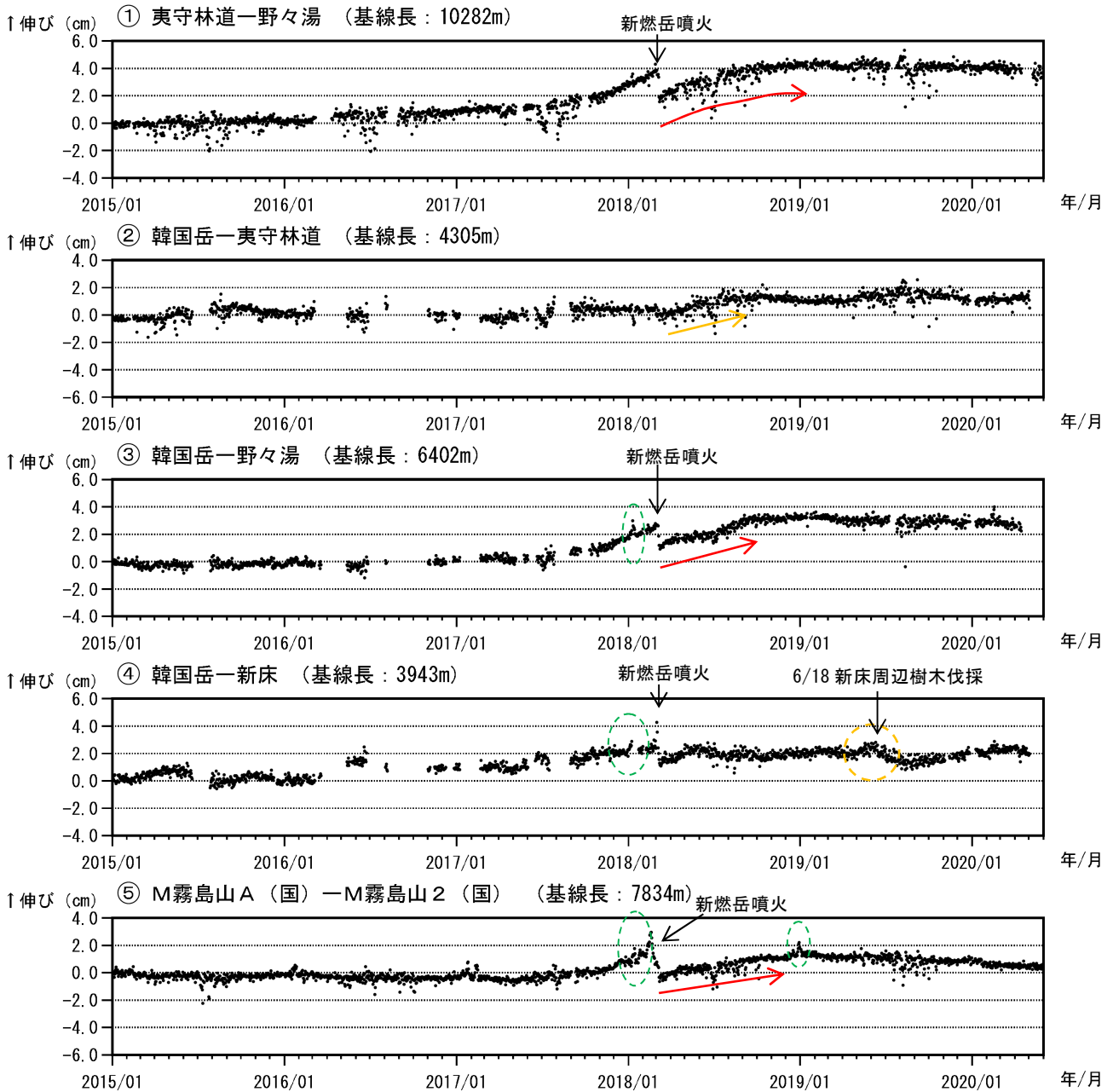
図 8-1 霧島山（えびの高原（硫黄山）周辺） GNSS 連続観測による基線長変化 (2015年1月～2020年5月)
