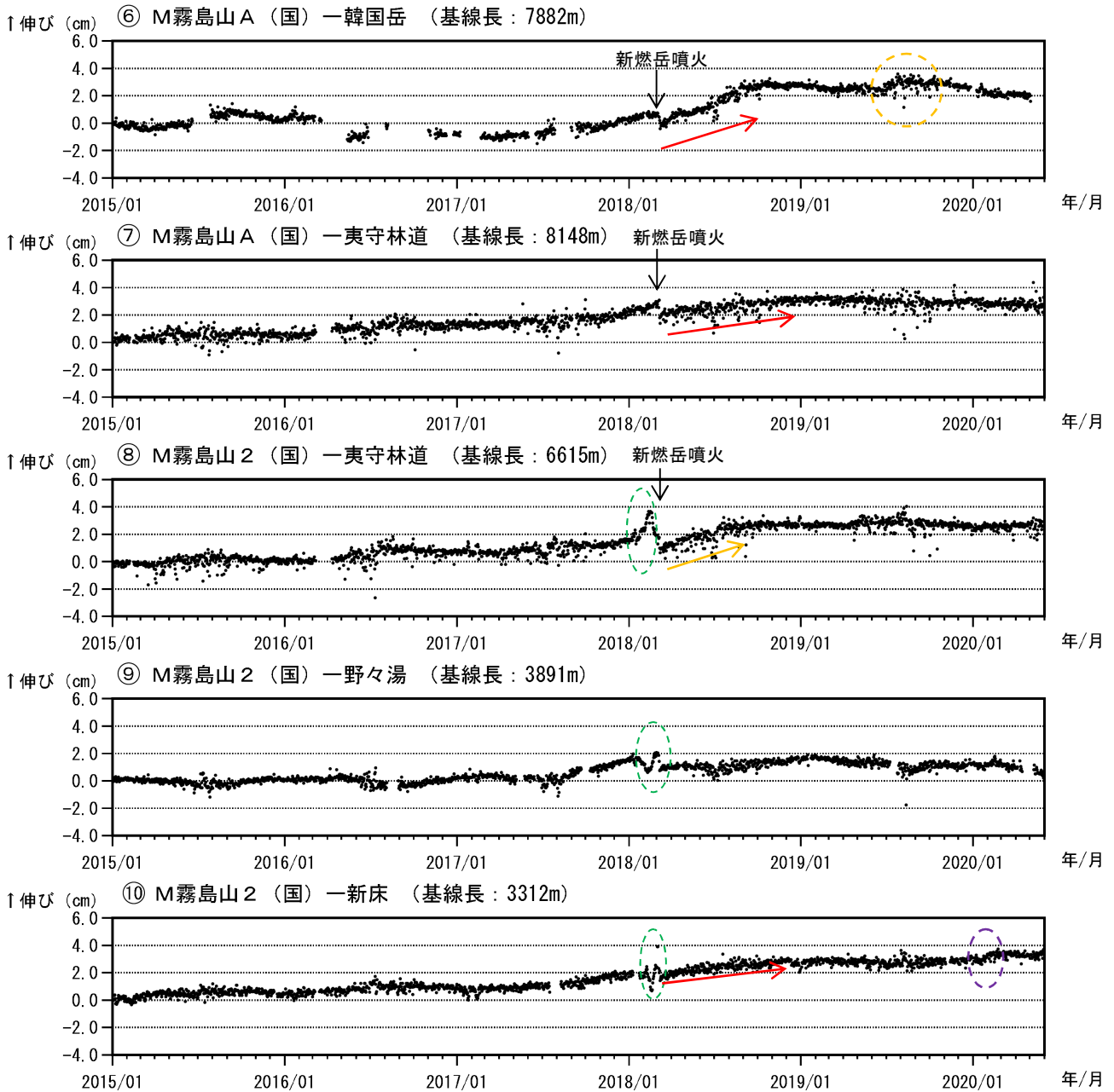
図 8-2 霧島山（えびの高原（硫黄山）周辺） GNSS 連続観測による基線長変化 (2015年1月～2020年5月)
