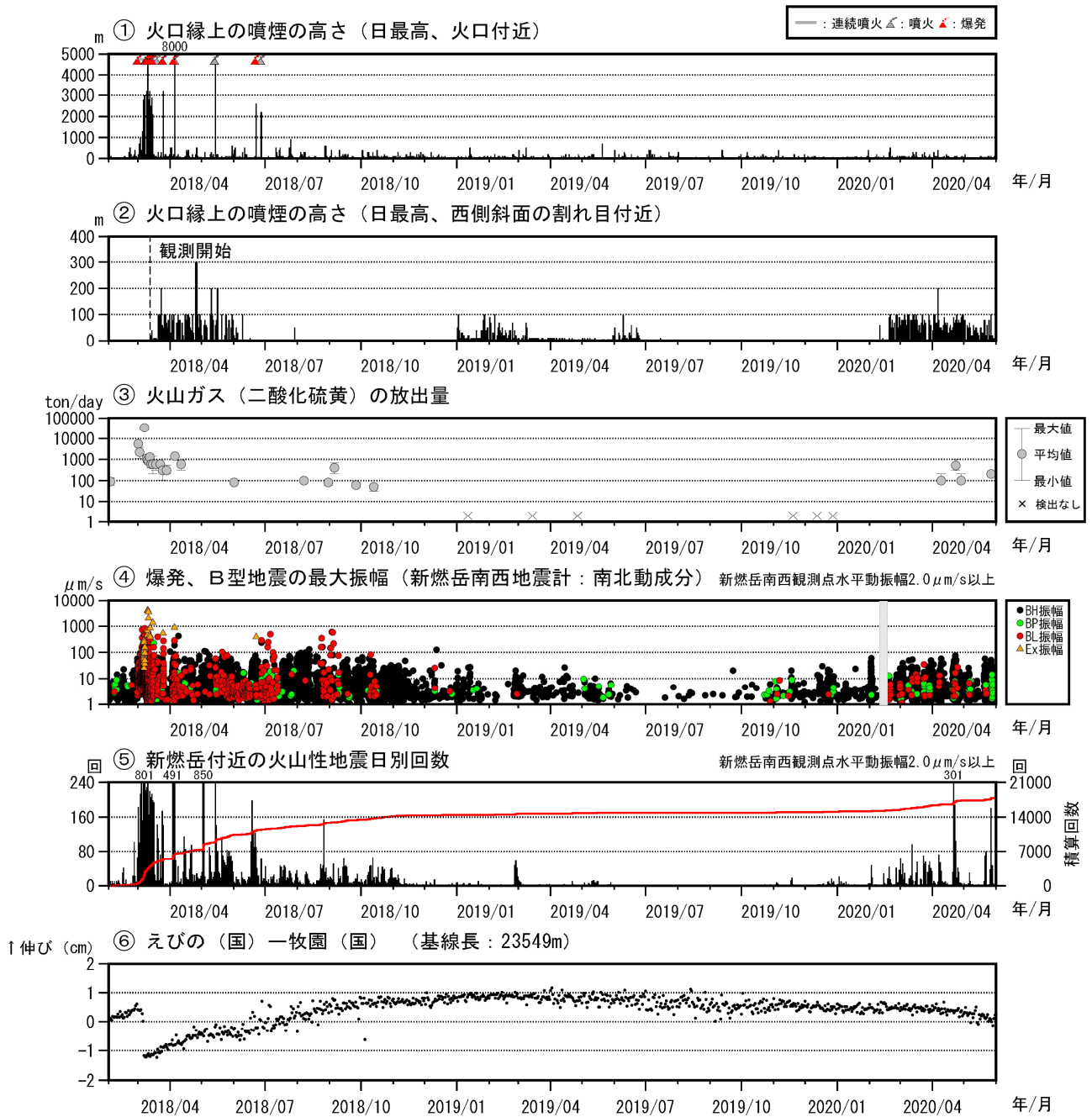
図4 霧島山（新燃岳） 火山活動経過図（2018年2月～2020年5月）
