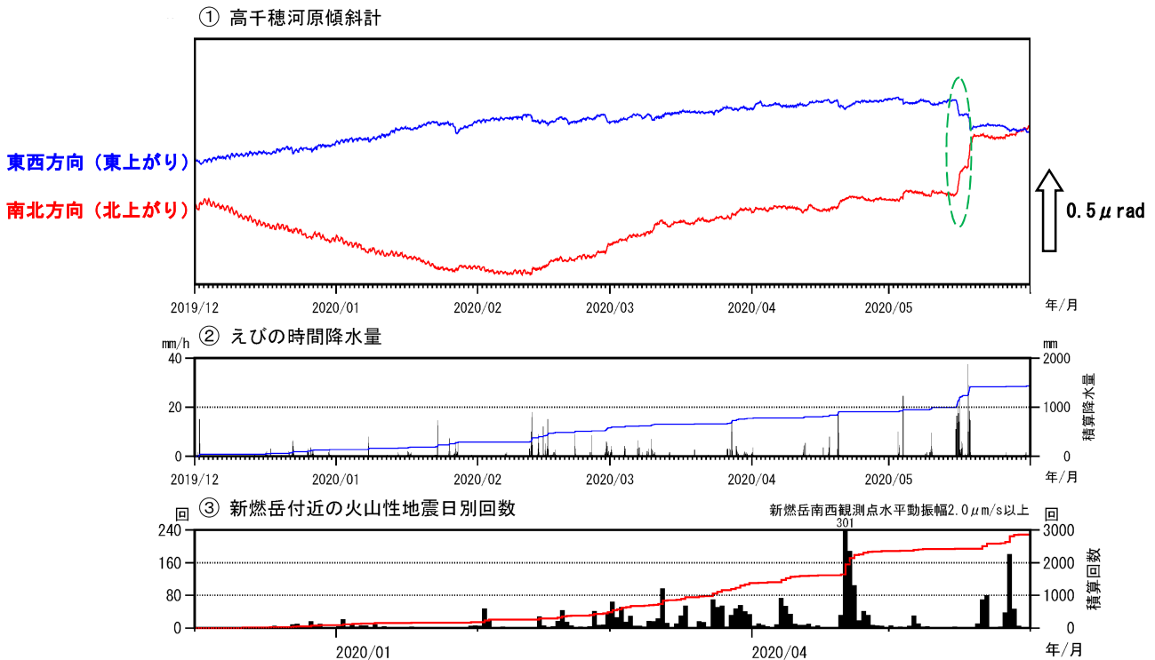
図6 霧島山（新燃岳） 高千穂河原観測点の傾斜変動の状況（2019年12月～2020年5月）
