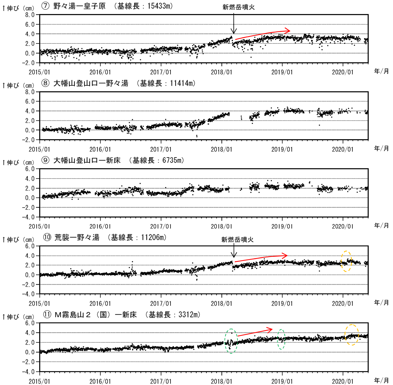
図 8-2 霧島山（新燃岳） GNSS 連続観測による基線長変化（2015 年 1 月～2020 年 5 月）
