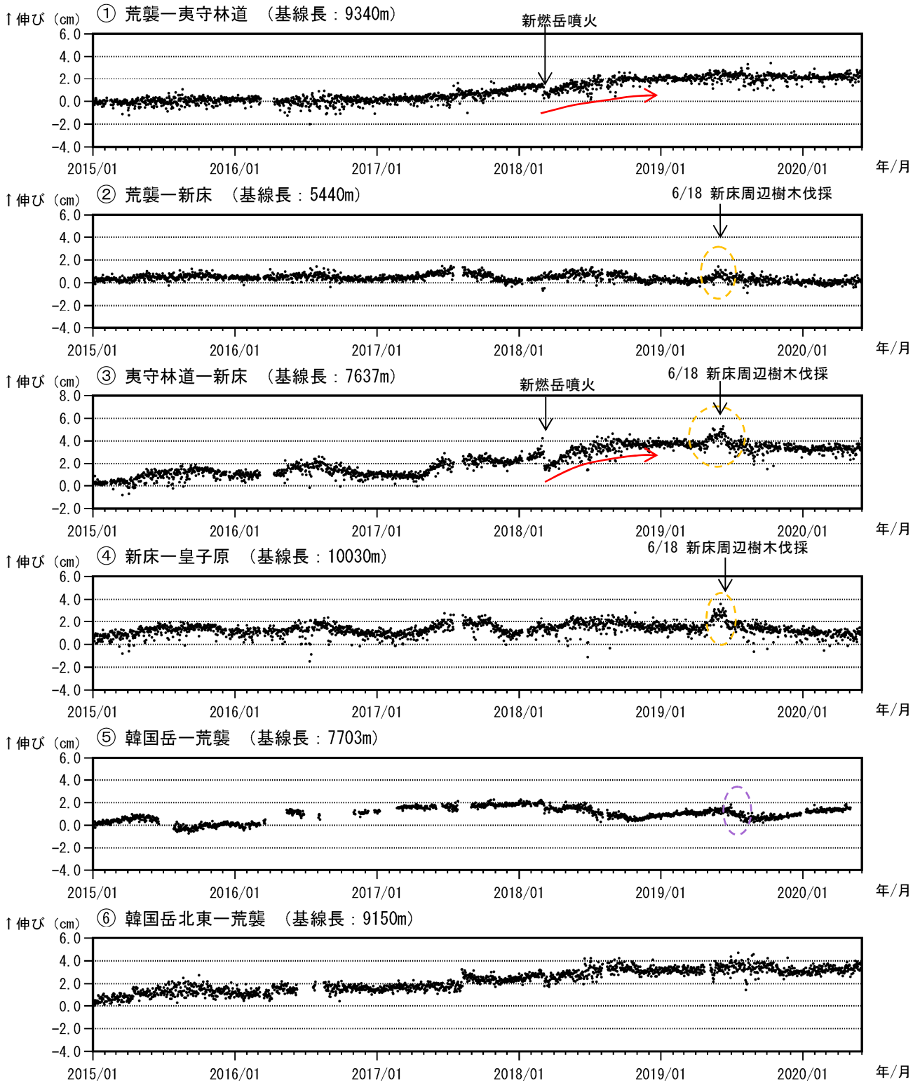
図 8-1 霧島山（新燃岳） GNSS 連続観測による基線長変化（2015 年 1 月～2020 年 5 月）
