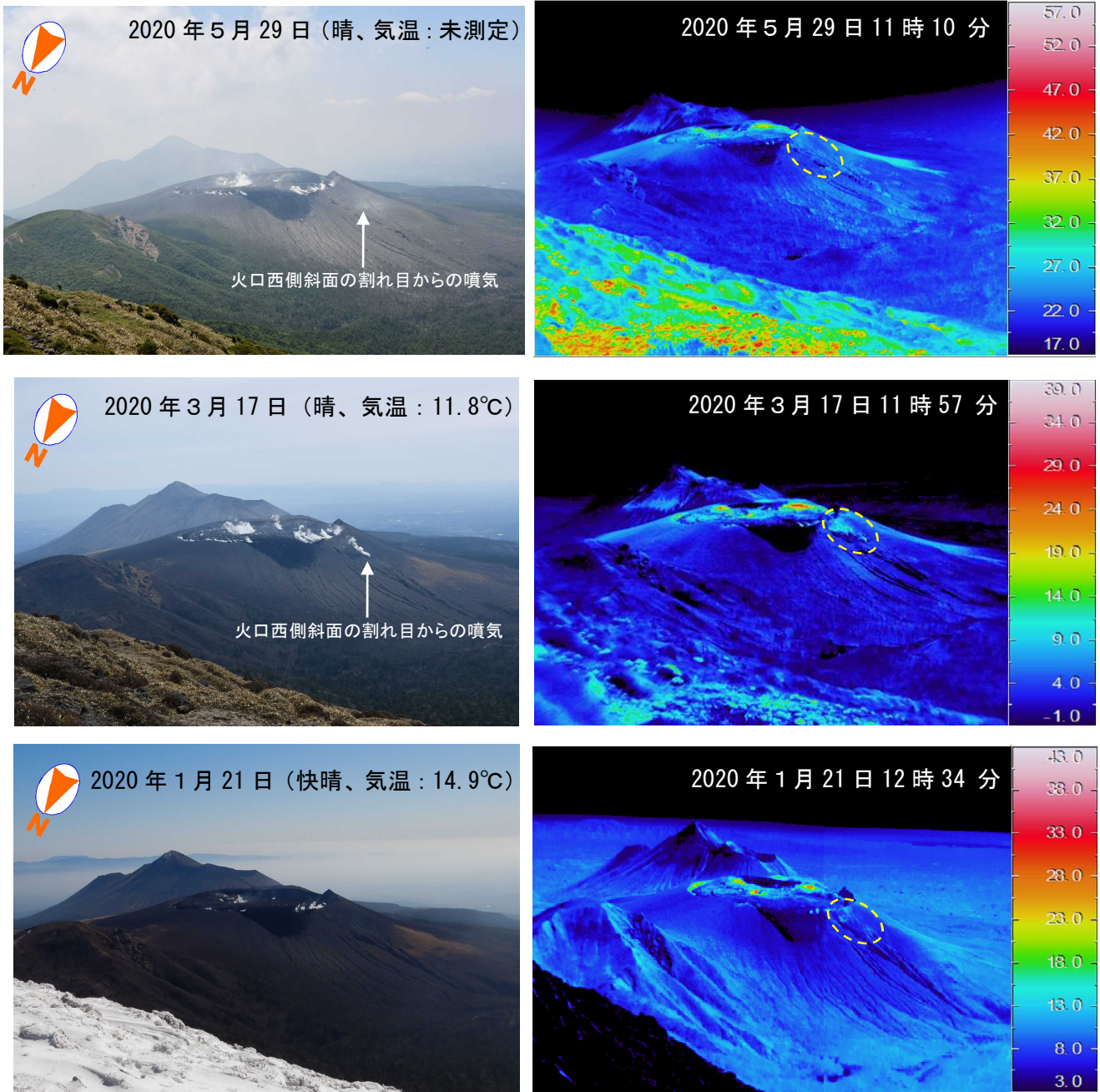
図 2-1 霧島山（新燃岳） 火口内及び西側斜面の状況（韓国岳から観測）
