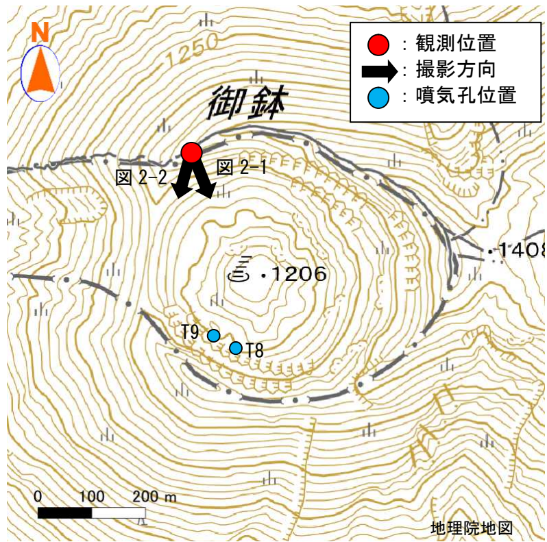
図3 霧島山（御鉢） 観測位置、撮影方向及び噴気孔位置
