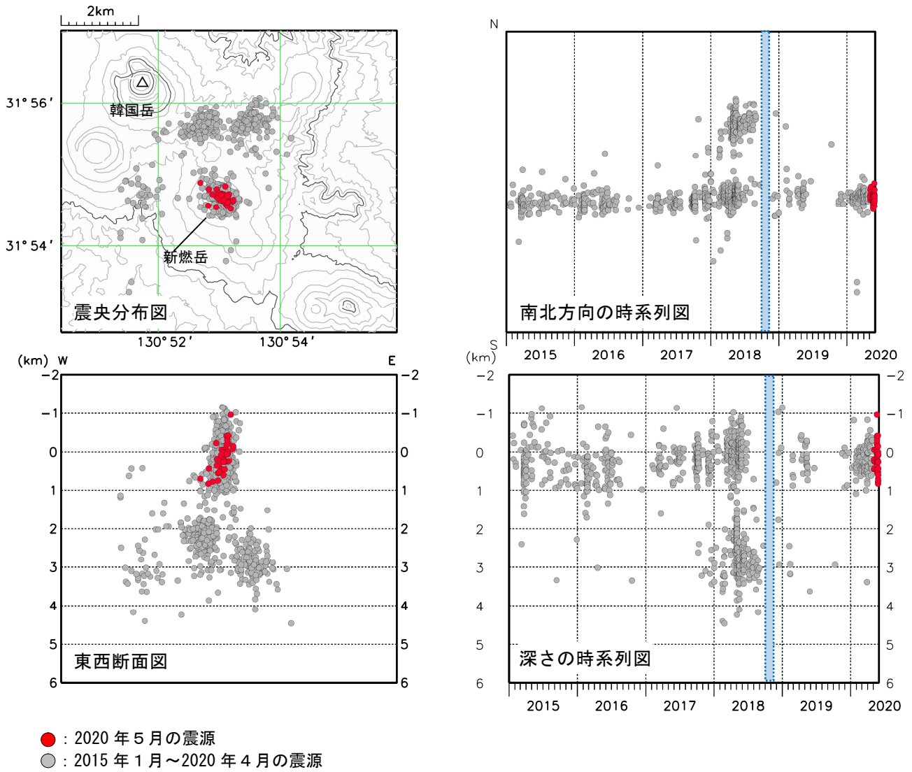
図7 霧島山（新燃岳） 震源分布図（2015年1月～2020年5月）
