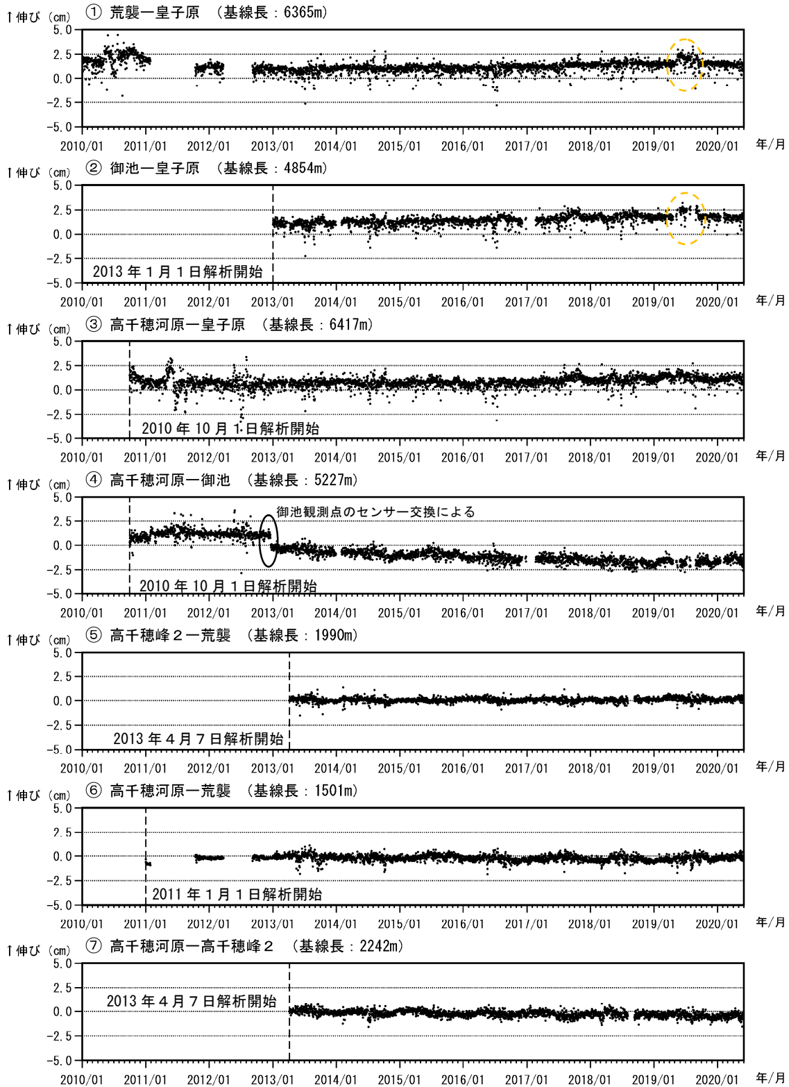
図6 霧島山（御鉢） GNSS 連続観測による基線長変化（2010年1月～2020年5月）
