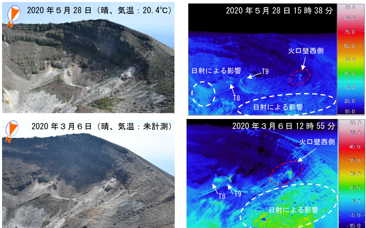
図 2-2 霧島山（御鉢） 火口内の状況（火口縁北西側から観測）
