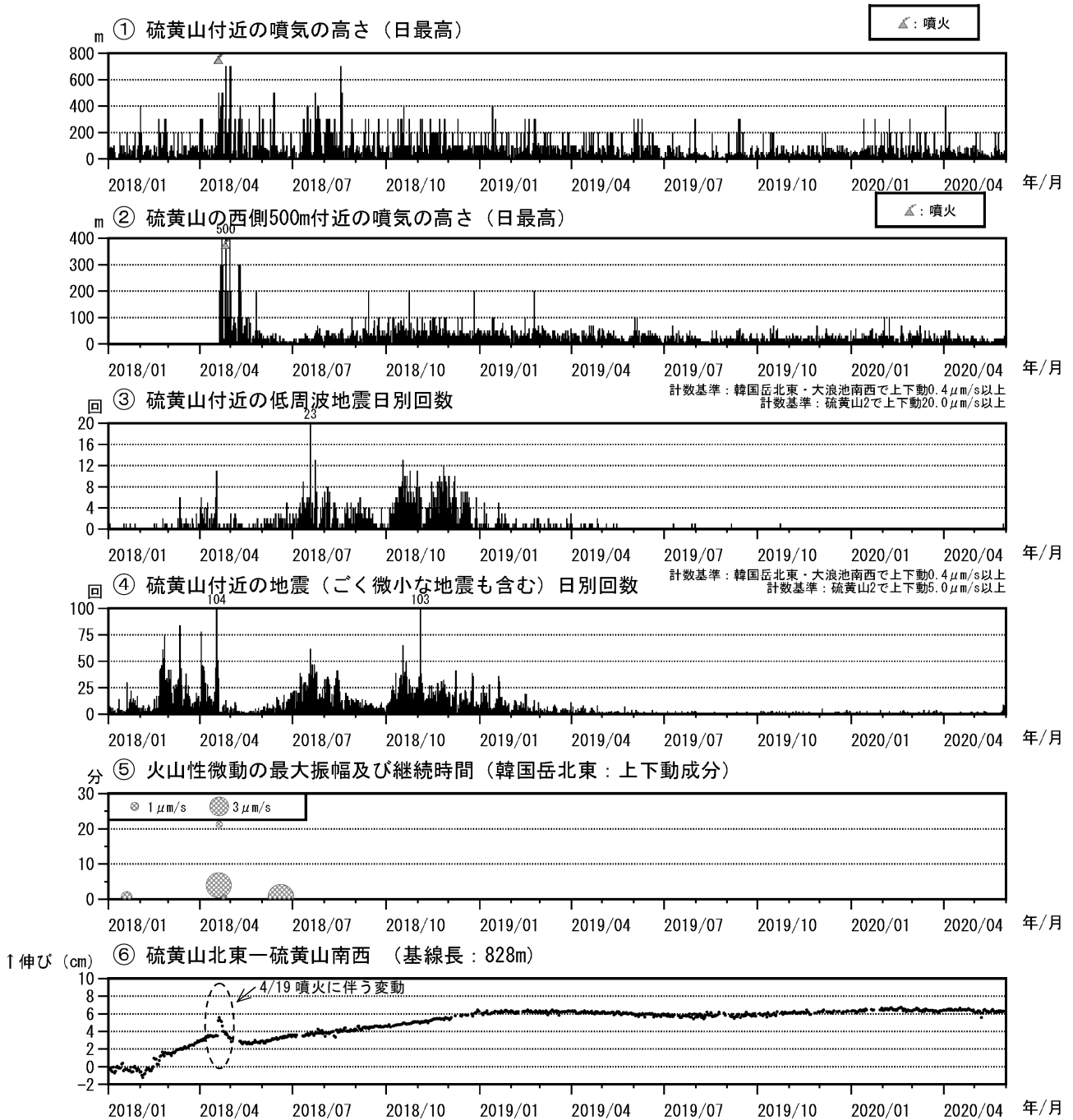
図5 霧島山（えびの高原（硫黄山）周辺） 火山活動経過図（2018年1月～2020年5月）
