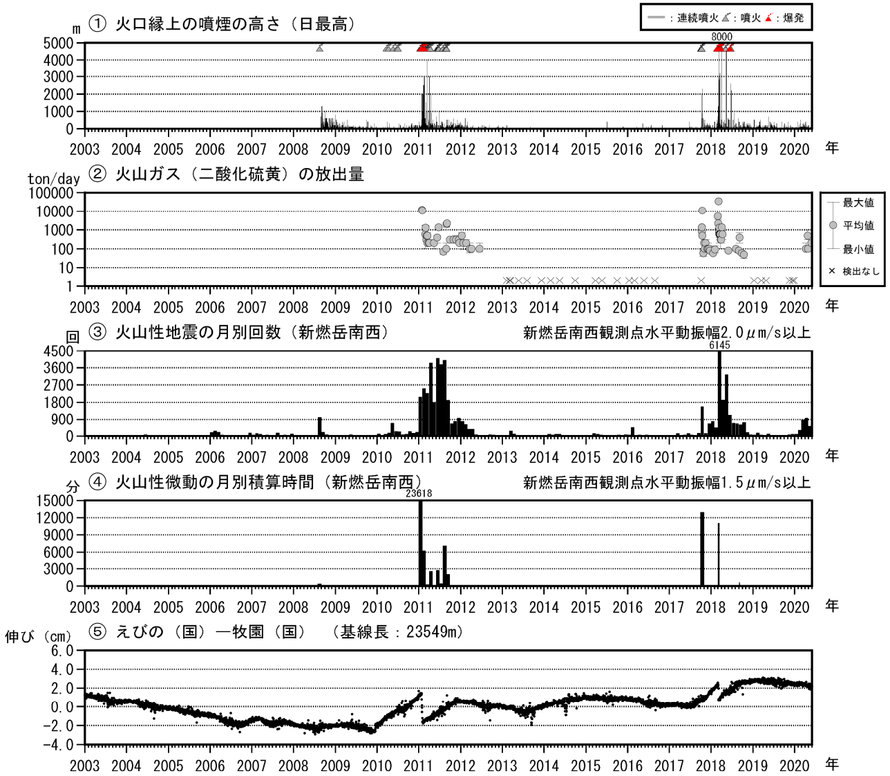
図3 霧島山（新燃岳） 火山活動経過図（2003年1月～2020年5月）
