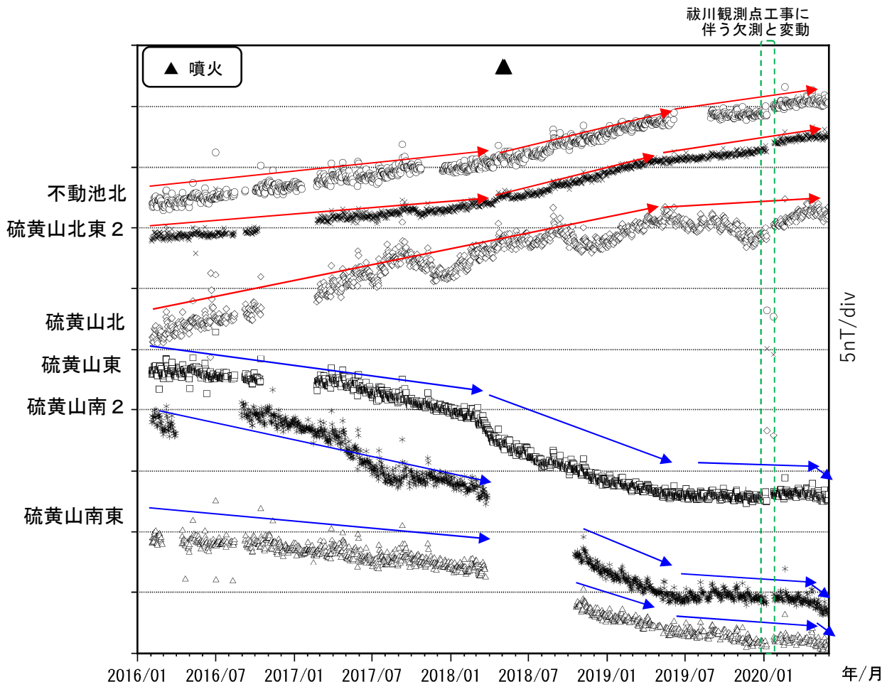
図 12 霧島山（えびの高原（硫黄山）周辺） 全磁力観測点で観測された全磁力変動（2016年2月～2020年5月）
