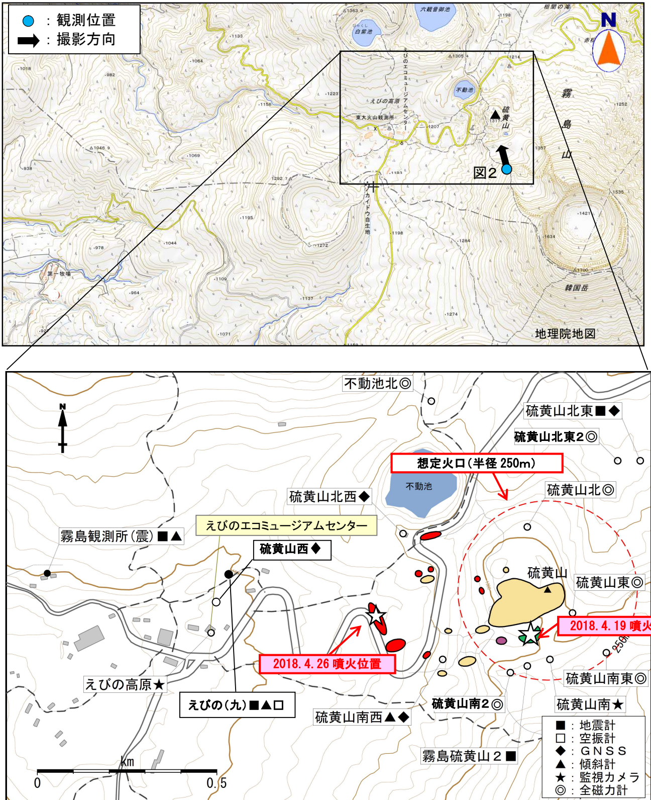
図3 霧島山（えびの高原（硫黄山）周辺） 図2の観測位置及び撮影方向（上段）、及び噴火位置、主な噴気地帯及び地熱域（下段）
