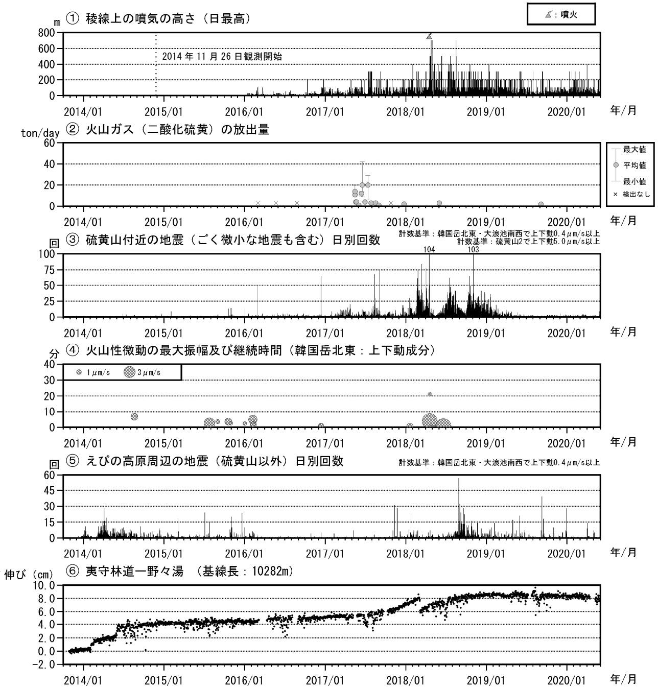
図6 霧島山（えびの高原（硫黄山）周辺）火山活動経過図（2014年1月～2020年5月）
