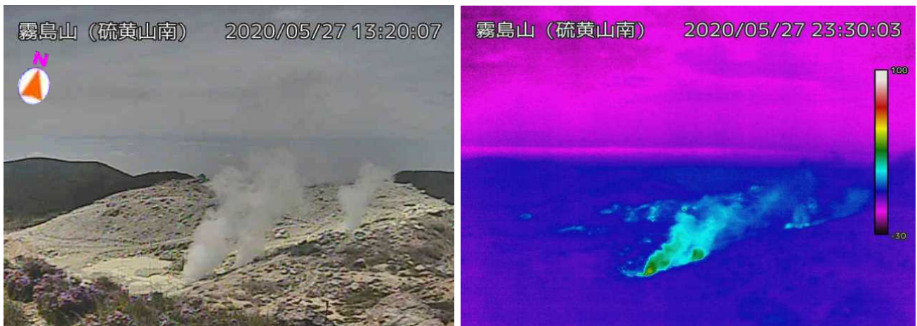
図 1-2 霧島山（えびの高原（硫黄山）周辺） 硫黄山南側の状況 （5月27日、硫黄山南監視カメラによる）
