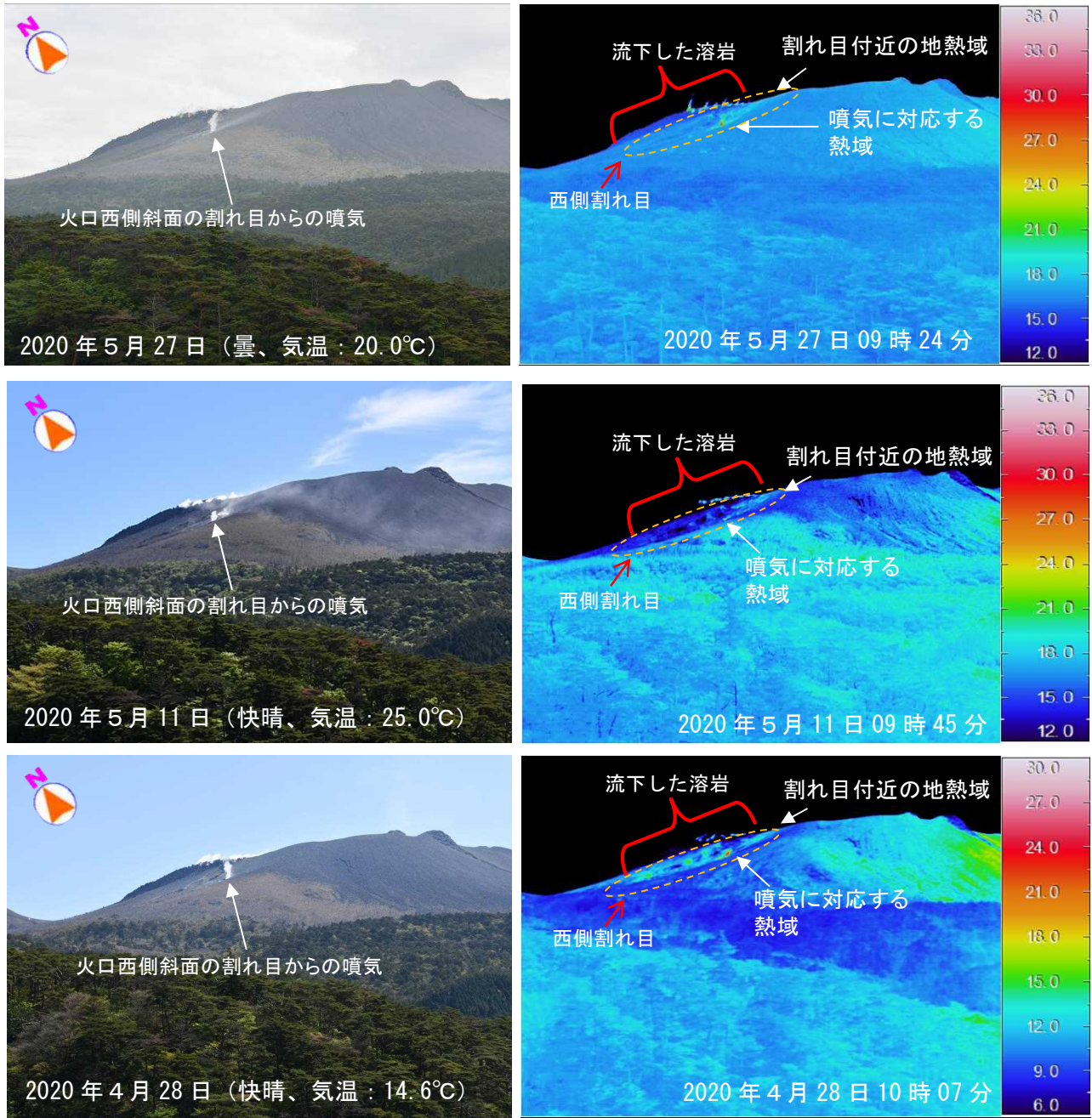
図 2-2 霧島山（新燃岳） 新燃岳南西側斜面の状況（新湯温泉付近から観測）
