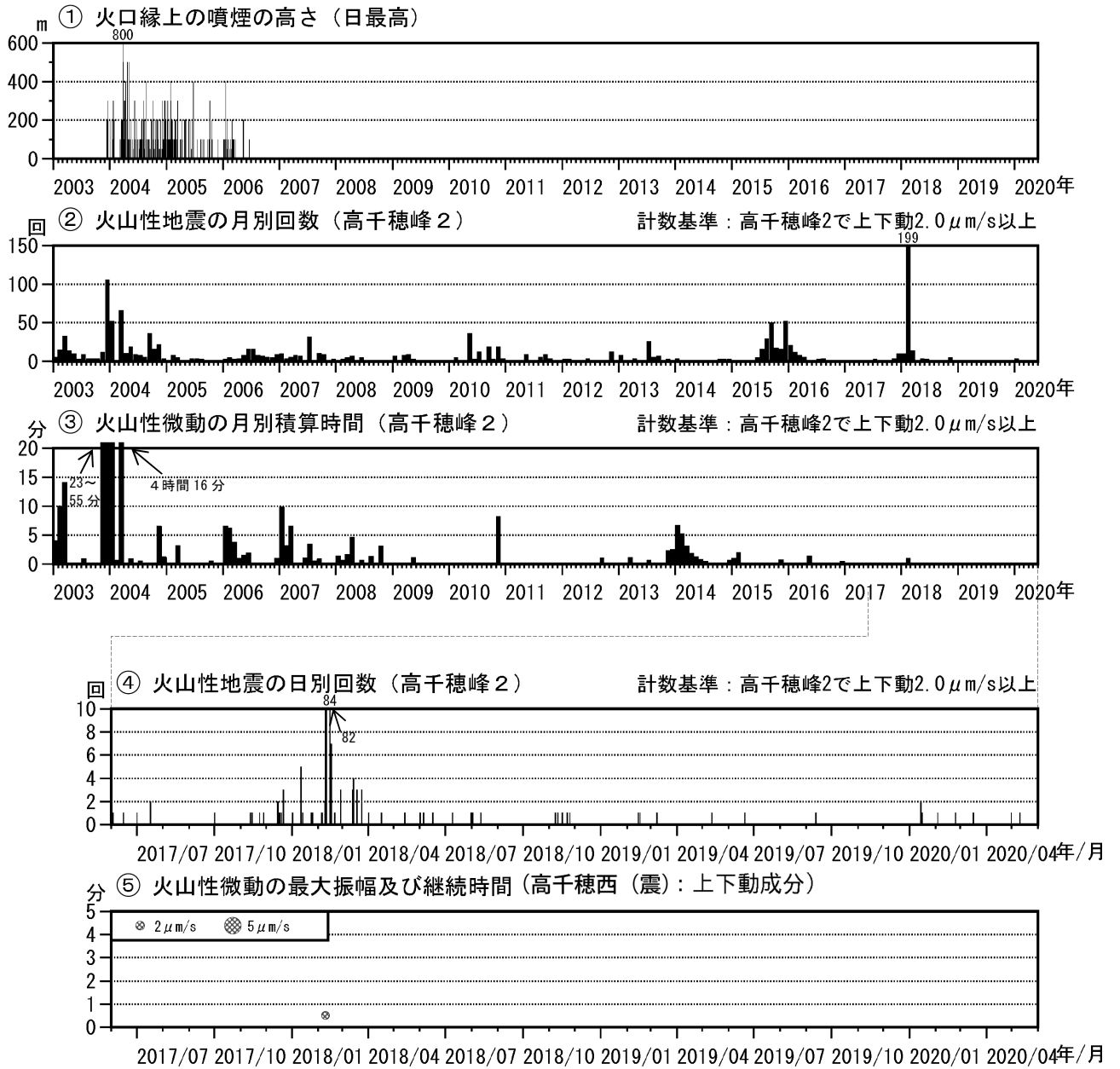
図4 霧島山（御鉢） 火山活動経過図（2003年1月～2020年5月）
