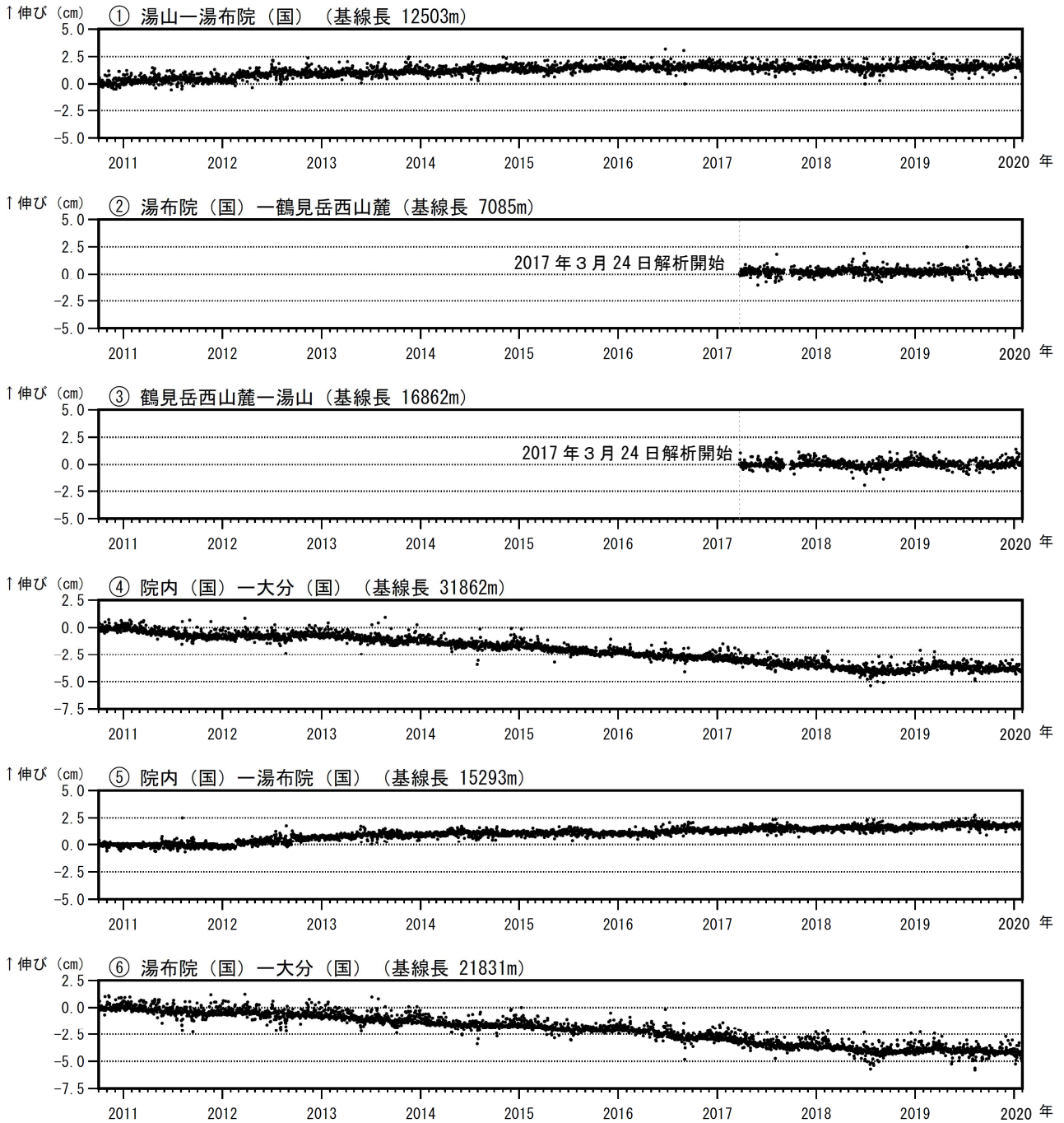
図4 鶴見岳・伽藍岳 GNSS連続観測による基線長変化（2010年10月～2020年1月）
