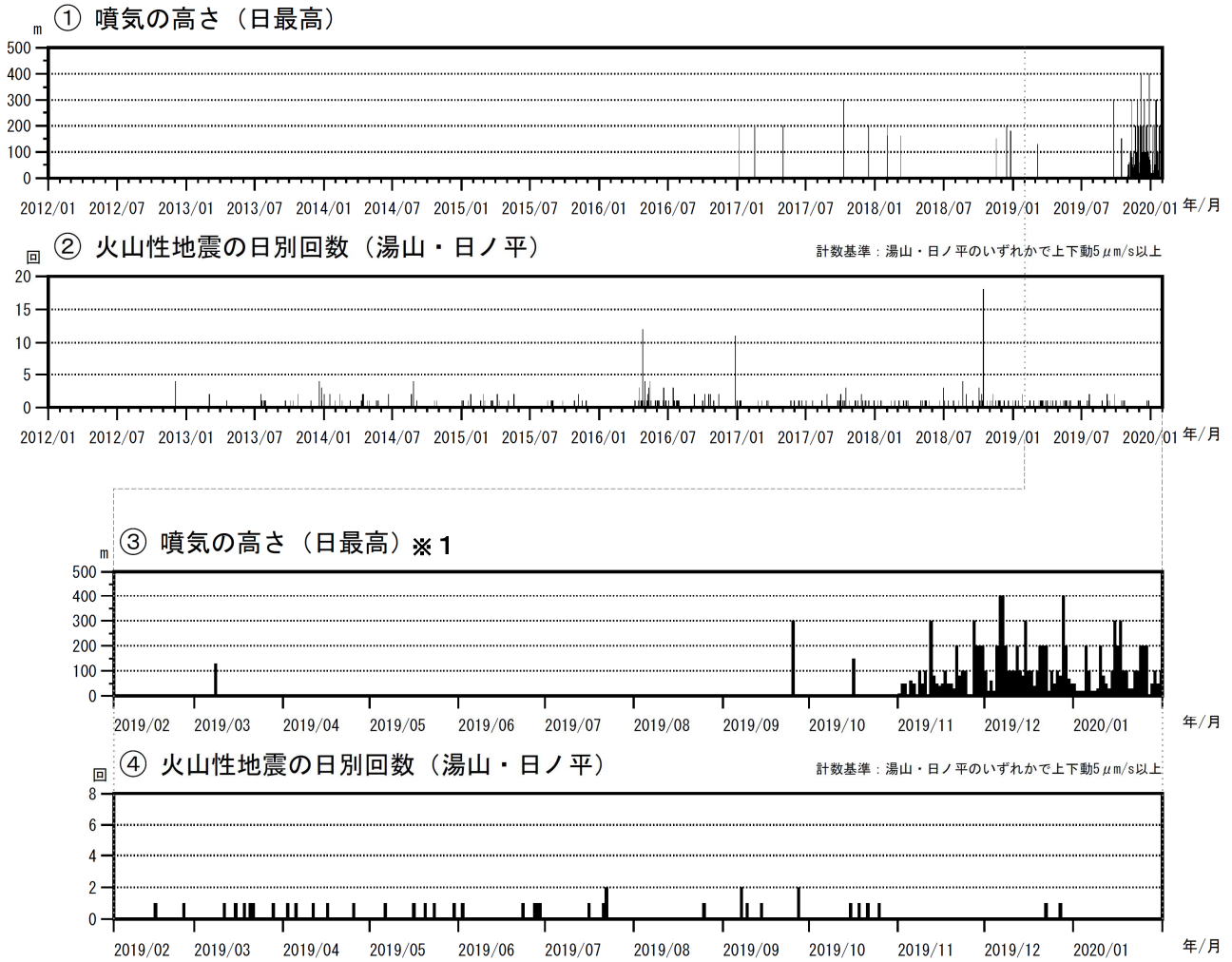
図2 鶴見岳・伽藍岳 火山活動経過図（2012年1月～2020年1月）
