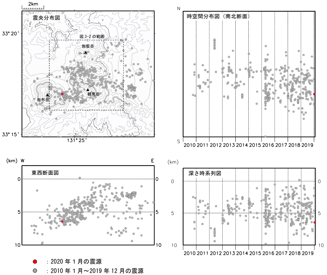
図3-1 鶴見岳・伽藍岳 震源分布図（広域）（2010年1月～2020年1月）
