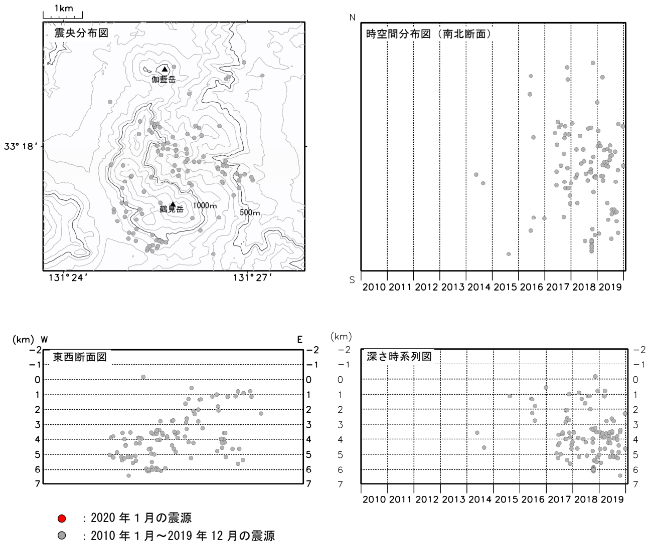
図 3-2 鶴見岳・伽藍岳 震源分布図（鶴見岳・伽藍岳付近の火山性地震） （2010年1月～2020年1月）
