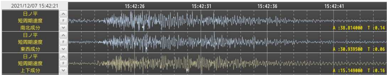
図4 鶴見岳・伽藍岳 B型地震の波形例（2021年12月7日15時、日ノ平観測点）
