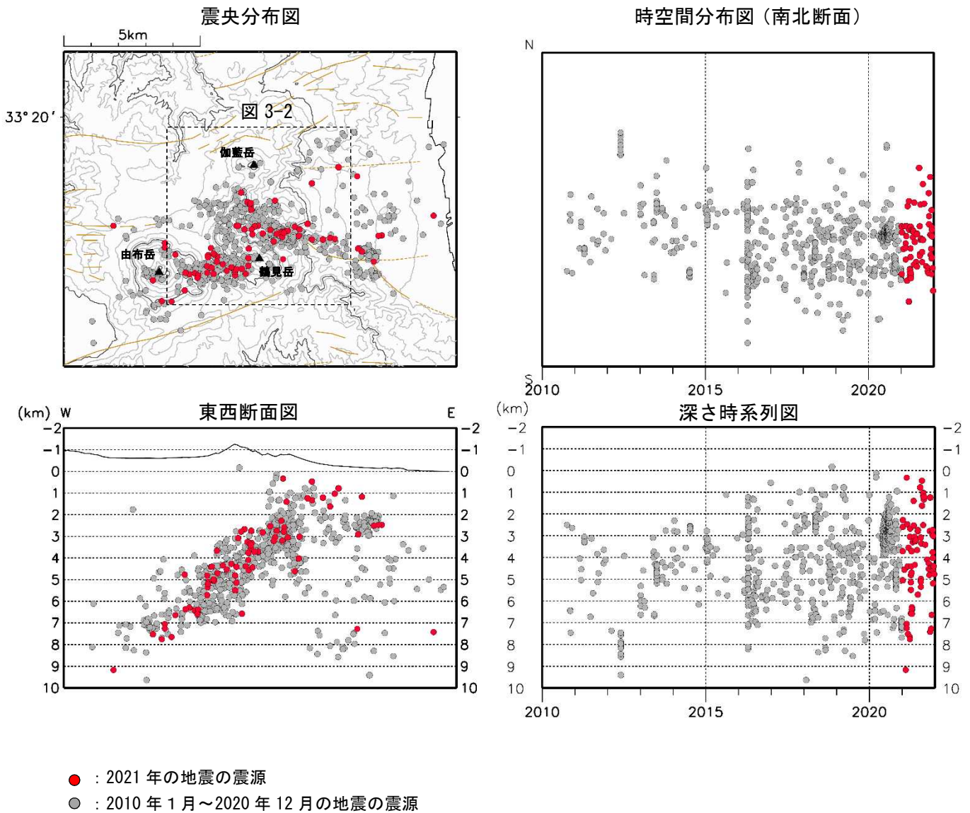
図 3-1 鶴見岳・伽藍岳 震源分布図（広域）（2010年1月～2021年12月）
