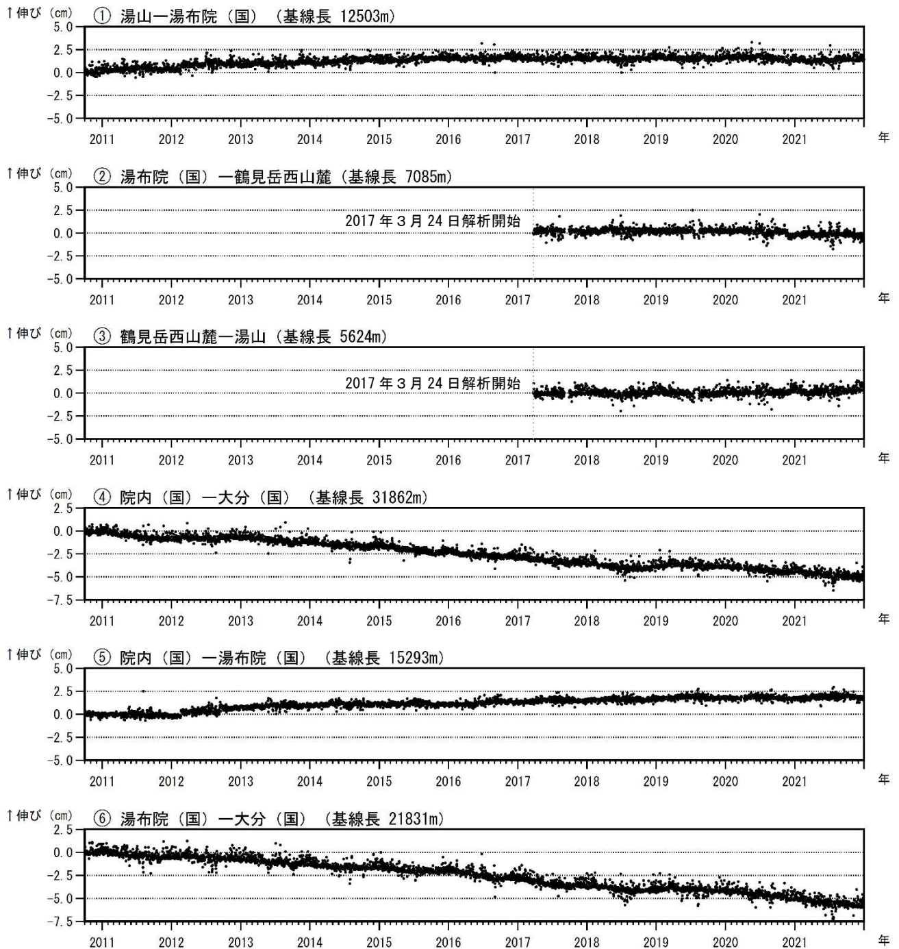
図 10 鶴見岳・伽藍岳 GNSS連続観測による基線長変化 (2010年10月～2021年12月)
