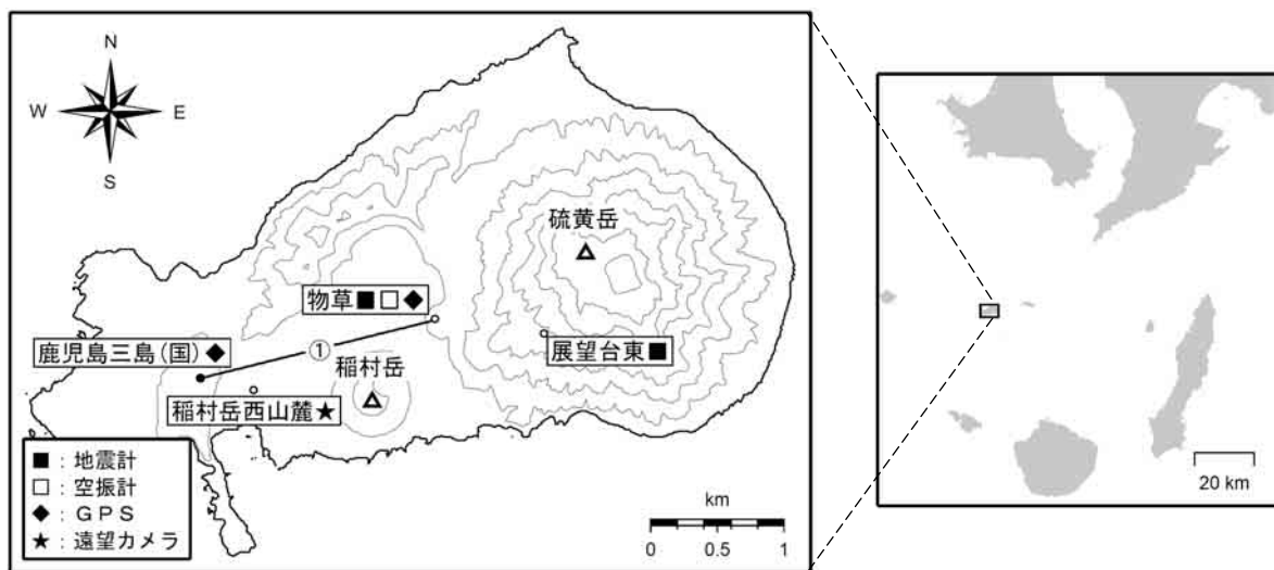
図 10 薩摩硫黄島 観測点配置図
