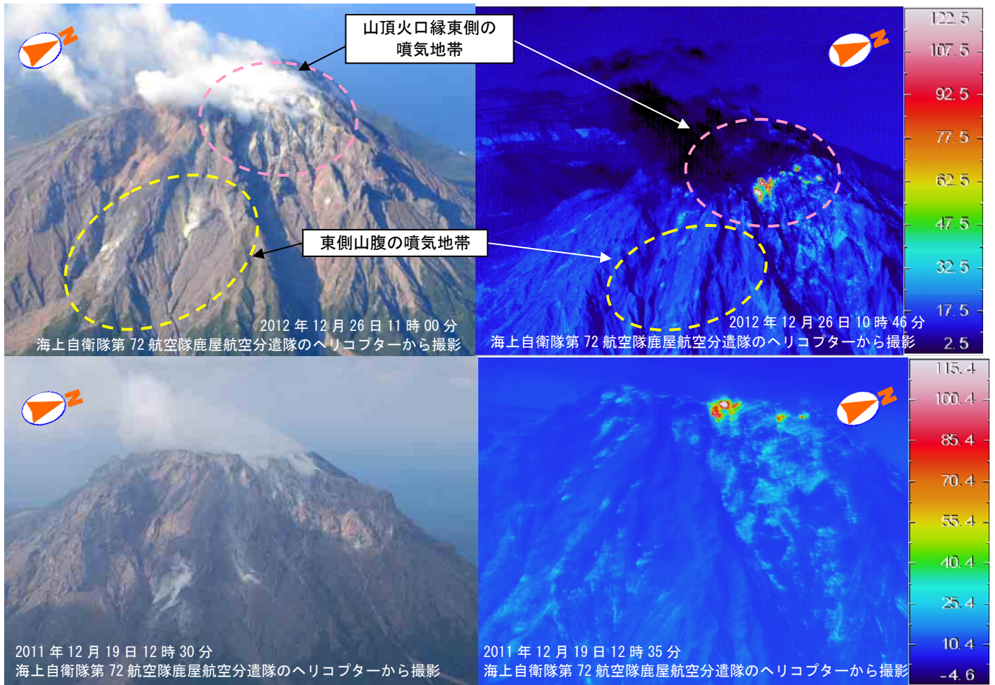
図 6 薩摩硫黄島 赤外熱映像装置による硫黄岳の地表面温度分布（図 8 ①方向から撮影）
