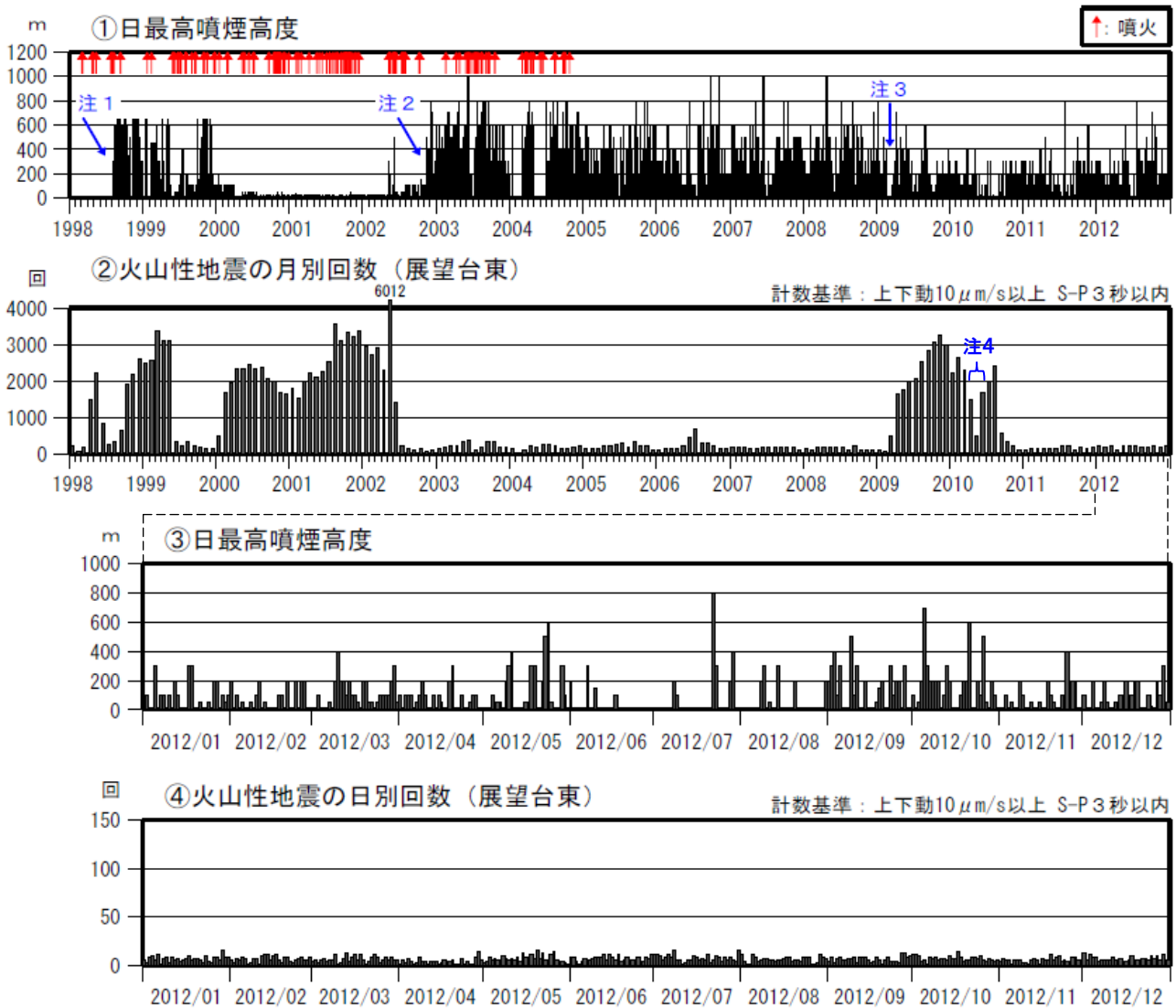
図 2 薩摩硫黄島 火山活動経過図 (1998 年 1 月～2012 年 12 月)
