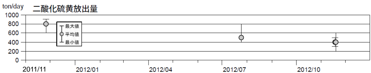
図 3 薩摩硫黄島 1 日あたりの二酸化硫黄放出量 (2011 年 11 月～2012 年 12 月)
