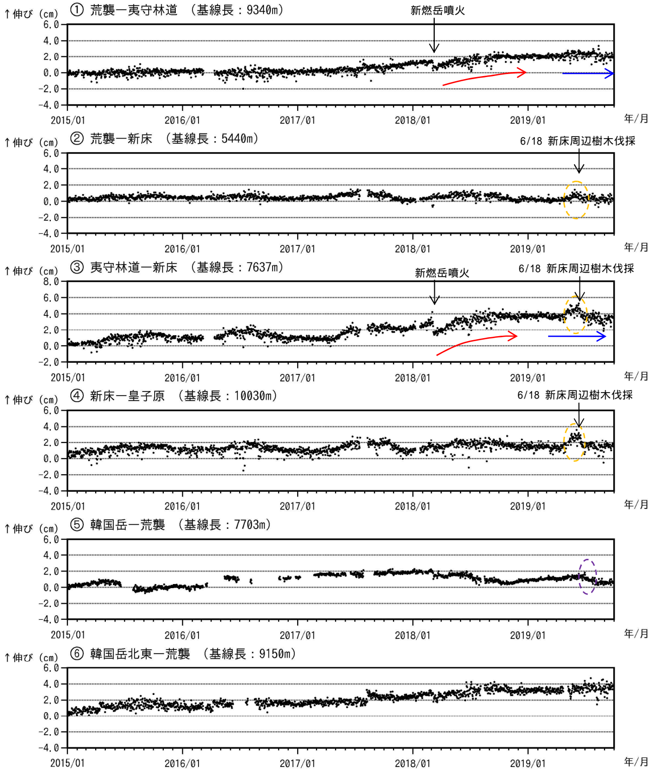
図 5-1 霧島山（新燃岳） GNSS 連続観測による基線長変化（2015 年 1 月～2019 年 9 月）
