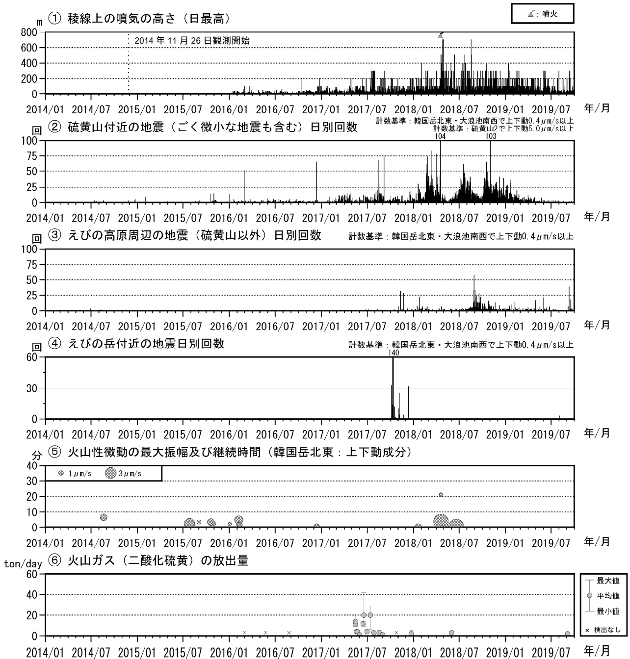
図6 霧島山（えびの高原（硫黄山）周辺）火山活動経過図（2014年1月～2019年9月）
