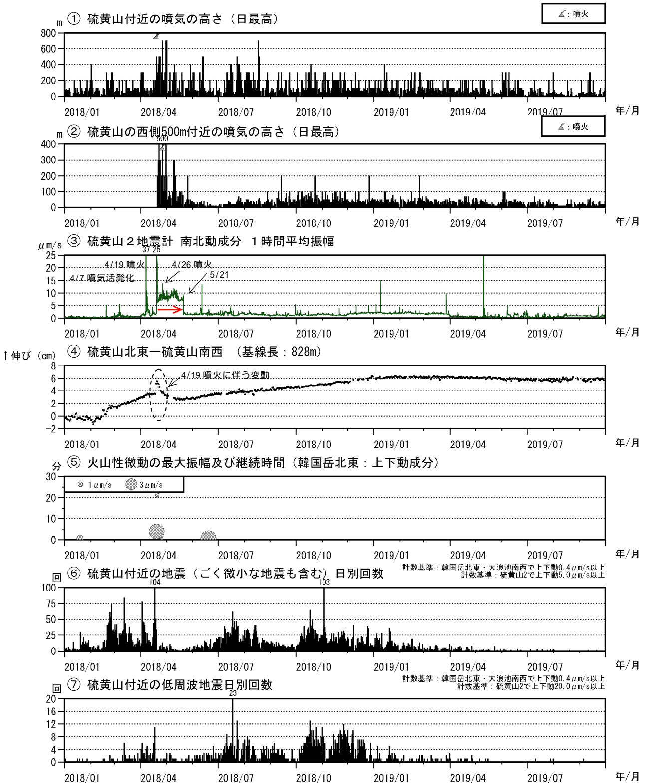
図5 霧島山（えびの高原（硫黄山）周辺） 火山活動経過図（2018年1月～2019年9月）
