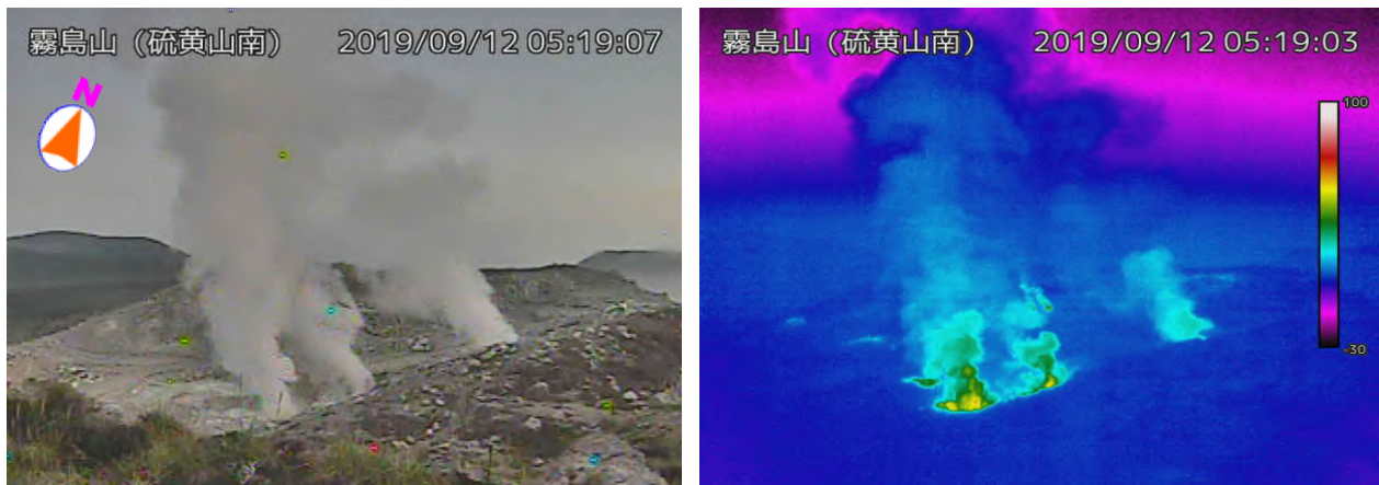
図 1-2 霧島山（えびの高原（硫黄山）周辺） 硫黄山南側の状況 （9月12日、硫黄山南監視カメラによる）
