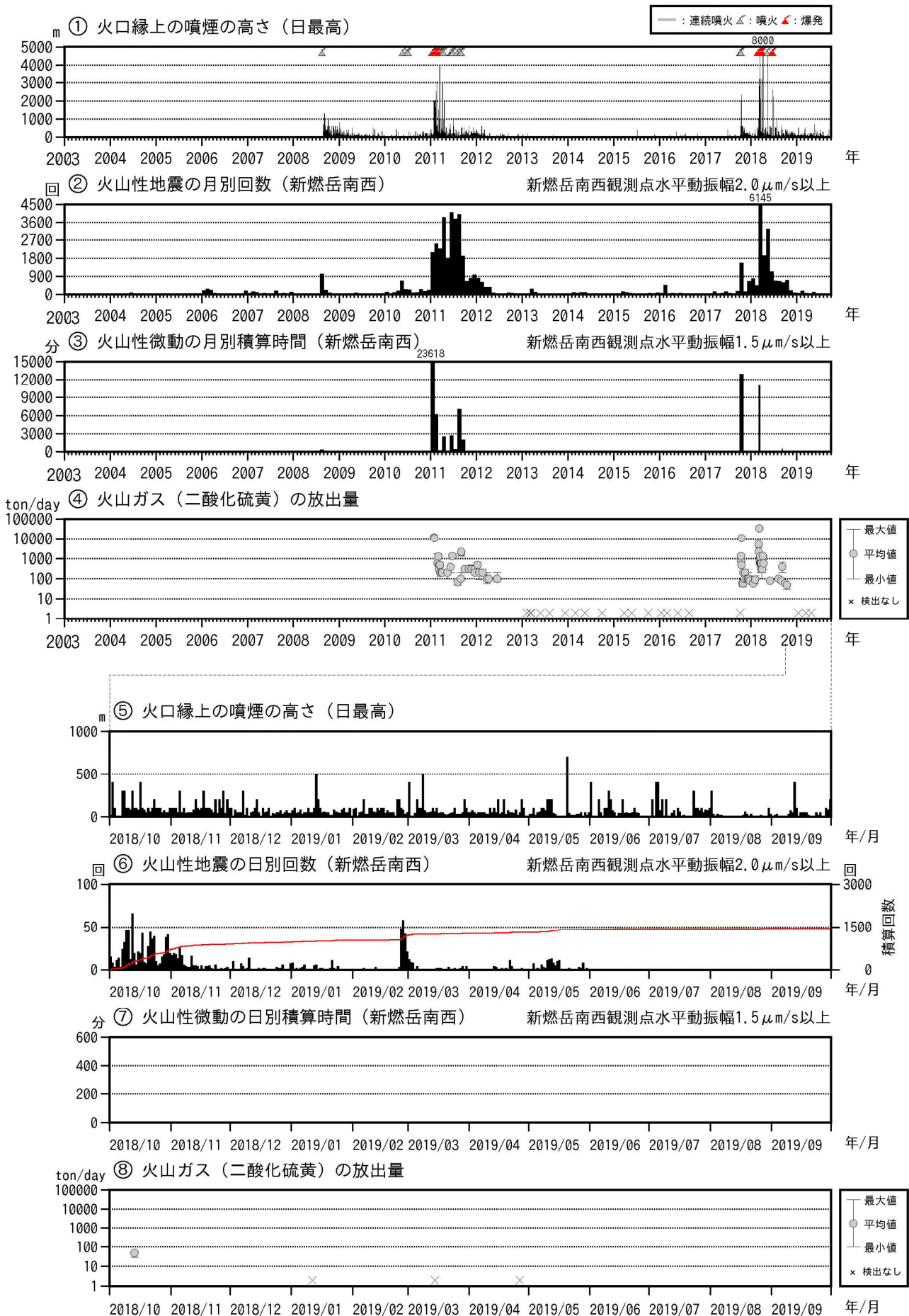
図2 霧島山（新燃岳） 火山活動経過図（2003年1月～2019年9月）
