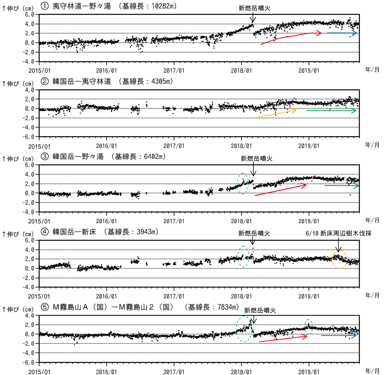
図 8-1 霧島山（えびの高原（硫黄山）周辺） GNSS 連続観測による基線長変化 （2015年1月～2019年9月）
