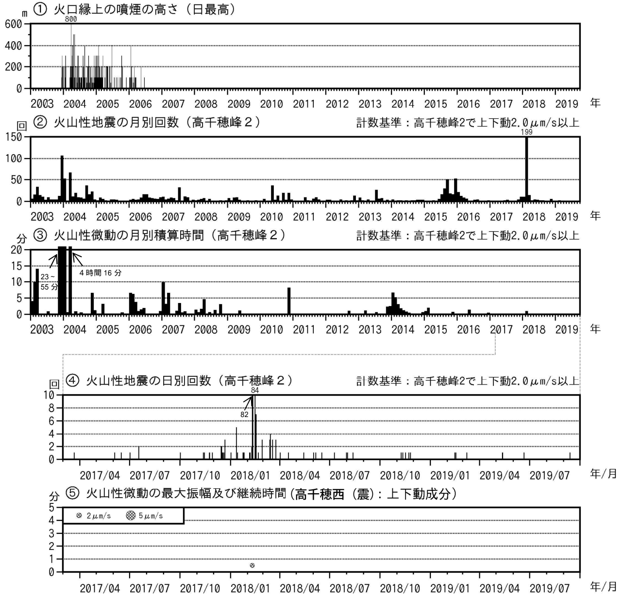
図2 霧島山（御鉢） 火山活動経過図（2003年1月～2019年9月）
