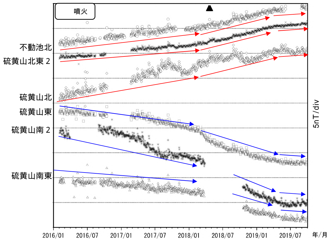
図 12 霧島山（えびの高原（硫黄山）周辺） 全磁力観測点で観測された全磁力変動 （2016 年 2 月～2019 年 9 月）
