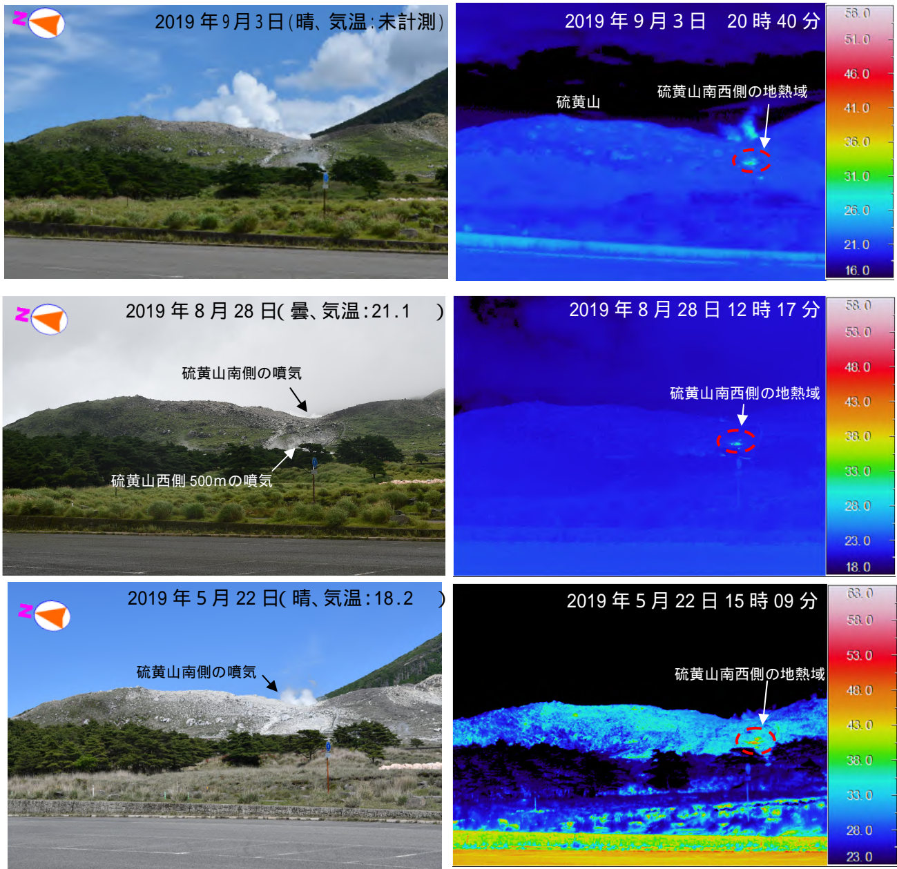
図3 霧島山（えびの高原（硫黄山）周辺） 硫黄山の状況（えびの高原（図2参照）から観測）
