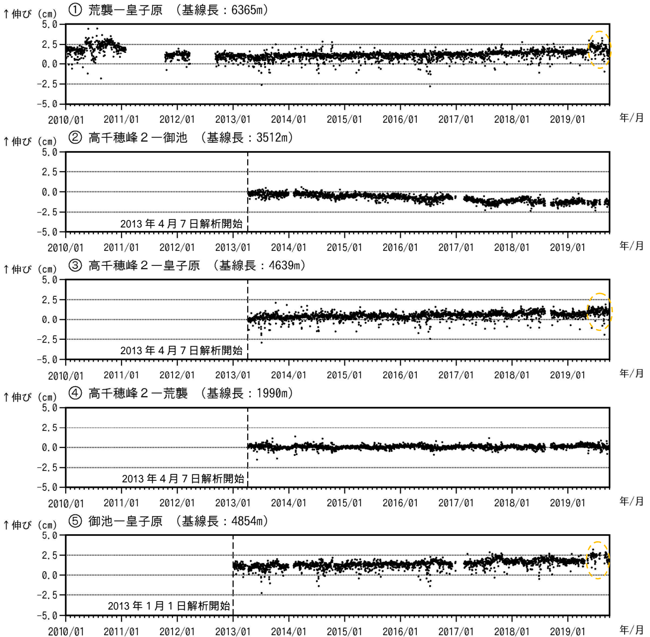
図4 霧島山（御鉢） GNSS連続観測による基線長変化（2010年1月～2019年9月）
