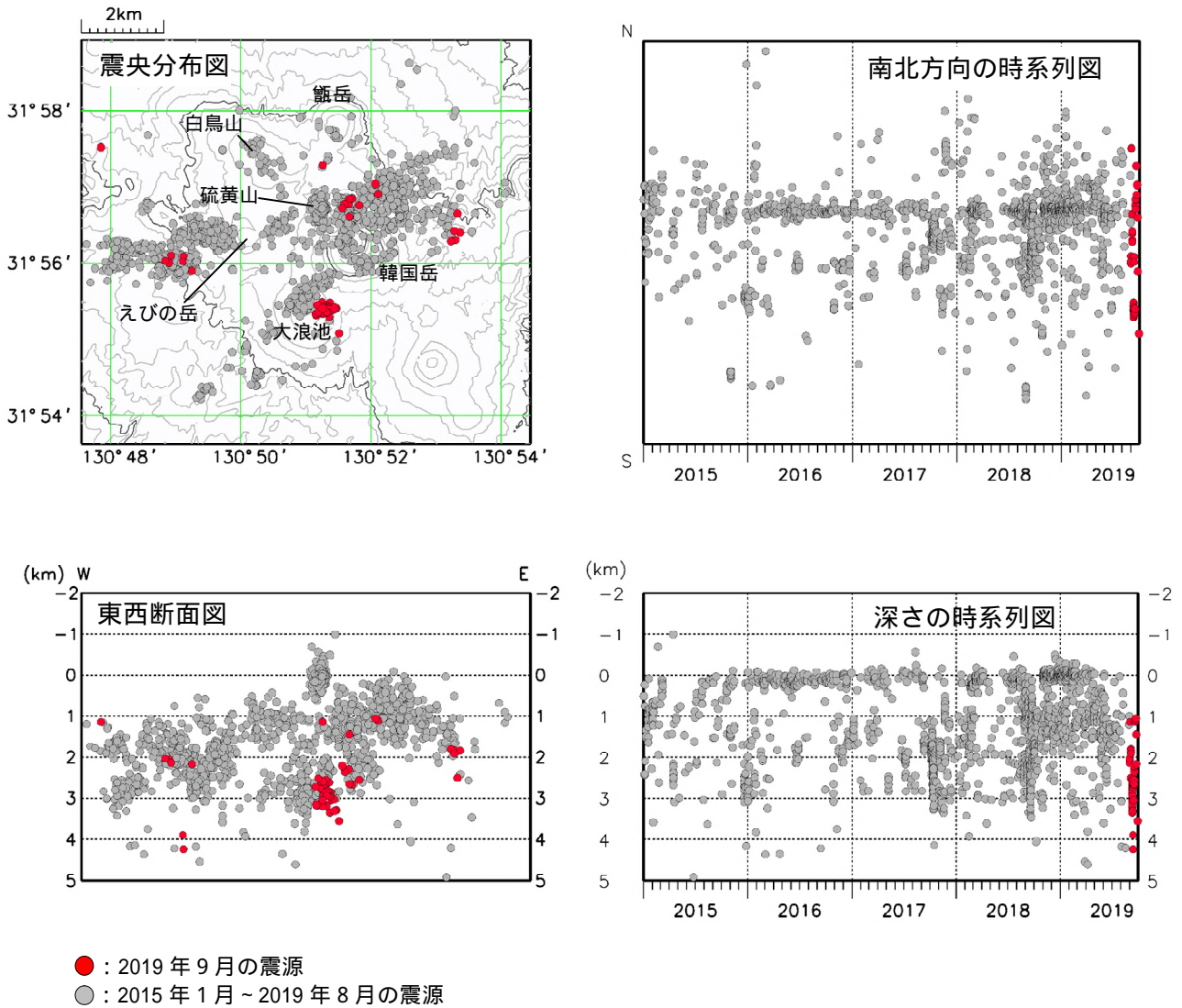
図4 霧島山（えびの高原（硫黄山）周辺） 震源分布図（2015年1月～2019年9月）
