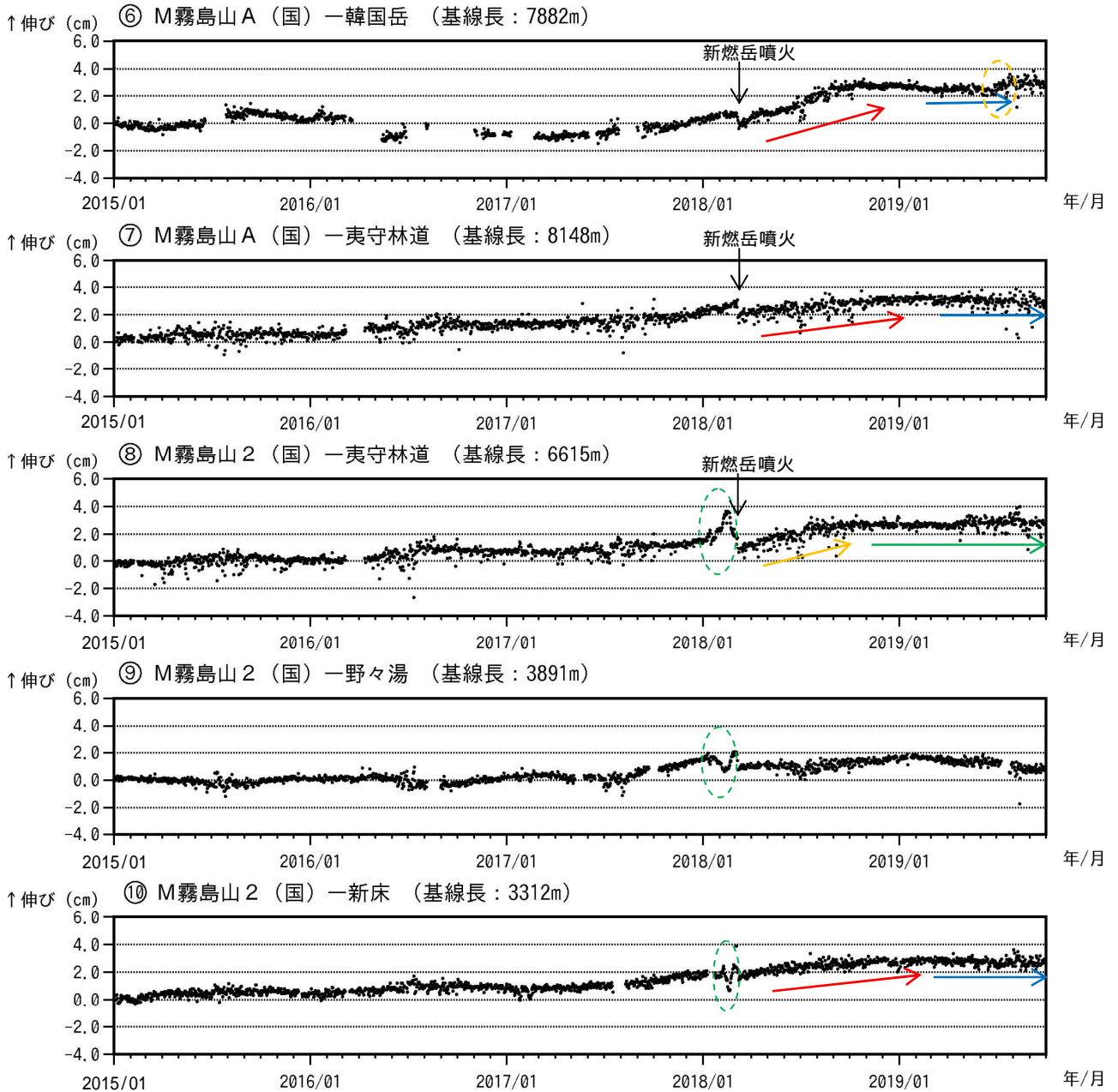
図 8-2 霧島山（えびの高原（硫黄山）周辺） GNSS 連続観測による基線長変化 （2015年1月～2019年9月）
