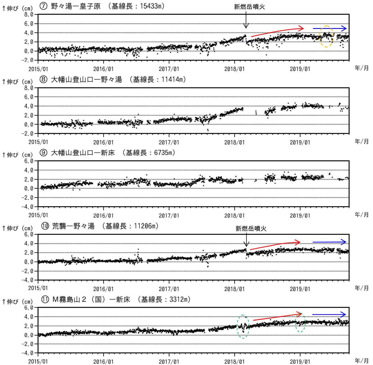
図 5-2 霧島山（新燃岳） GNSS 連続観測による基線長変化（2015 年 1 月～2019 年 9 月）
