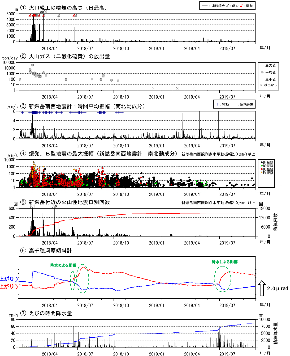
図3 霧島山（新燃岳） 火山活動経過図（2018年2月～2019年9月）
