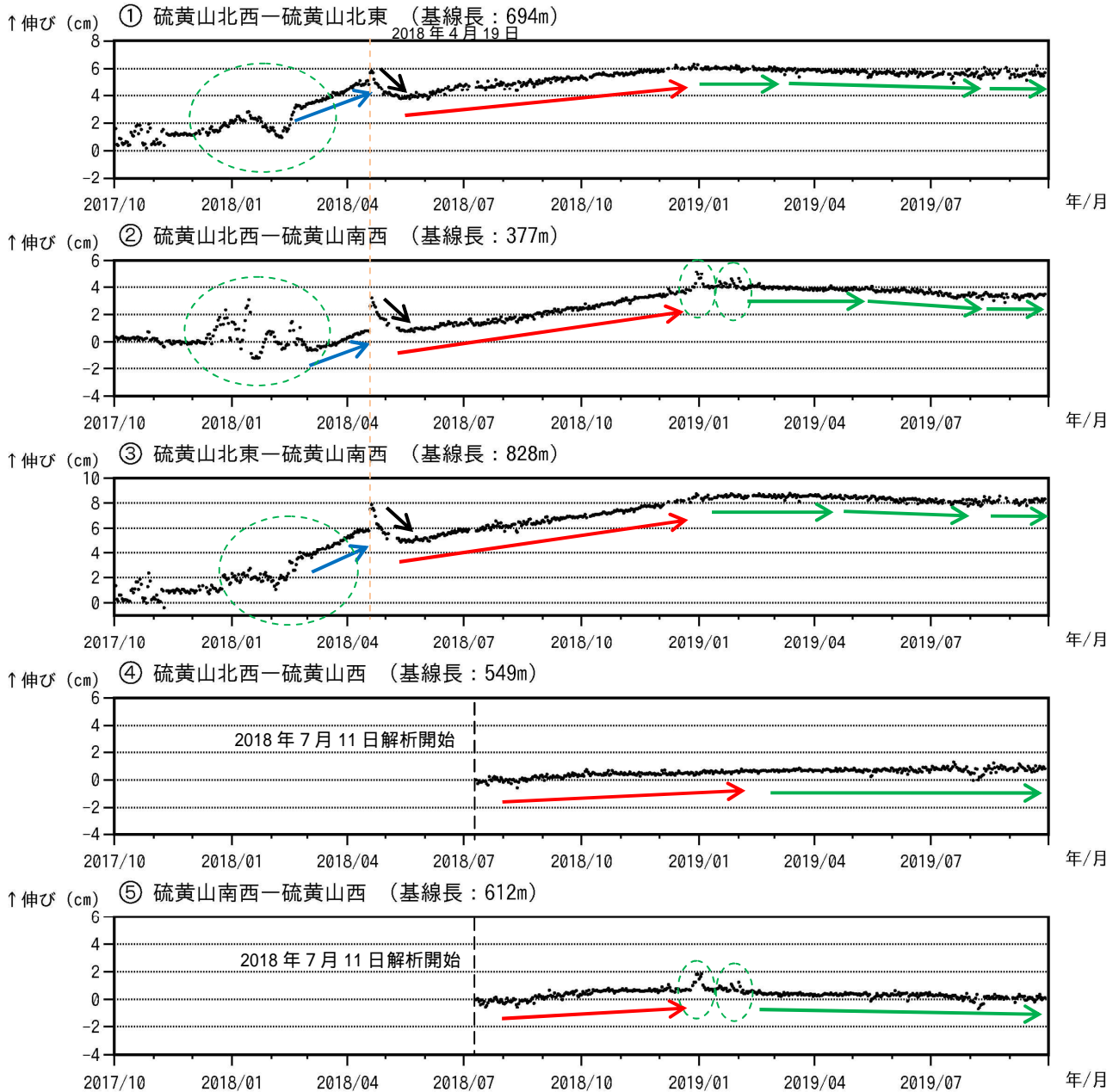
図7 霧島山（えびの高原（硫黄山）周辺） GNSS連続観測による基線長変化 (2017年10月～2019年9月)
