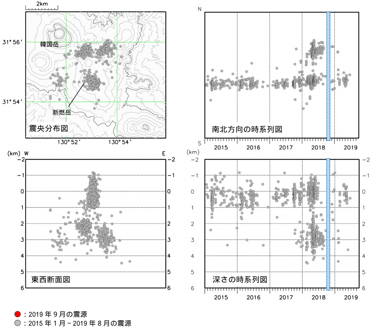
図4 霧島山（新燃岳）震源分布図（2015年1月～2019年9月）
