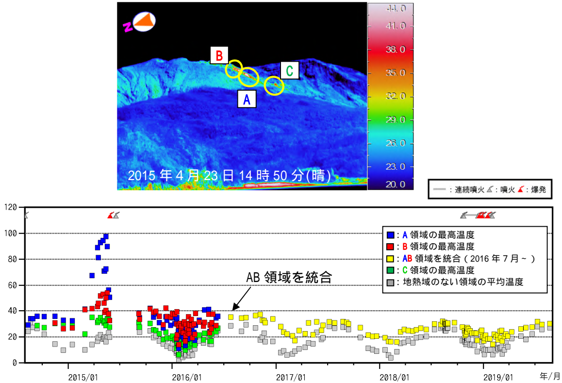
図 3 口永良部島 新岳西斜面及び新岳南西側斜面の地熱域の温度時系列 （2014 年 8 月～2019 年 8 月）
