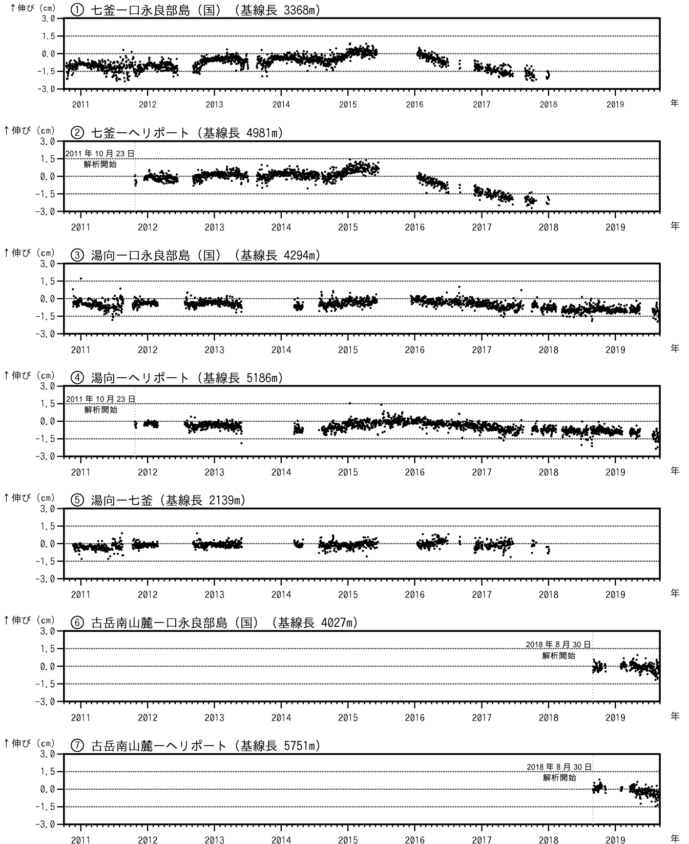
図 10 口永良部島 GNSS 連続観測による基線長変化（2010年10月～2019年8月）
