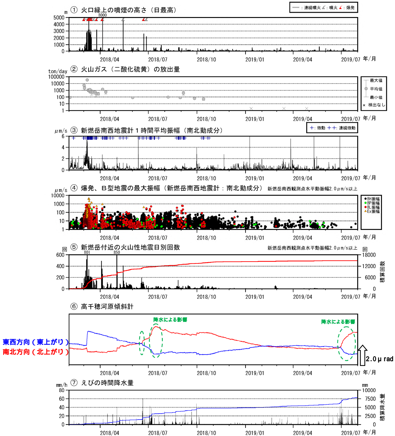
図3 霧島山（新燃岳） 火山活動経過図（2018年2月～2019年7月）
