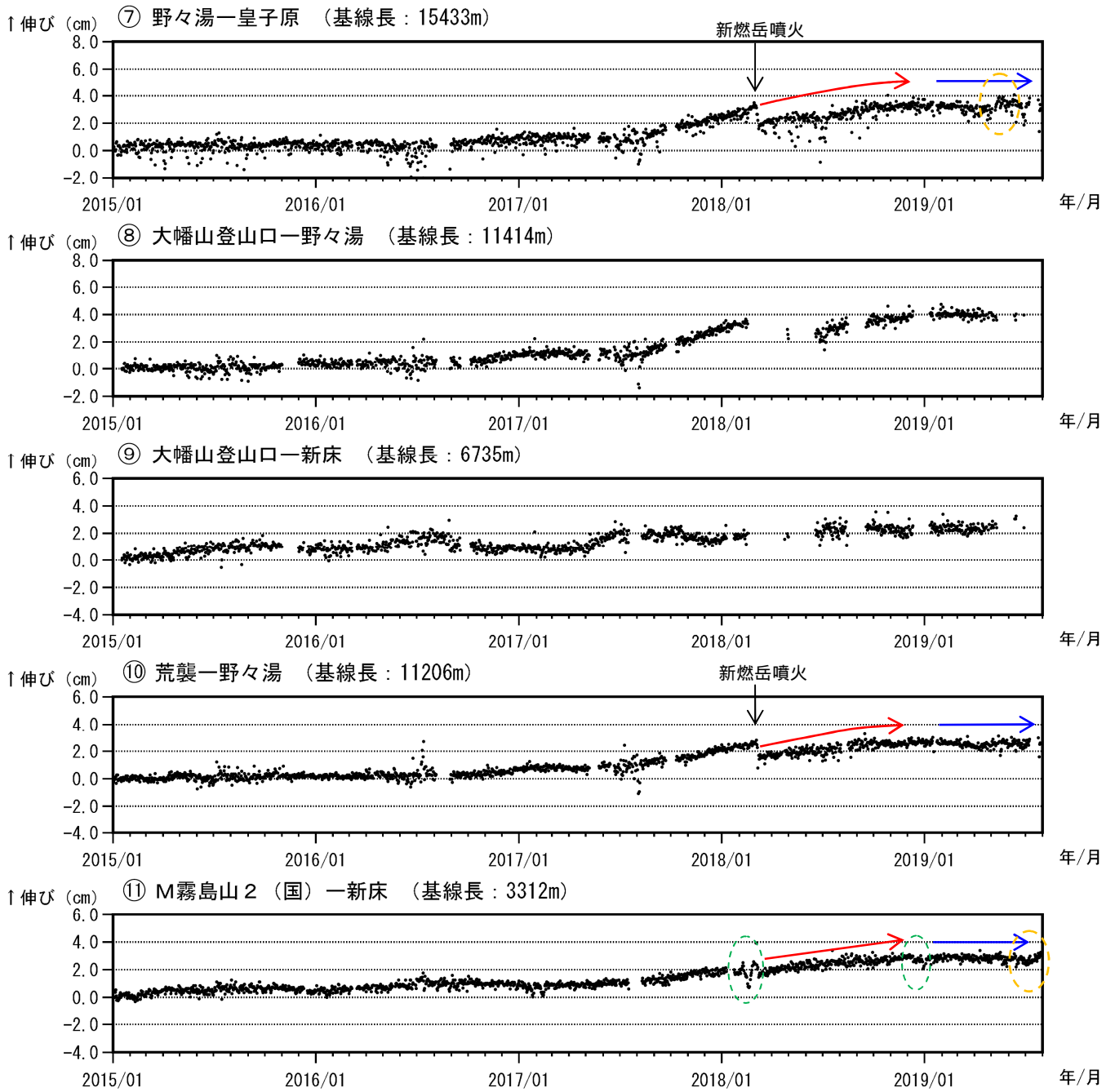
図 5-2 霧島山（新燃岳） GNSS 連続観測による基線長変化（2015 年 1 月～2019 年 7 月）
