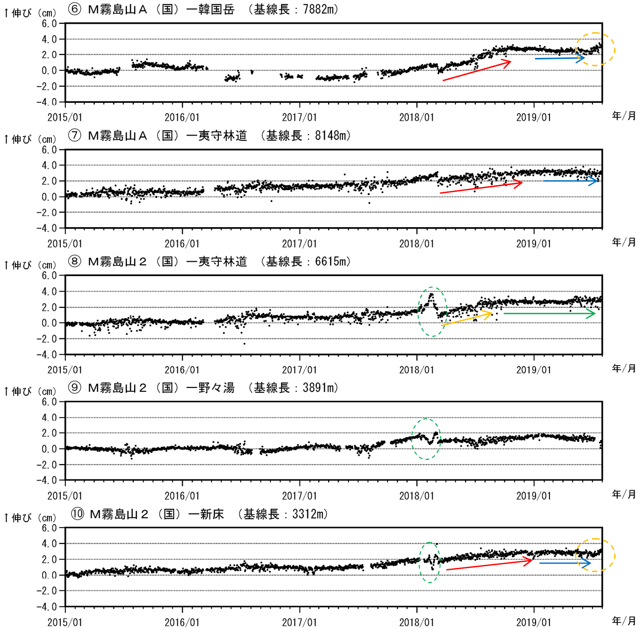
図 9-2 霧島山（えびの高原（硫黄山）周辺） GNSS 連続観測による基線長変化 （2015年1月～2019年7月）
