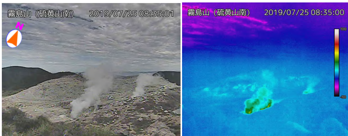
図 1-2 霧島山（えびの高原（硫黄山）周辺） 硫黄山南側の状況 （7月25日、硫黄山南監視カメラによる）
