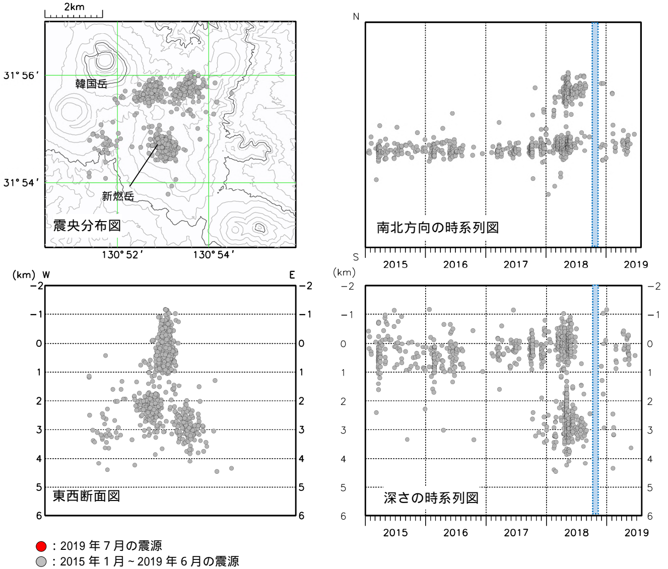
図4 霧島山（新燃岳）震源分布図（2015年1月～2019年7月）
