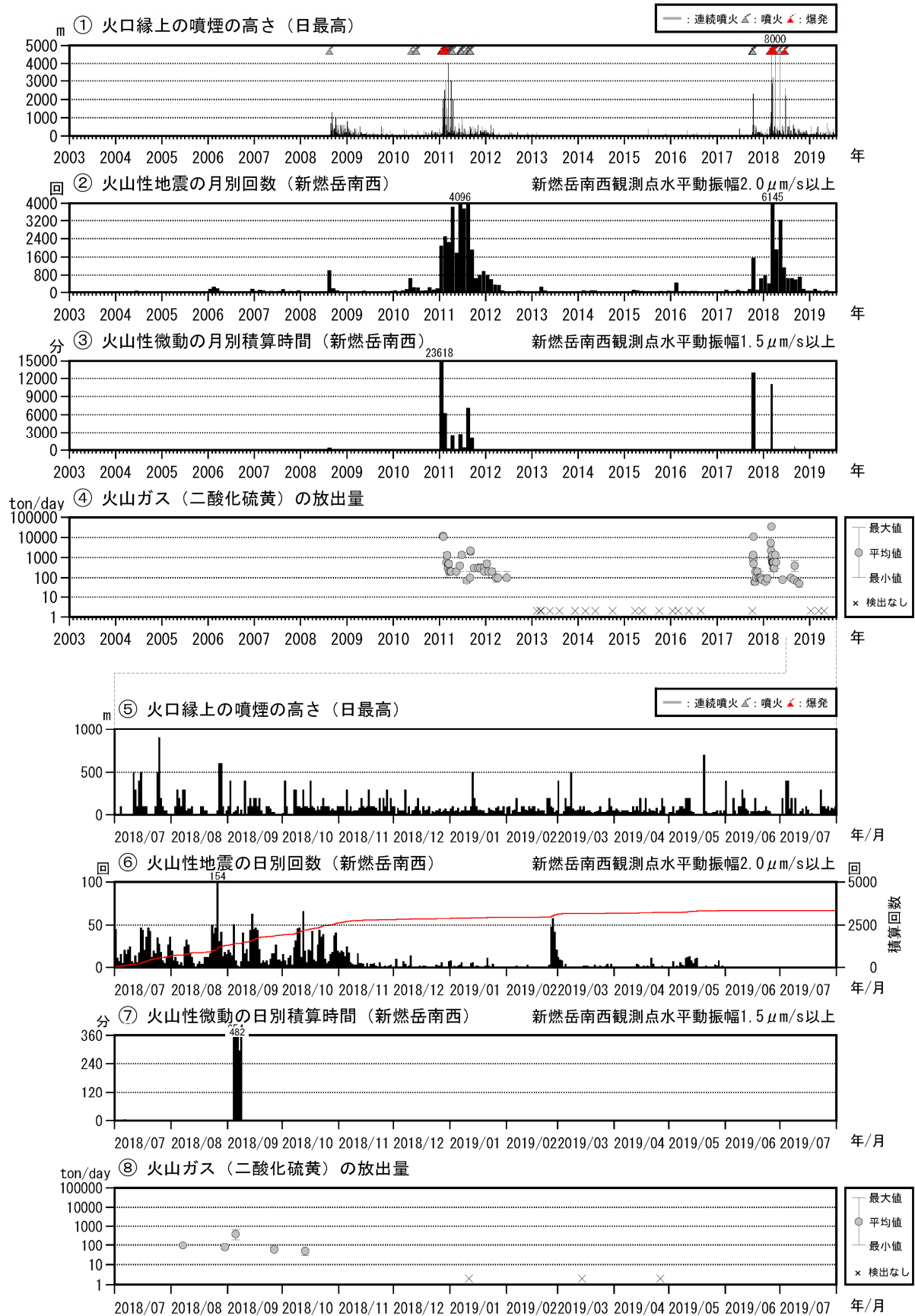
図2 霧島山（新燃岳）火山活動経過図（2003年1月～2019年7月）
