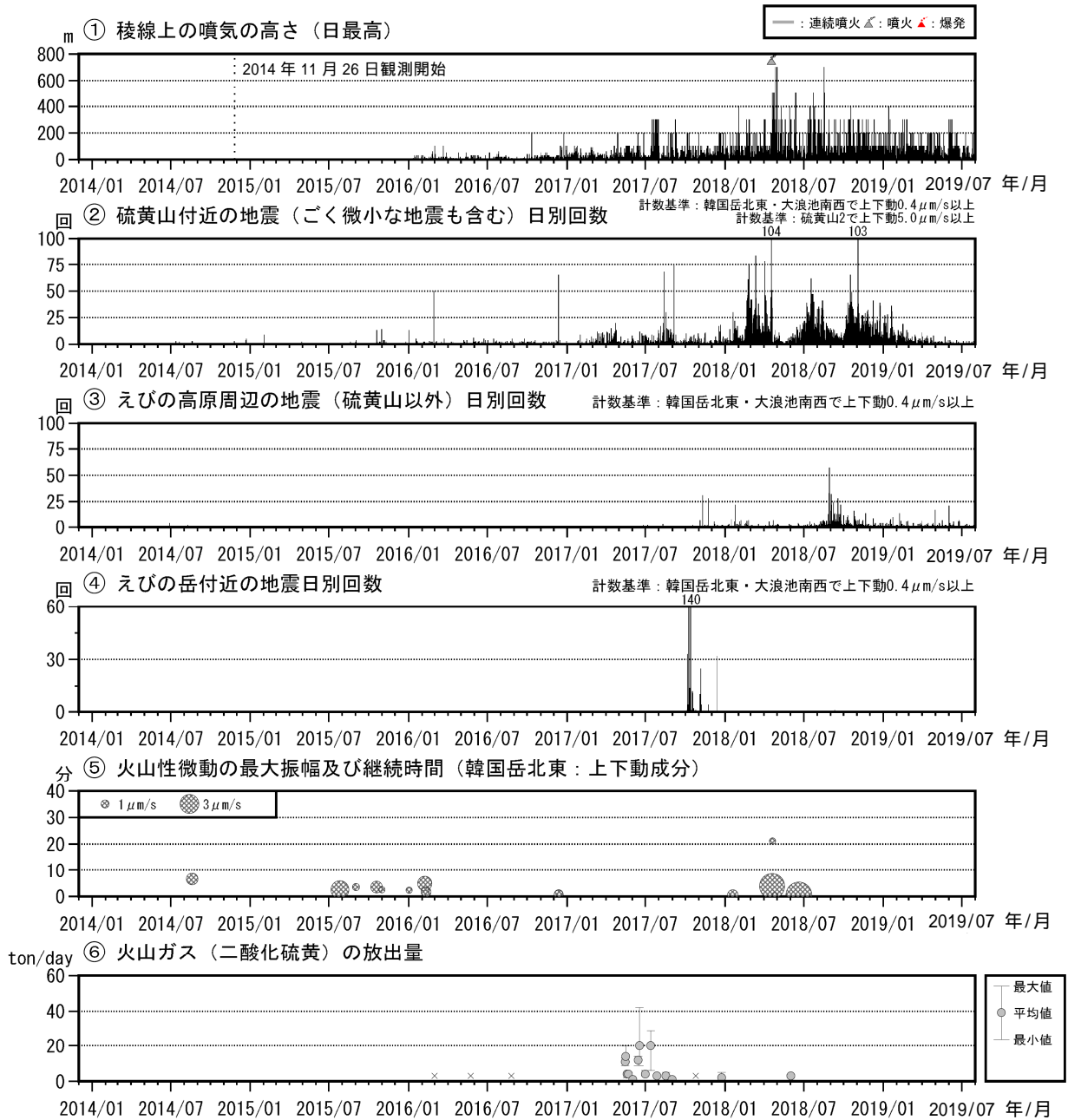
図7 霧島山（えびの高原（硫黄山）周辺）火山活動経過図（2013年12月～2019年7月）
