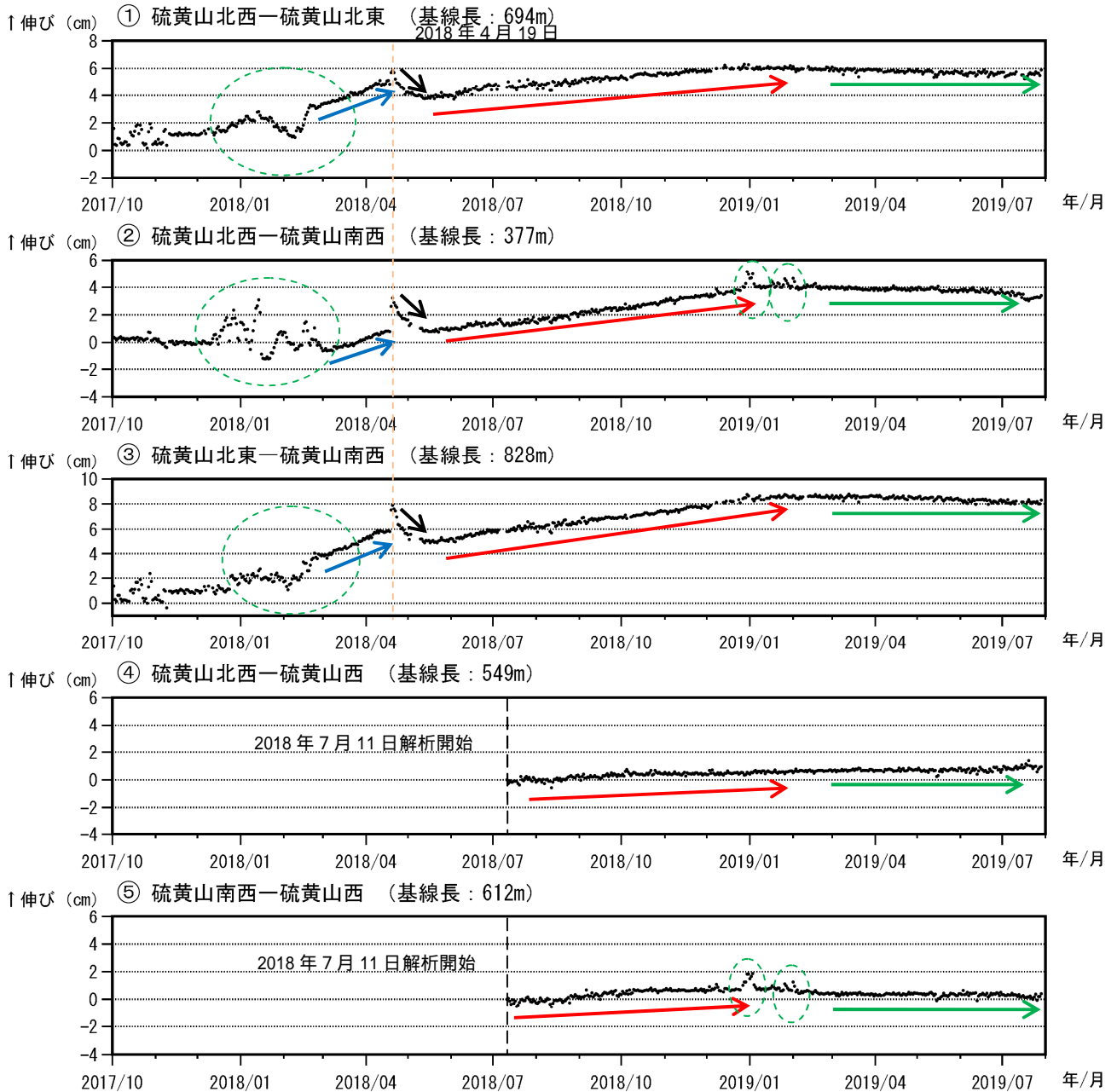
図8 霧島山（えびの高原（硫黄山）周辺） GNSS連続観測による基線長変化 (2017年10月～2019年7月)
