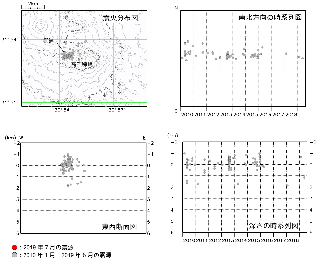
図3 霧島山（御鉢） 震源分布図（2010年1月～2019年7月）
