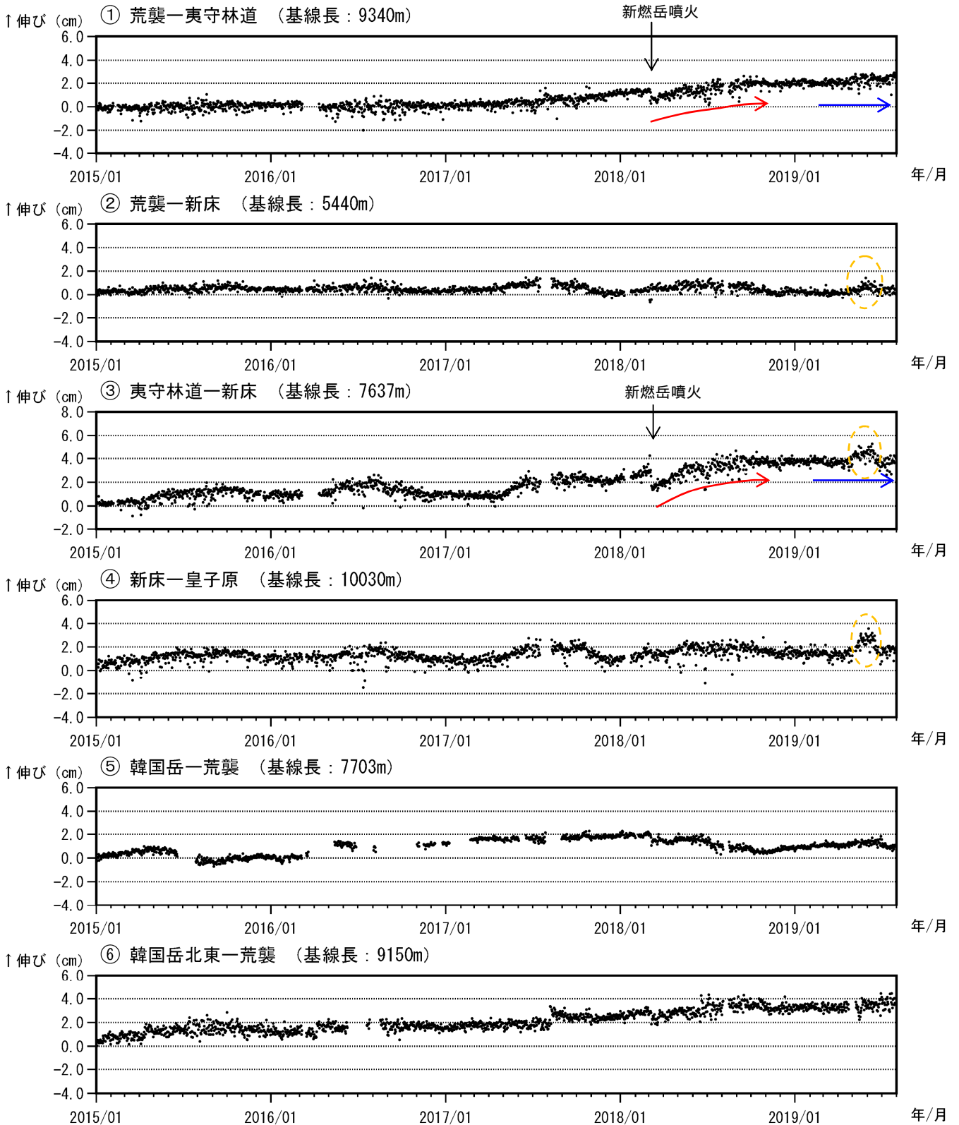
図 5-1 霧島山（新燃岳） GNSS 連続観測による基線長変化（2015 年 1 月～2019 年 7 月）
