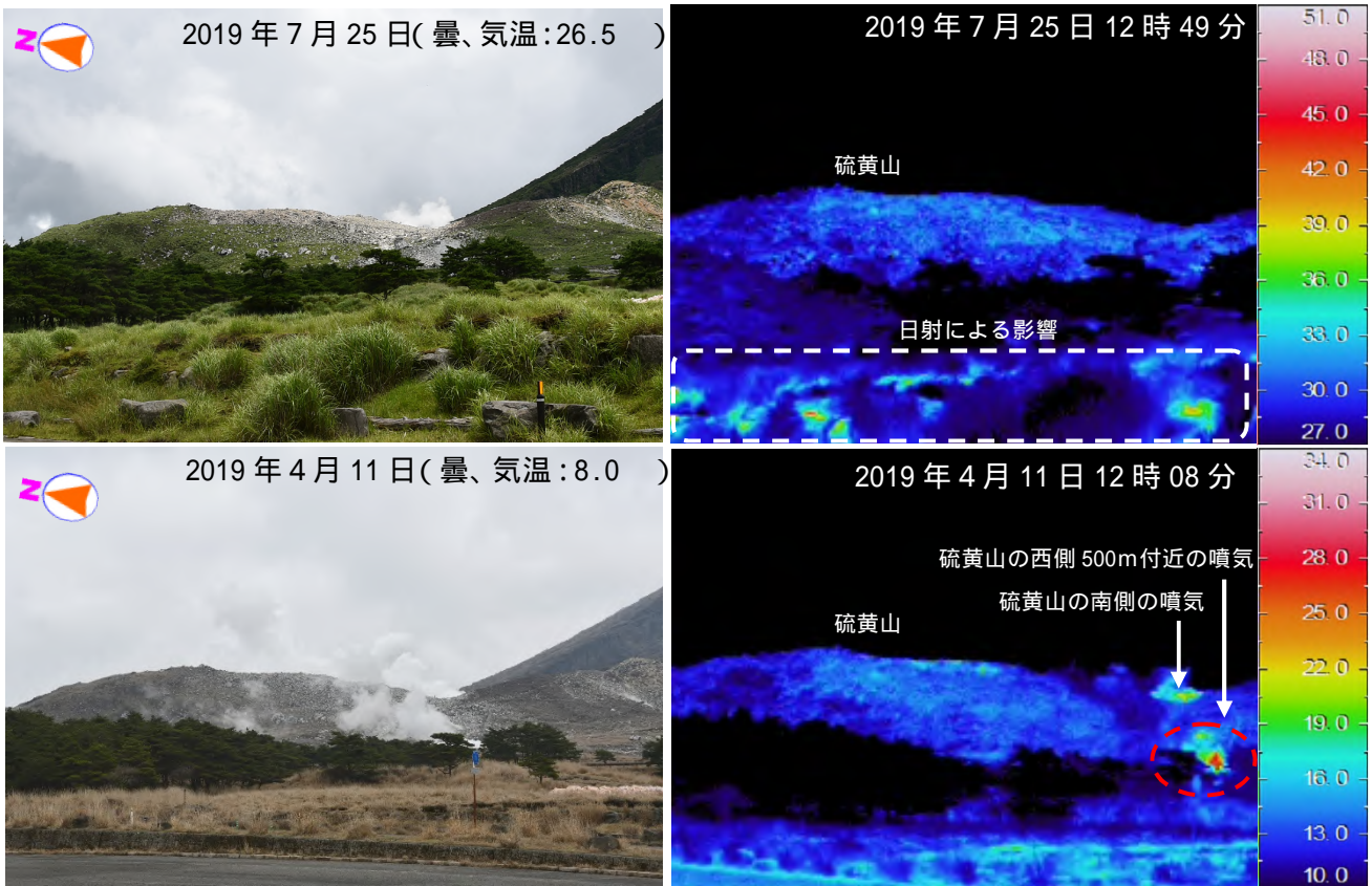
図4 霧島山（えびの高原（硫黄山）周辺） 硫黄山の状況（えびの高原（図2参照）から観測） ・硫黄山の南側の噴気地帯では、引き続き活発な噴気を確認しました。また、硫黄山の西側500m付近でも引き続き噴気を確認しました。 ・硫黄山付近では引き続き地熱域を確認しましたが、これまでの観測と比べ特段の変化は認められませんでした。
