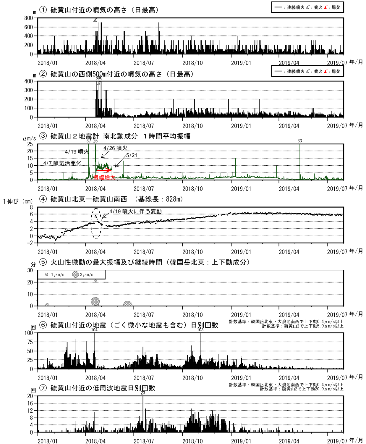
図6 霧島山（えびの高原（硫黄山）周辺） 火山活動経過図（2018年1月～2019年7月）
