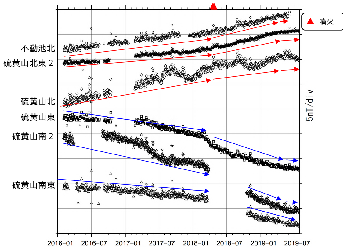
図 13 霧島山（えびの高原（硫黄山）周辺） 全磁力観測点で観測された全磁力変動 （2016 年 2 月～2019 年 7 月）
