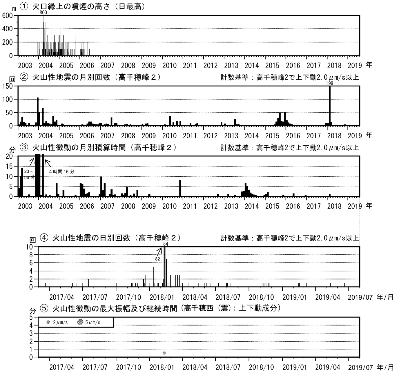
図2 霧島山（御鉢） 火山活動経過図（2003年1月～2019年7月）
