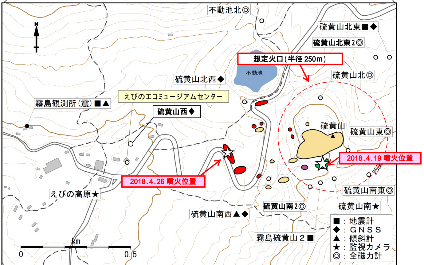
図2 霧島山（えびの高原（硫黄山）周辺） 噴火位置、主な噴気地帯及び地熱域、及び図3、4の観測位置及び観測方向
