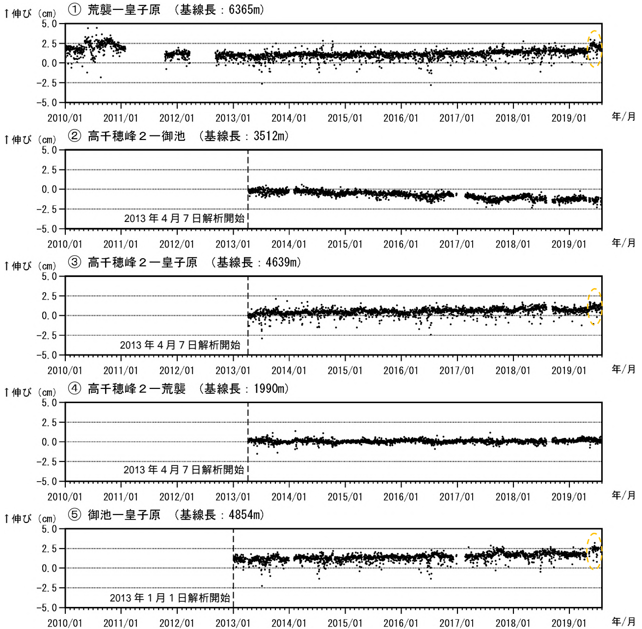
図4 霧島山（御鉢） GNSS 連続観測による基線長変化（2010年1月～2019年7月）
