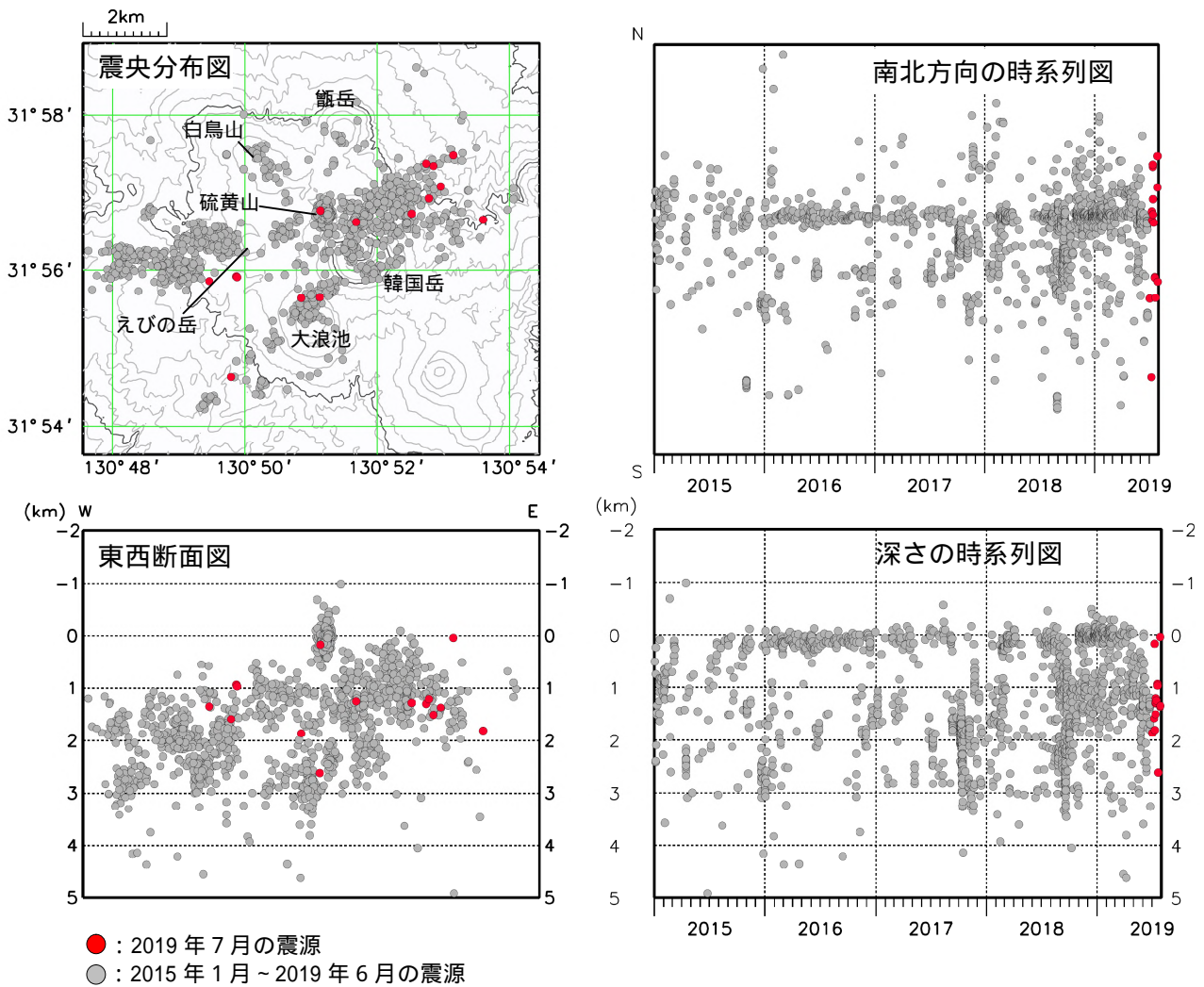
図5 霧島山（えびの高原（硫黄山）周辺）震源分布図（2015年1月～2019年7月）
