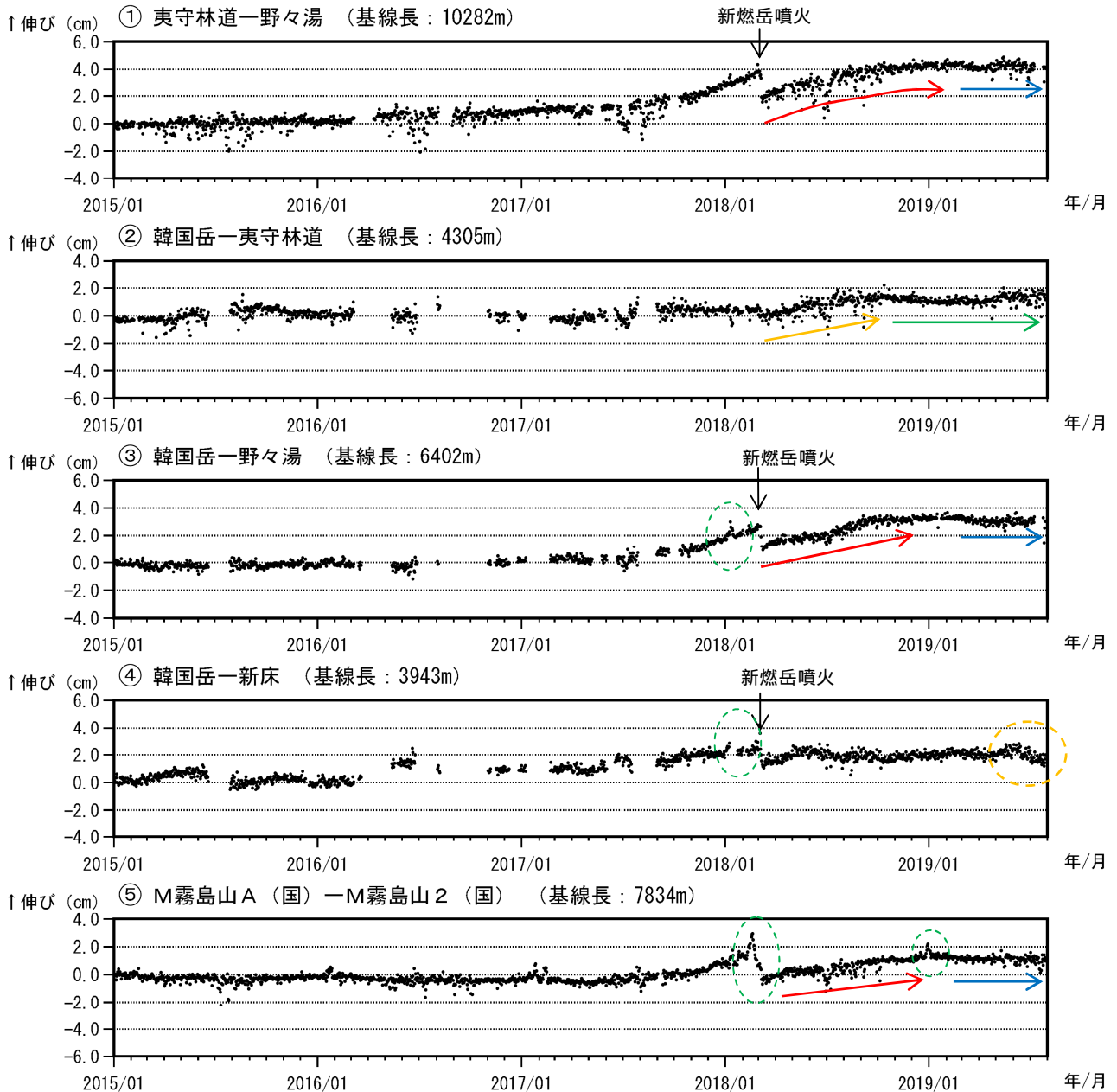
図 9-1 霧島山（えびの高原（硫黄山）周辺） GNSS 連続観測による基線長変化 （2015年1月～2019年7月）
