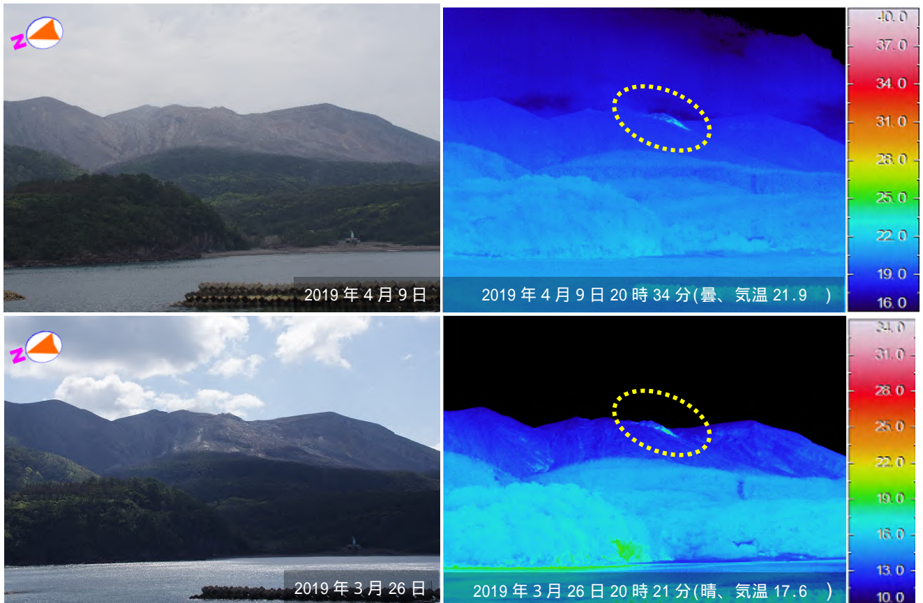
図4 口永良部島 新岳火口及び新岳火口西側割れ目付近の状況（本村から観測） 4月に実施した現地調査では、地熱域（黄破線）に特段の変化は認められませんでした。
