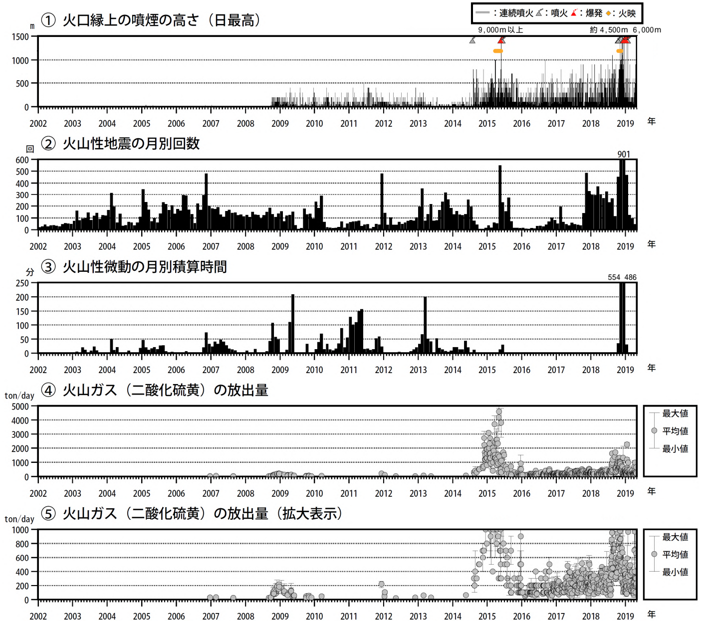
図5 口永良部島 火山活動経過図（2002年1月～2019年4月）
