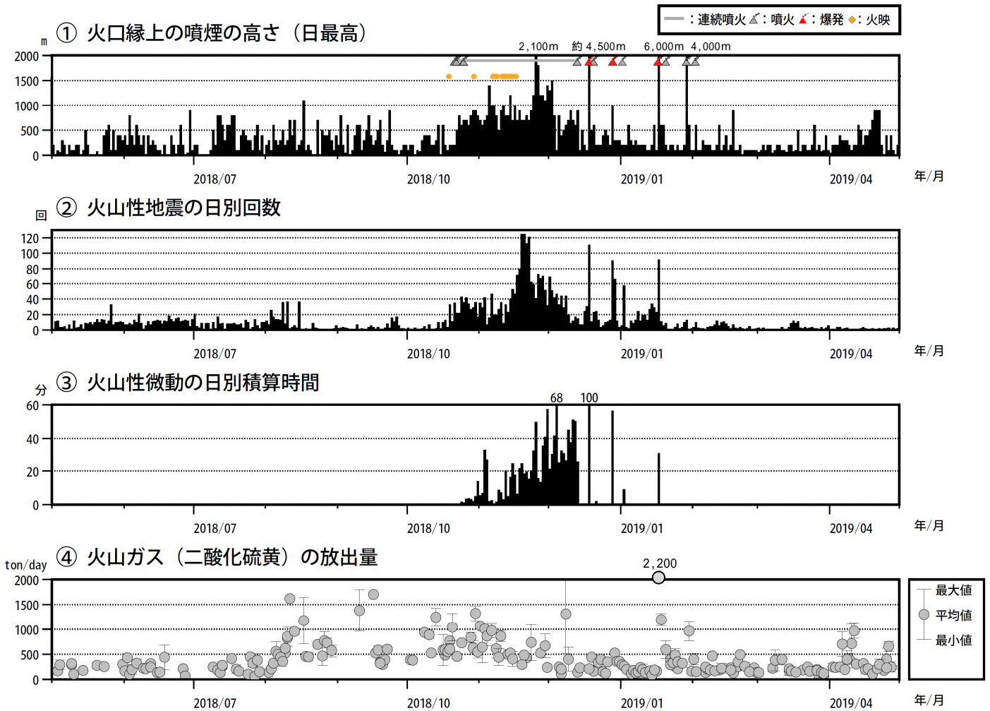
図6 口永良部島 最近の火山活動経過図(2018年5月~2019年4月)
