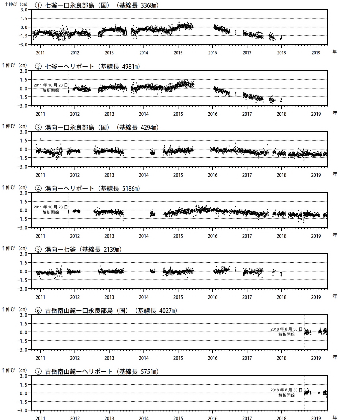
図9 口永良部島 GNSS連続観測による基線長変化(2010年10月~2019年4月)
