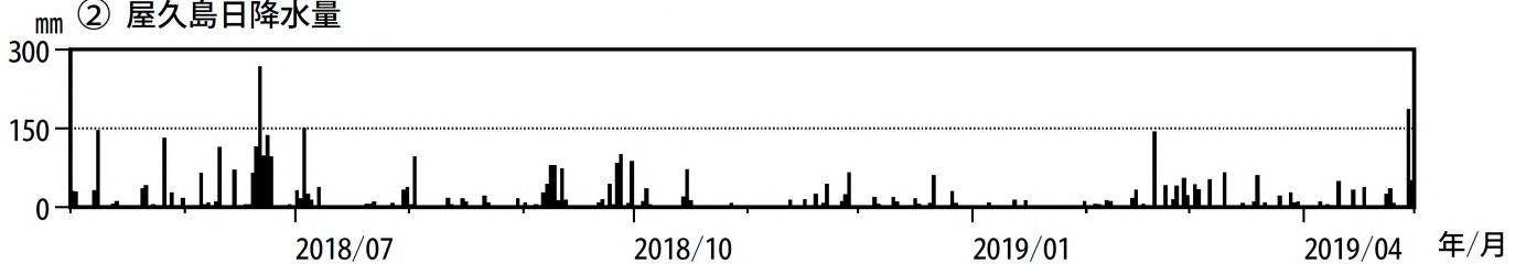
図8 口永良部島 新岳北東山麓観測点の傾斜変動(上段:2018年5月~2019年4月)
