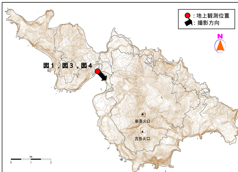
図2 口永良部島 観測位置及び撮影方向
