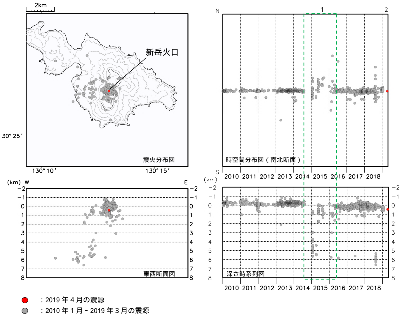
図 7 口永良部島 震源分布図(2010 年 1 月 ~ 2019 年 4 月)
