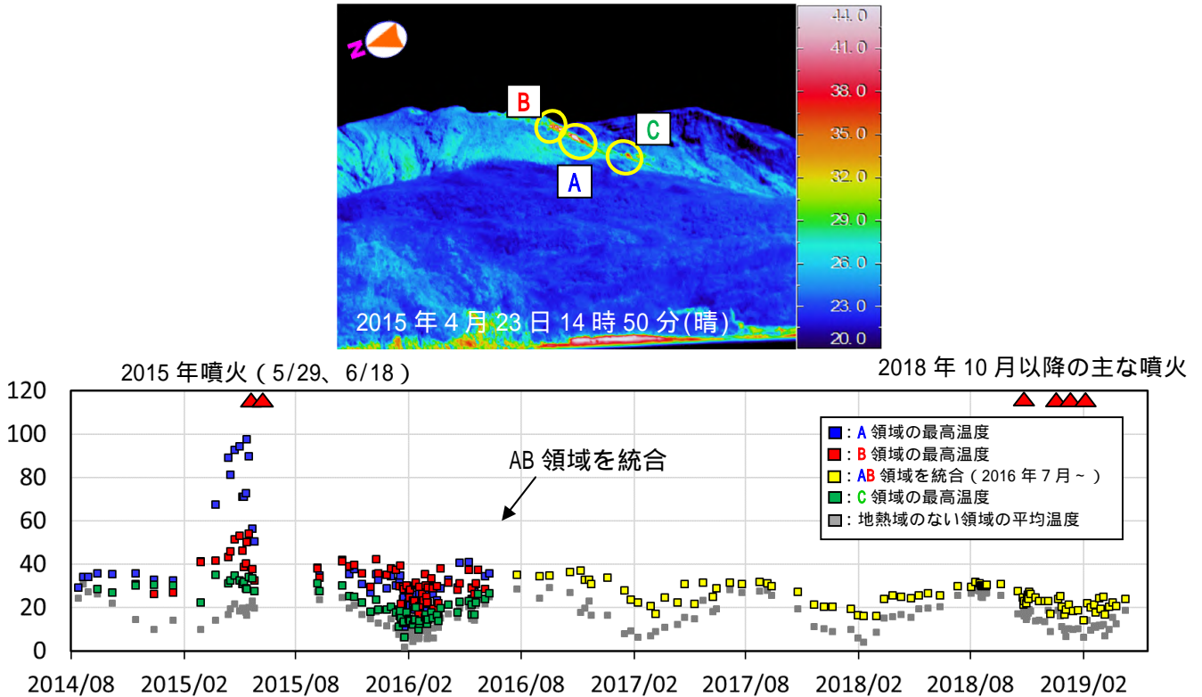
図3 口永良部島 新岳西斜面及び新岳南西側斜面の地熱域の温度時系列（2014年8月～2019年4月）
