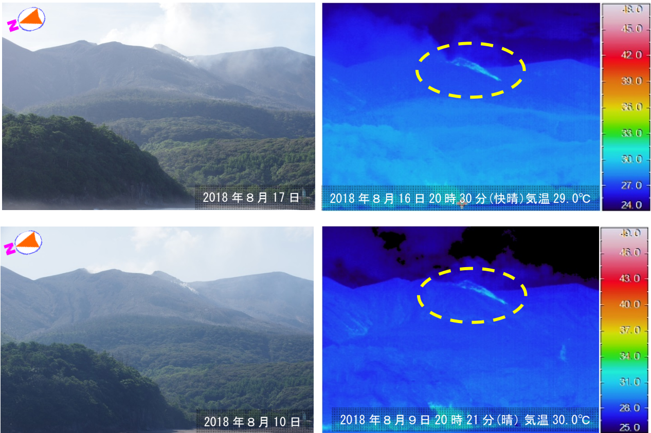
図 3-1 口永良部島 新岳火口及び新岳火口西側割れ目付近の可視画像と地表面温度分布 前回（8月9日）と比較して、噴気及び熱異常域（黄破線）に特段の変化は認められませんでした。
