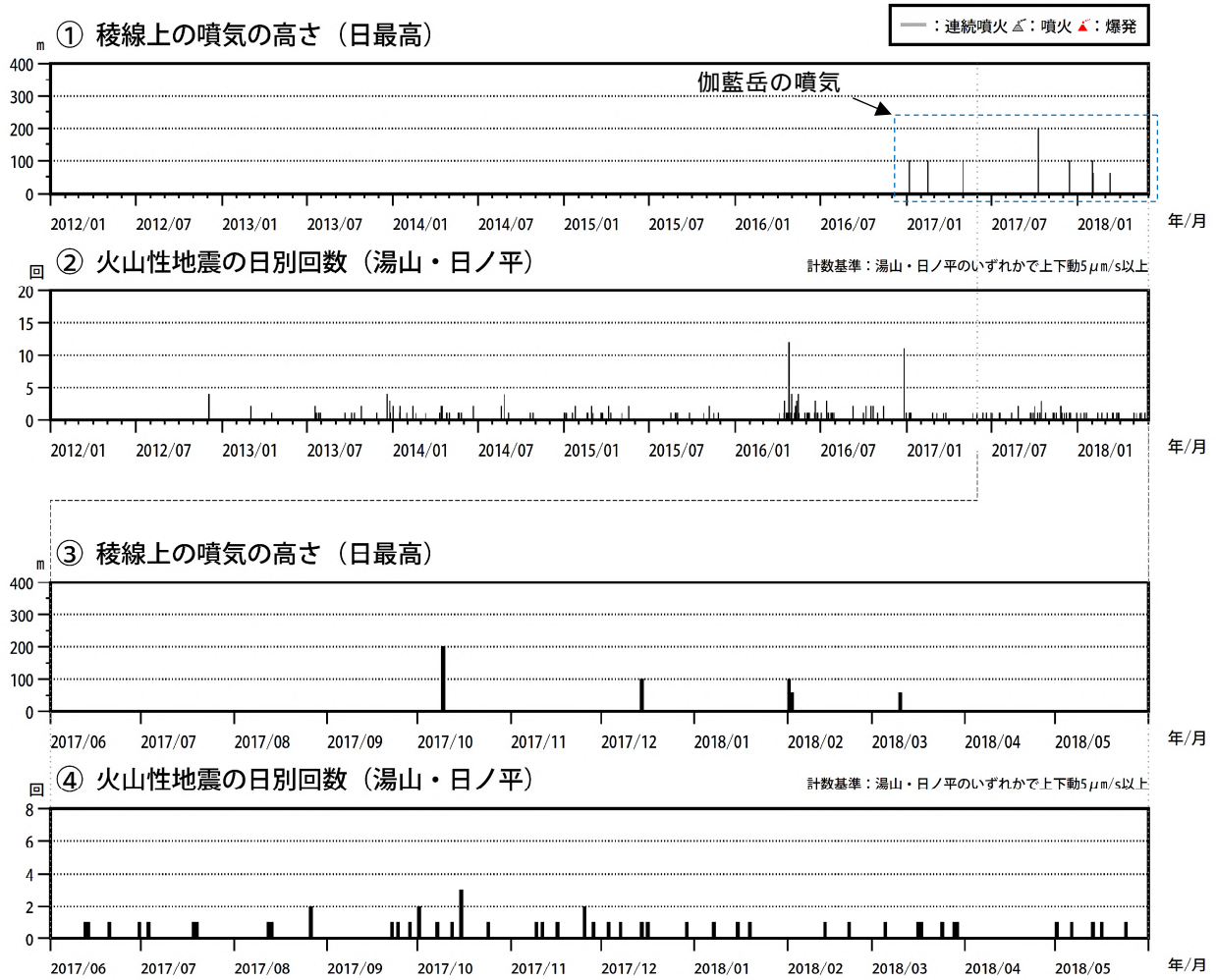
図2 鶴見岳・伽藍岳 火山活動経過図(2012年1月～2018年5月)
