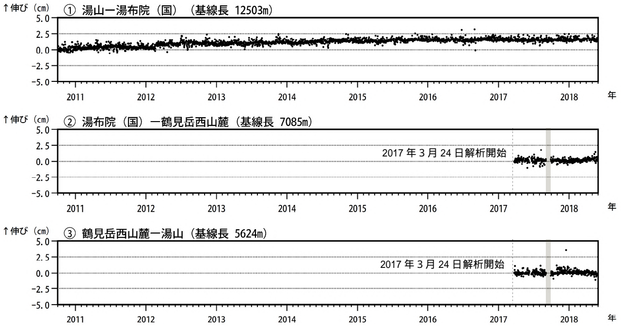
図 4 鶴見岳・伽藍岳 GNSS連続観測による基線長変化（2010年10月～2018年5月）
