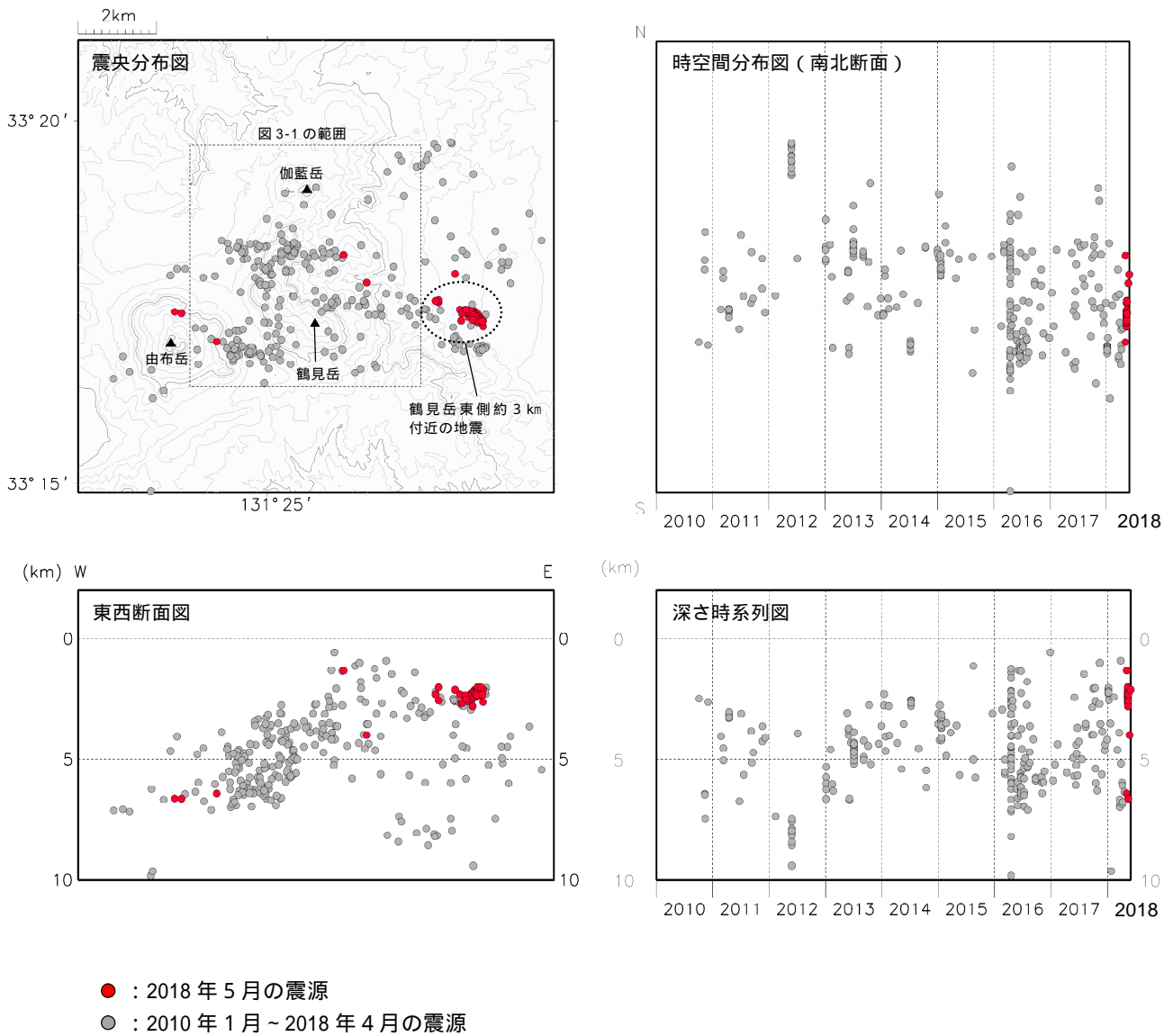
図3-2 鶴見岳・伽藍岳 震源分布図(広域)(2010年1月~2018年5月)
