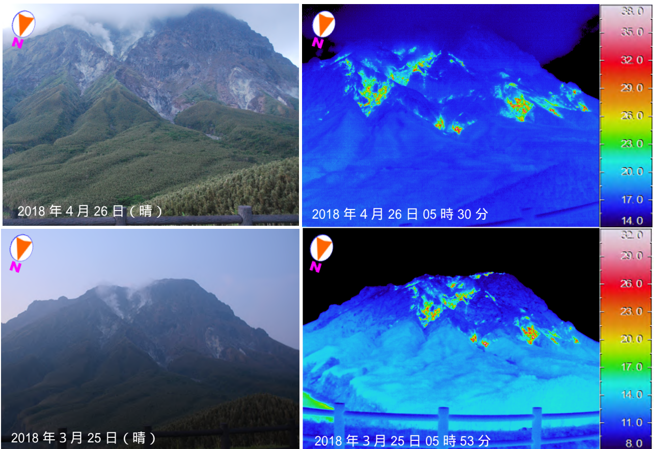
図 2 薩摩硫黄島 硫黄岳北側の状況（平家城展望台から観測） （上段：2018 年 4 月 26 日、下段：2018 年 3 月 25 日） 噴気及び熱異常域の分布に特段の変化は認められませんでした。
