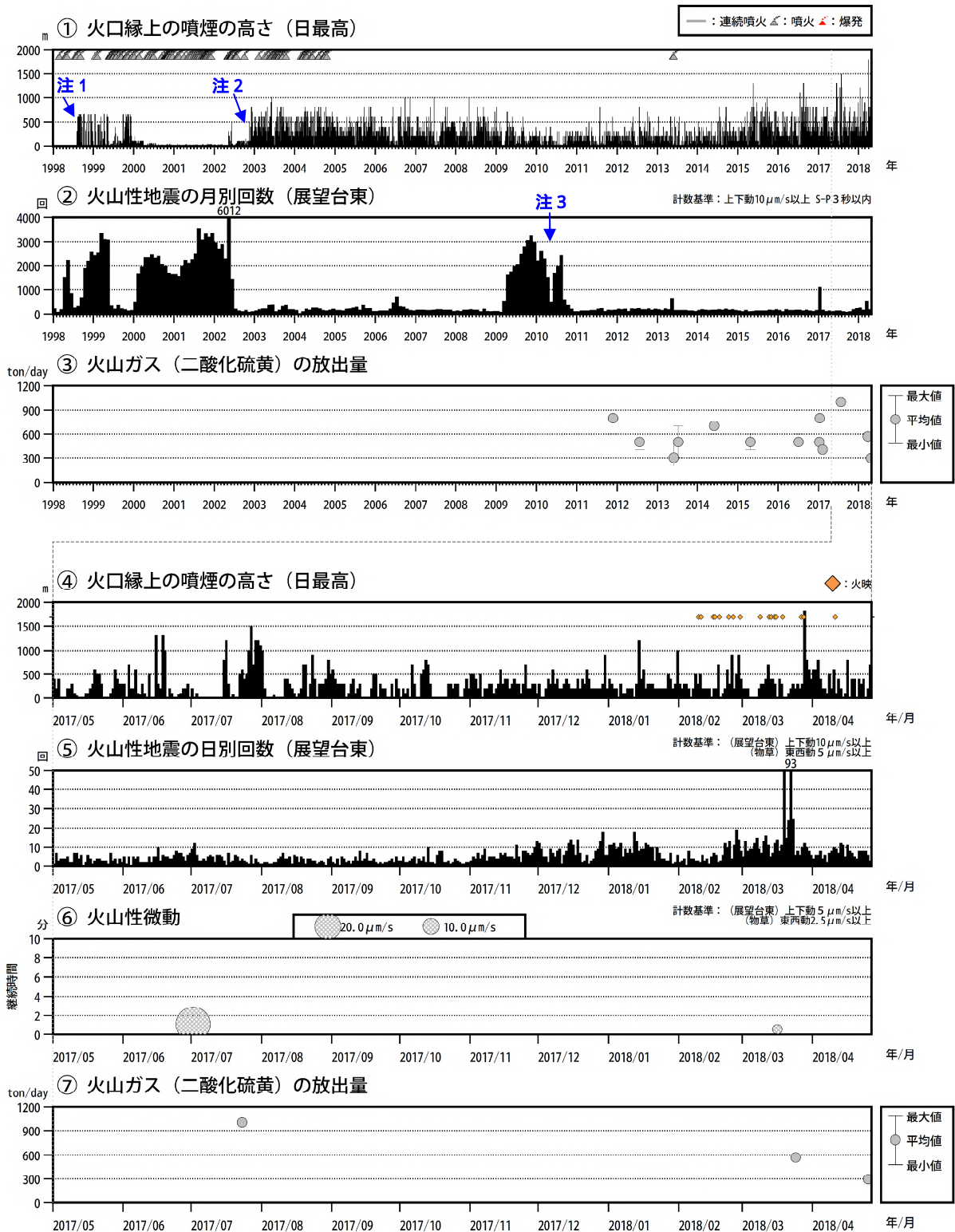
図 4 薩摩硫黄島 火山活動経過図 (1998 年 1 月 ~ 2018 年 4 月 26 日)
