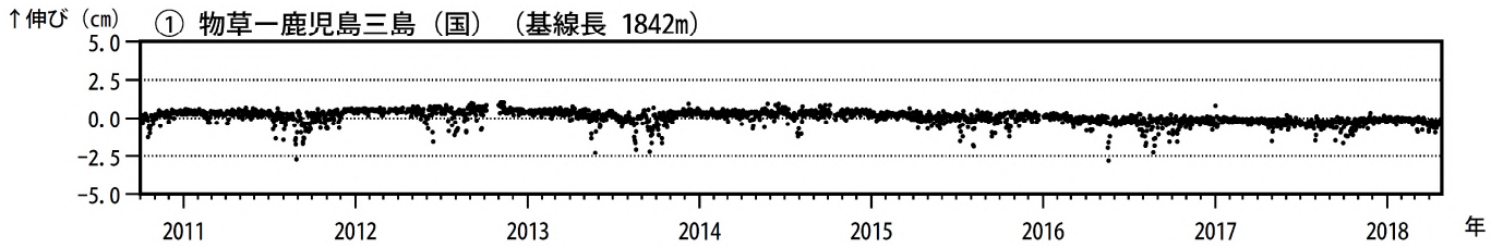
図 5 薩摩硫黄島 GNSS連続観測による基線長変化 (2010 年 10 月 ~ 2018 年 4 月 26 日)
