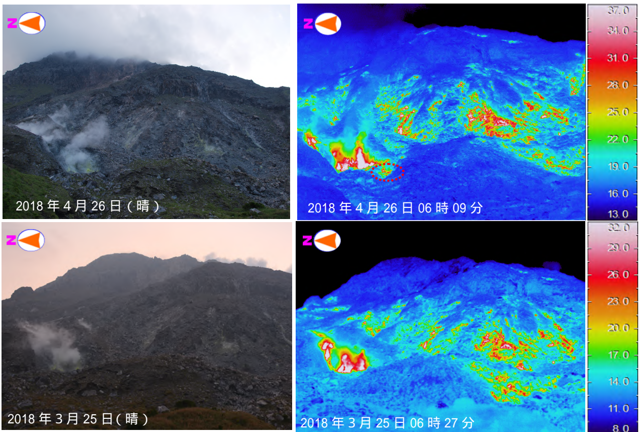
図 3 薩摩硫黄島 硫黄岳西側の状況（砂防ダム上流左岸から観測） （上段：2018 年 4 月 26 日、下段：2018 年 3 月 25 日） 噴気の状態に特段の変化は認められませんでした。が、わずかな熱異常域の広がり（赤破線）を確認しました。
