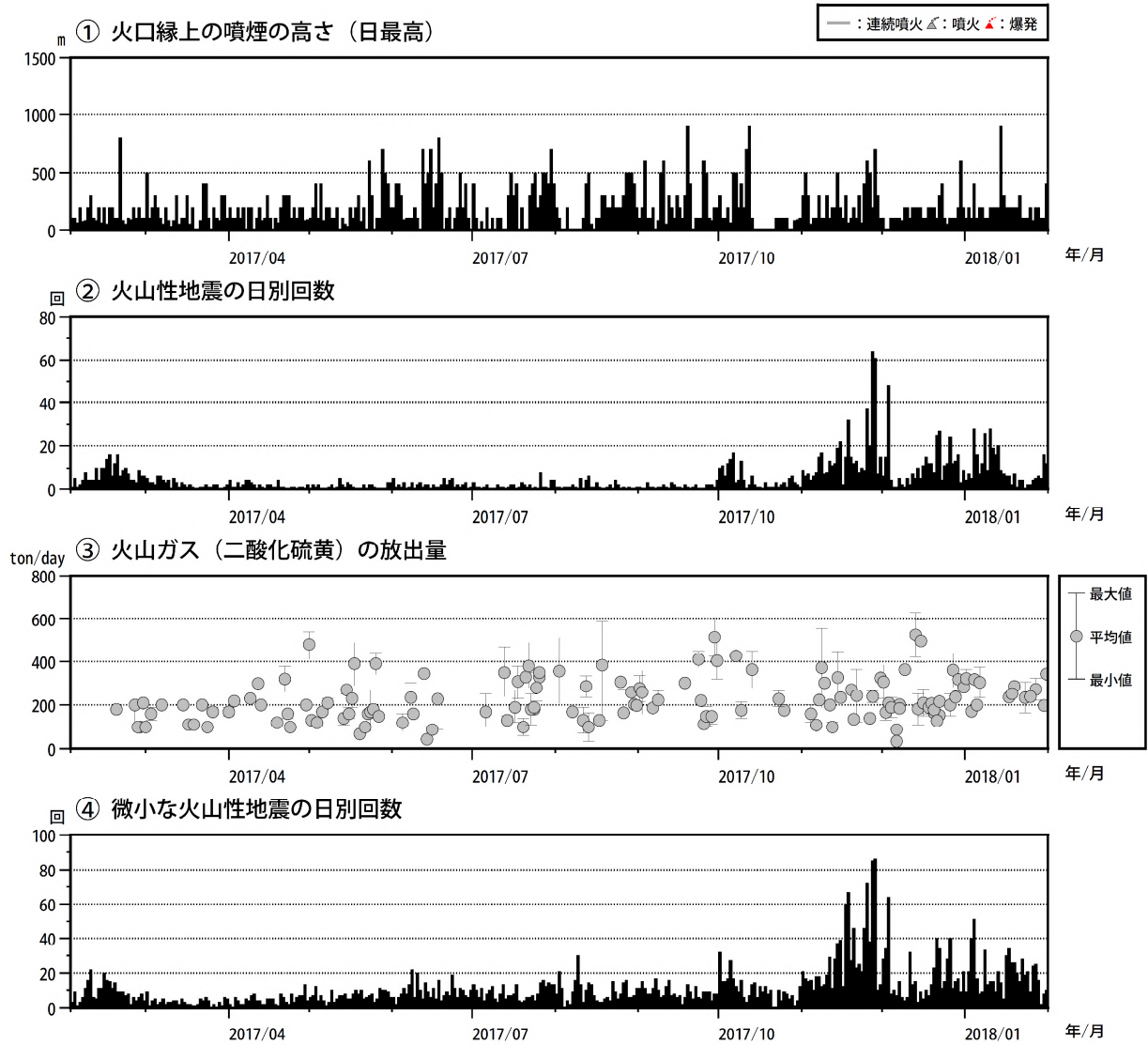
図5 口永良部島 最近の火山活動経過図(2017年2月~2018年1月)
