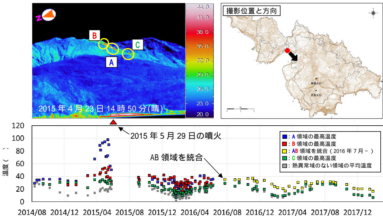
図3 口永良部島 新岳西斜面の熱異常域の温度時系列(2014年8月~2018年1月)
