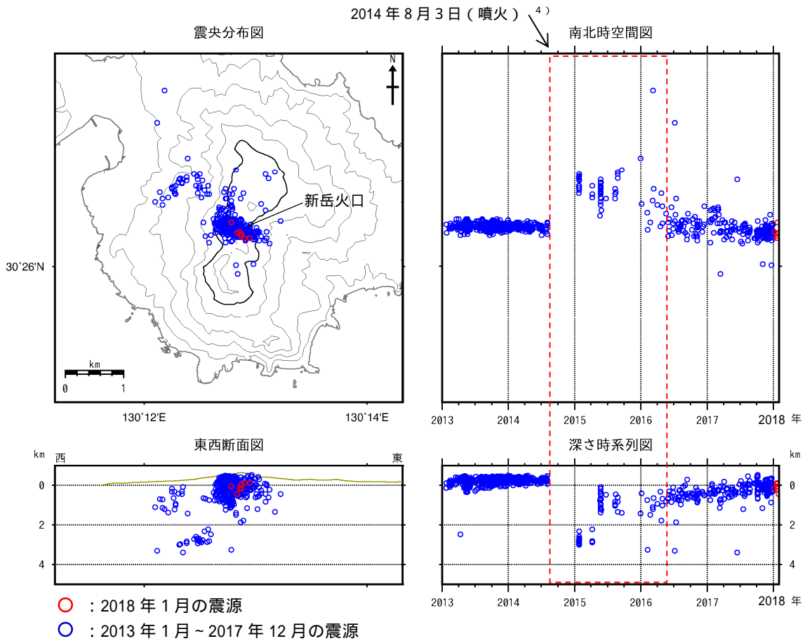
図6 口永良部島 震源分布図(2013年1月~2018年1月)
