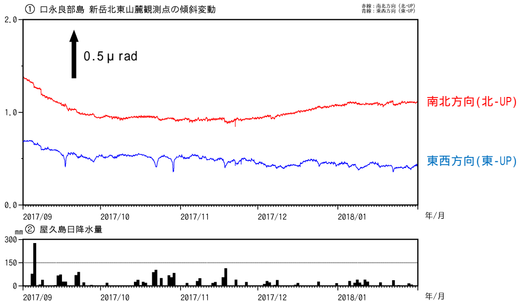
図7 口永良部島 新岳北東山麓観測点の傾斜変動(2017年9月~2018年1月)
