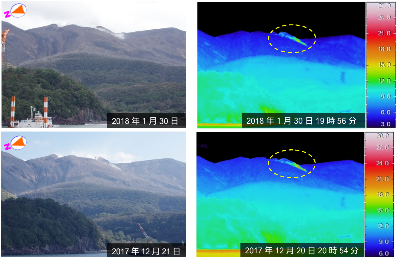
図2 口永良部島 本村から撮影した新岳火口及び新岳火口西側割れ目付近の可視画像と地表面温度分布 前月(12月20日、21日)と比較して、噴気及び熱異常域(黄色破線)に特段の変化は認められませんでした。
