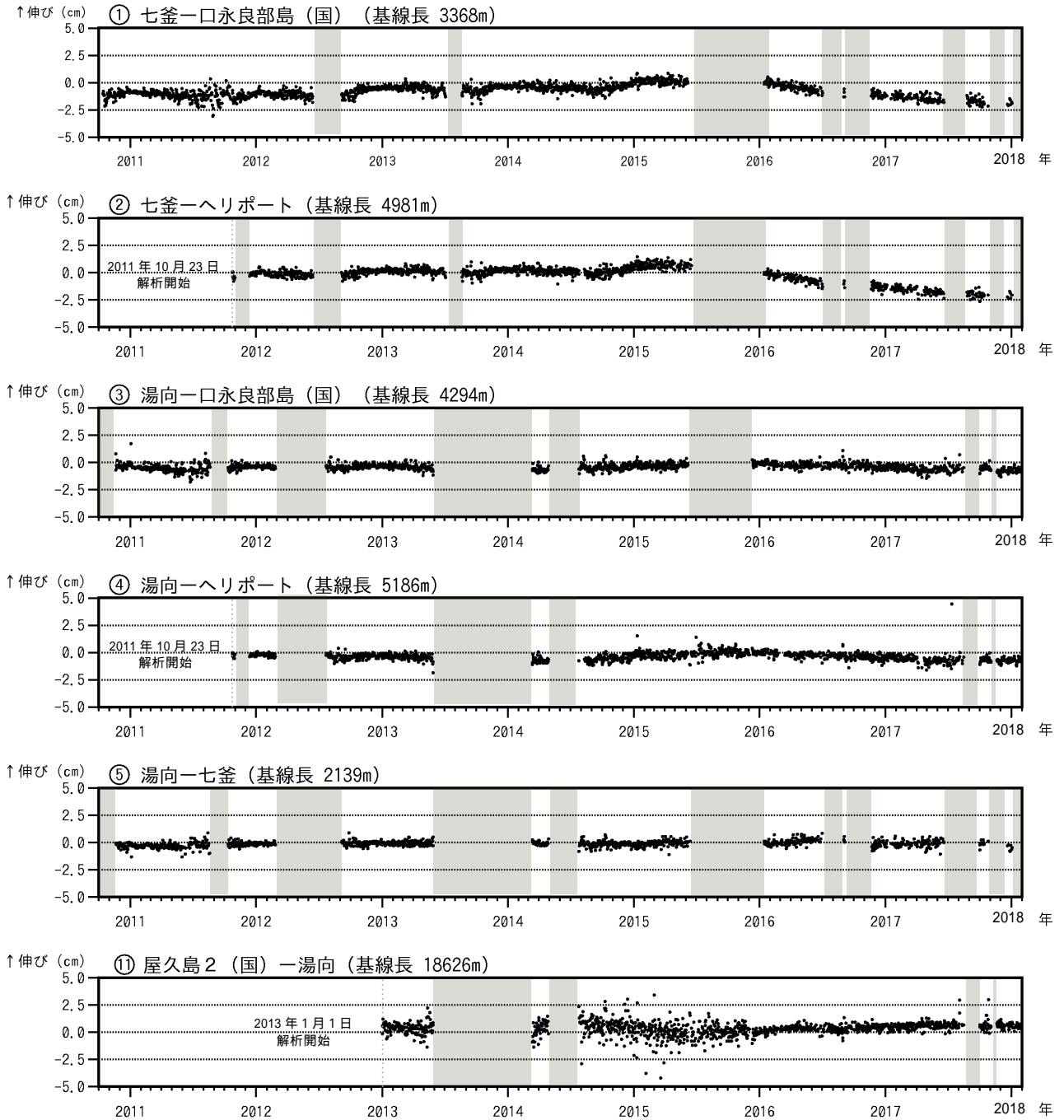
図8 口永良部島 GNSS連続観測による基線長変化(2010年10月~2018年1月)
