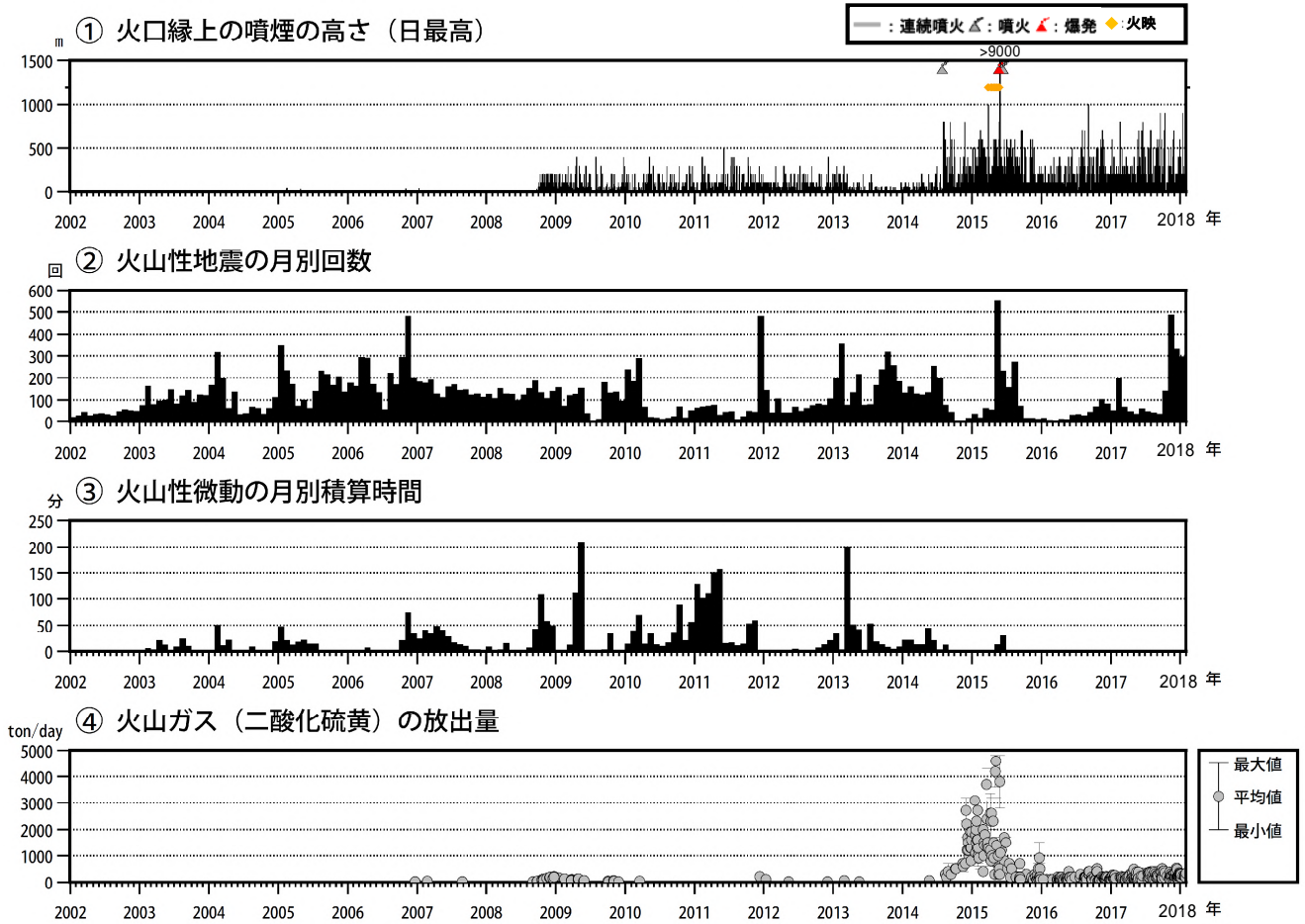
図 4 口永良部島 火山活動経過図（2002 年 1 月～2018 年 1 月）
