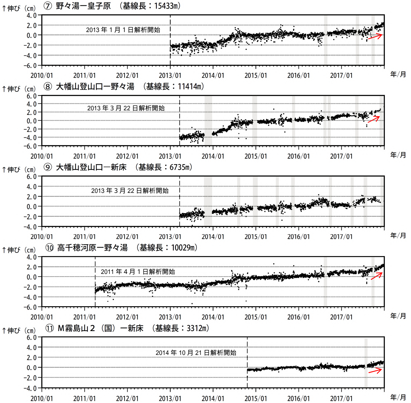
図 9-2 霧島山（新燃岳） GNSS 連続観測による基線長変化（2010 年 1 月～2017 年 12 月）
