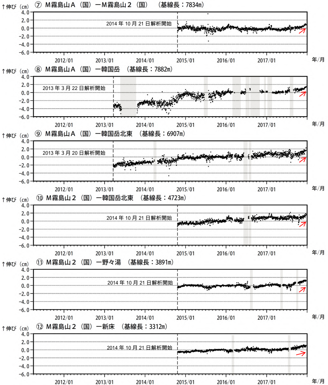
図 9-2 霧島山(えびの高原(硫黄山)周辺) GNSS 連続観測による基線長変化 (2011年4月~2017年12月)
