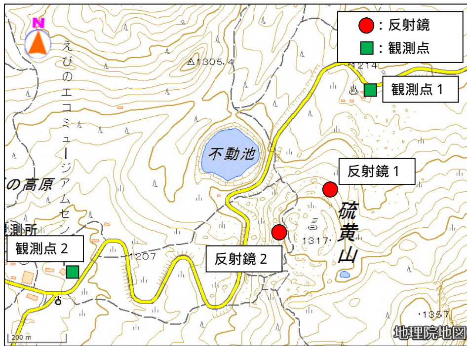
図 5 霧島山（えびの高原（硫黄山）周辺） 光波測距観測点配置図
