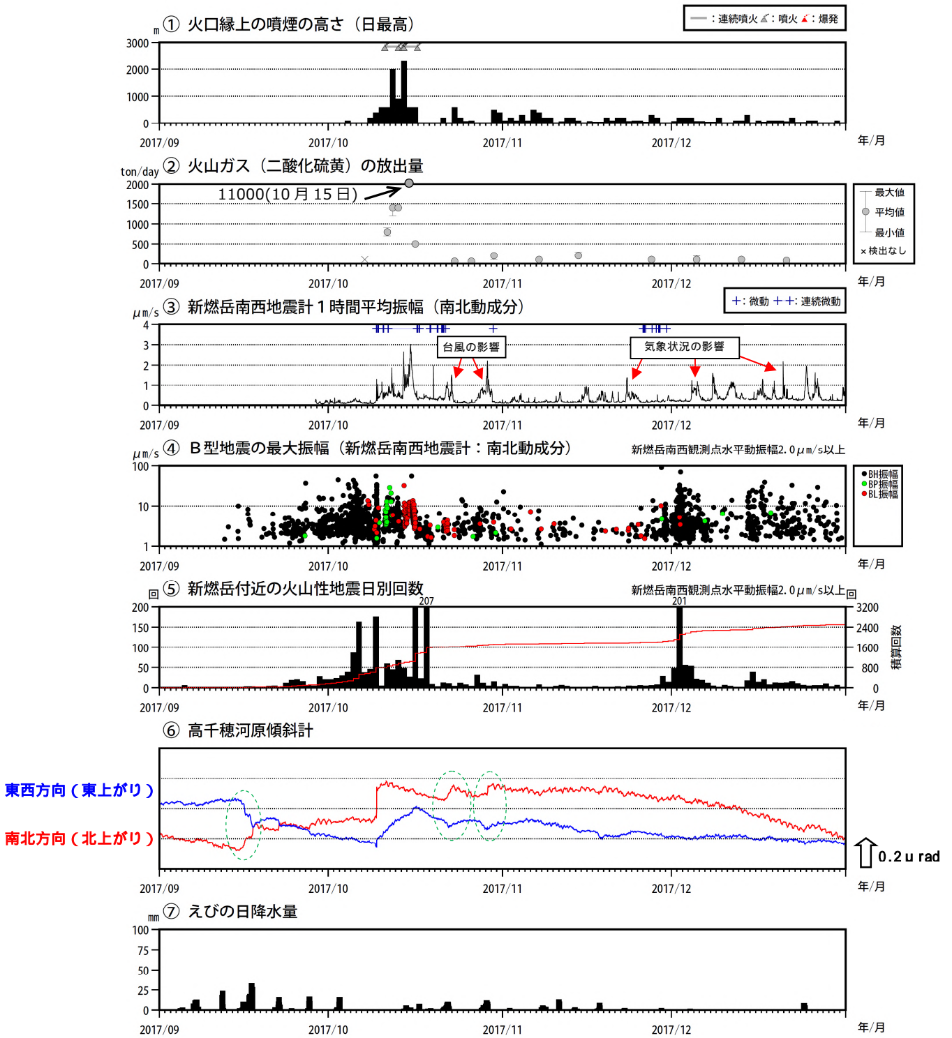
図 7 霧島山（新燃岳） 火山活動経過図（2017 年 9 月～12 月）
