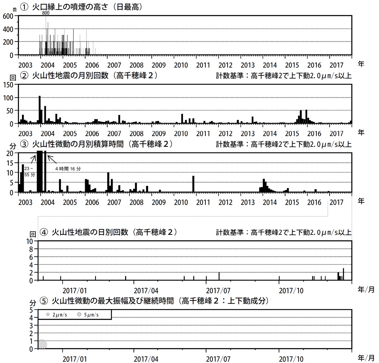
図2 霧島山（御鉢） 火山活動経過図（2003年1月～2017年12月）
