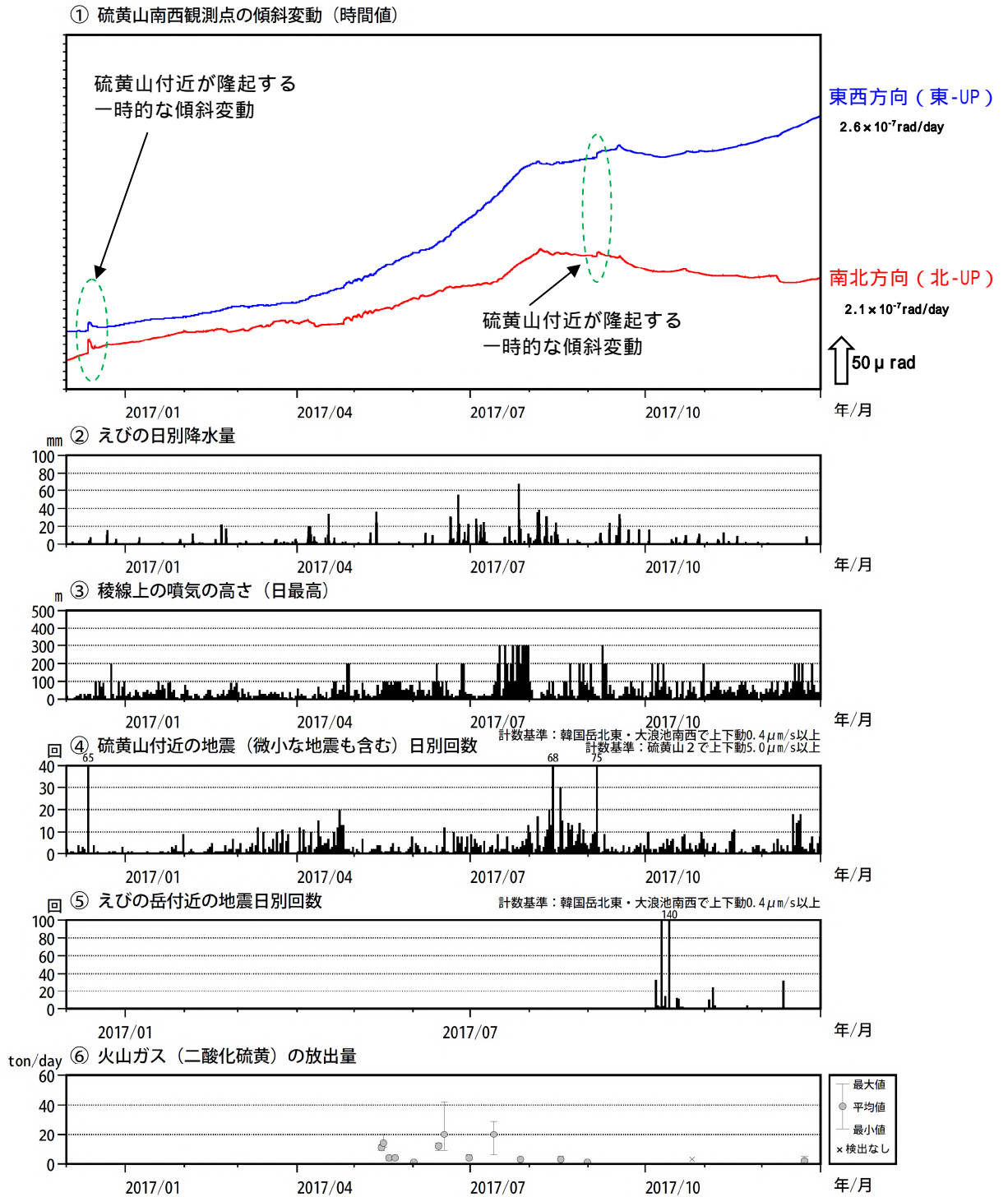
図 2 霧島山（えびの高原（硫黄山）周辺） 硫黄山南西傾斜計の傾斜変動と火山活動経過図 （2016 年 12 月～2017 年 12 月）
