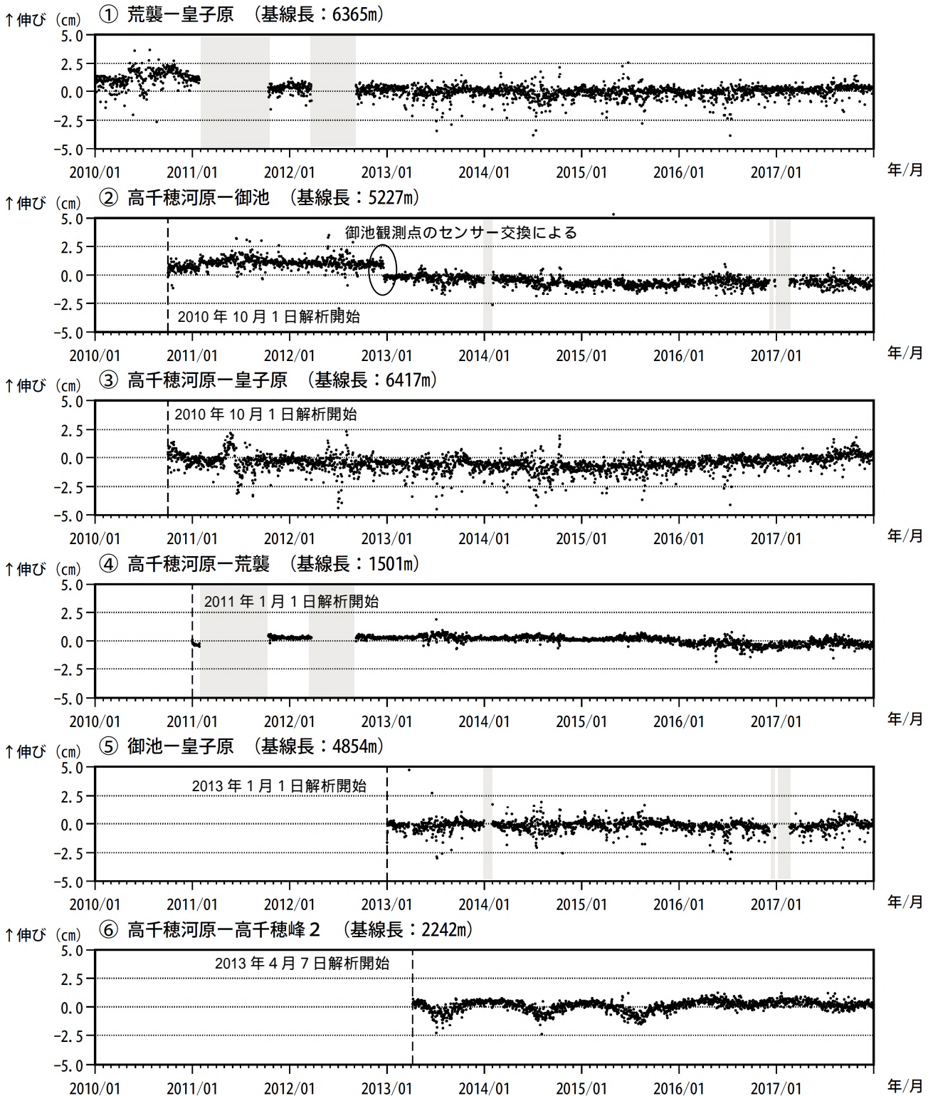
図3 霧島山（御鉢） GNSS連続観測による基線長変化（2010年1月～2017年12月）
