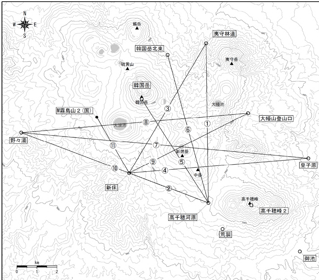
図 10 霧島山（新燃岳） GNSS 連続観測点と基線番号
