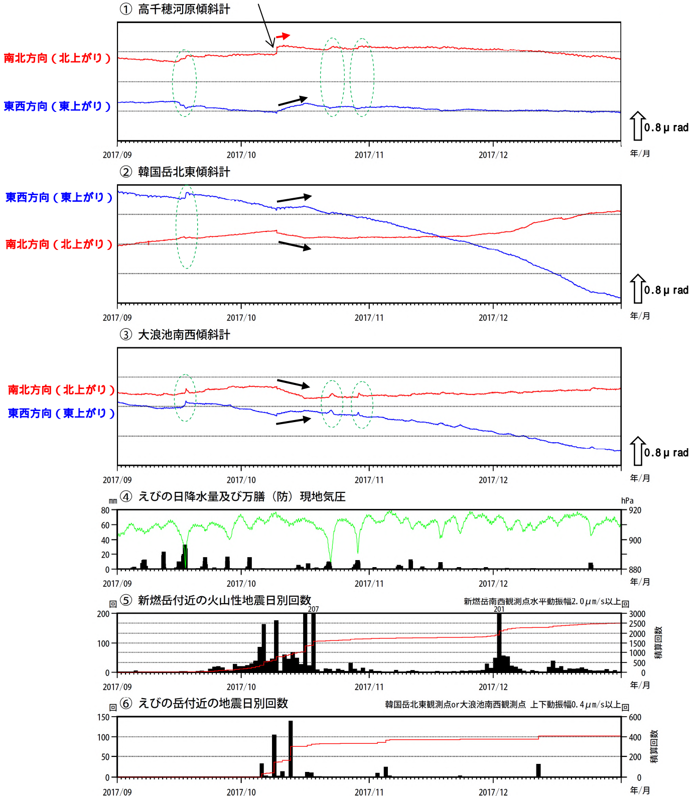
図 8 霧島山（新燃岳） 傾斜変動と火山性地震の日別回数（2017年9月～12月）
