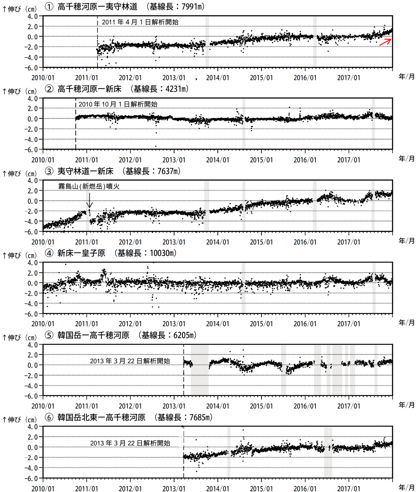
図9-1 霧島山(新燃岳) GNSS連続観測による基線長変化(2010年1月~2017年12月)
