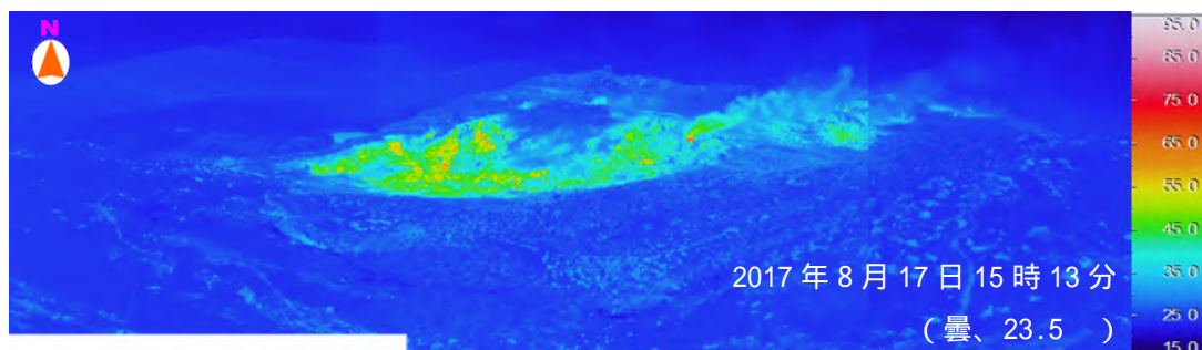
図 7 霧島山（えびの高原（硫黄山）周辺） 硫黄山南側斜面の状況
