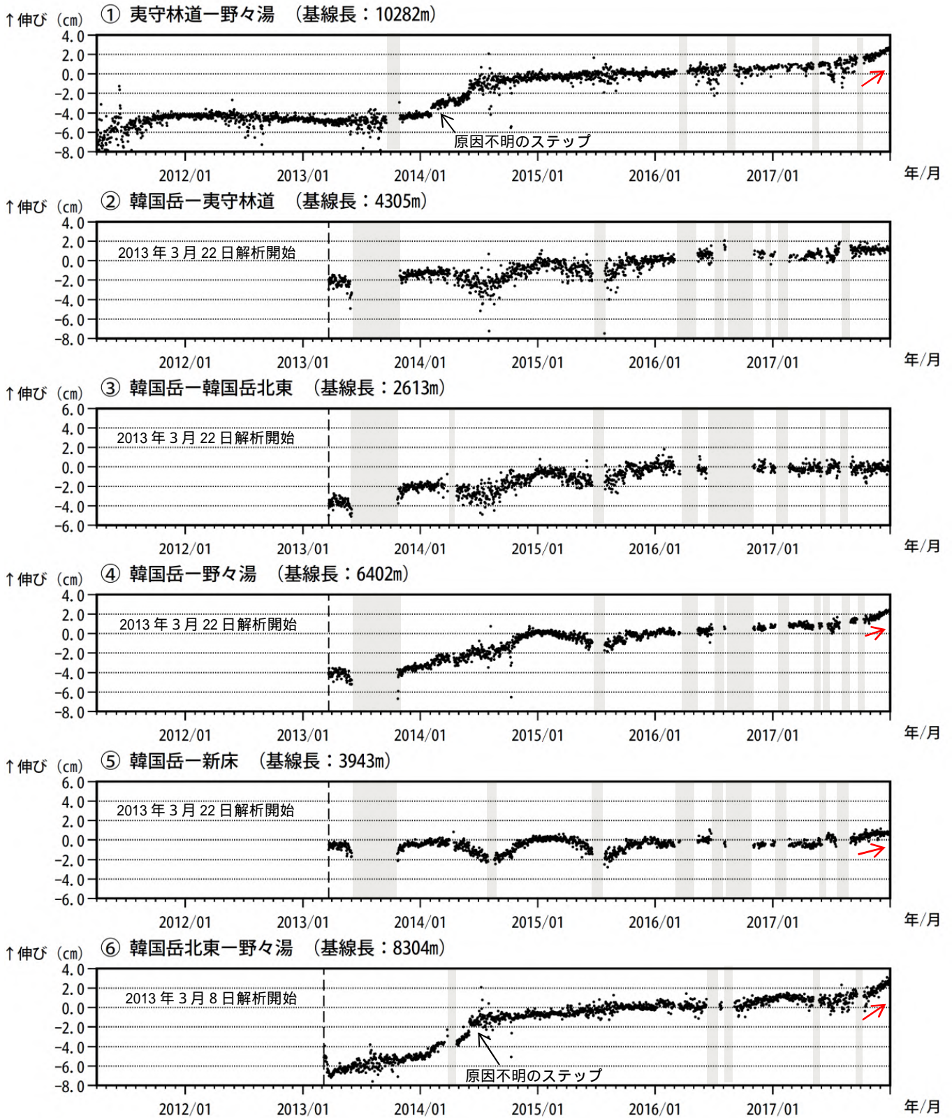
図 9-1 霧島山(えびの高原(硫黄山)周辺) GNSS 連続観測による基線長変化 (2011年4月~2017年12月)
