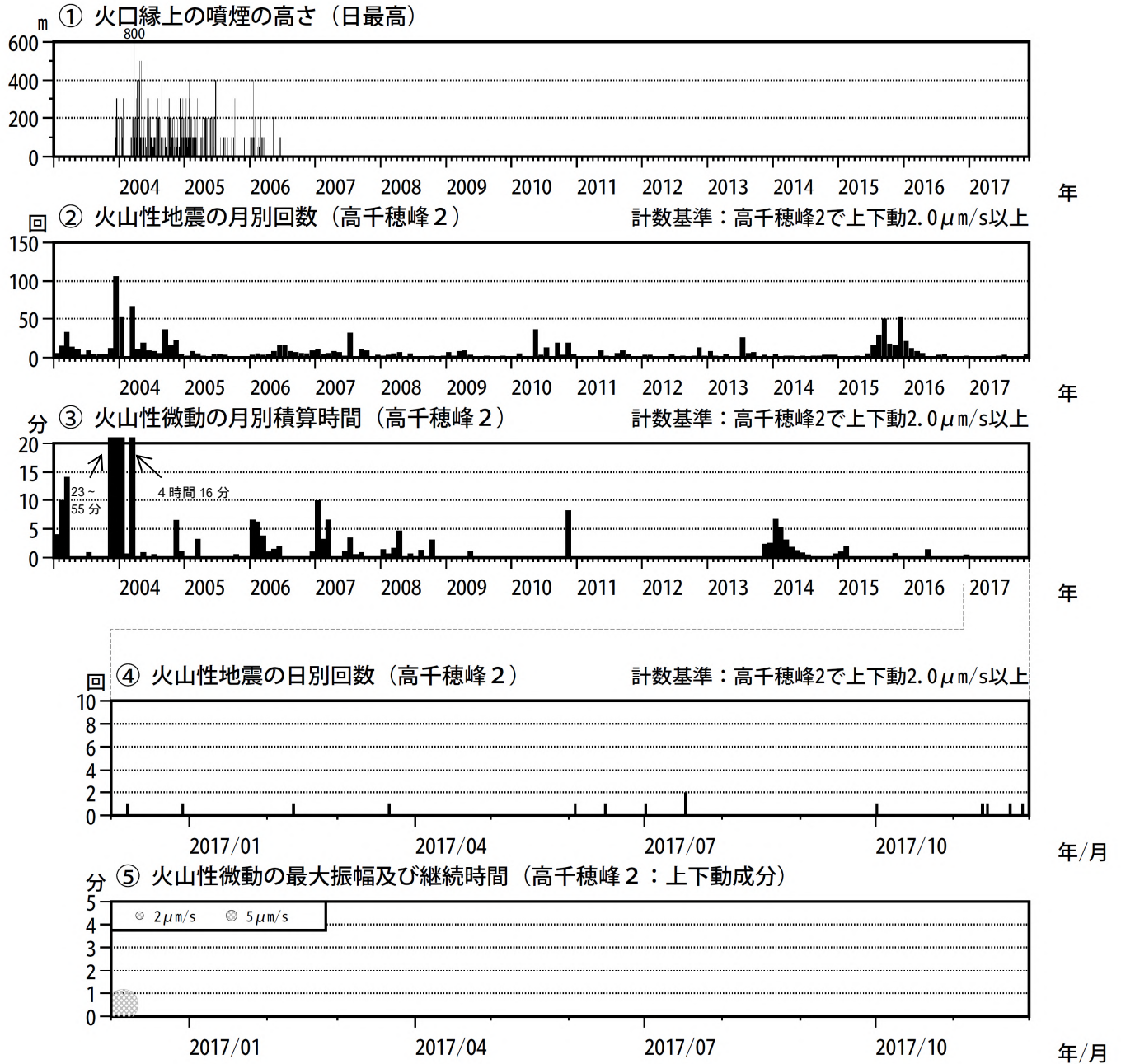
図2 霧島山（御鉢） 火山活動経過図（2003年1月～2017年11月）
