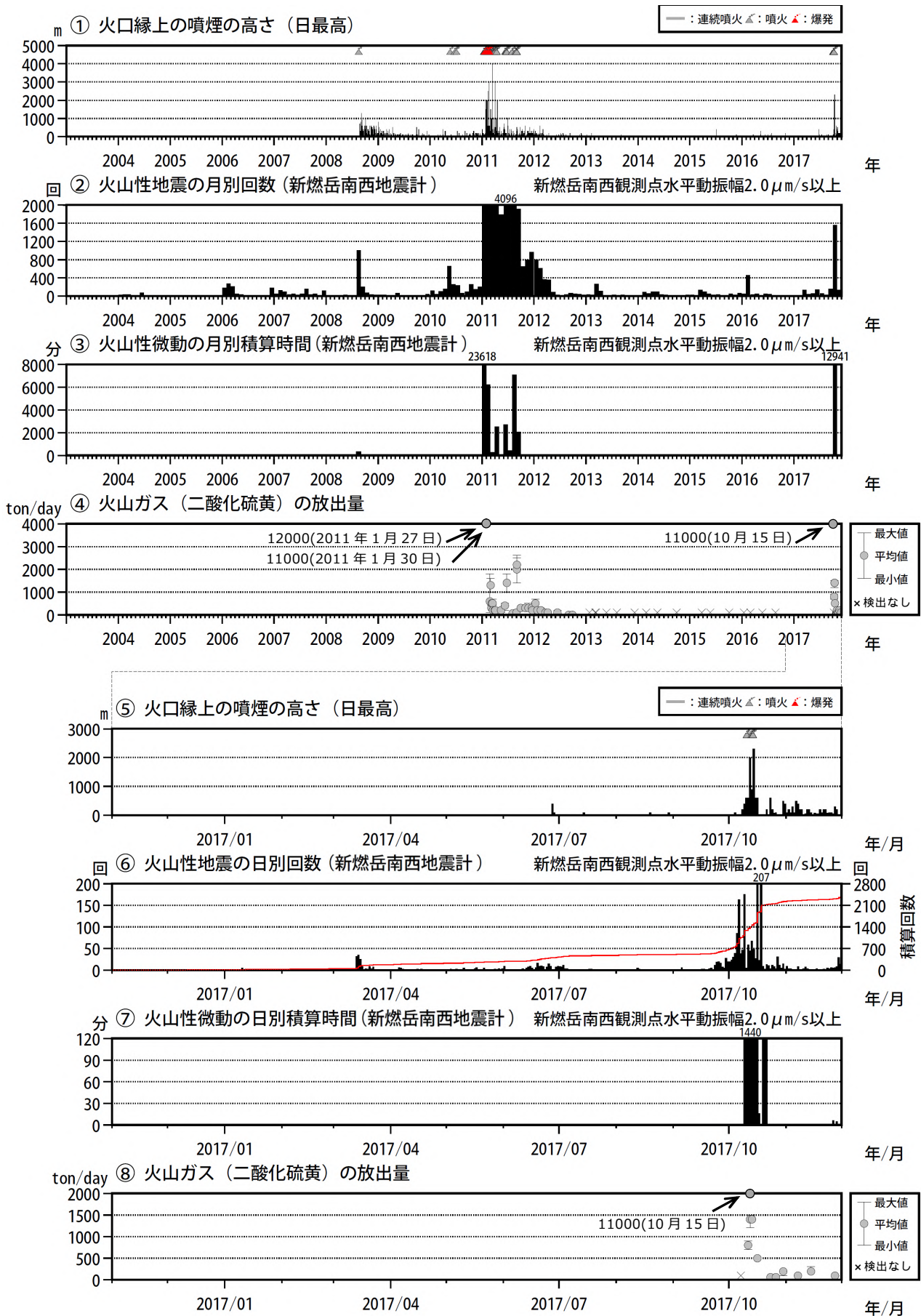
図6 霧島山（新燃岳） 火山活動経過図（2003年1月～2017年11月）
