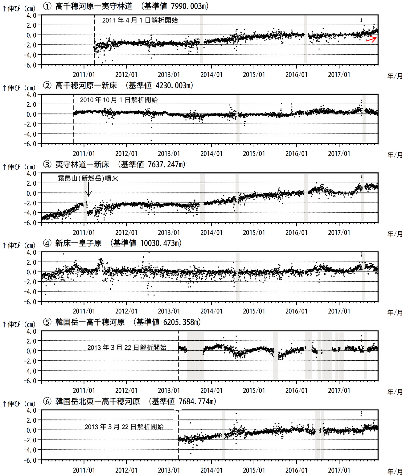
図 9-1 霧島山（新燃岳） GNSS 連続観測による基線長変化（2010 年 1 月～2017 年 11 月）
