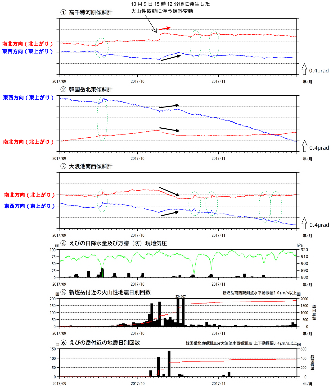
図 8 霧島山（新燃岳） 傾斜変動と火山性地震の日別回数（2017年9月～11月）
