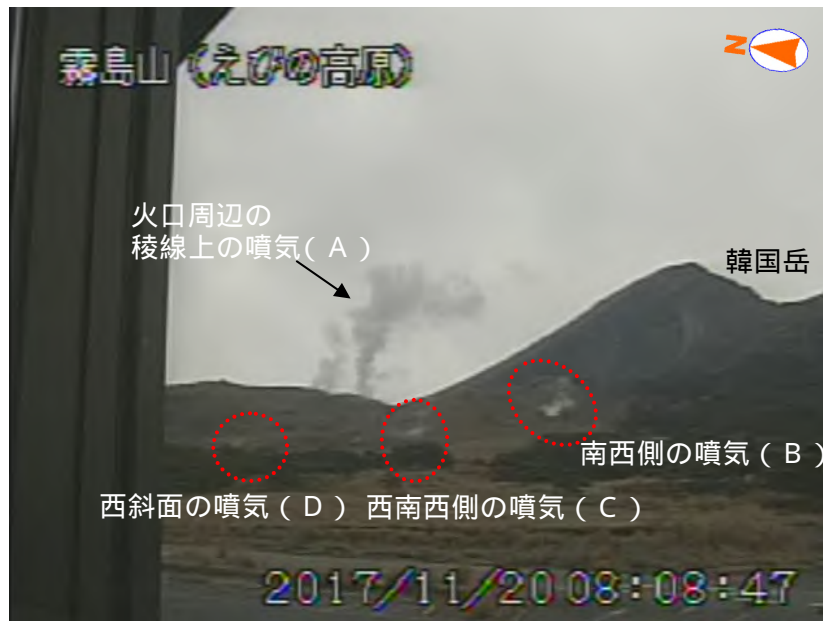
図 1 霧島山（えびの高原（硫黄山）周辺） 硫黄山付近の状況 （11 月 20 日 えびの高原監視カメラによる）
