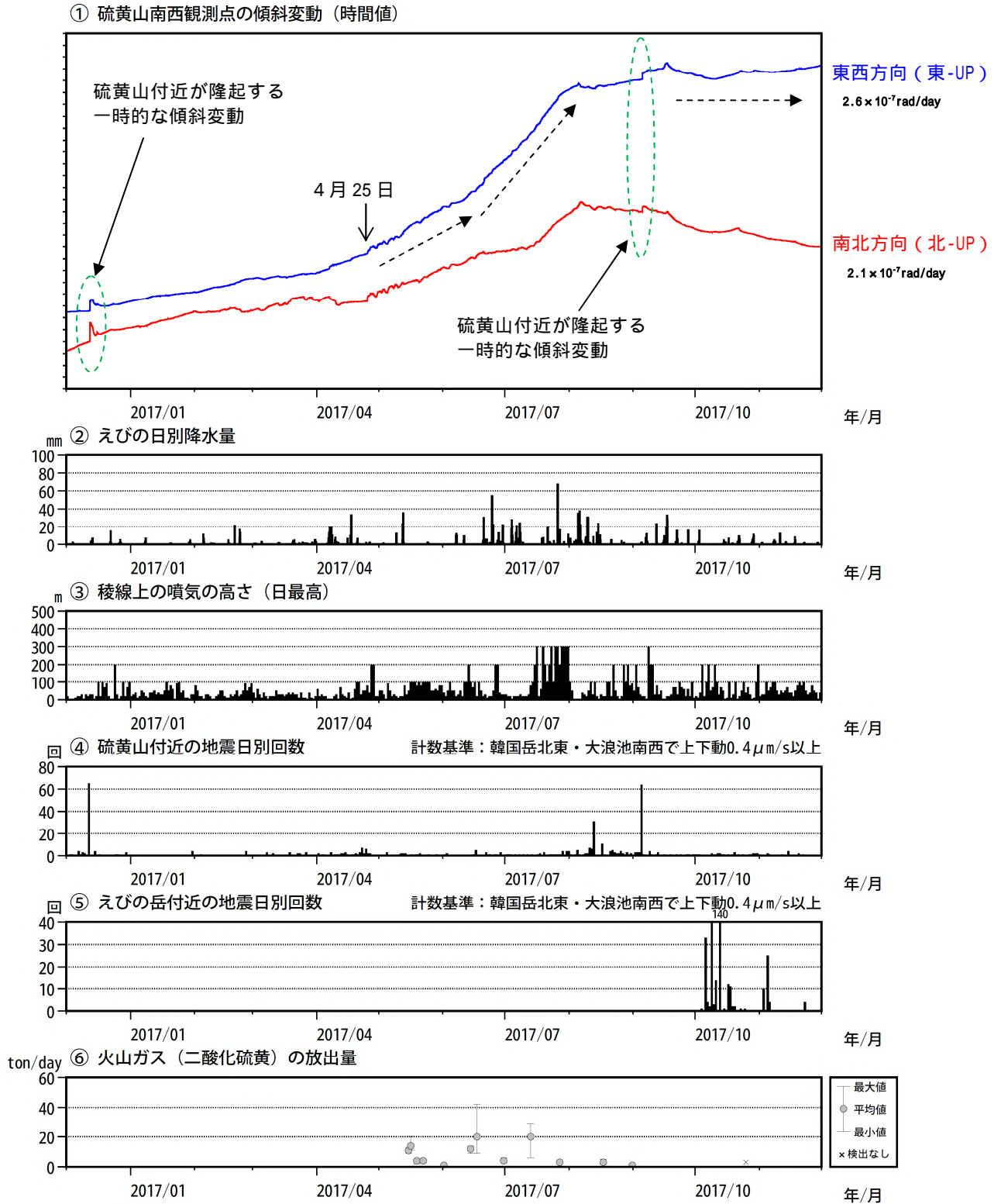
図3 霧島山（えびの高原（硫黄山）周辺） 硫黄山南西傾斜計の傾斜変動と火山活動経過図（2016年12月～2017年11月）
