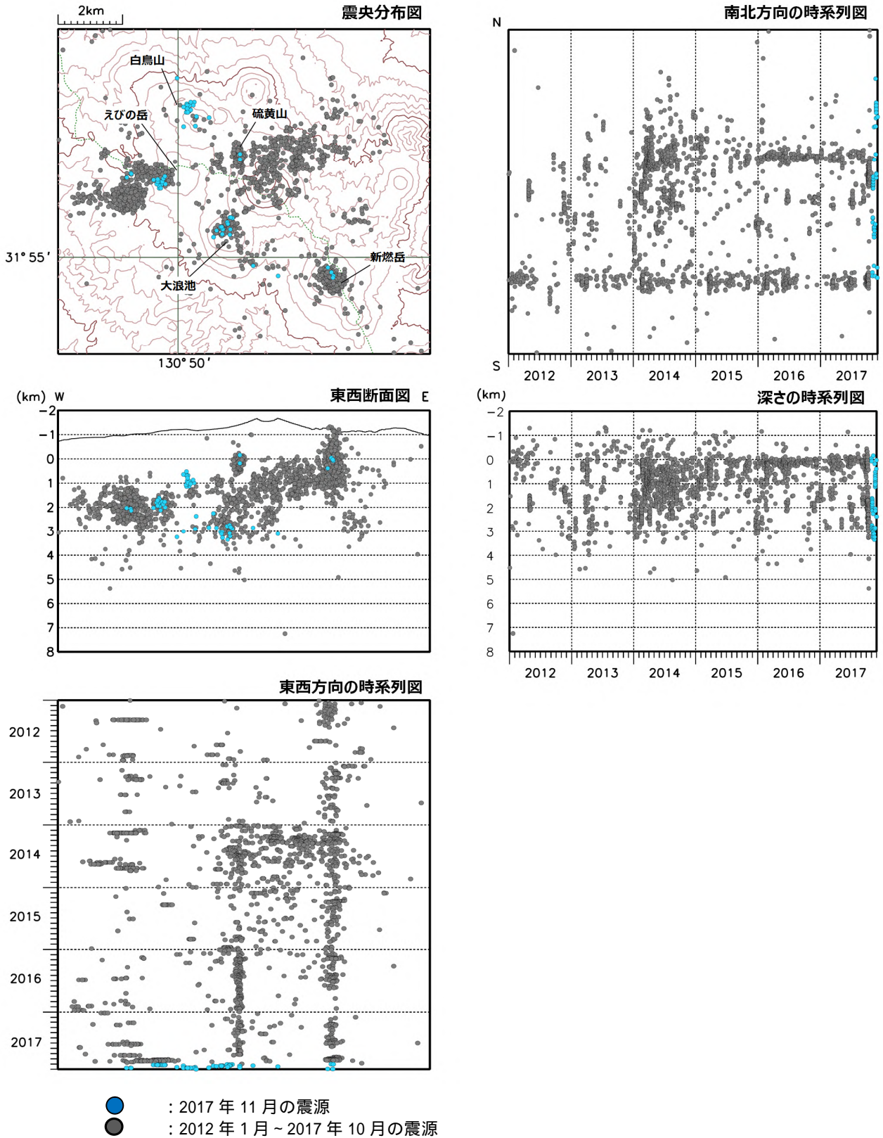
図 5 霧島山 新燃岳から硫黄山周辺の火山性地震の震源分布図 (2012 年 1 月 ~ 2017 年 11 月)
