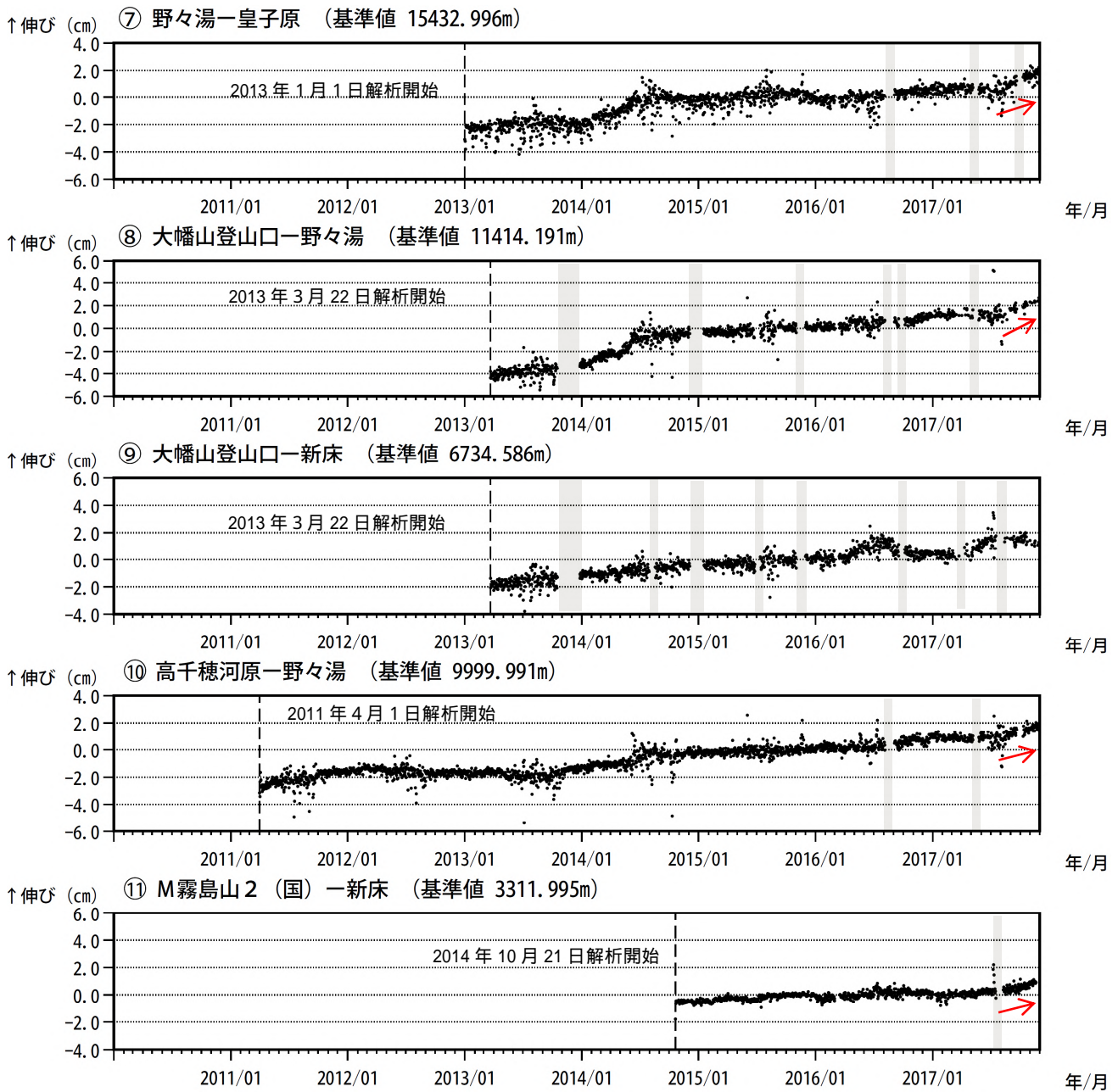
図 9-2 霧島山（新燃岳） GNSS 連続観測による基線長変化（2010 年 1 月～2017 年 11 月）
