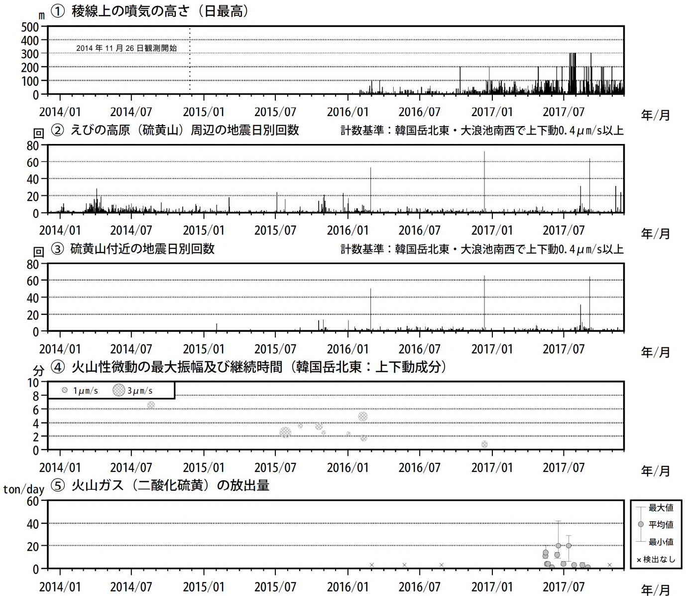
図4 霧島山（えびの高原（硫黄山）周辺） 火山活動経過図（2013年12月～2017年11月）
