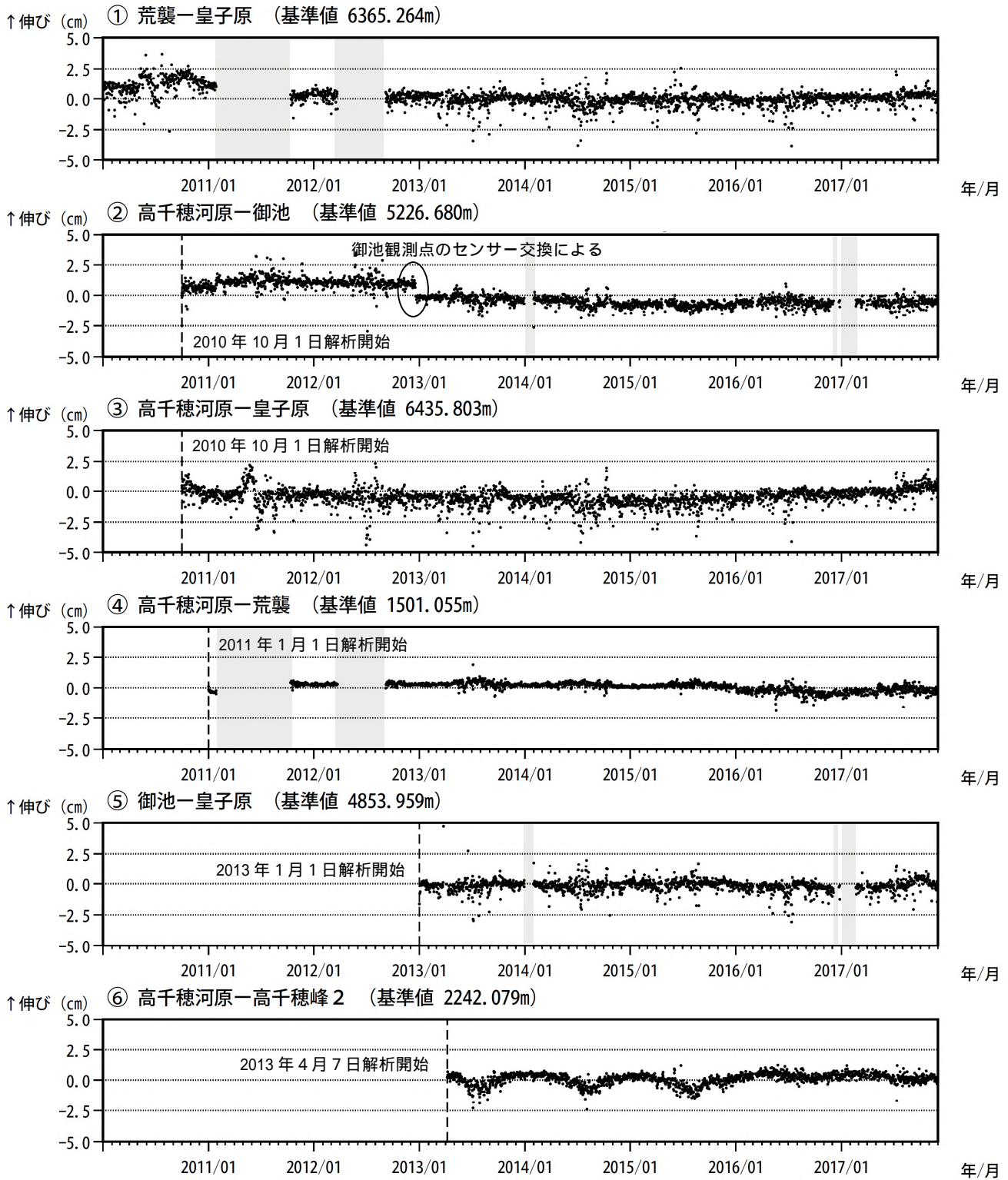
図3 霧島山（御鉢） GNSS 連続観測による基線長変化（2010年1月～2017年11月）
