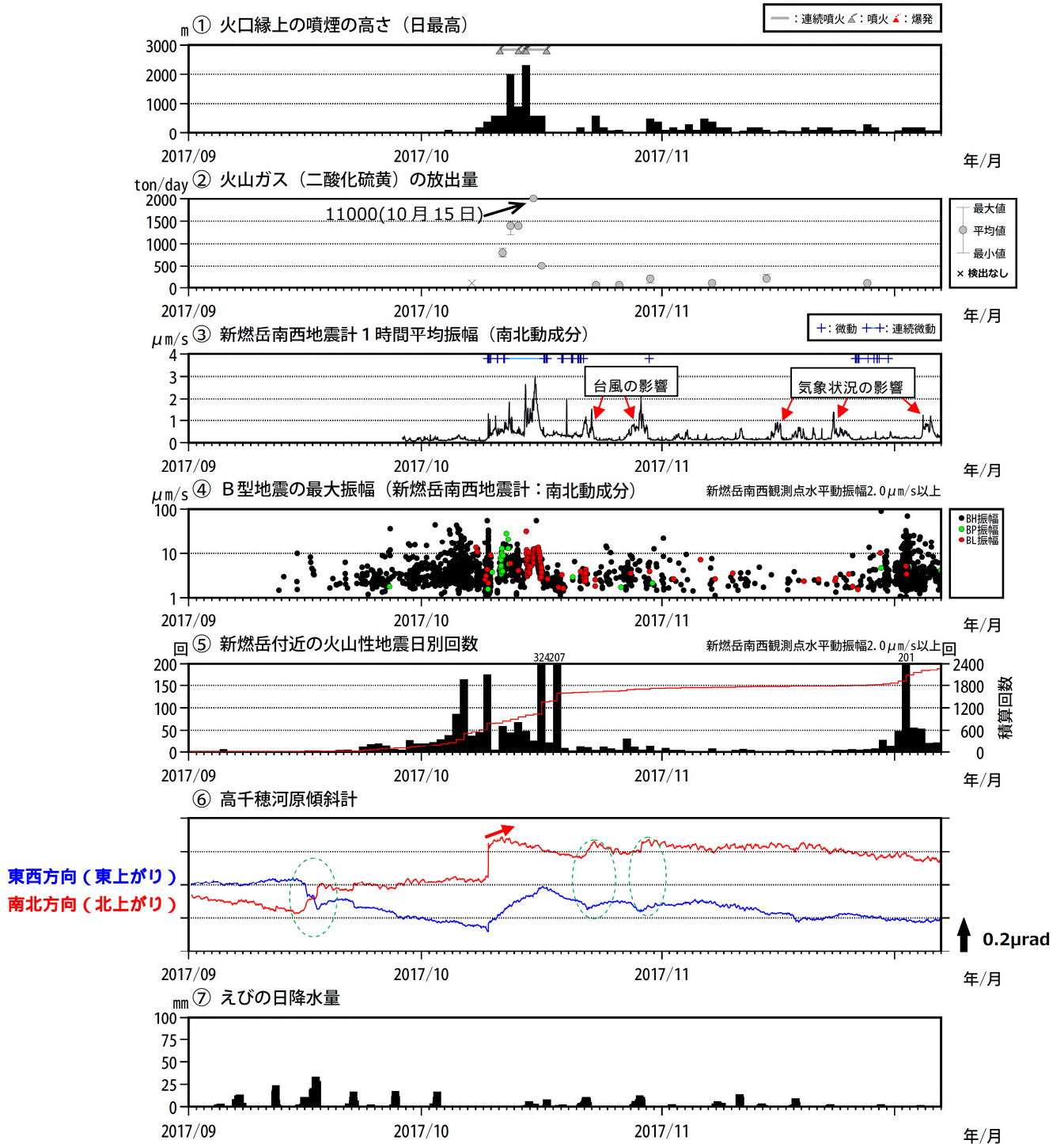
図 7 霧島山（新燃岳） 火山活動経過図（2017 年 9 月～12 月 6 日）
