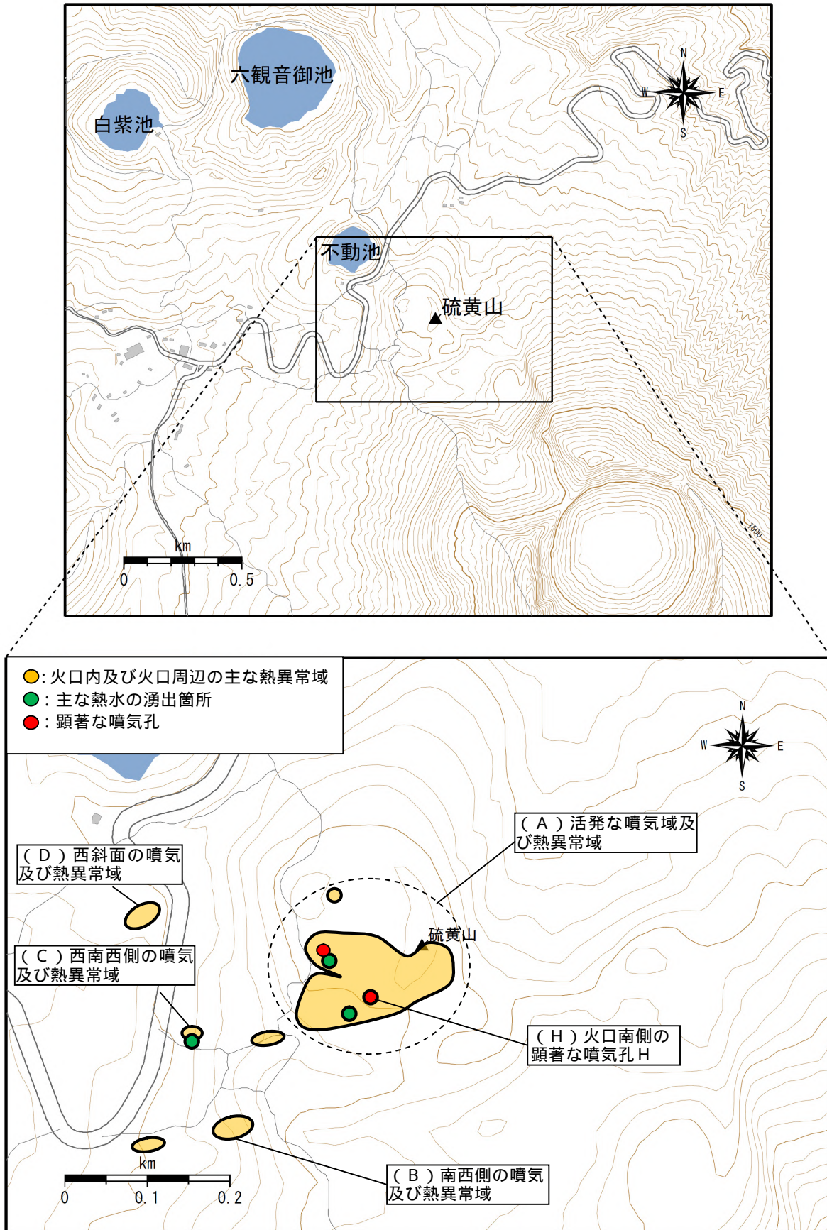
図6 霧島山（えびの高原(硫黄山)周辺） 主な噴気位置
