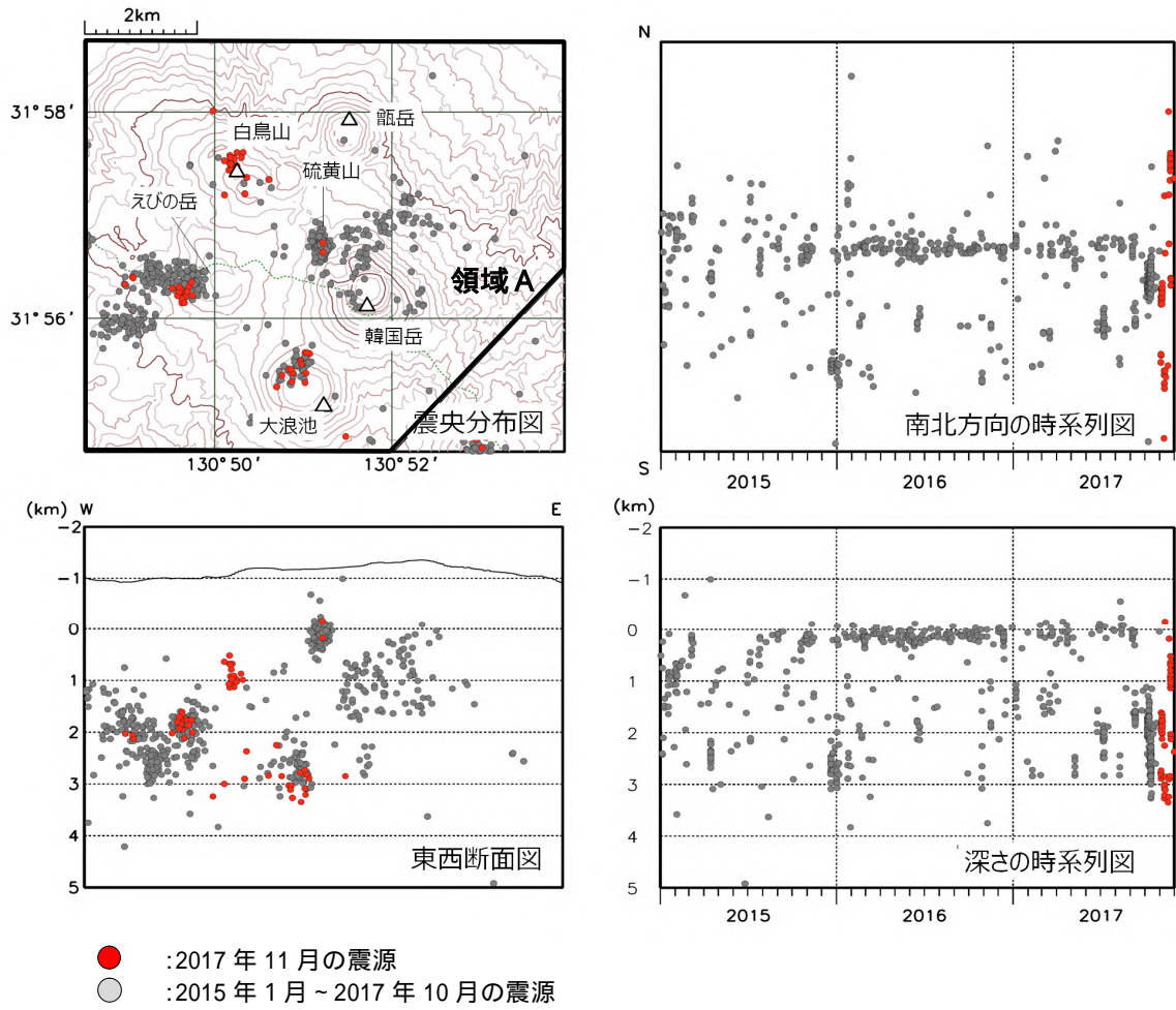
図 5 霧島山（えびの高原（硫黄山）周辺） 震源分布図（2015 年 1 月～2017 年 11 月）
