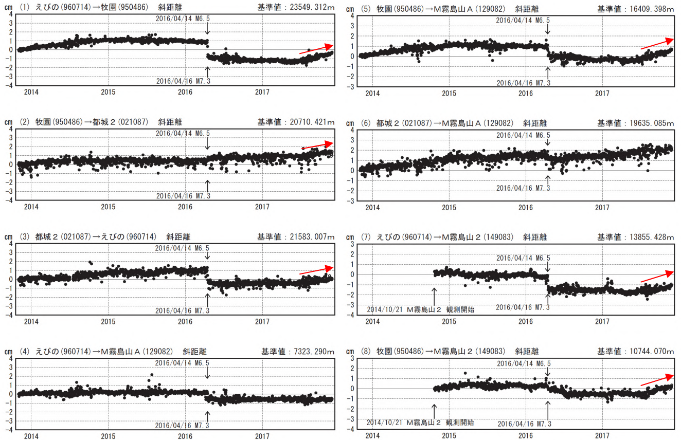
図11 霧島山 国土地理院による地殻変動観測結果（2013年11月1日～2017年11月27日）
