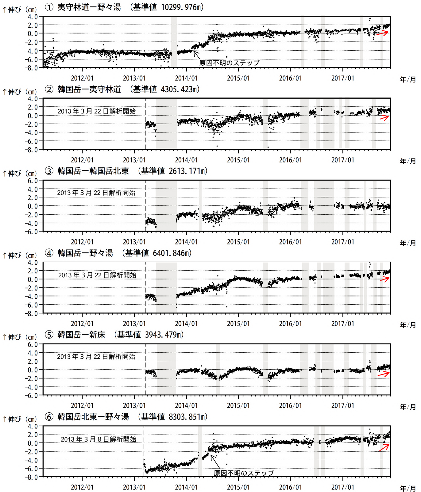
図 7-1 霧島山（えびの高原（硫黄山）周辺） GNSS 連続観測による基線長変化 （2011 年 4 月～2017 年 11 月）
