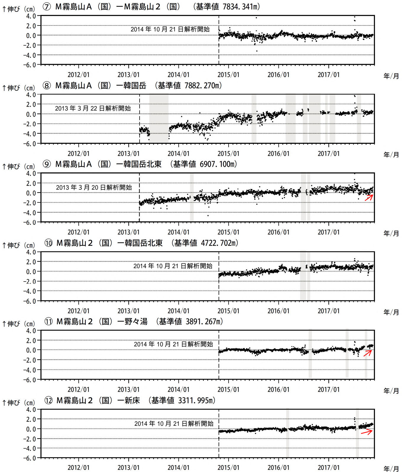
図 7-2 霧島山（えびの高原（硫黄山）周辺） GNSS 連続観測による基線長変化 （2011 年 4 月～2017 年 11 月）
