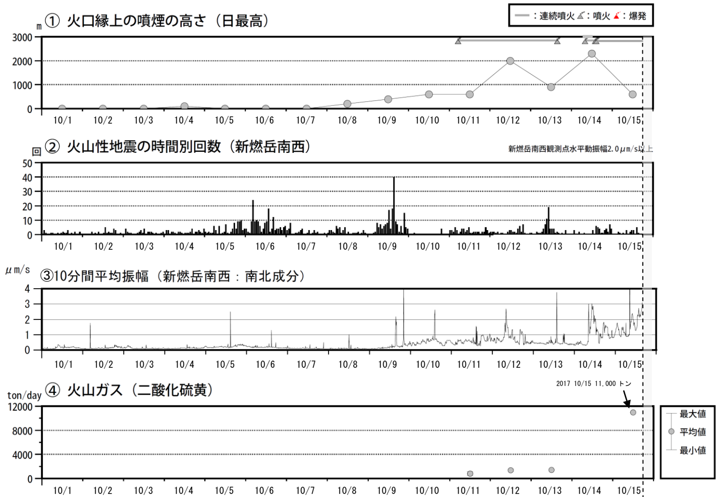
図 1 霧島山（新燃岳） 火山活動経過図（2017年10月1日～10月15日18時） 10月15日18時
