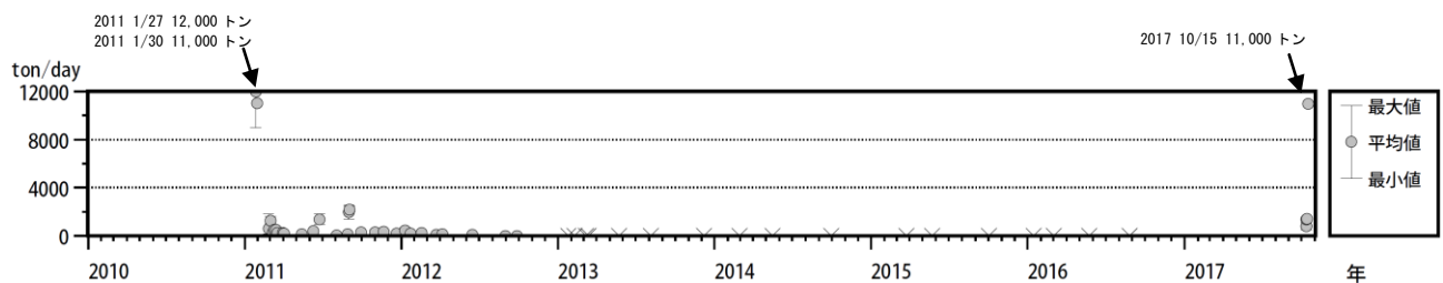
図 2 霧島山（新燃岳） 火山ガスの観測状況（2010年1月1日～2017年10月15日） 15日に実施した現地調査では、火山ガス（二酸化硫黄）の放出量は1日あたり11,000トン（前回13日1,400トン）と急増しました。 火山ガスの放出量が1日あたり10,000トンを超えたのは、2011年1月の本格的なマグマ噴火時以来です。 ×は検出限界未満を示す。
