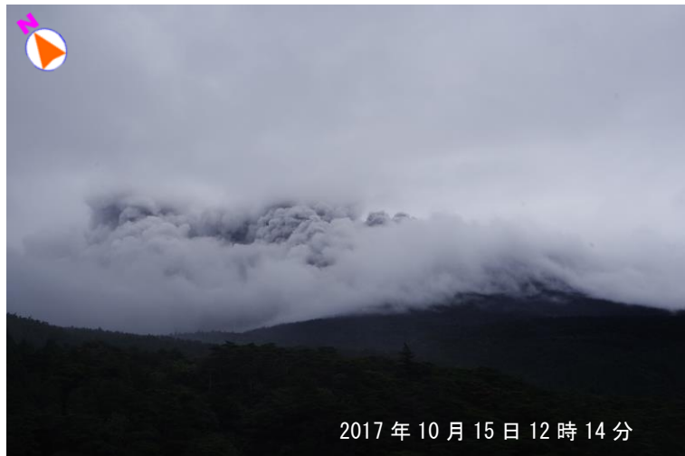
図 3 霧島山（新燃岳） 噴火の状況（新燃岳南西約 3 km の新湯温泉付近から観測） 灰白色の噴煙が雲に入るのを確認しました。
