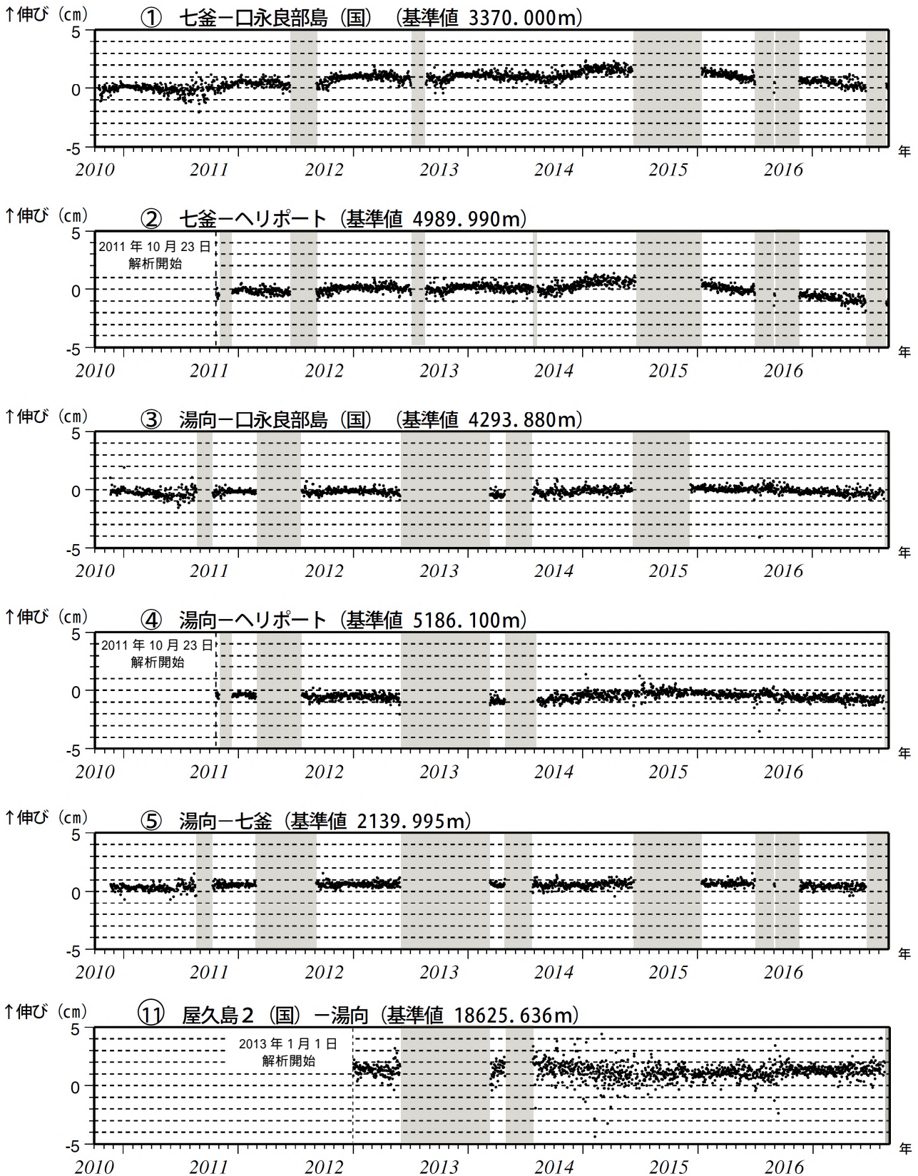
図7 口永良部島 GNSS 連続観測による基線長変化(2010年10月~2017年8月)
