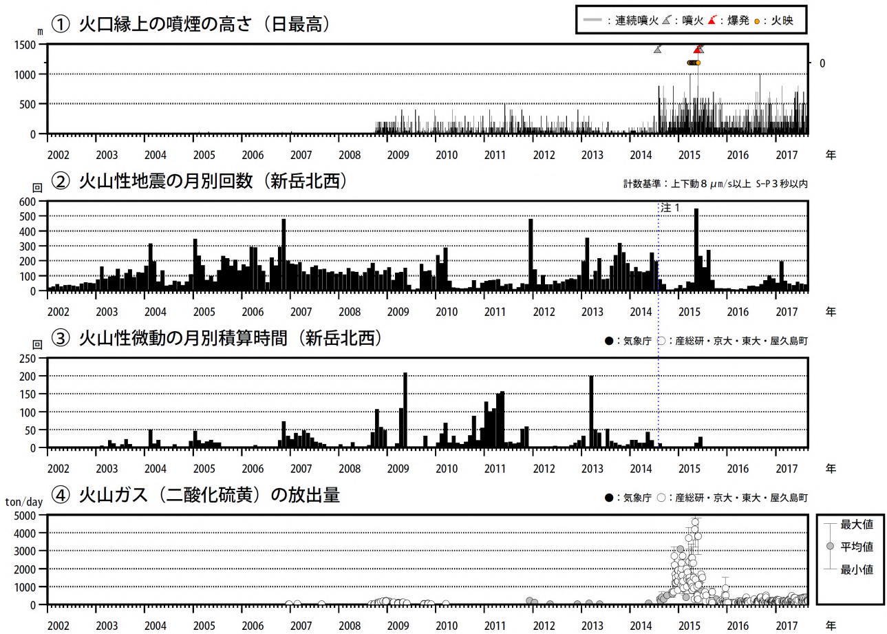
図4 口永良部島 火山活動経過図 (2002年1月～2017年8月)
