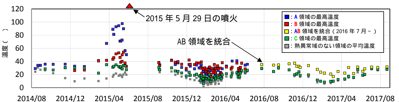
図3 口永良部島 新岳西斜面の熱異常域の温度時系列(2014年8月~2017年8月) < 8月の状況 >
