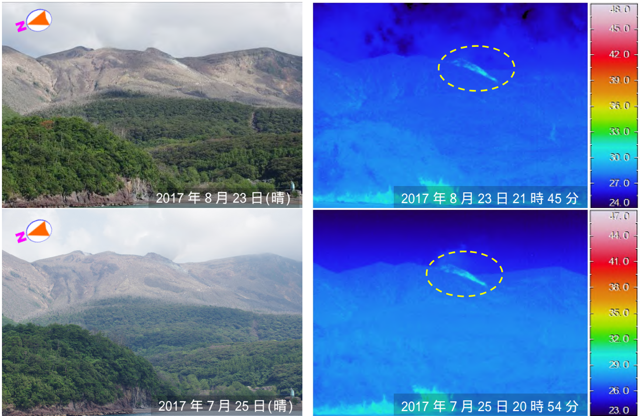
図2 口永良部島 本村から撮影した新岳火口及び新岳火口西側割れ目付近の可視画像と地表面温度分布 前月(7月25日)と比較して、噴気及び熱異常域(黄色破線)に特段の変化は認められませんでした。
