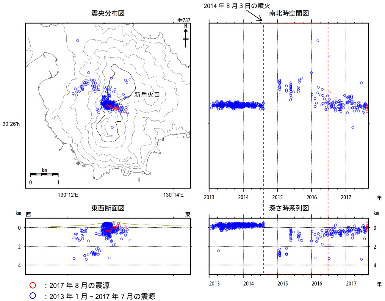
図 6 口永良部島 震源分布図(2013 年 1 月 ~ 2017 年 8 月)
