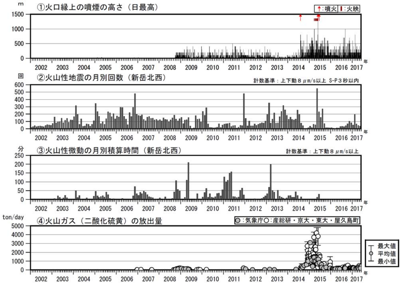
図 4 口永良部島 火山活動経過図（2002 年 1 月～2017 年 5 月）
