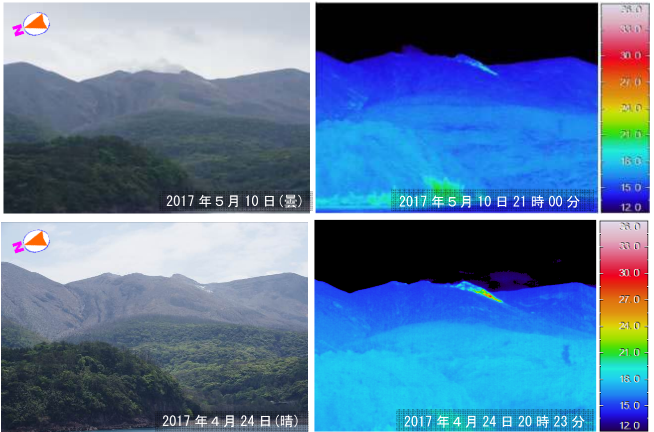
図 2 口永良部島 本村から撮影した可視画像と地表面温度分布 前月（4月24日）と比較して、噴気及び熱異常域に特段の変化は認められませんでした。
