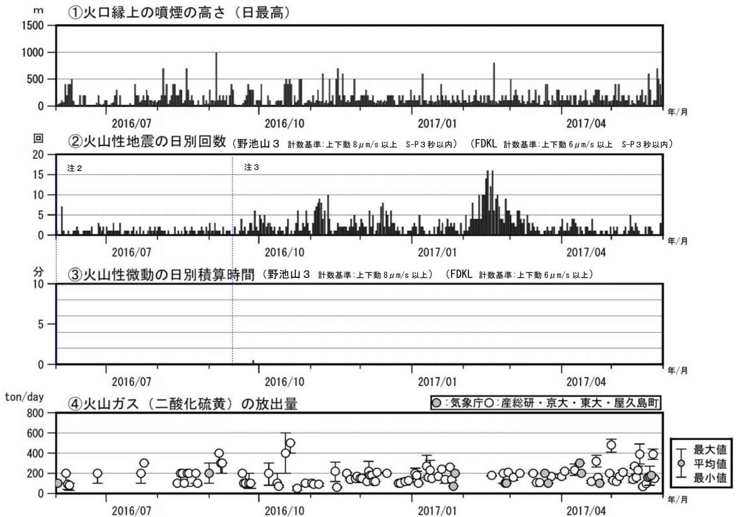
図5 口永良部島 最近の火山活動経過図（2016年6月～2017年5月）
