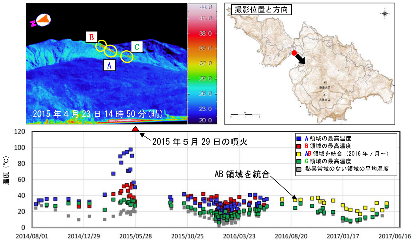
図 3 口永良部島 新岳西斜面の熱異常域の温度時系列（2014年8月～2017年5月）
