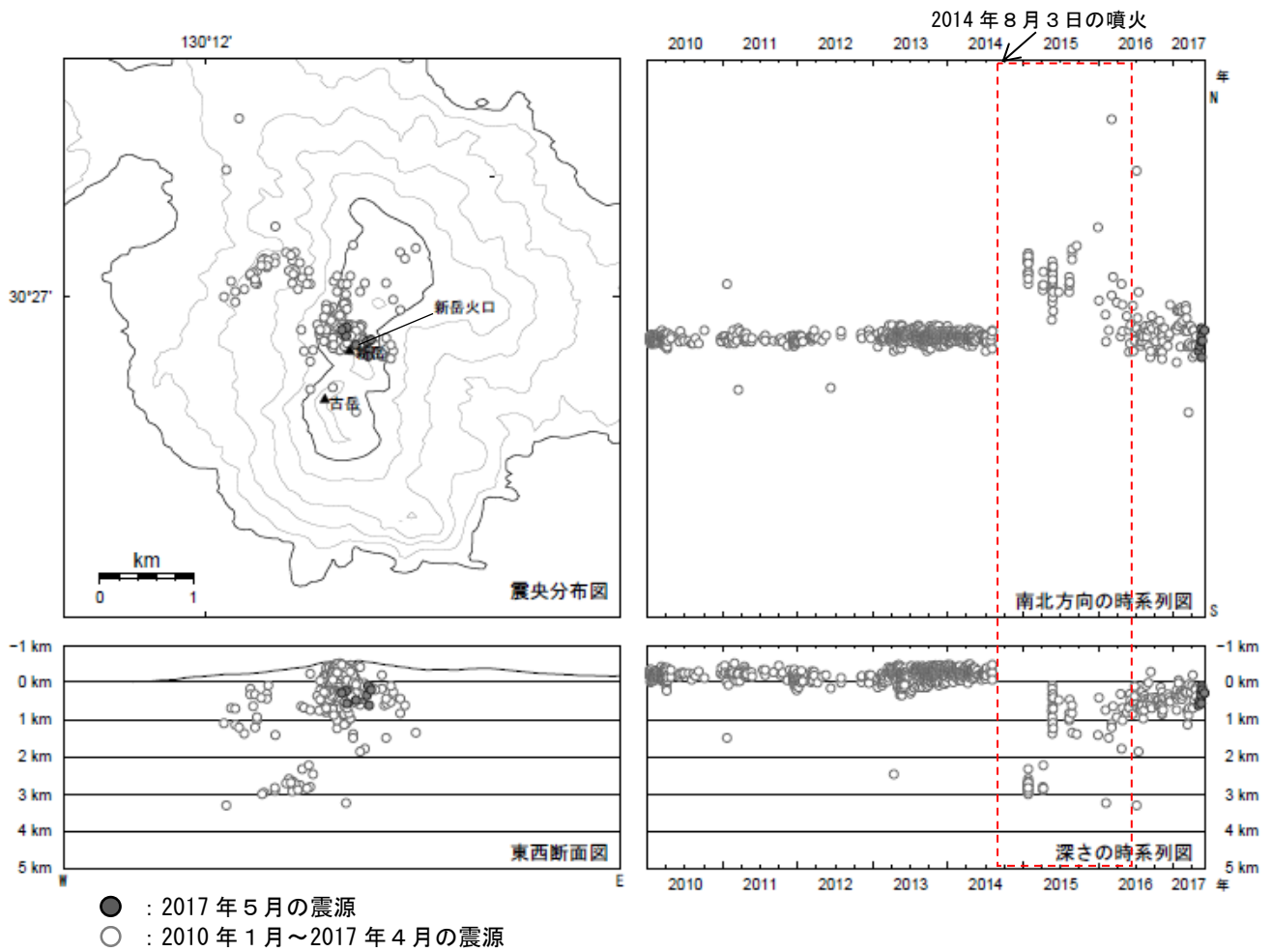
図 6 口永良部島 震源分布図（2010 年 1 月～2017 年 5 月）
