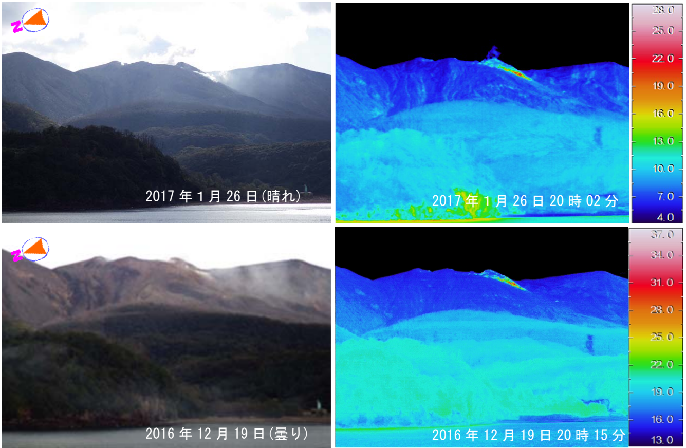
図2 口永良部島 本村から撮影した可視画像と地表面温度分布 前回（2016年12月19日）と比較して、噴気及び熱異常域に特段の変化はみられていません。
