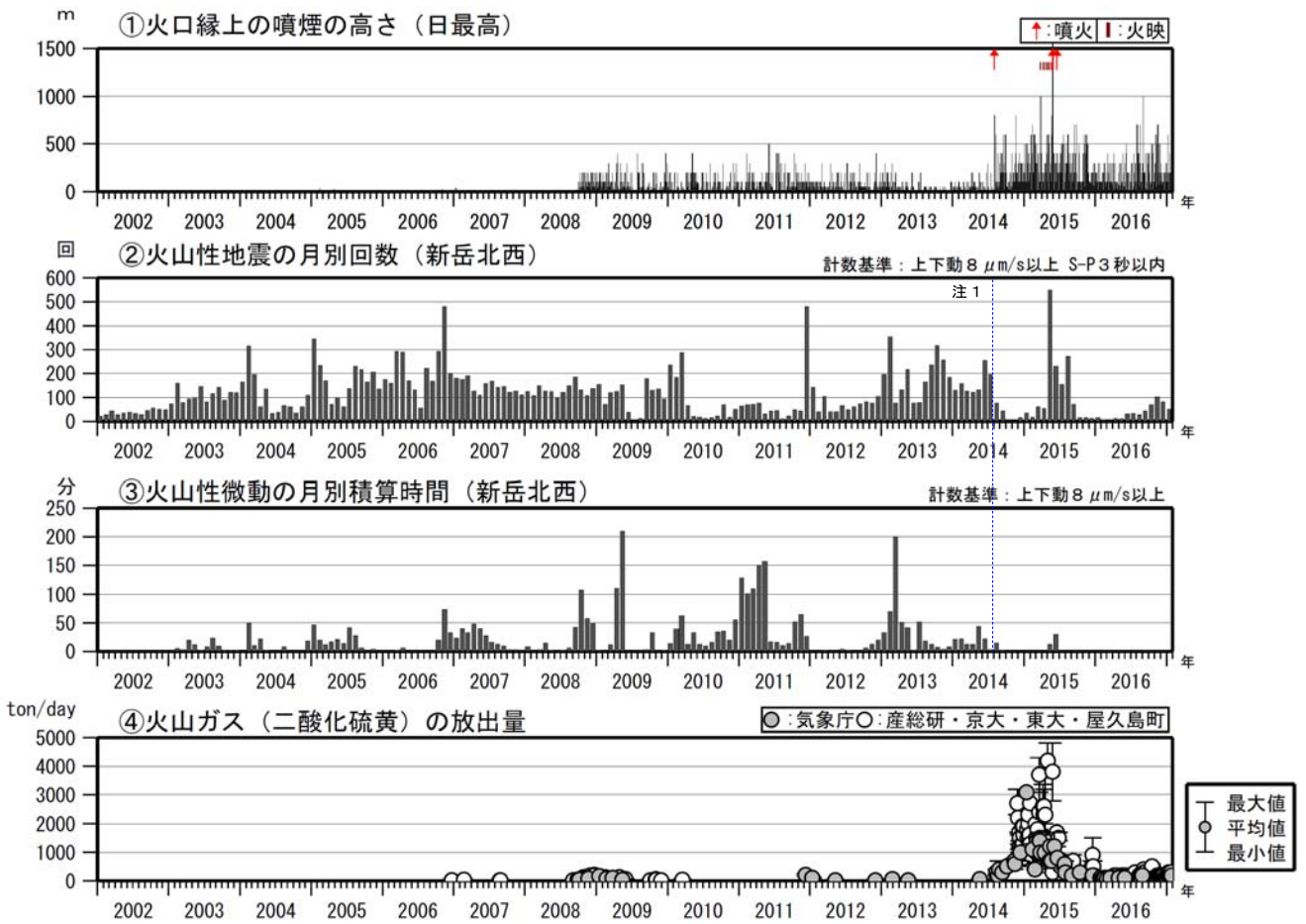
図 4 口永良部島 火山活動経過図（2002 年 1 月～2017 年 1 月）
