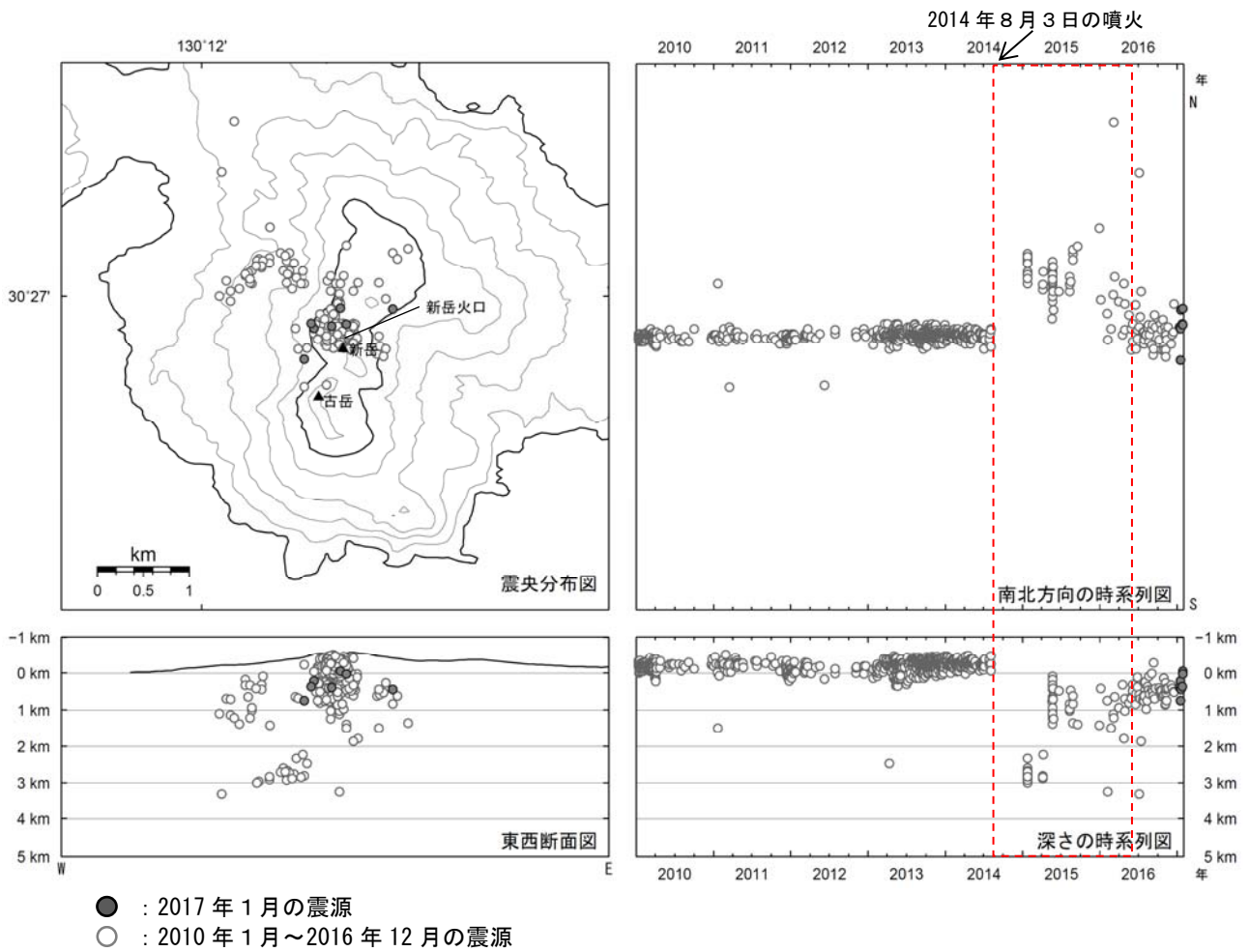
図 6 口永良部島 震源分布図（2010 年 1 月～2017 年 1 月）
