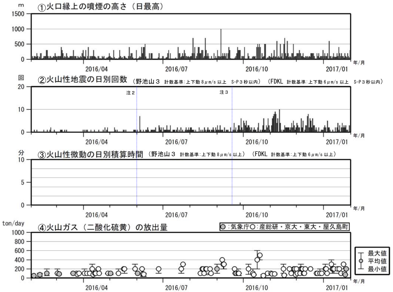
図5 口永良部島 最近の火山活動経過図（2016年2月～2017年1月）
