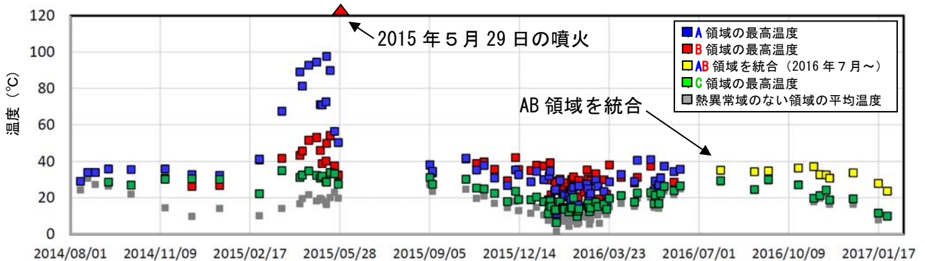
図3 口永良部島 新岳西斜面の地表面温度分布と熱異常域の温度時系列 （2014年8月～2017年1月：本村から新岳の北西側を撮影）
