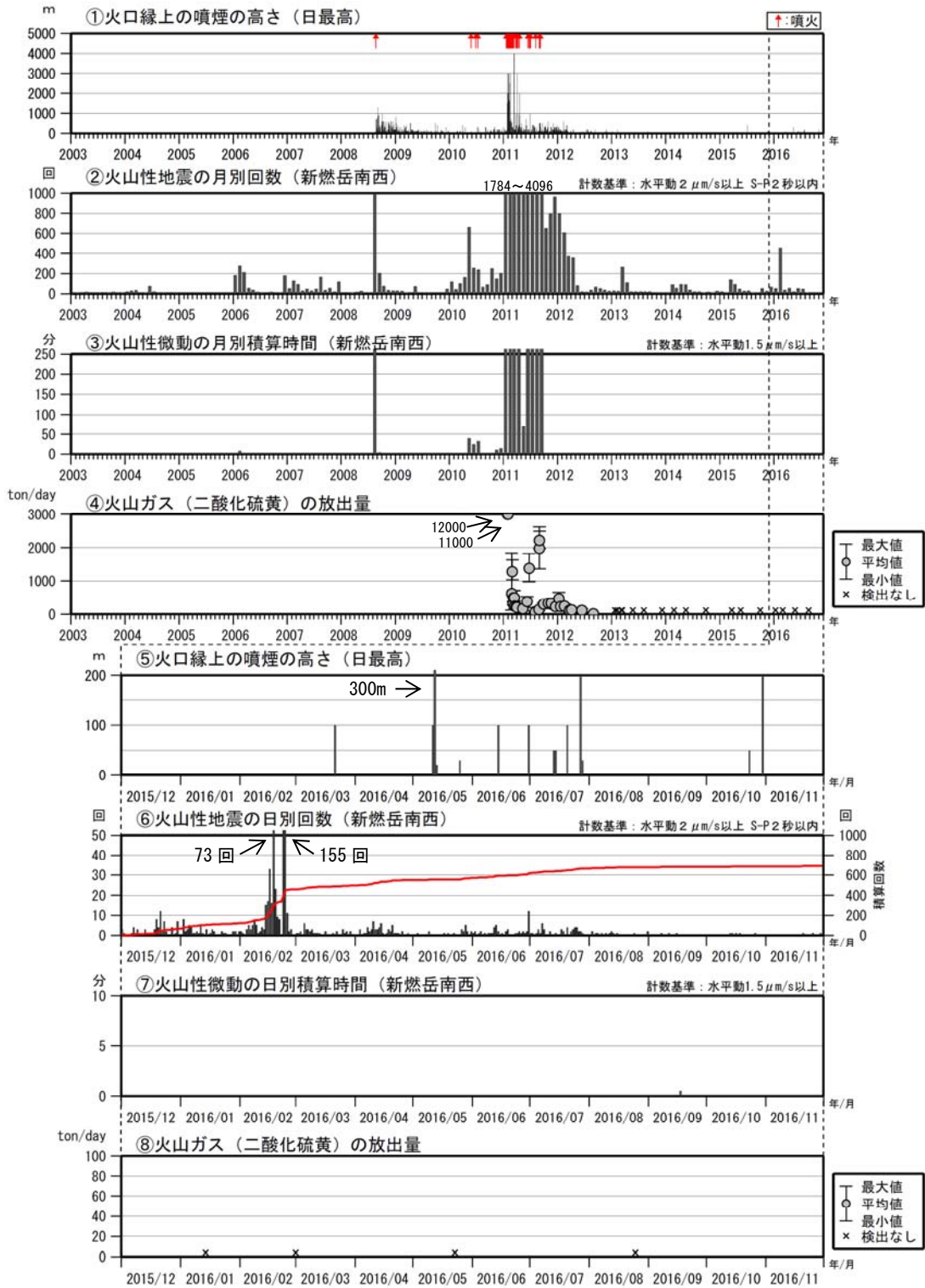
図2 霧島山（新燃岳） 火山活動経過図（2003年1月～2016年11月）
