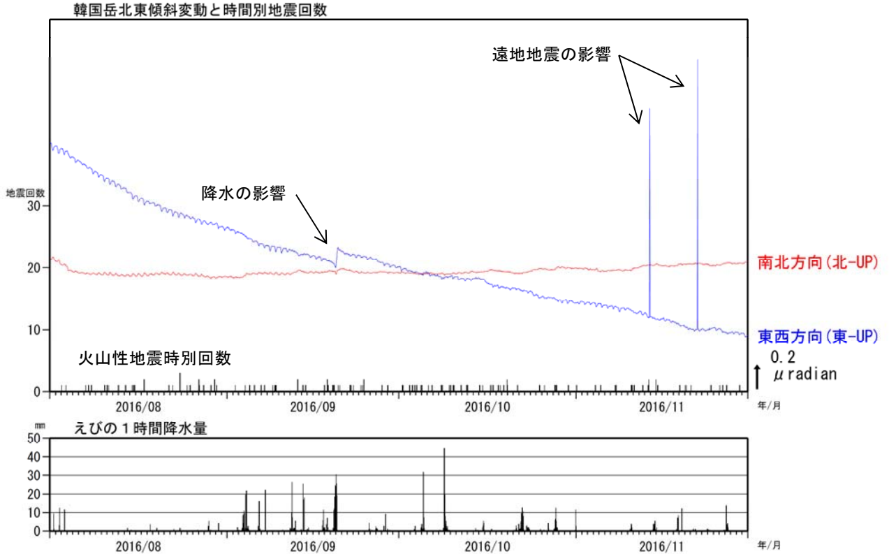
図 25 霧島山（えびの高原（硫黄山）周辺） 韓国岳北東傾斜計の傾斜変動と火山性地震の時間別回数（2016 年 8 月～2016 年 11 月）
