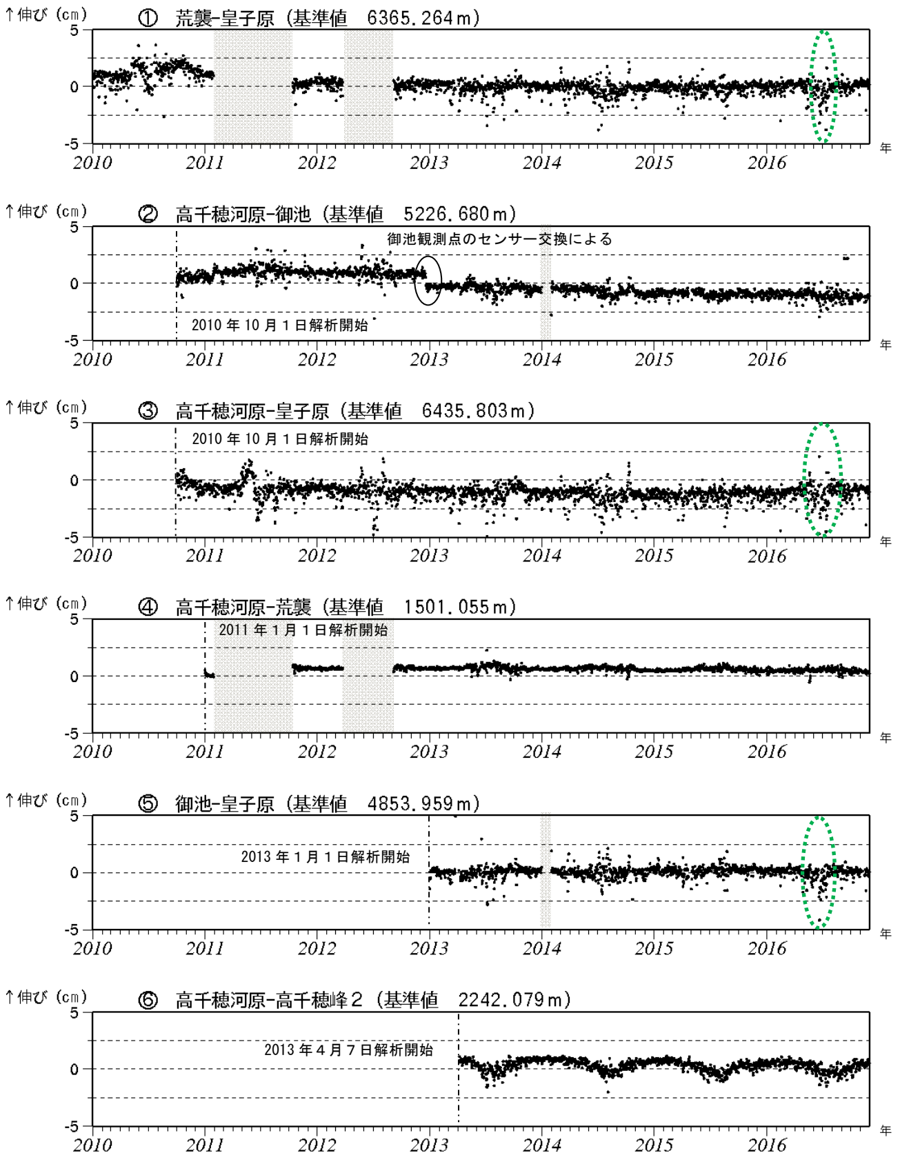
図 15 霧島山 (御鉢) GNSS 連続観測による基線長変化 (2010 年 1 月～2016 年 11 月)
