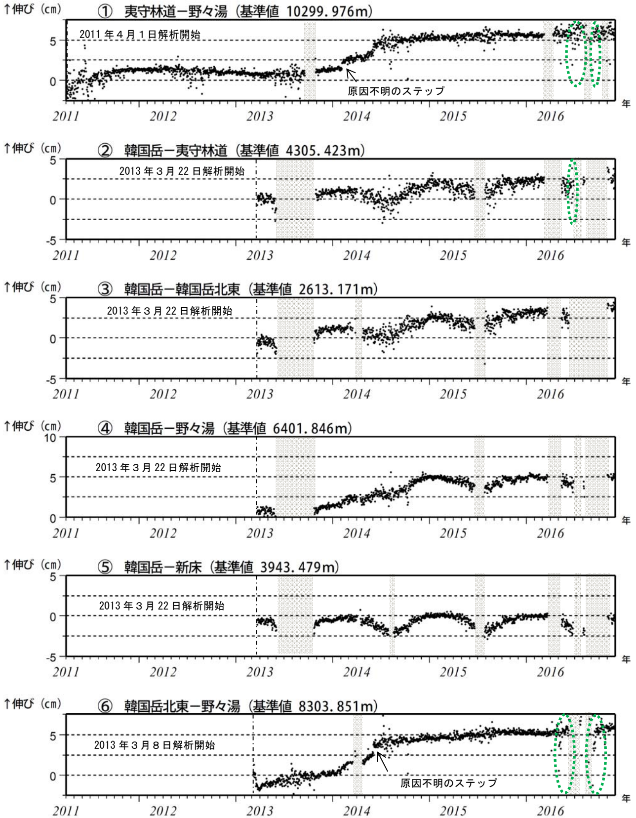
図 26-1 霧島山（えびの高原（硫黄山）周辺） GNSS 連続観測による基線長変化 （2011年4月～2016年11月）
