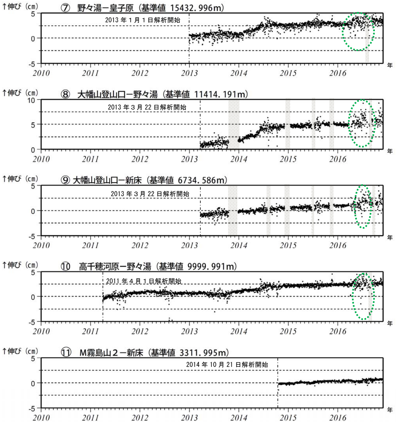
図5-2 霧島山（新燃岳） GNSS 連続観測による基線長変化（2010年1月～2016年11月）
