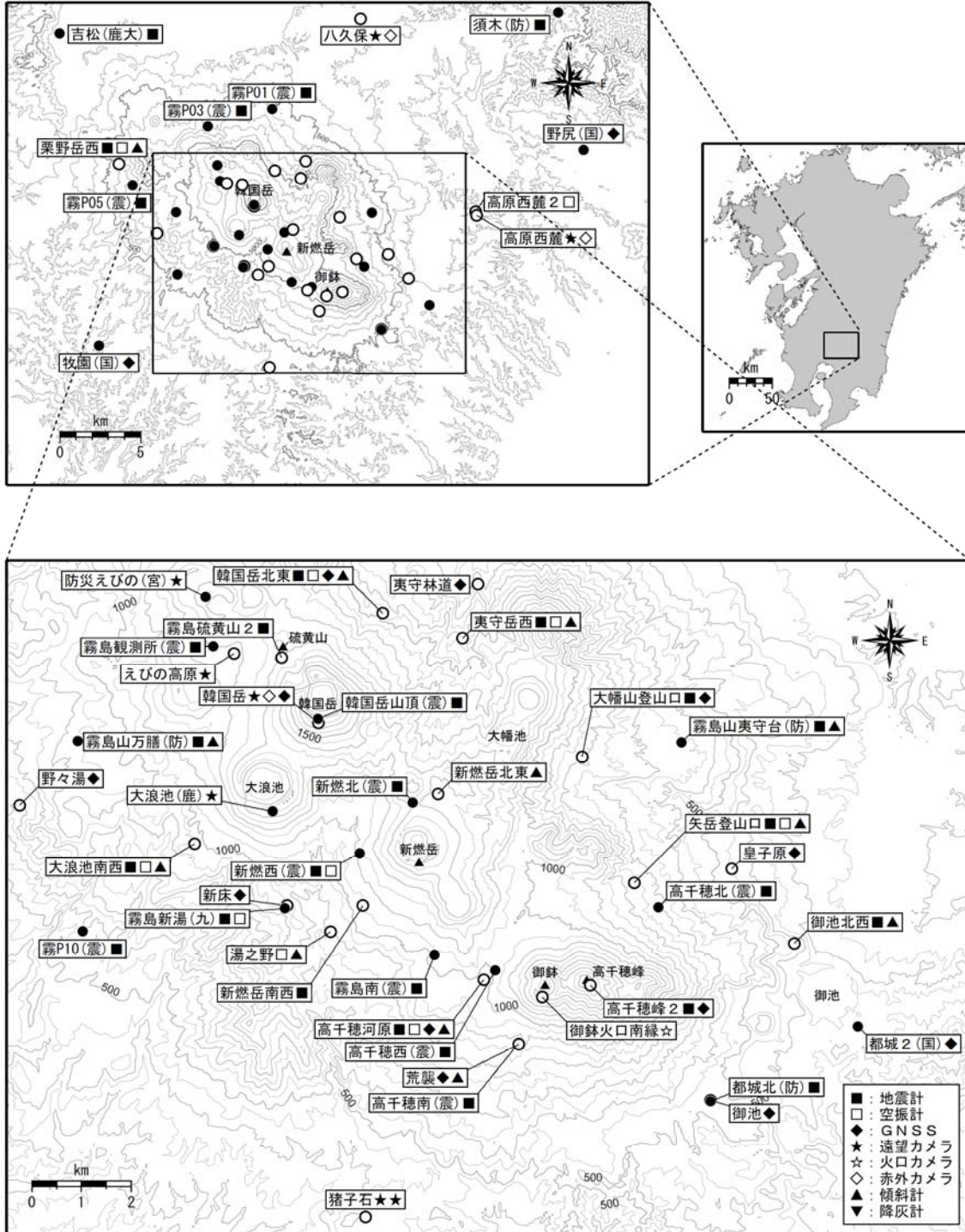
図 12 霧島山 観測点配置図
