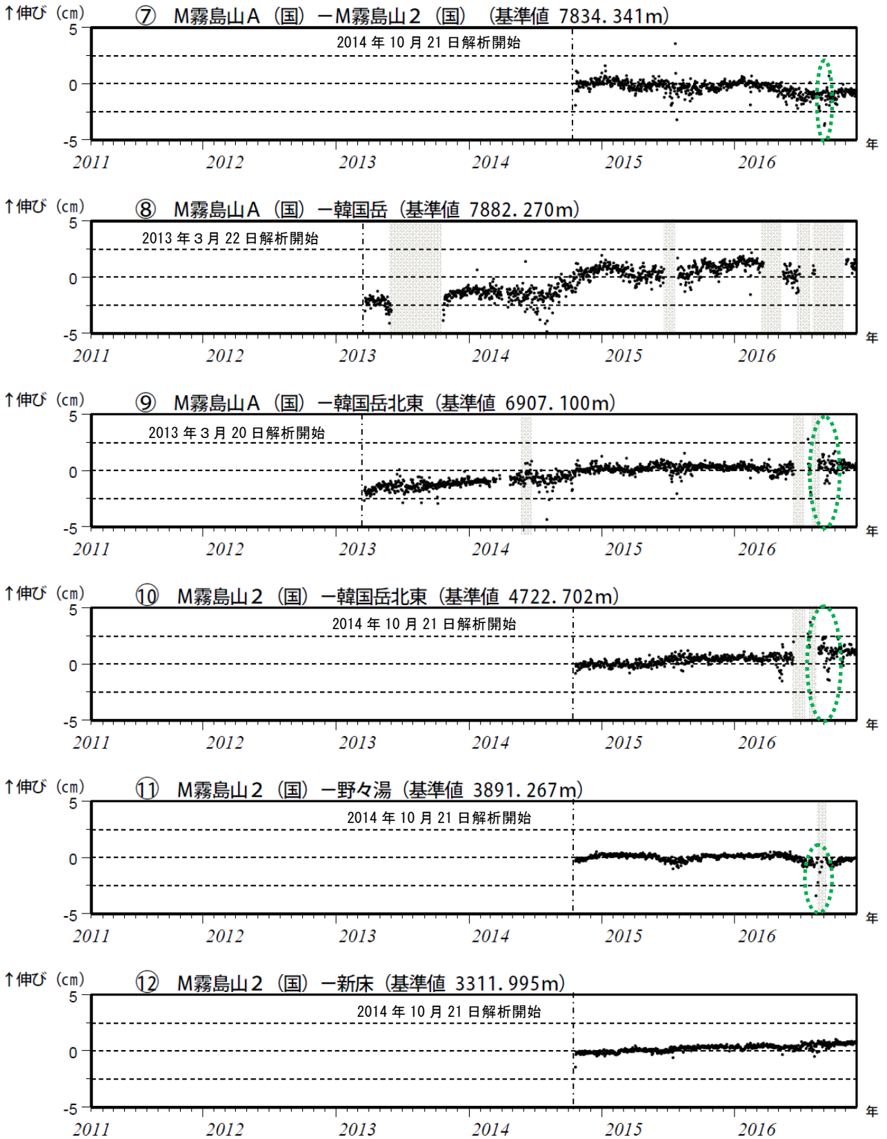
図 26-2 霧島山（えびの高原（硫黄山）周辺） GNSS 連続観測による基線長変化 (2011 年 4 月～2016 年 11 月)
