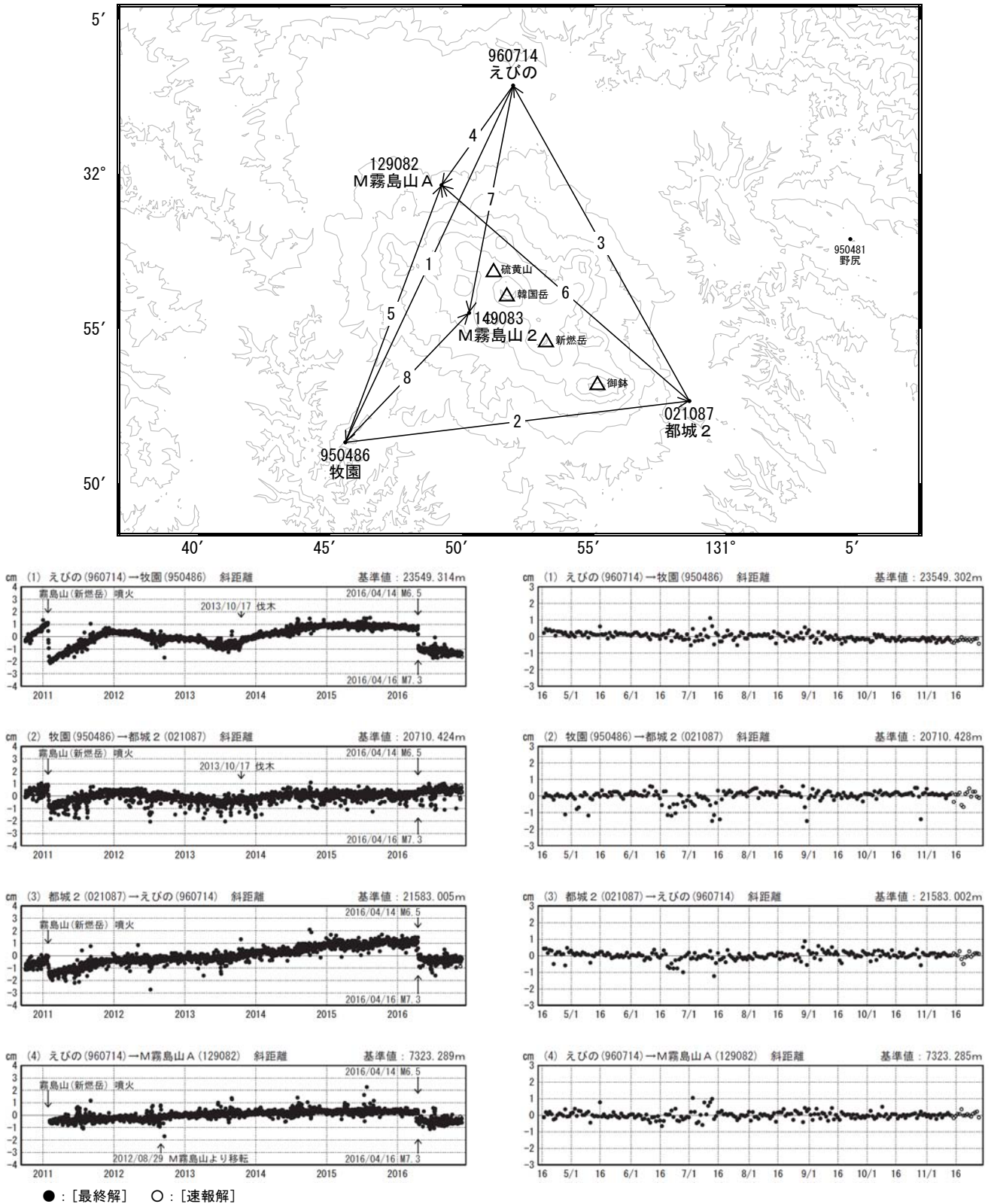
図 4 霧島山 国土地理院による広域的な地殻変動観測結果* (2010 年 10 月 1 日～2016 年 11 月 27 日)
