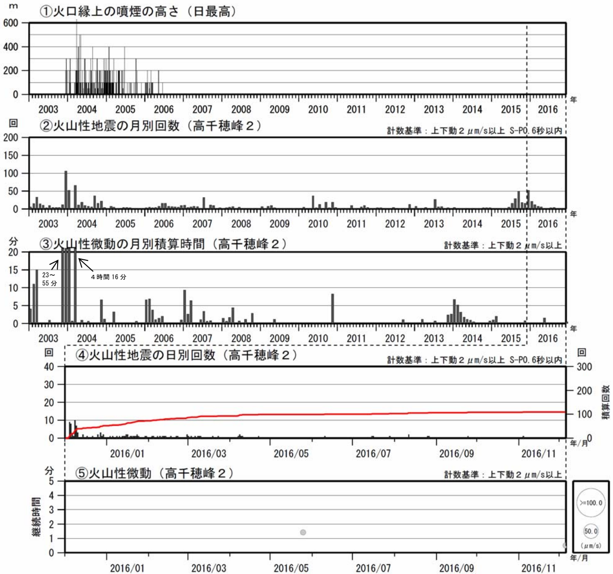
図 14 霧島山（御鉢） 火山活動経過図（2003 年 1 月～2016 年 12 月 5 日）
