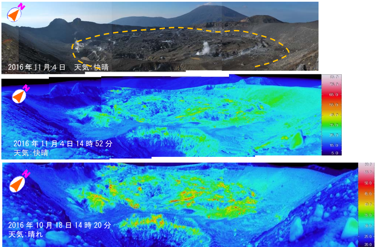
図 11 新燃岳火口内の可視画像及び地表面温度分布（新燃岳火口縁南東側から撮影）
