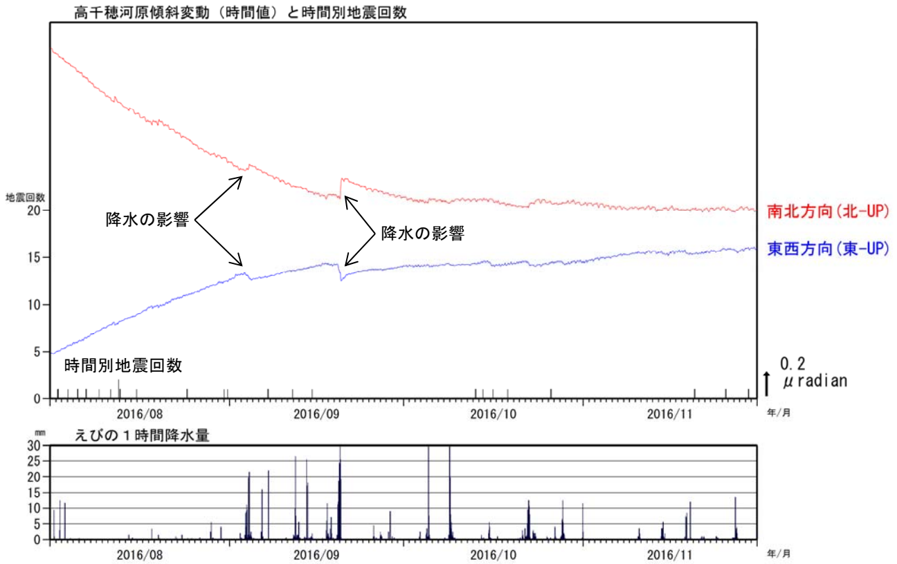
図3 霧島山（新燃岳） 高千穂河原傾斜計の傾斜変動と火山性地震の時間別回数 （2016年8月～2016年11月）
