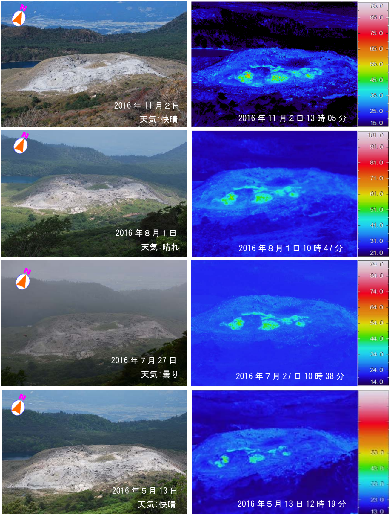
図 29 霧島山（えびの高原(硫黄山)周辺) 可視画像及び地表面温度分布（韓国岳 4 合目から） ・ 硫黄山火口内及び火口周辺で引き続き噴気を確認しました。 ・ 赤外熱映像装置による観測では引き続き、熱異常域を確認しました。
