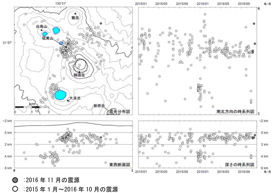
図 24 霧島山（えびの高原（硫黄山）周辺） 震源分布図（2015 年 1 月～2016 年 11 月）
