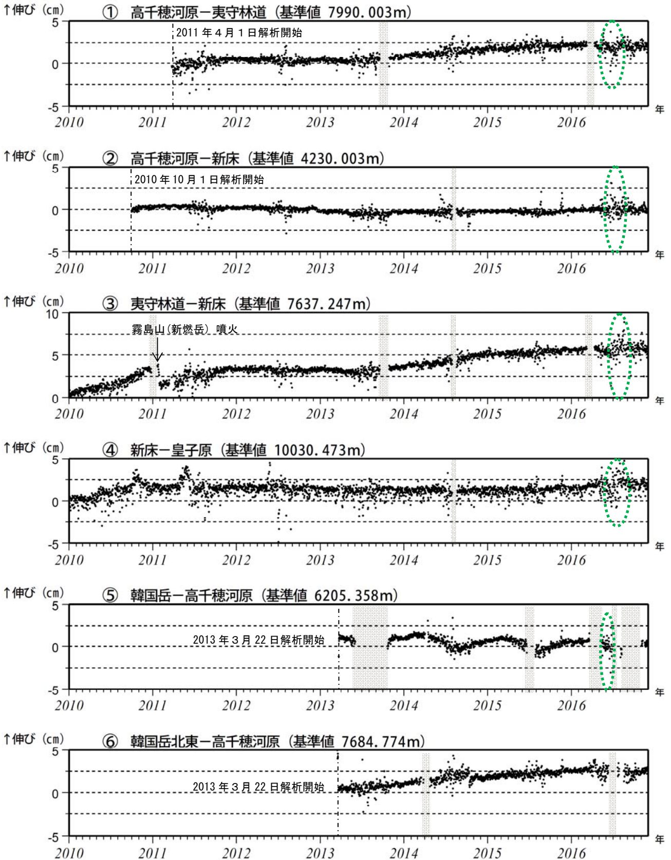
図5-1 霧島山(新燃岳) GNSS連続観測による基線長変化(2010年1月~2016年11月)
