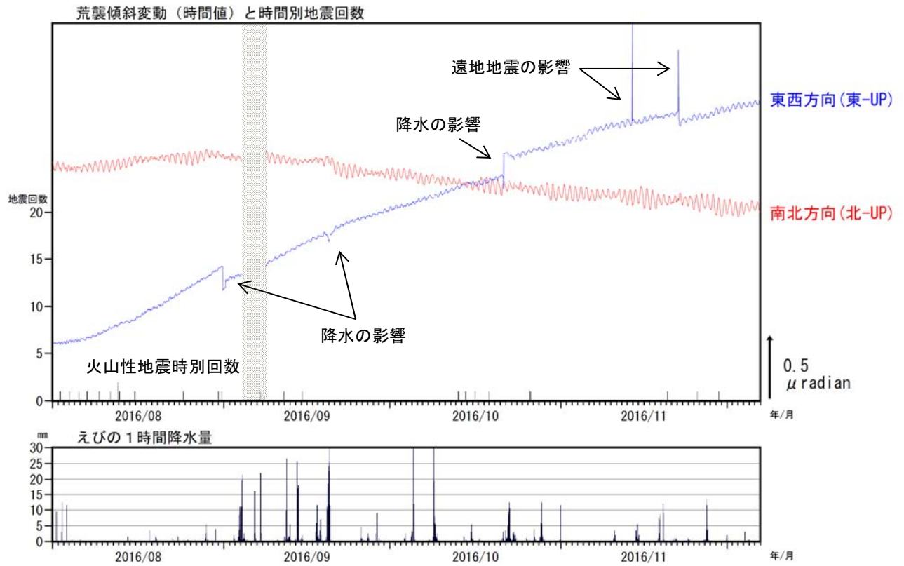
図 19 霧島山（御鉢） 荒襲傾斜計の傾斜変動と火山性地震の時間別回数 （2016 年 8 月 1 日～2016 年 12 月 6 日）
