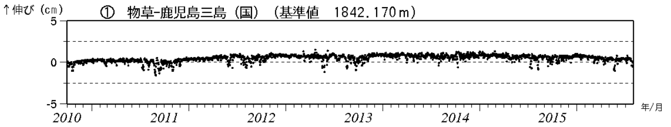
図5 薩摩硫黄島 GNSS連続観測による基線長変化（2010年10月～2016年7月）
