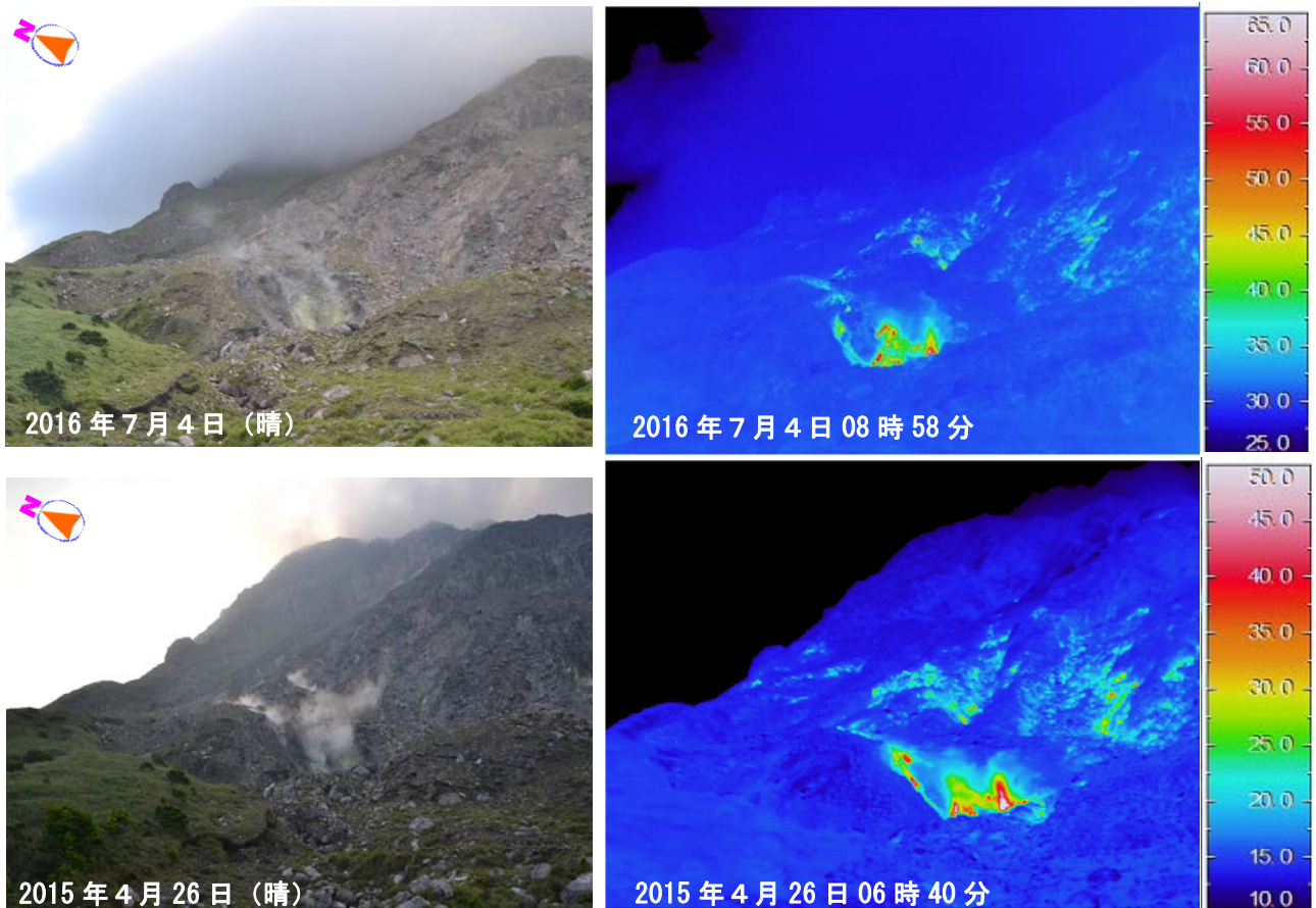
図 2-2 薩摩硫黄島 可視画像及び赤外熱映像装置による温度分布の変化（砂防ダム上流左岸から撮影） （上段：2016 年 7 月 4 日、下段：2015 年 4 月 26 日）
