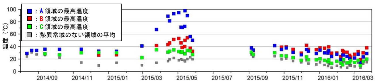
図2 口永良部島 新岳西斜面の地表面温度分布と熱異常域の温度時系列 （本村から新岳の北西側を撮影、2014年8月～2016年3月）
