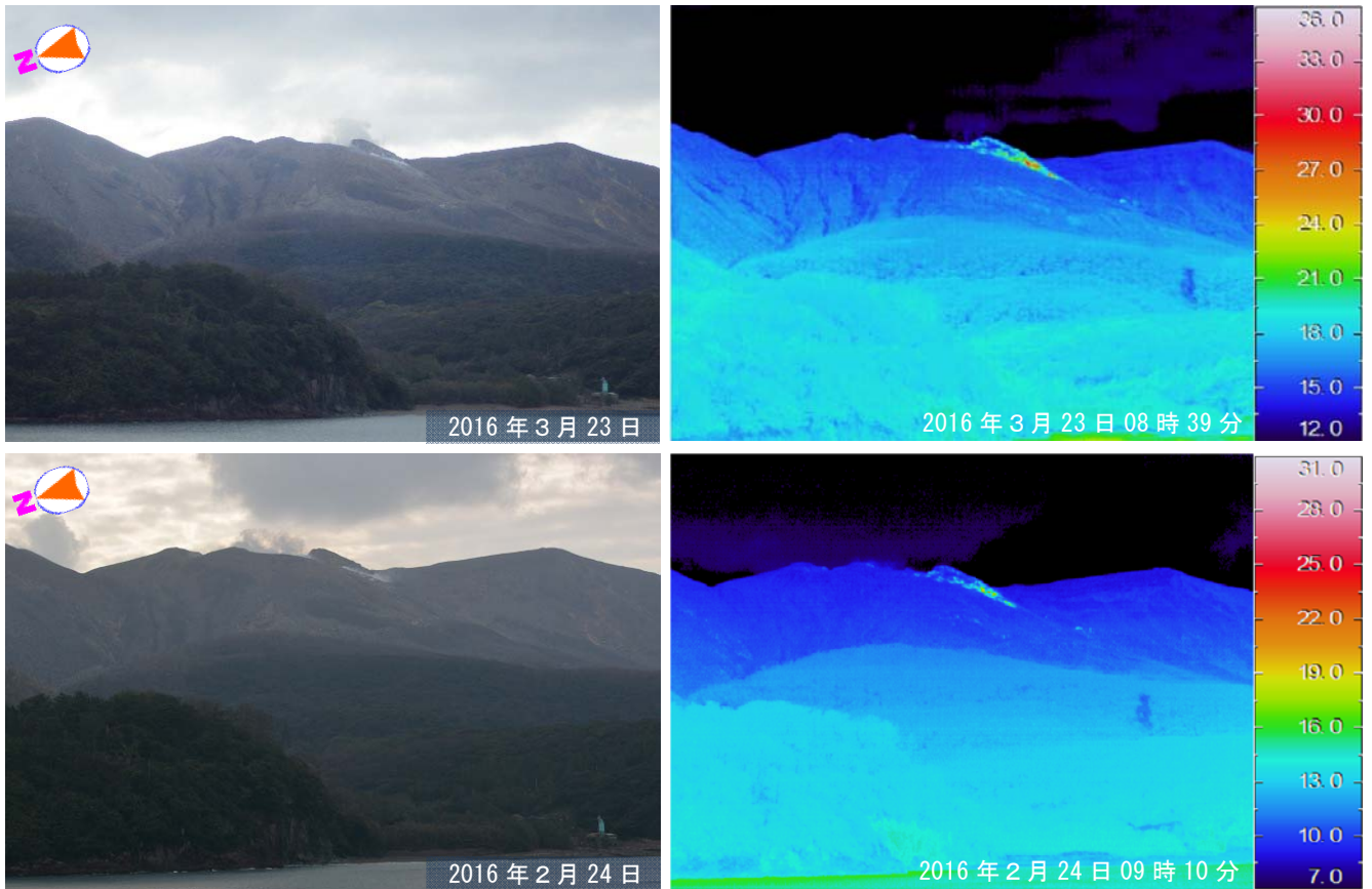
本村から撮影した可視画像と地表面温度分布（上図：2016年3月23日、下図：2016年2月24日）
