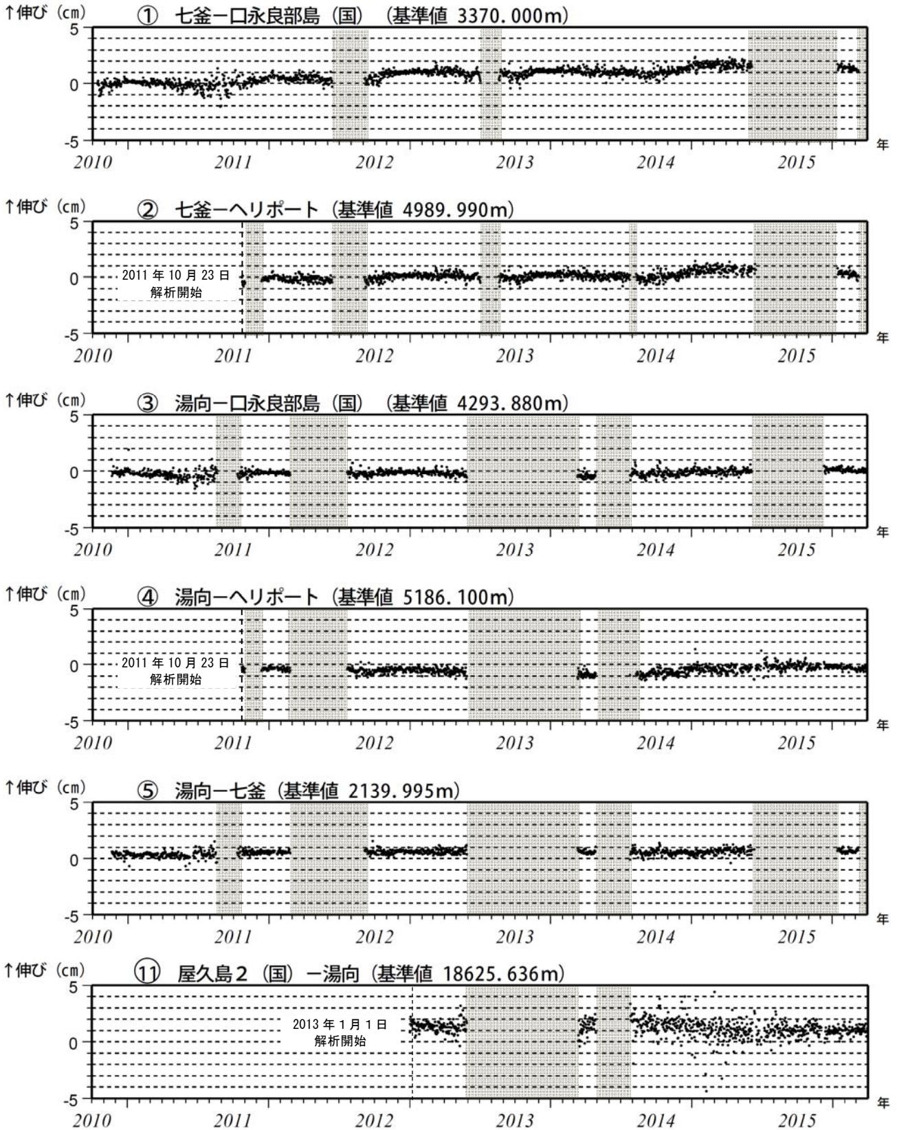
図5 口永良部島 GNSS 連続観測による基線長変化 (2010年10月~2016年3月)
