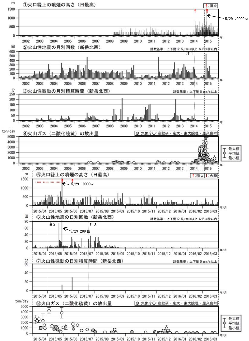
図3 口永良部島 火山活動経過図（2002年1月～2016年3月）
