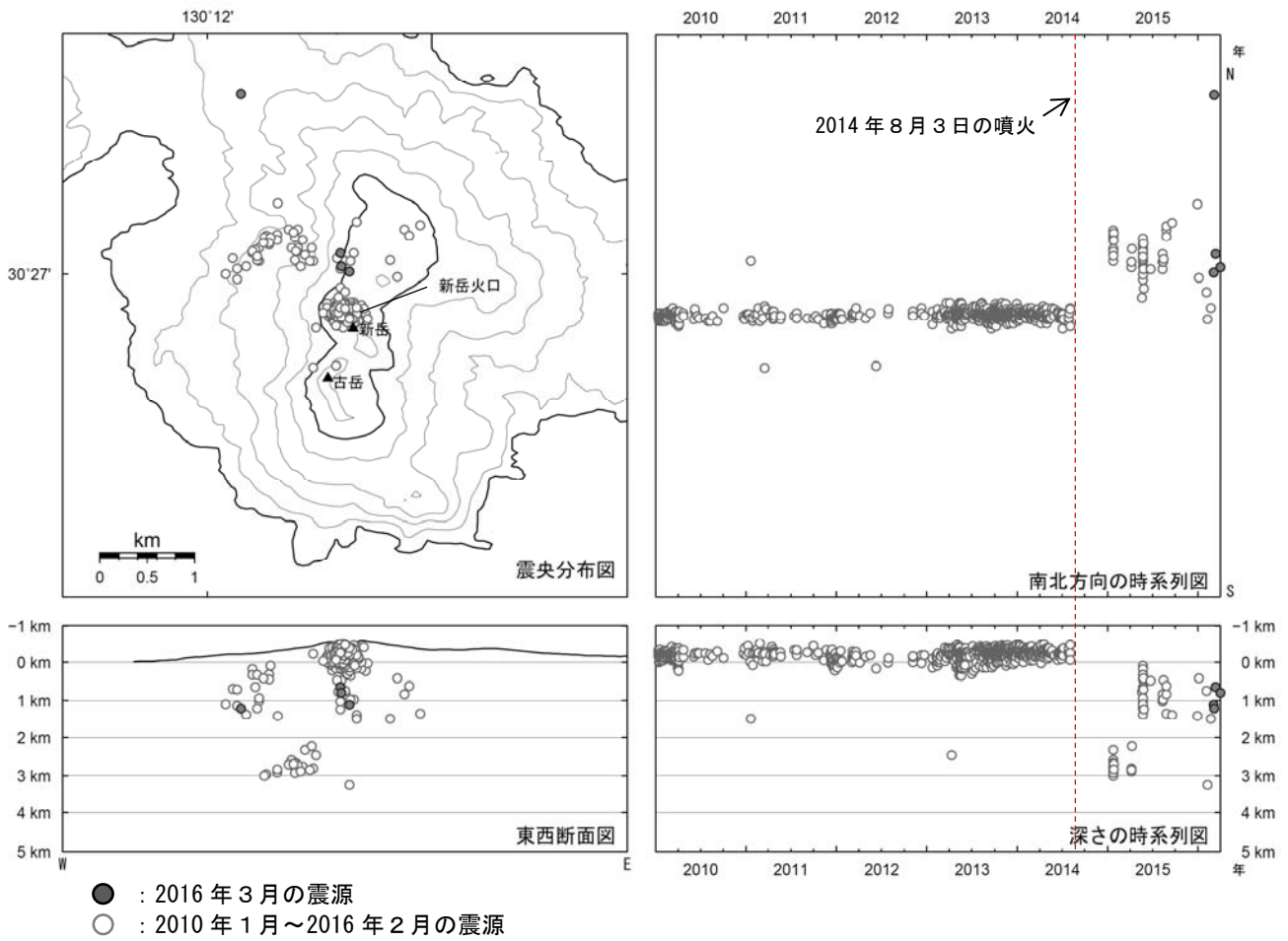
図 4 口永良部島 震源分布図（2010 年 1 月～2016 年 3 月）
