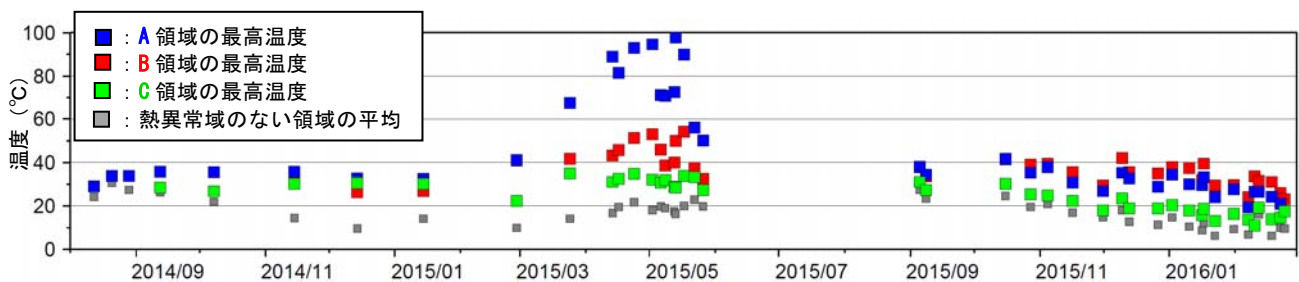
図2 口永良部島 新岳西斜面の地表面温度分布と熱異常域の温度時系列 （本村から新岳の北西側を撮影、2014年8月～2016年2月）
