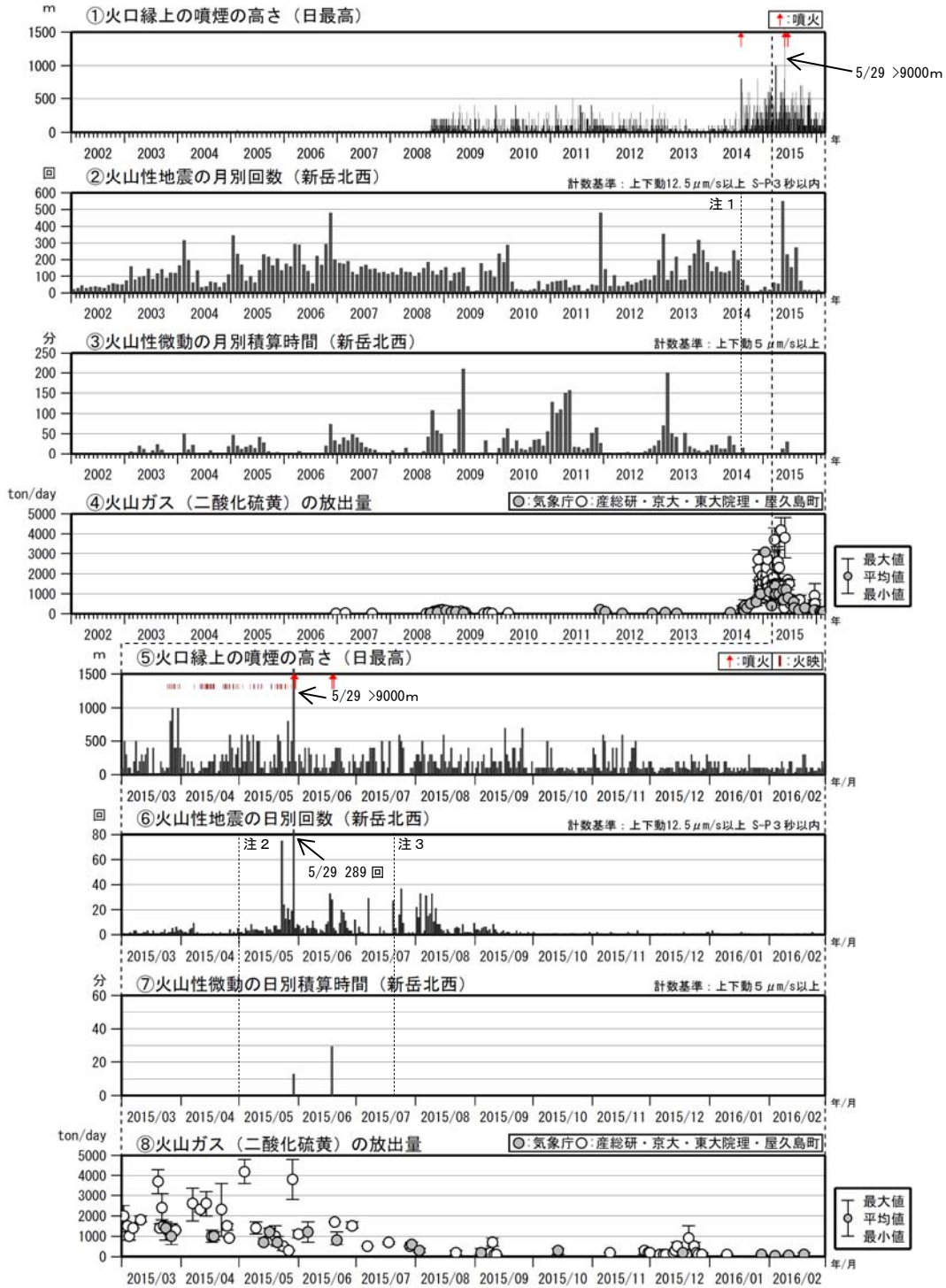
図3 口永良部島 火山活動経過図（2002年1月～2016年2月）
