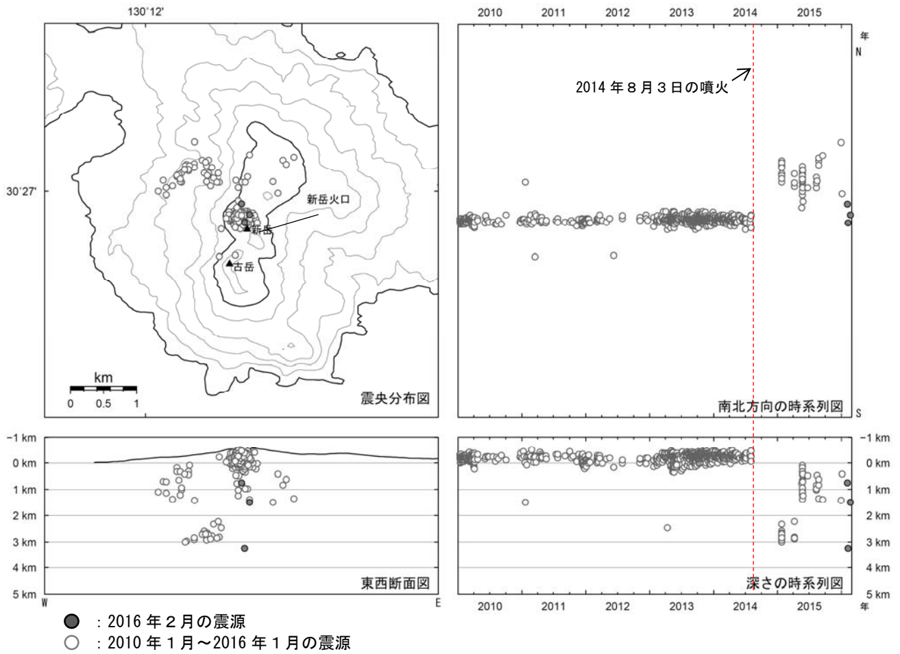
図 4 口永良部島 震源分布図（2010 年 1 月～2016 年 2 月）
