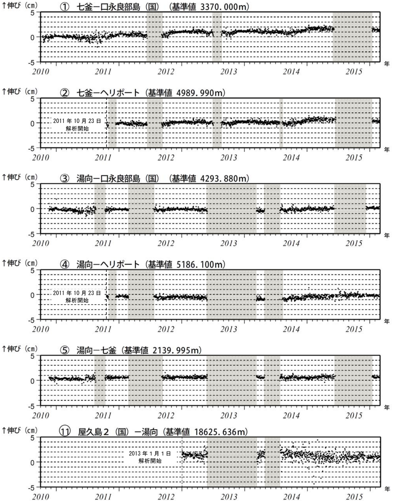
図5 口永良部島 GNSS 連続観測による基線長変化（2013 年 1 月～2016 年 2 月）
