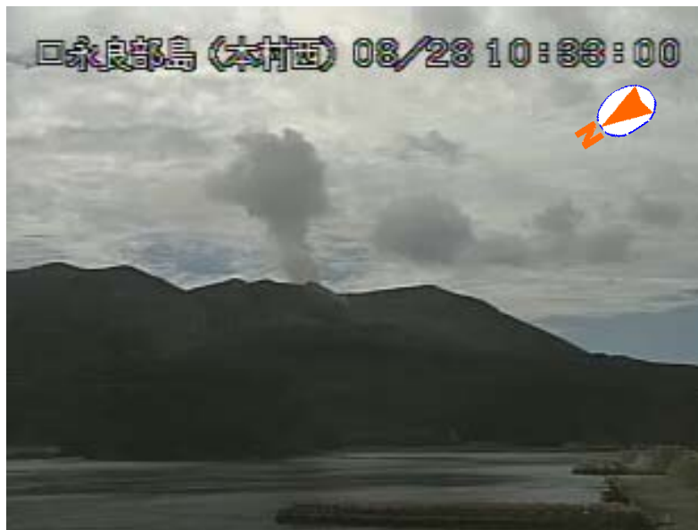
図 1 口永良部島 噴煙の状況（8 月 28 日、本村西遠望カメラによる）
