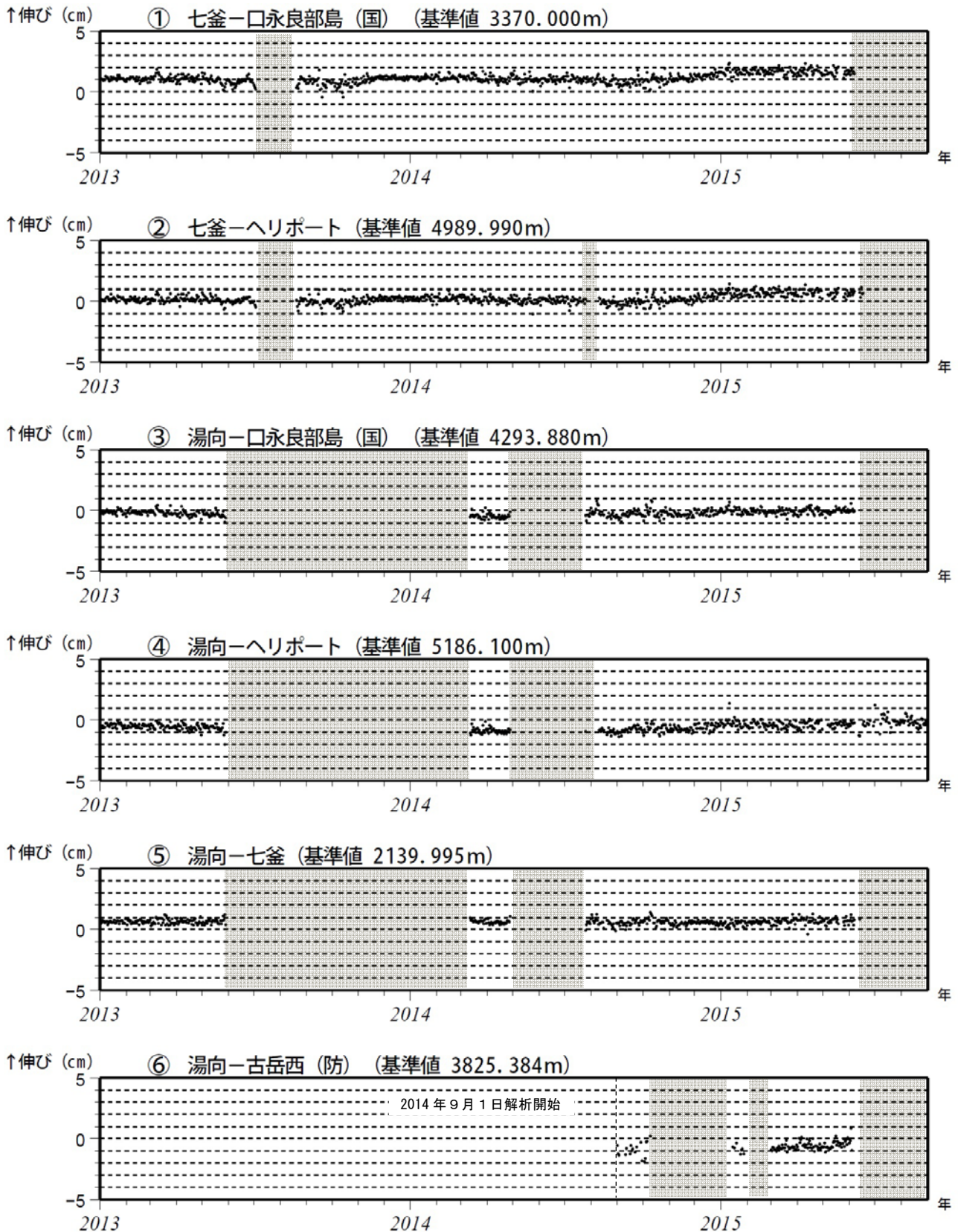
図3 口永良部島 GNSS 連続観測による基線長変化 (2013 年 1 月～2015 年 8 月)
