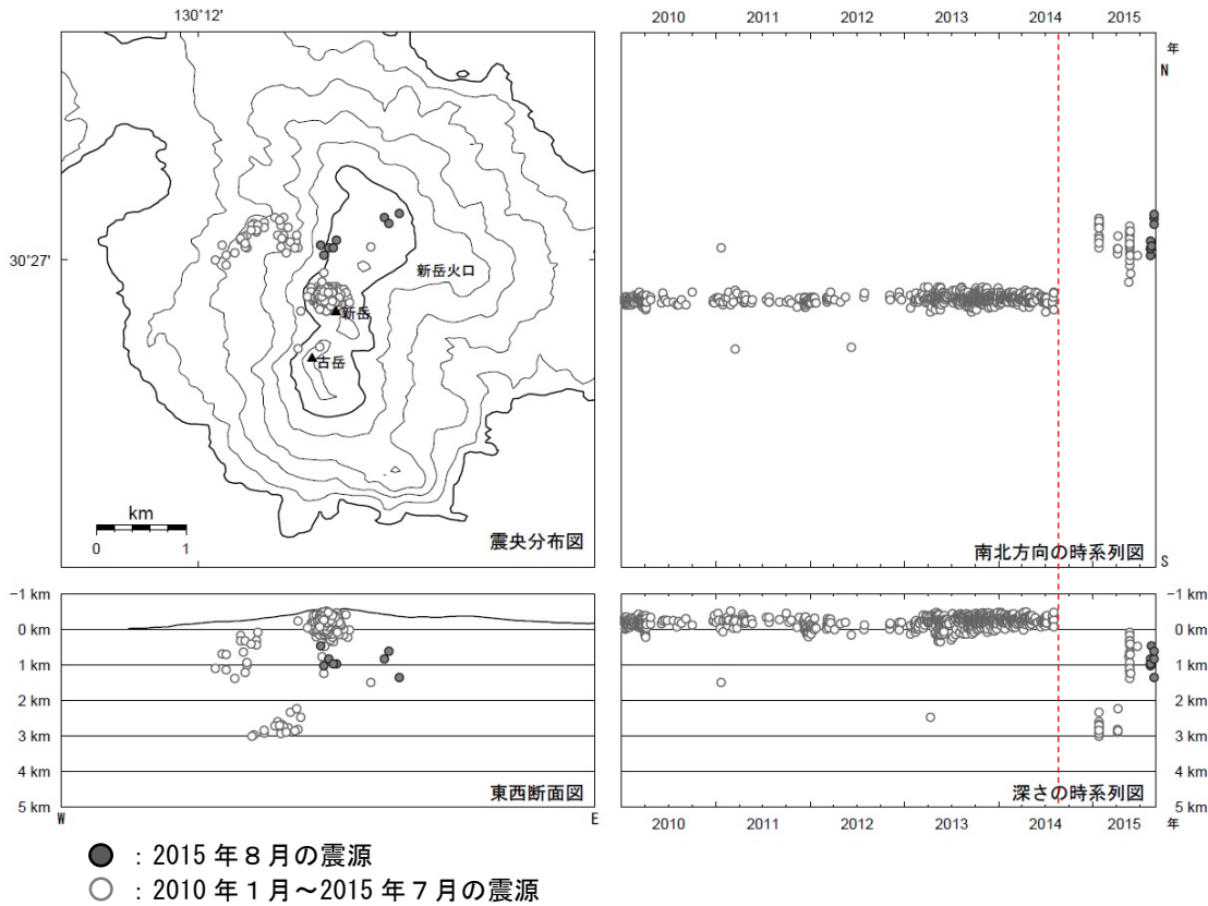
図5 口永良部島 震源分布図 (2010年1月~2015年8月)
