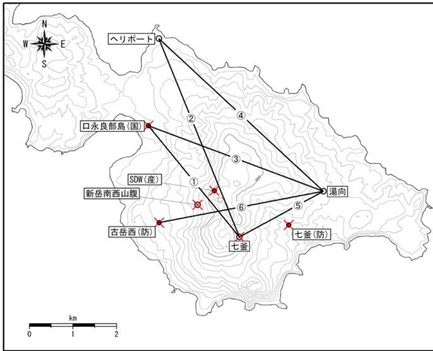
図4 口永良部島 GNSS 連続観測点と基線番号
