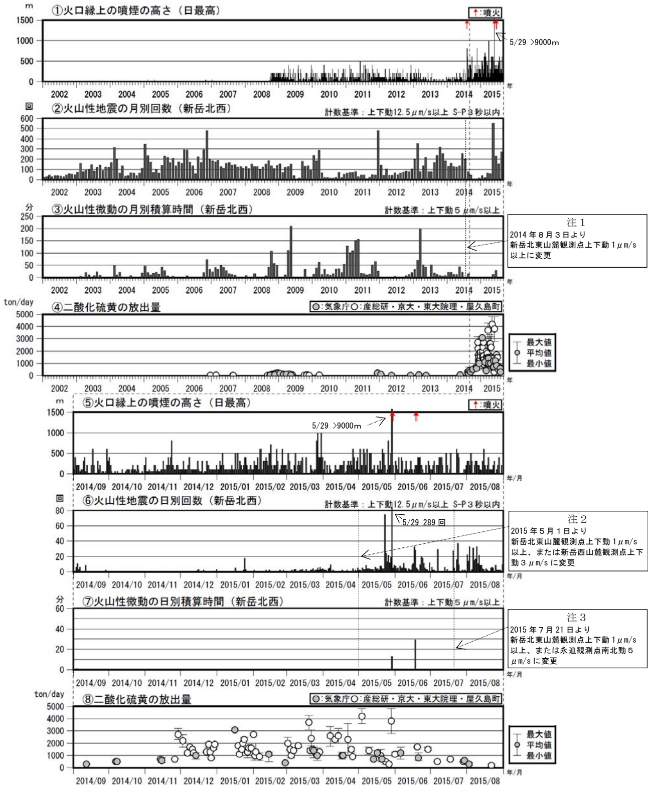
図2 口永良部島 火山活動経過図 (2002年1月～2015年8月)
