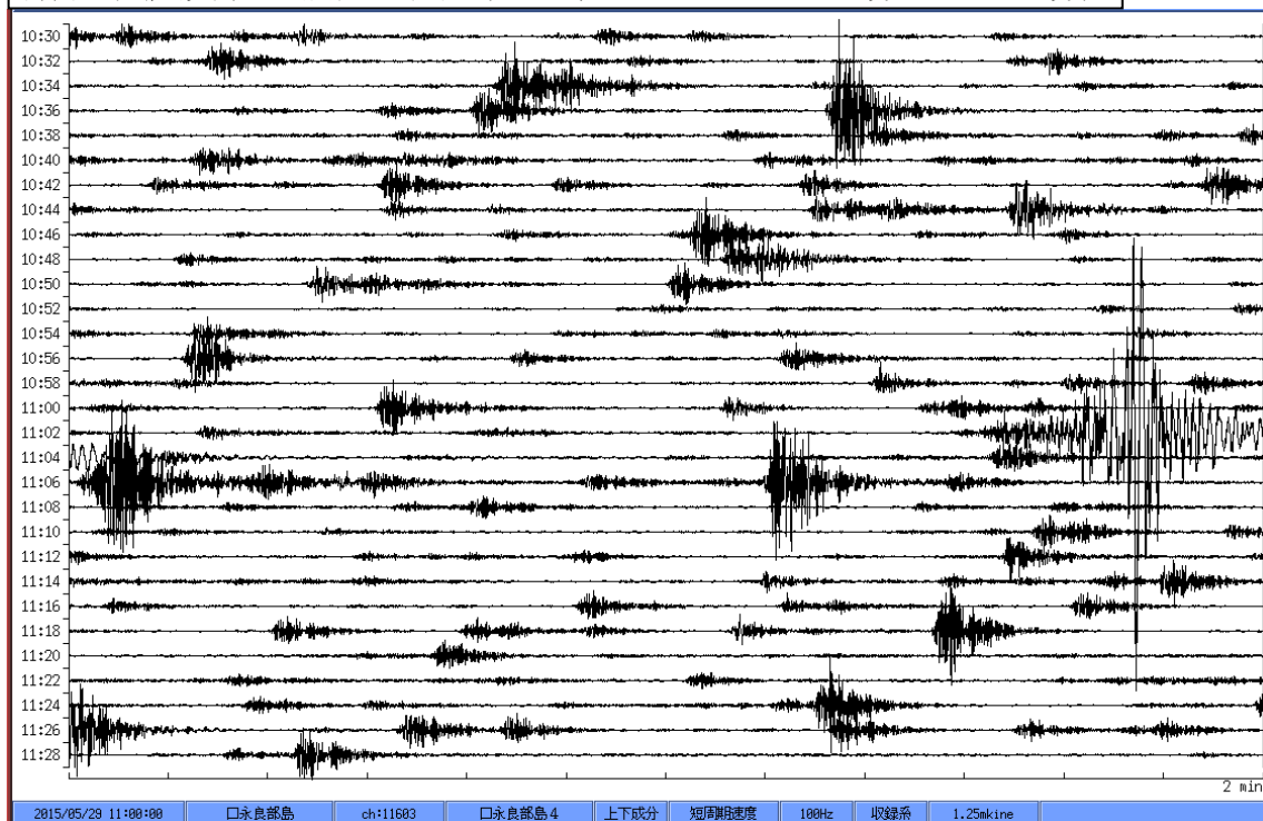
図 9 口永良部島 噴火時の地震波形 (5 月 29 日 09 時 30 分～11 時 30 分) 新岳西山麓観測点 (地震計: 上下動)
