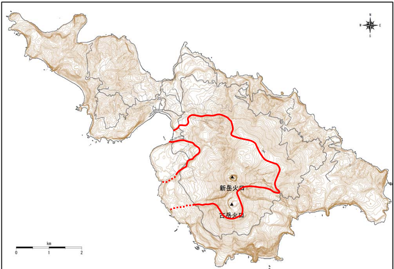
図7 口永良部島 火砕流の流下範囲
