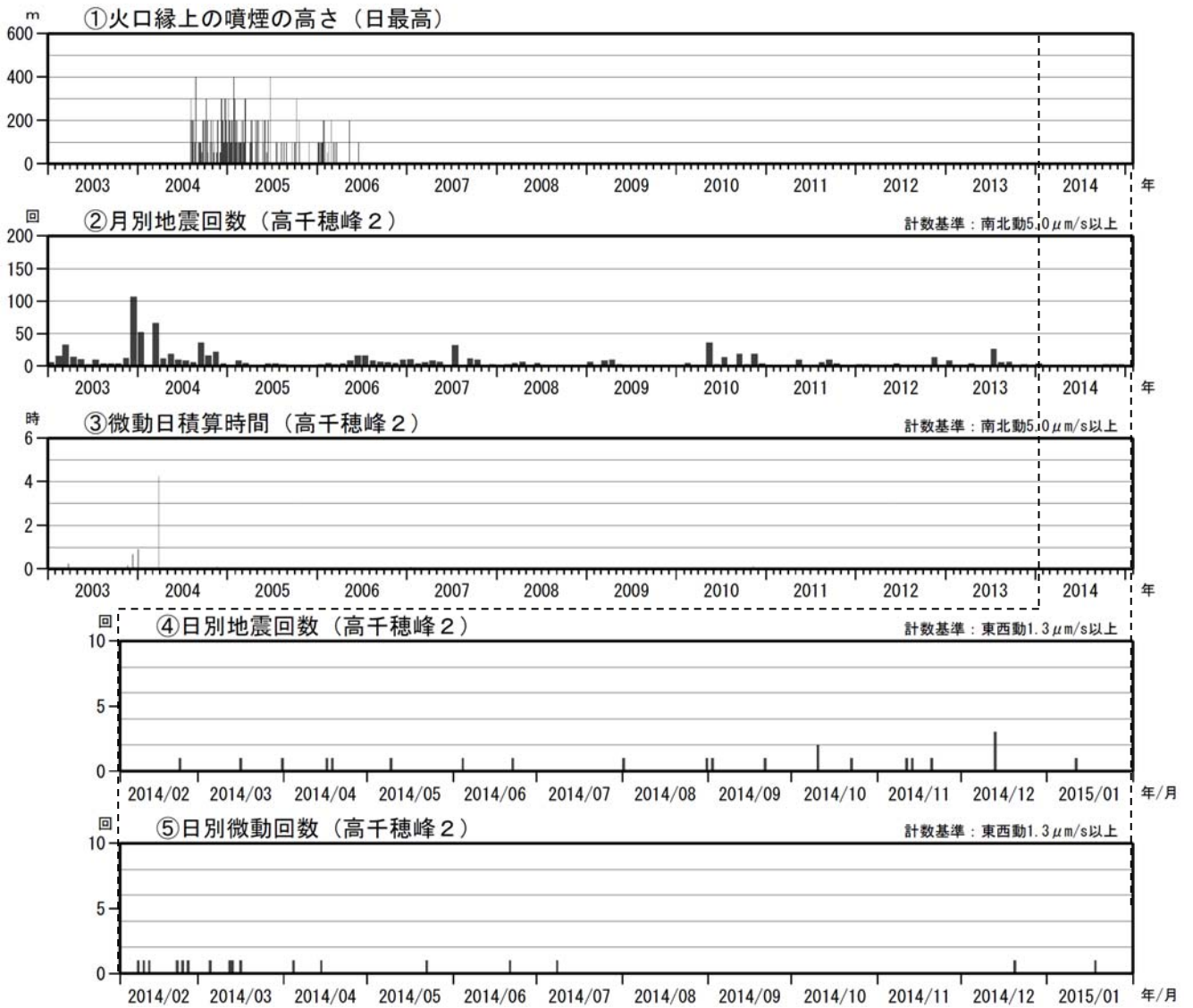
図 10 霧島山（御鉢） 火山活動経過図（2003 年 1 月～2015 年 1 月）
