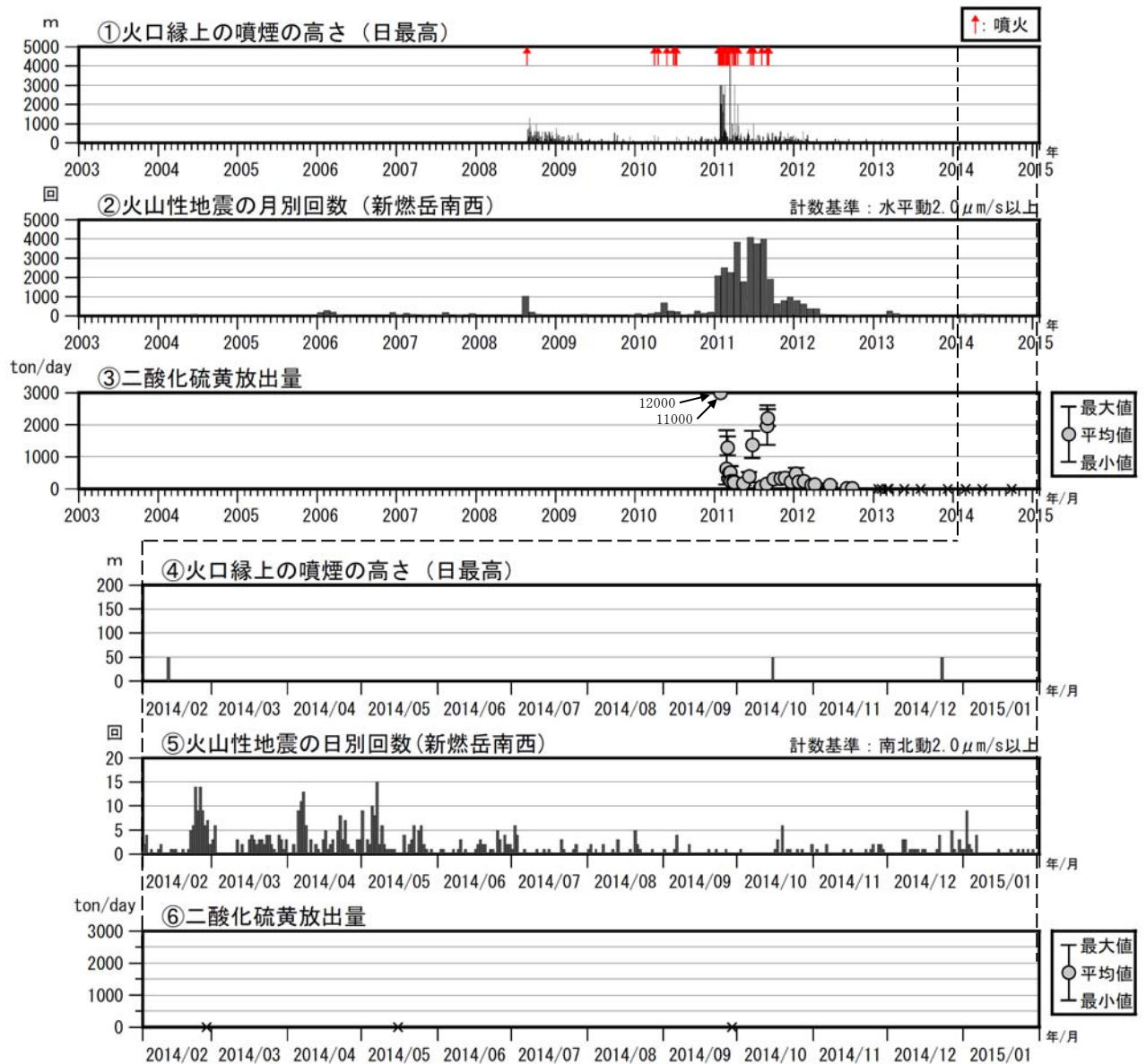
図3 霧島山（新燃岳） 火山活動経過図（2003年1月～2015年1月）
