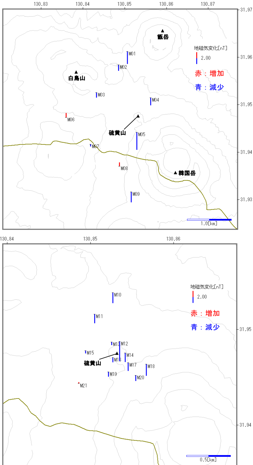
図 16 霧島山（えびの高原（硫黄山）周辺） 繰返し観測による全磁力の変化 （上段：えびの高原周辺 2014 年 10 月 25 日～2015 年 1 月 21 日、下段：硫黄山周辺 2014 年 12 月 9 日～2015 年 1 月 21 日）
