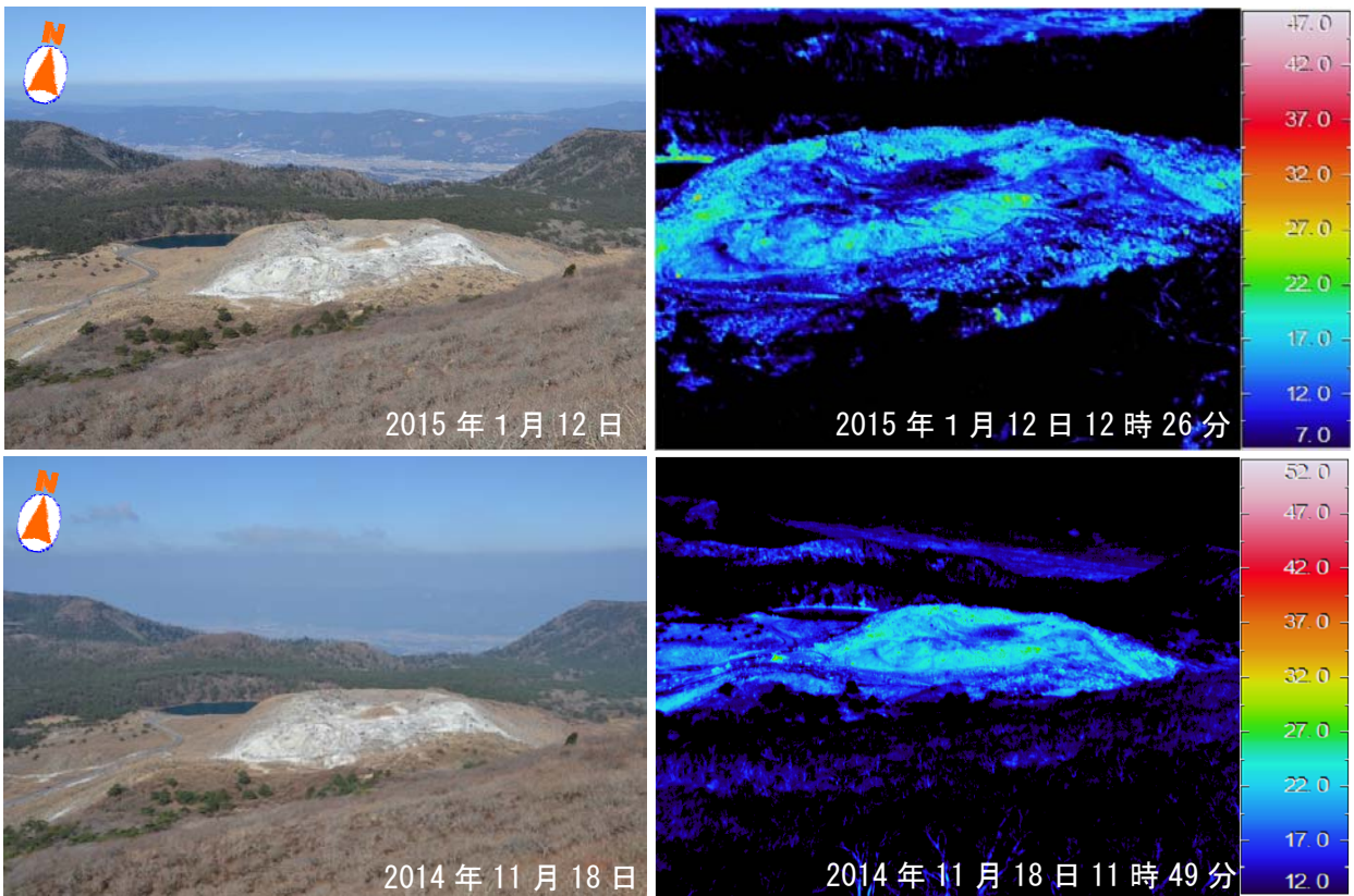
図 14 霧島山（えびの高原（硫黄山）周辺） 可視画像および赤外熱映像装置による地表面温度分布（韓国岳中腹から硫黄山の南側及び火口内を撮影）
