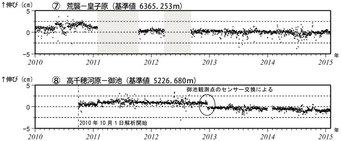
図 6-2 霧島山 GNSS 連続観測による基線長変化（2010 年 1 月～2015 年 1 月）
