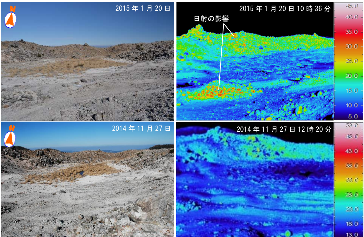
図 15 霧島山（えびの高原（硫黄山）周辺） 可視画像および赤外熱映像装置による地表面温度分布（硫黄山火口の南側から火口内を撮影）
