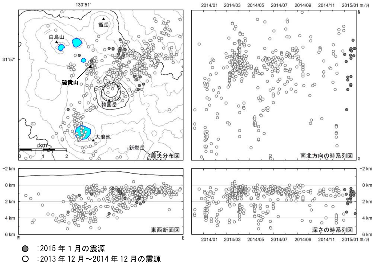
図 13 霧島山（えびの高原（硫黄山）周辺） 震源分布図（2013 年 12 月～2015 年 1 月）
