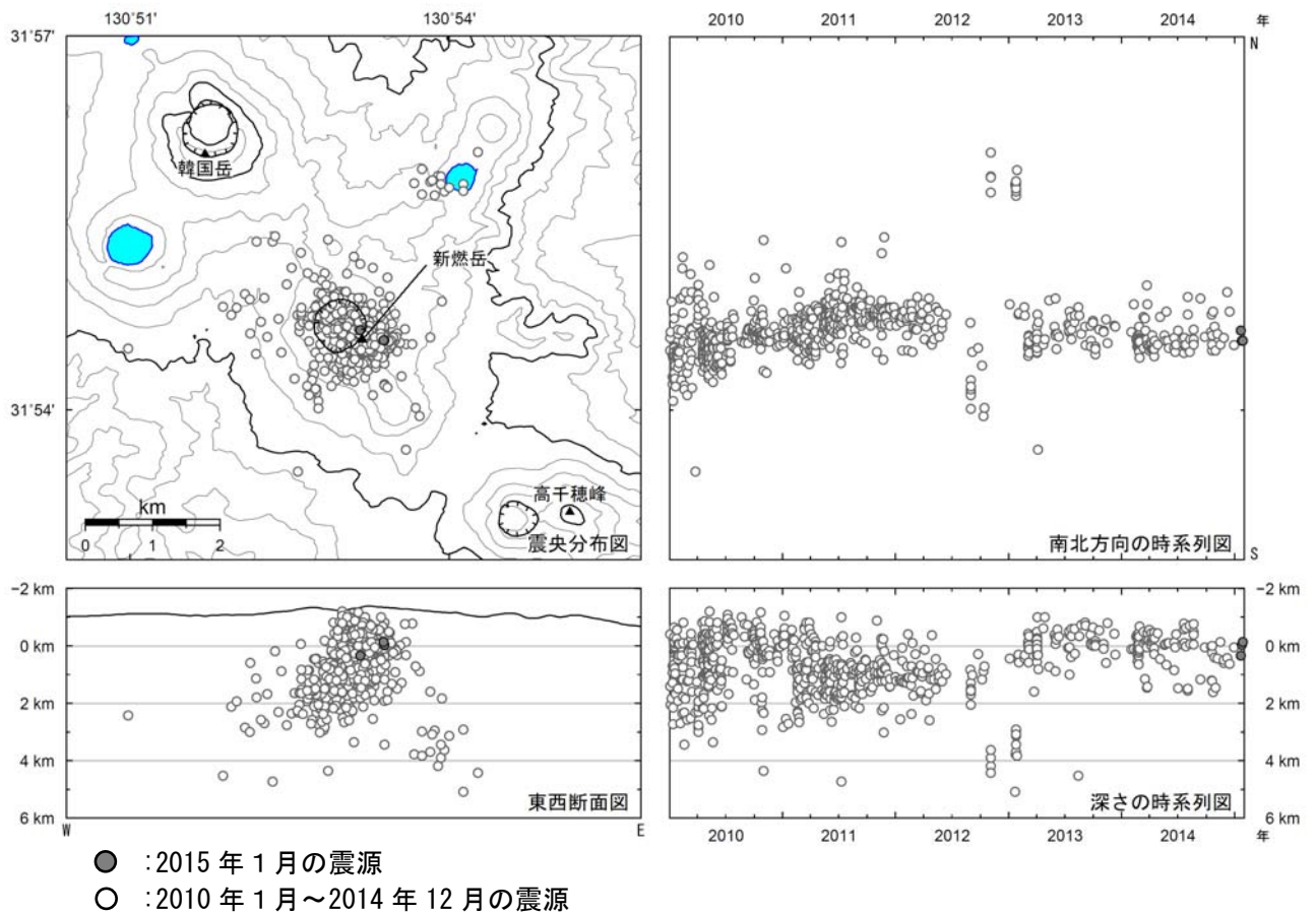
図 2 霧島山（新燃岳） 震源分布図（2010年1月～2015年1月）
