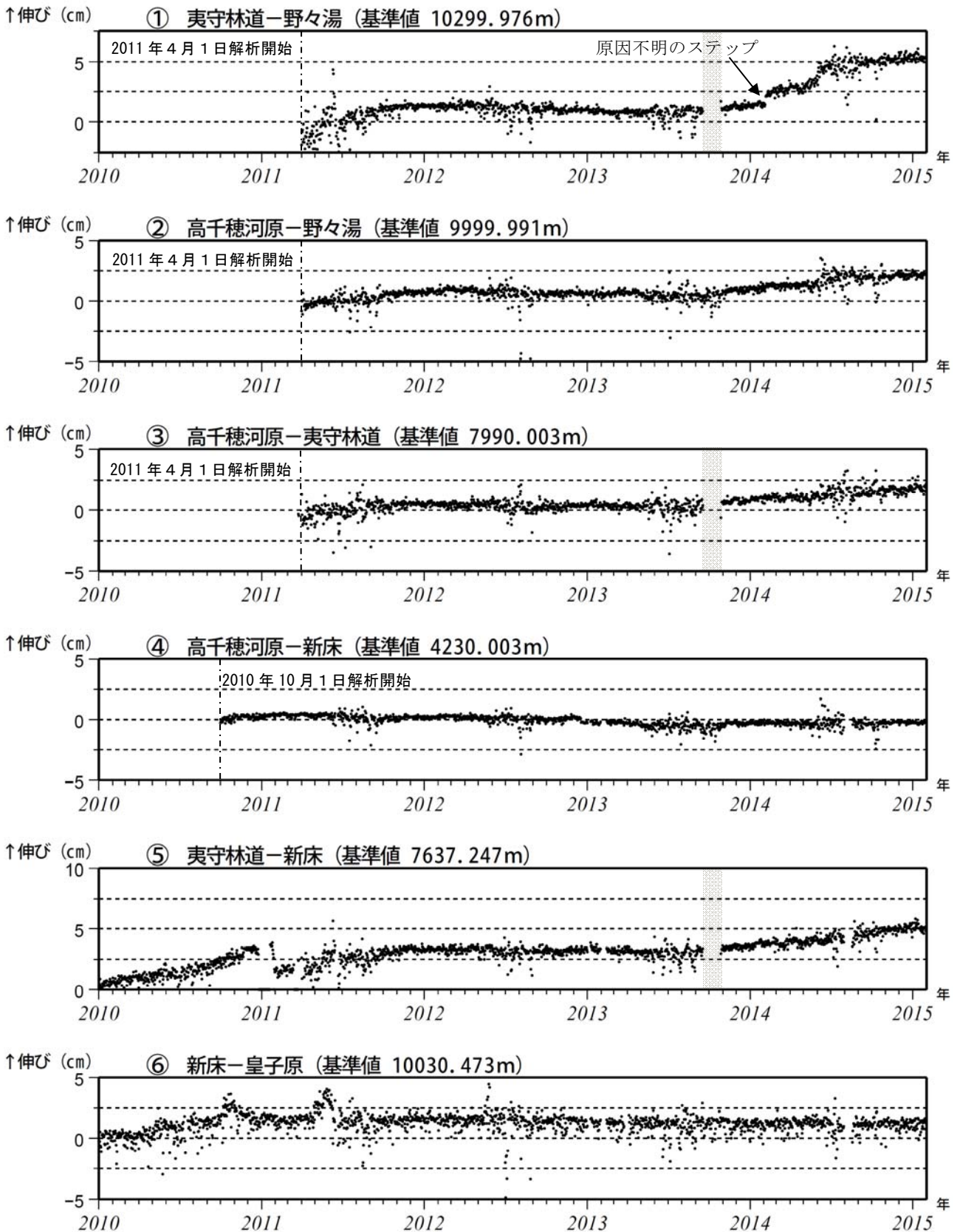
図 6-1 霧島山 GNSS 連続観測による基線長変化 (2010 年 1 月～2015 年 1 月)
