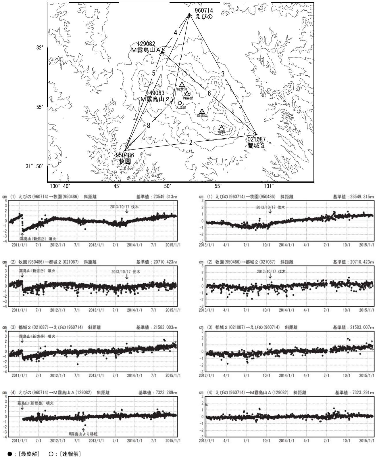
図5 霧島山（新燃岳） 国土地理院による広域的な地殻変動観測結果* (2010年10月1日～2015年1月26日)
