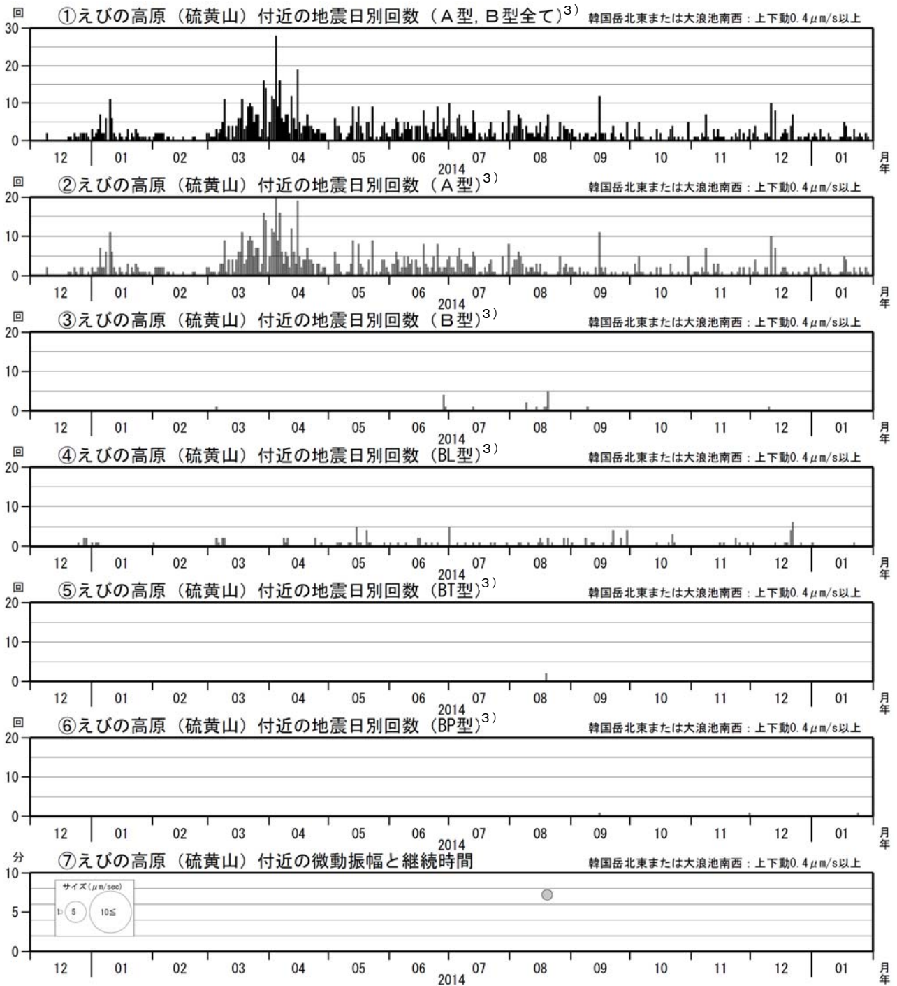
図 12 霧島山（えびの高原（硫黄山）周辺） 火山活動経過図（2013 年 12 月～2015 年 1 月）
