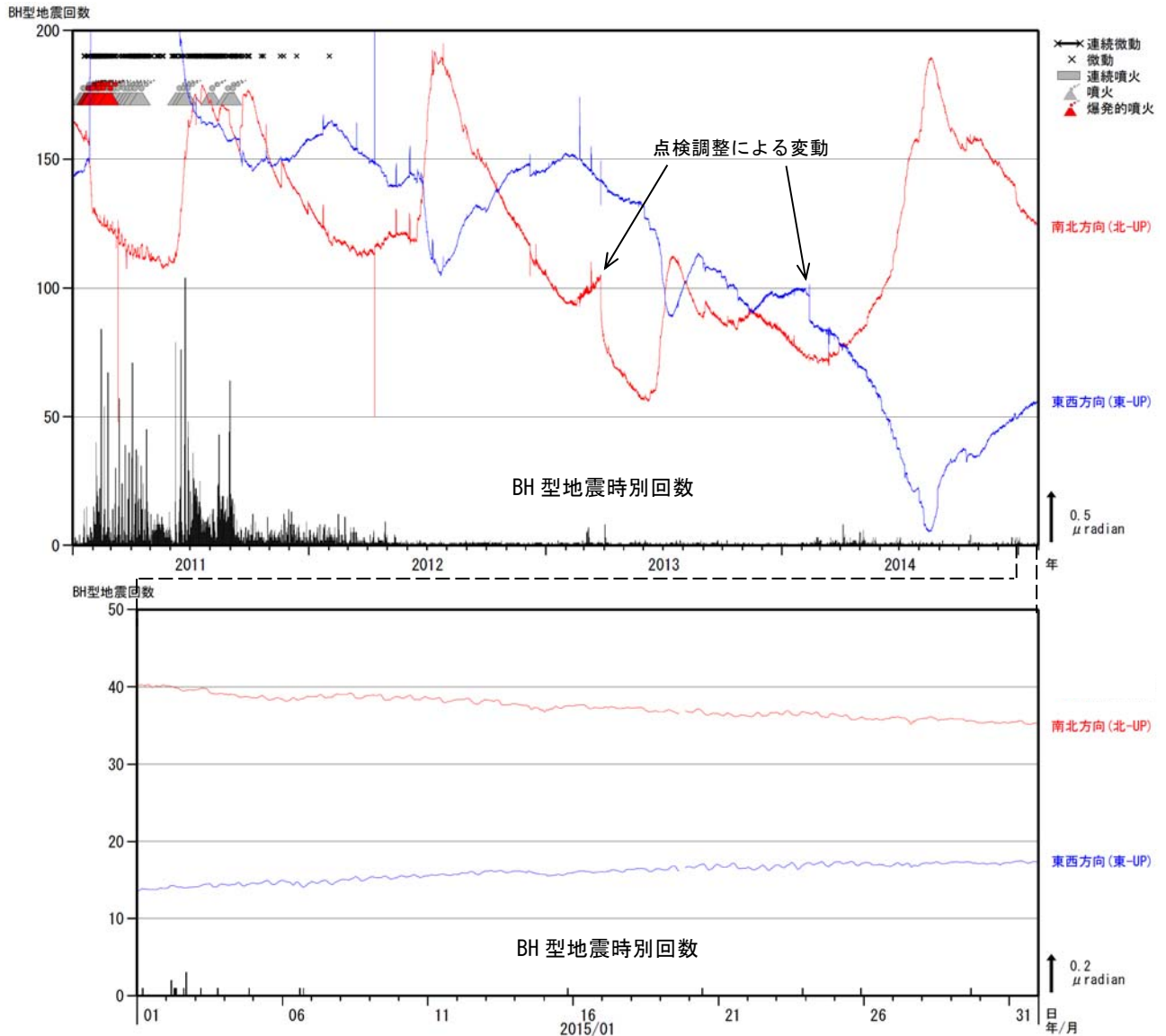
図4 霧島山（新燃岳） BH型地震の時間別回数と高千穂河原傾斜計の傾斜変動（2011年1月～2015年1月）
