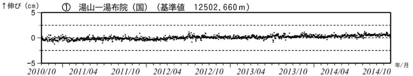
図3 鶴見岳・伽藍岳 GNSS連続観測による基線長変化（2010年10月～2014年11月）
