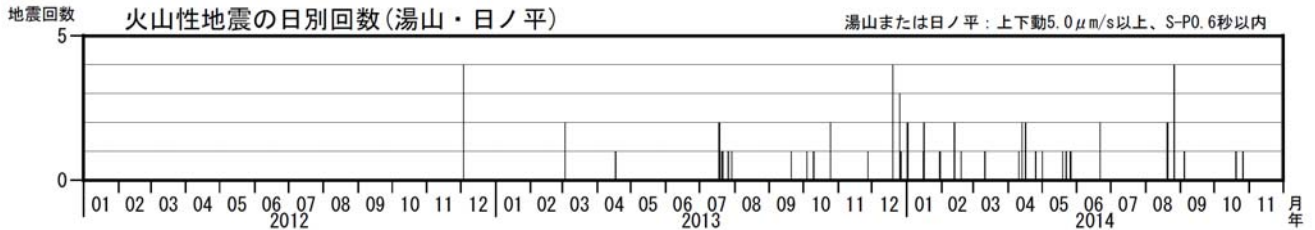
図2 鶴見岳・伽藍岳 火山性地震の日別回数（2012年1月～2014年11月）
