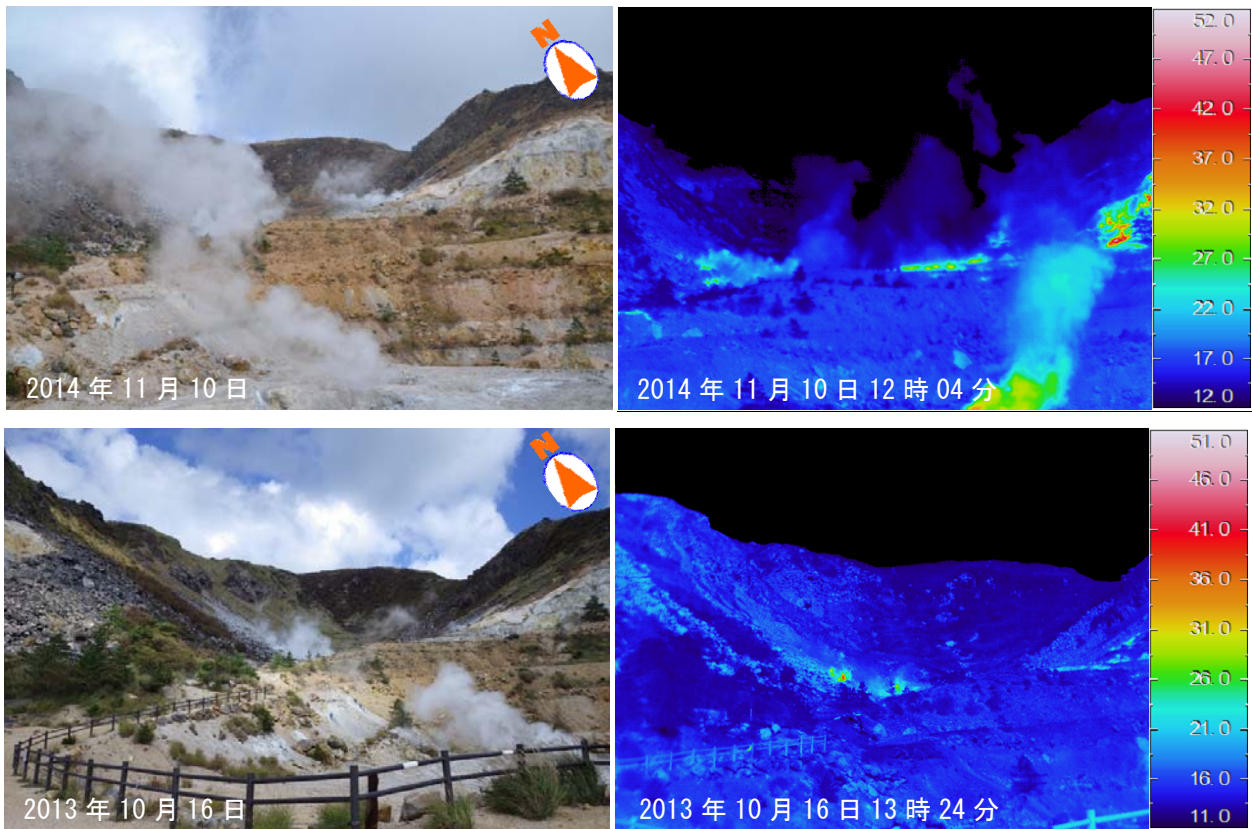
図 7 鶴見岳・伽藍岳 伽藍岳西側の可視及び赤外熱映像装置による地表面温度分布の変化 熱異常域の分布に特段の変化は認められませんでした。
