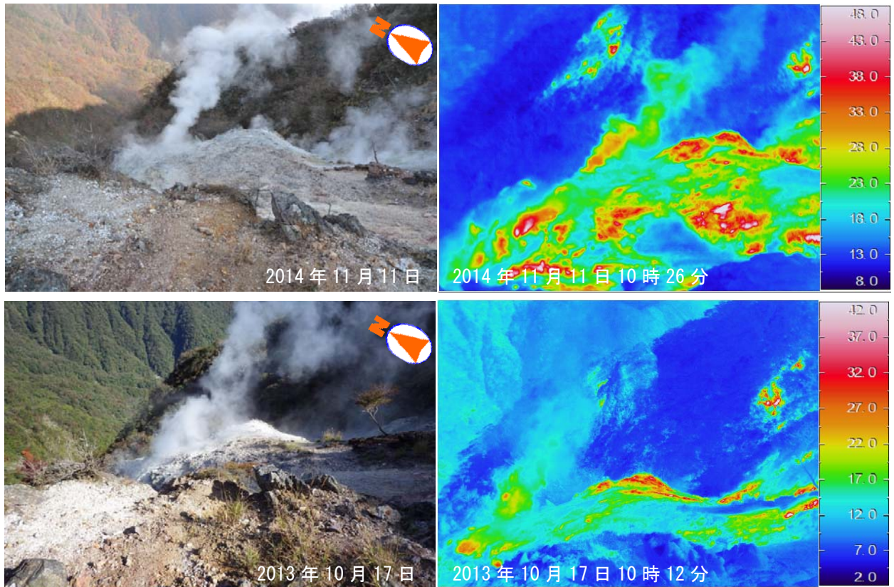
図9 鶴見岳・伽藍岳 鶴見岳地獄谷赤池噴気孔の可視及び赤外熱映像装置による 地表面温度分布の変化
