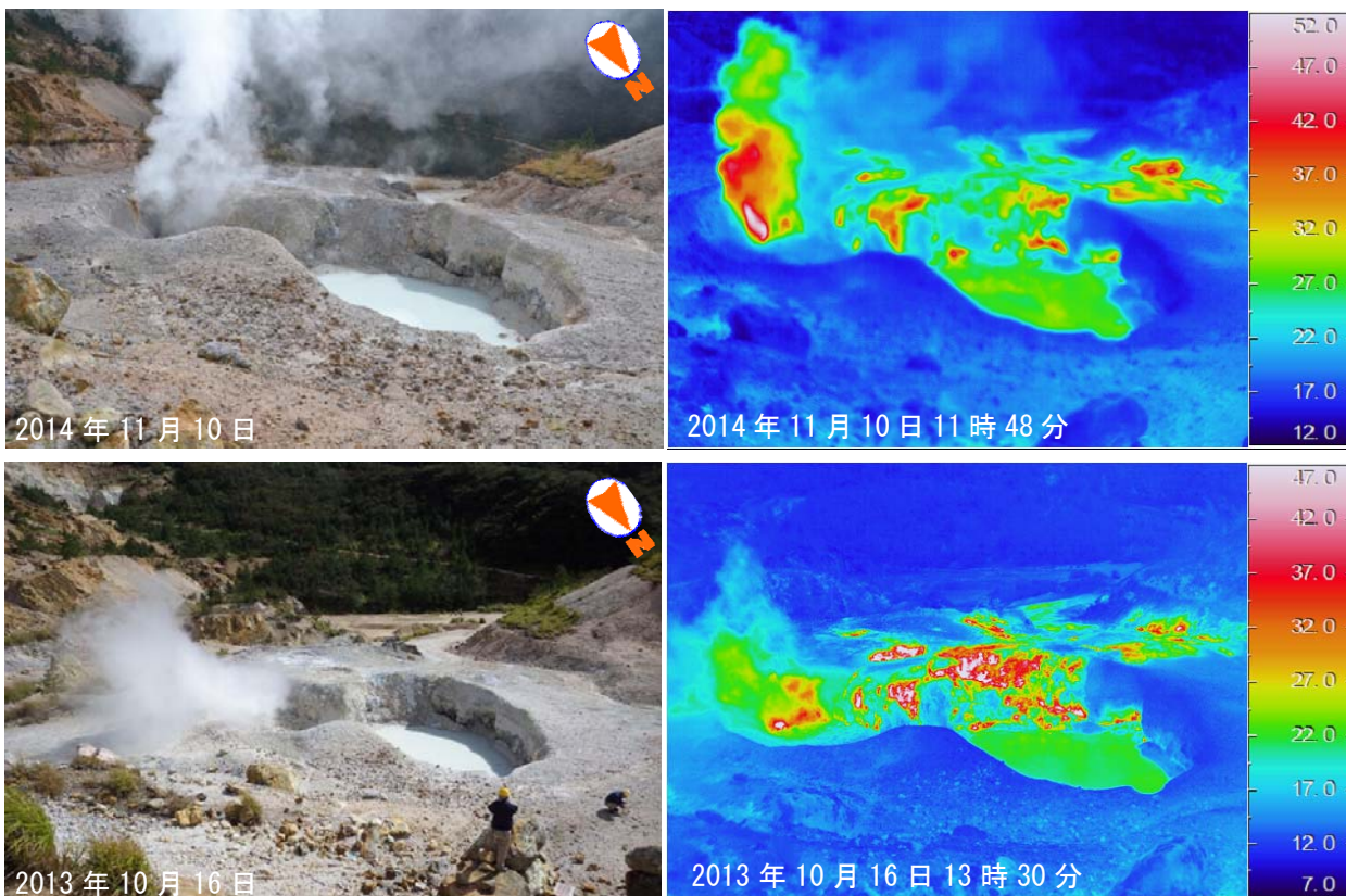
図 5 鶴見岳・伽藍岳 伽藍岳泥火山の可視及び赤外熱映像装置による地表面温度分布の変化 熱異常域の分布に特段の変化は認められませんでした。
