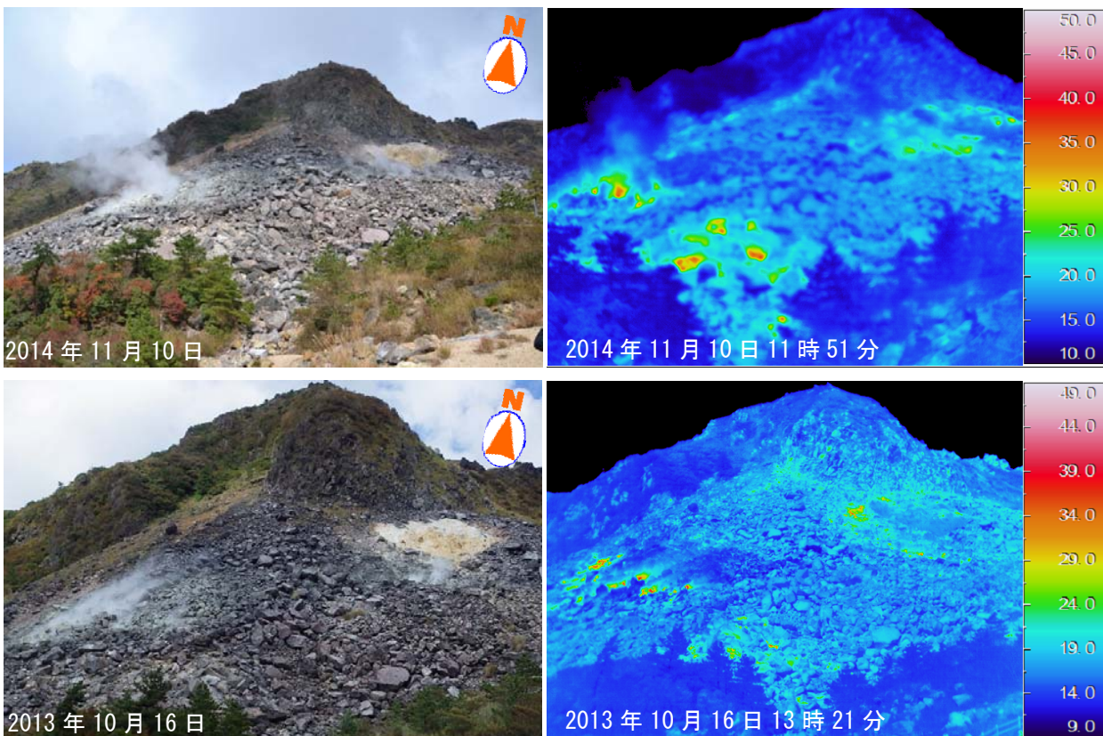
図 6 鶴見岳・伽藍岳 伽藍岳南側の可視及び赤外熱映像装置による地表面温度分布の変化 熱異常域の分布に特段の変化は認められませんでした。
