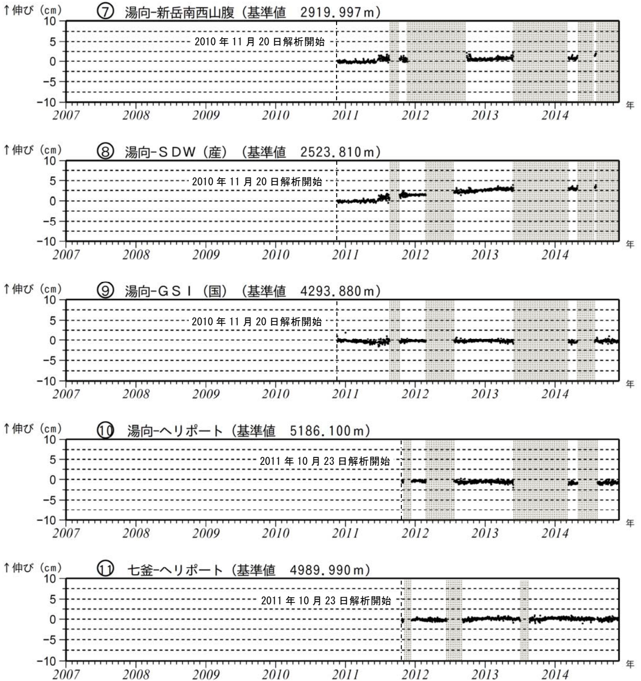
図 3-2 口永良部島 GNSS 連続観測による基線長変化（2007 年 1 月～2014 年 11 月）
