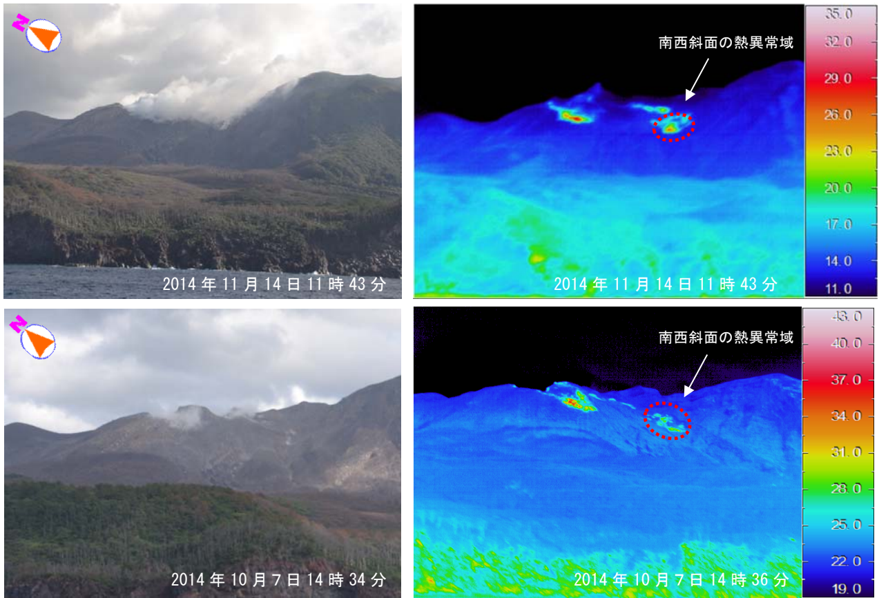
図 6-2 口永良部島 赤外熱映像装置による新岳火口付近の地表面温度分布（西南西側海上より撮影） ・新岳火口および西側割れ目付近や、前回（10月7日）の調査で新たに確認された新岳の南西斜面の噴気は、今回の観測でも確認しました。 ・赤外熱映像装置による観測では、新岳火口縁の西側、西側の割れ目付近および南西斜面の噴気地帯で熱異常域を確認しました。
