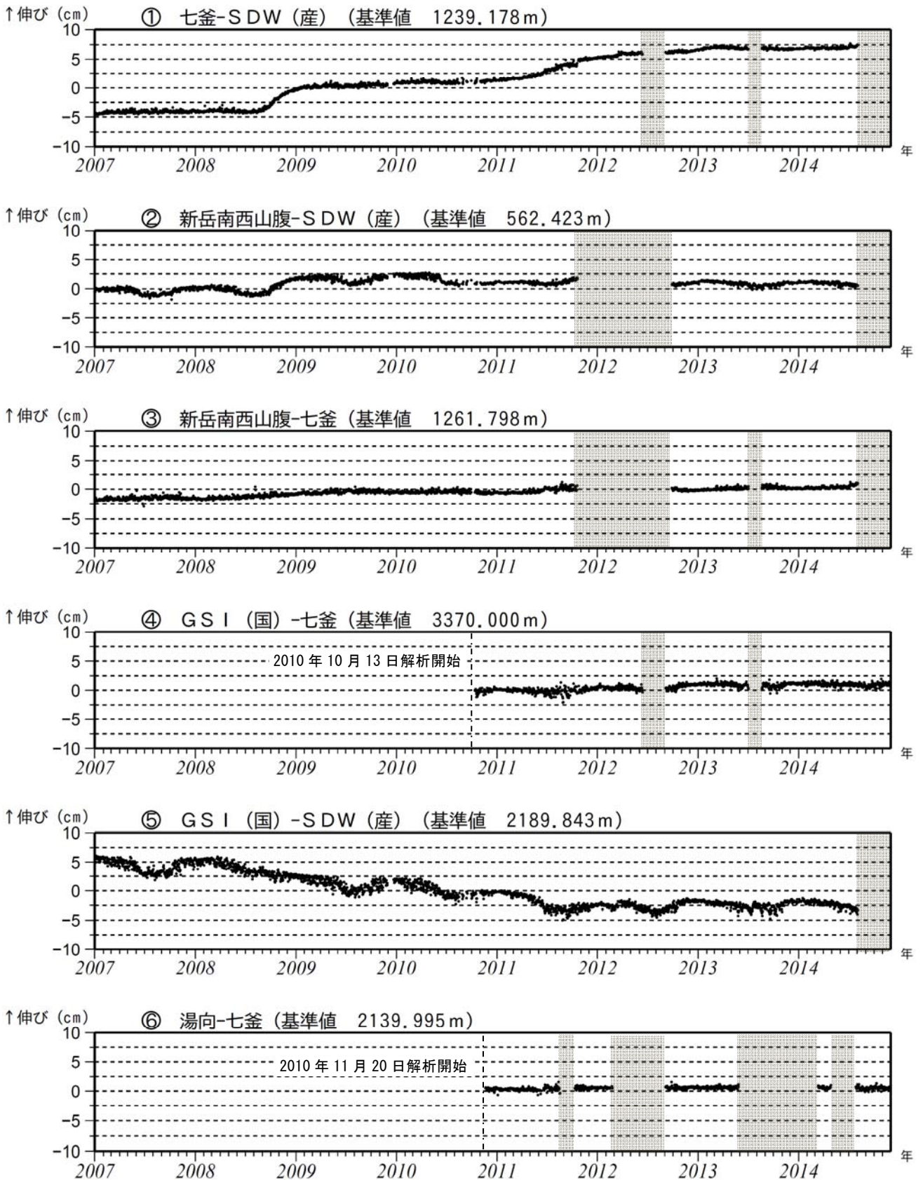
図 3-1 口永良部島 GNSS 連続観測による基線長変化（2007 年 1 月～2014 年 11 月）
