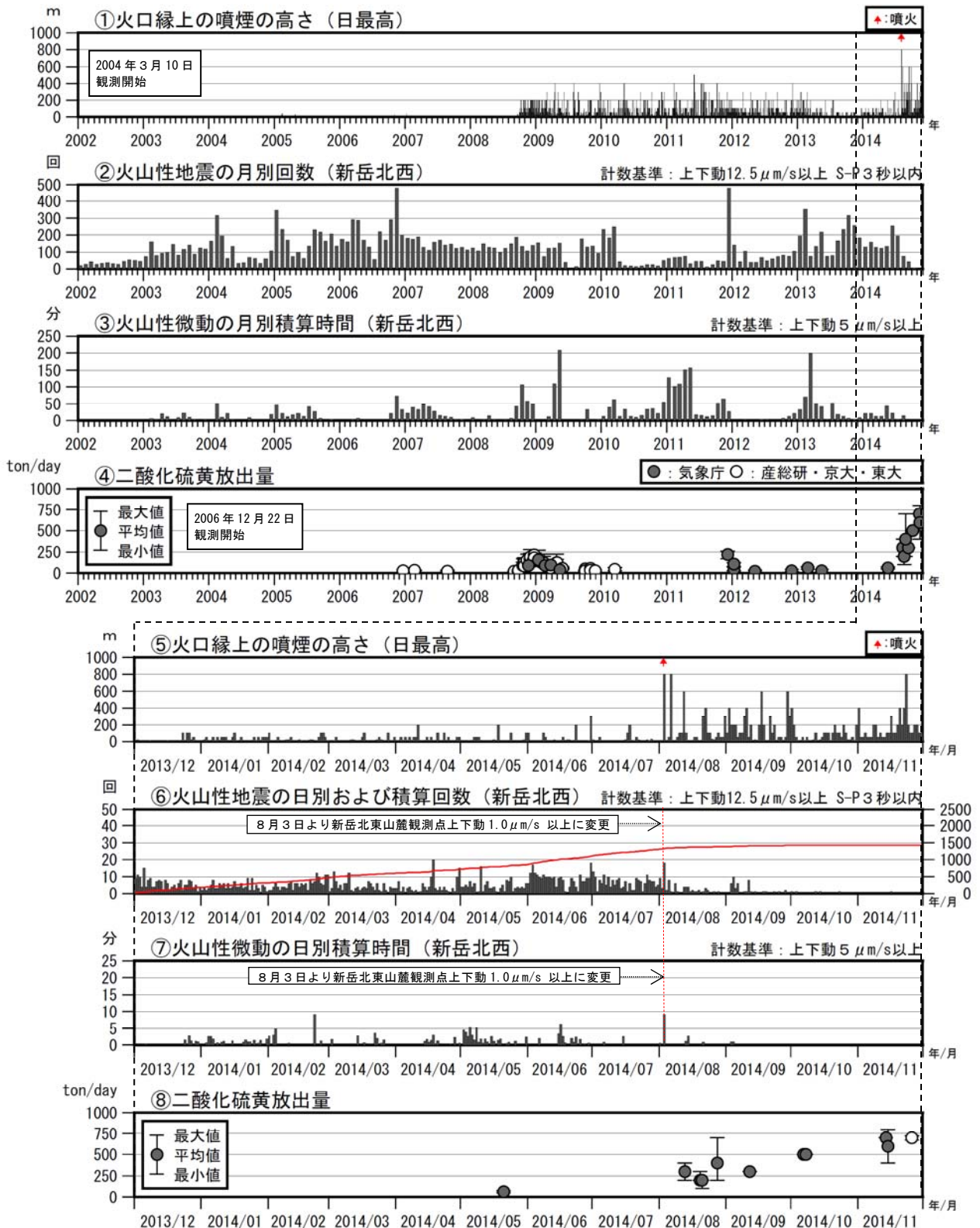
図2 口永良部島 火山活動経過図（2002年1月～2014年11月）
