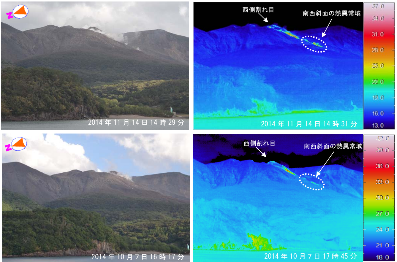
図 6-1 口永良部島 赤外熱映像装置による新岳火口付近の地表面温度分布（本村より撮影） 新岳火口縁の西側、西側の割れ目付近および南西斜面の噴気地帯で熱異常域を確認しました。
