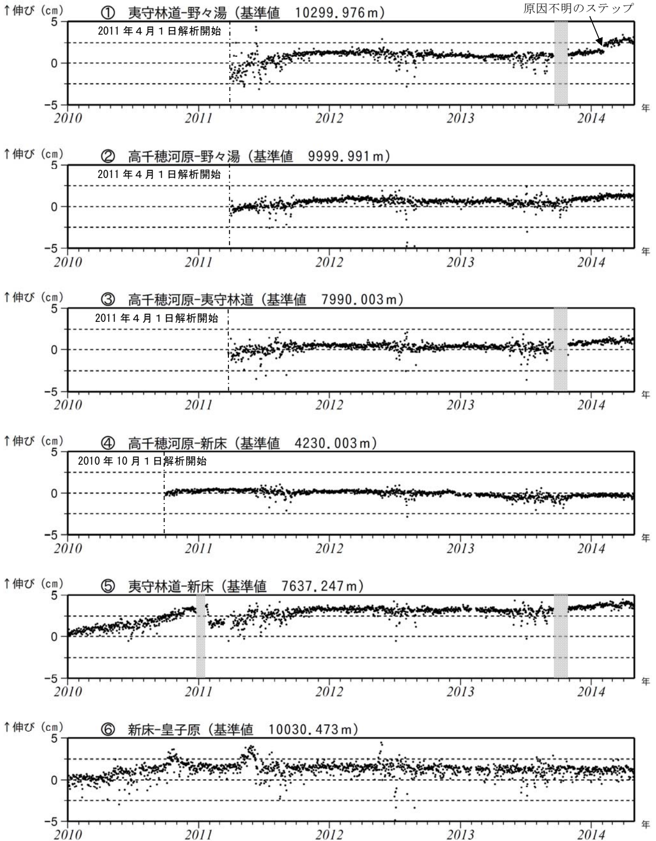
図 6-1 霧島山 GNSS 連続観測による基線長変化（2010 年 1 月～2014 年 4 月）
