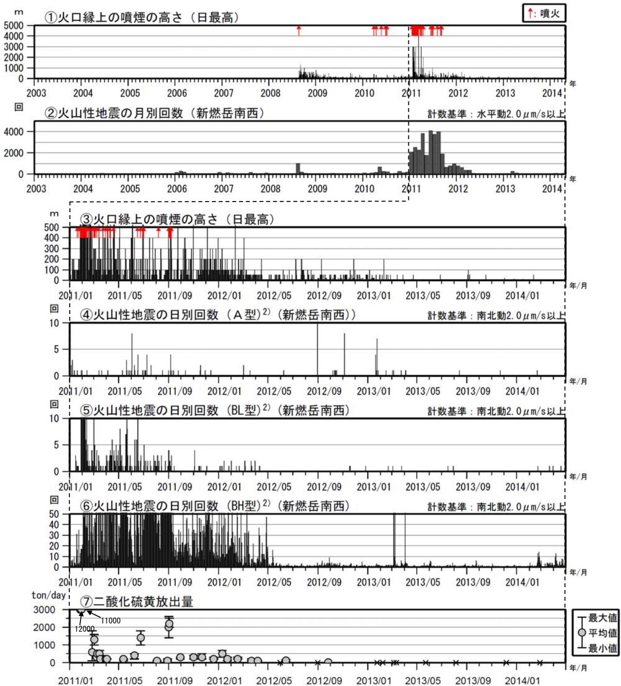
図3 霧島山（新燃岳） 火山活動経過図（2003年1月～2014年4月）
