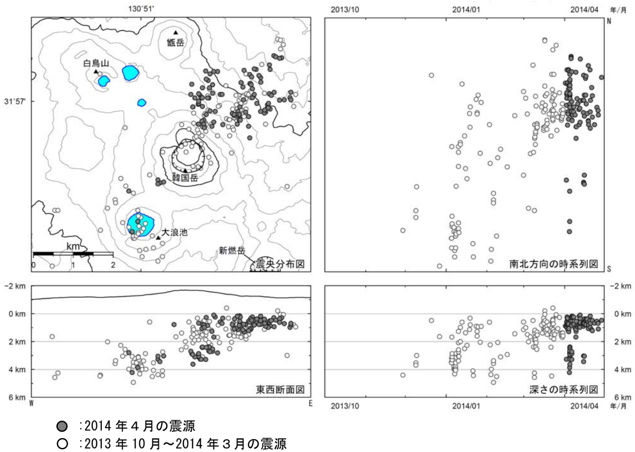
図9 霧島山（韓国岳、大浪池付近） 震源分布図（2013 年 10 月～2014 年 4 月）
