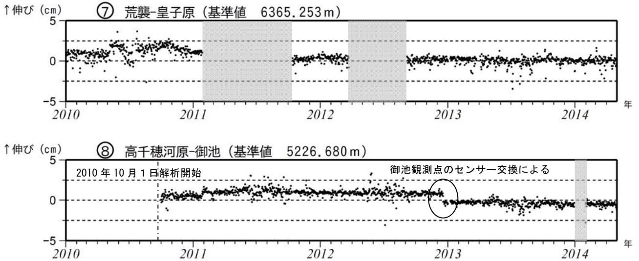
図 6-2 霧島山 GNSS 連続観測による基線長変化（2010 年 1 月～2014 年 4 月）
