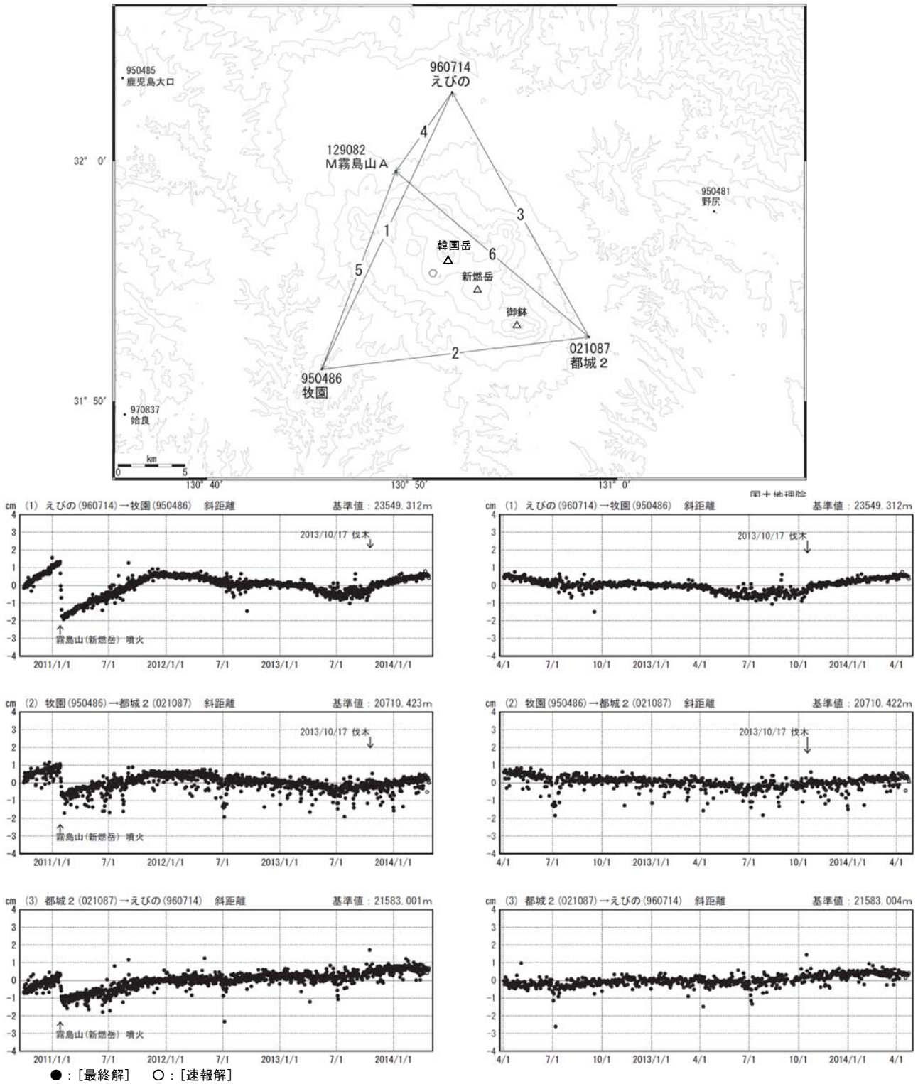
図 5 霧島山（新燃岳） 国土地理院による広域的な地殻変動観測結果*
