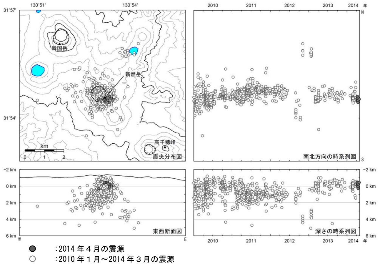
図 2 霧島山（新燃岳） 震源分布図（2010 年 1 月～2014 年 4 月）
