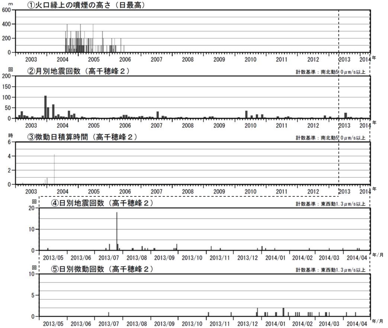
図 11 霧島山（御鉢） 火山活動経過図（2003 年 1 月～2014 年 4 月）
