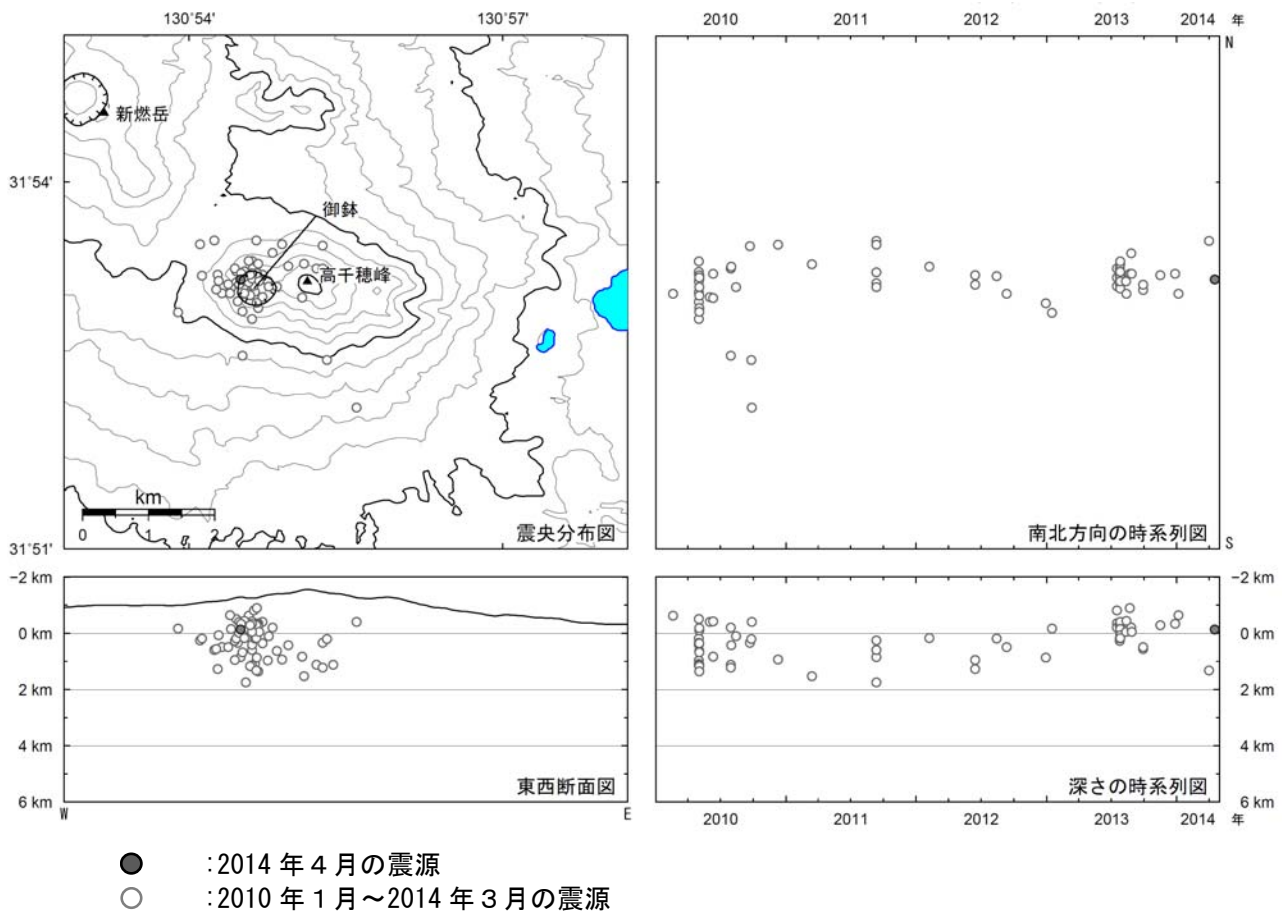
図 12 霧島山（御鉢） 震源分布図（2010 年 1 月～2014 年 4 月）
