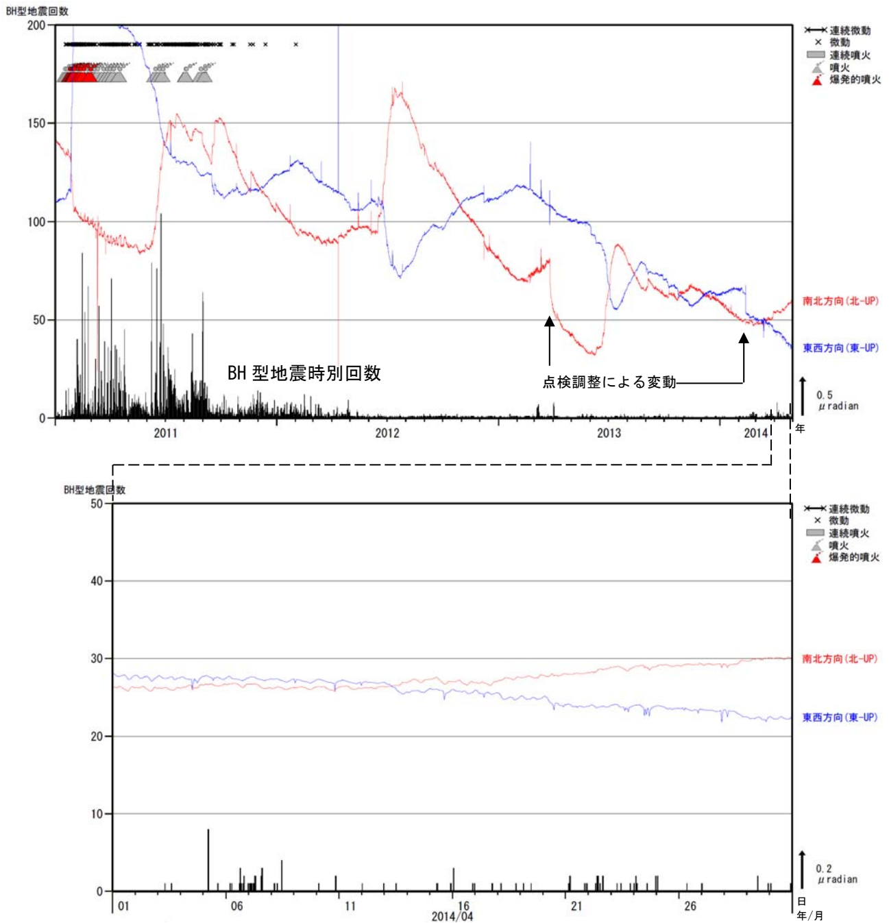
図4 霧島山（新燃岳） BH型地震の時間別回数と高千穂河原傾斜計の傾斜変動（2011年1月～2014年4月）
