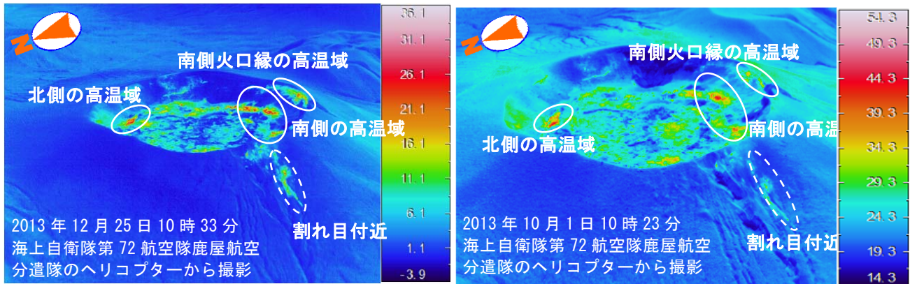
図 11 霧島山（新燃岳）新燃岳の火口内および西側斜面の地表面温度分布 （左：2013 年 12 月 25 日、右：2013 年 10 月 1 日）
