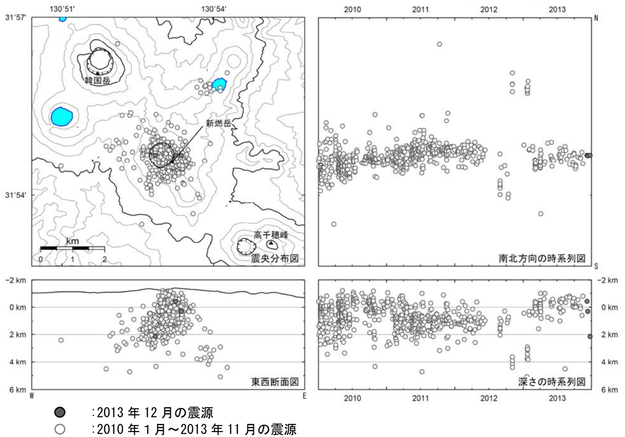
図 2 霧島山（新燃岳） 震源分布図（2010年1月～2013年12月）
