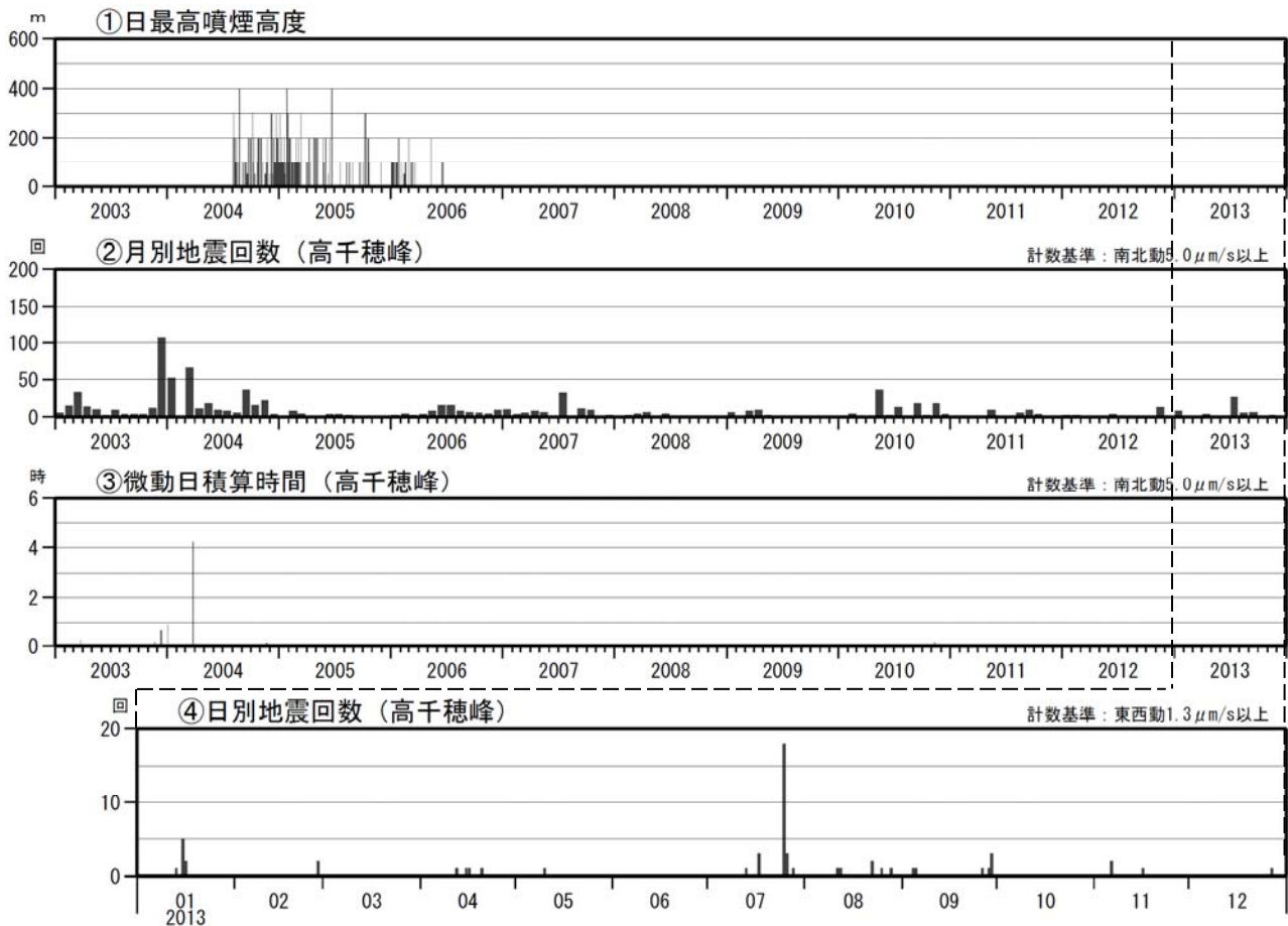
図 14 霧島山（御鉢） 火山活動経過図（2003 年 1 月～2013 年 12 月）
