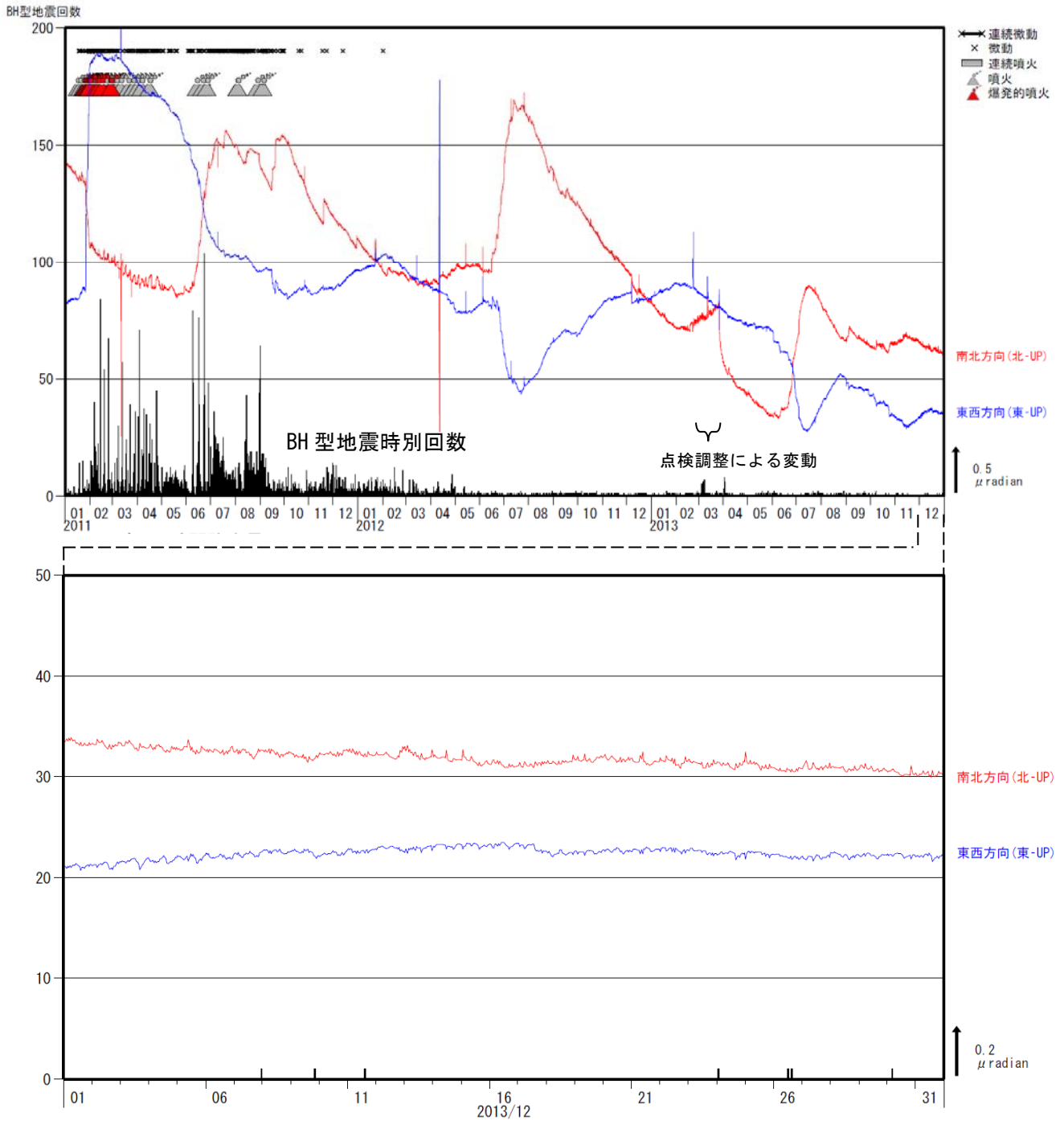
図4 霧島山（新燃岳） BH型地震の時間別回数と高千穂河原傾斜計の傾斜変動 (2011年1月～2013年12月)
