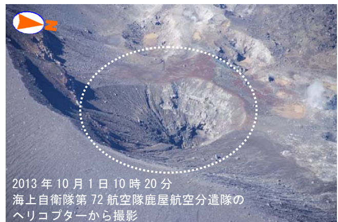
図 10 霧島山（新燃岳）新燃岳の火口内の状況 （左：2013 年 12 月 25 日、右：2013 年 10 月 1 日、北東側より撮影）
