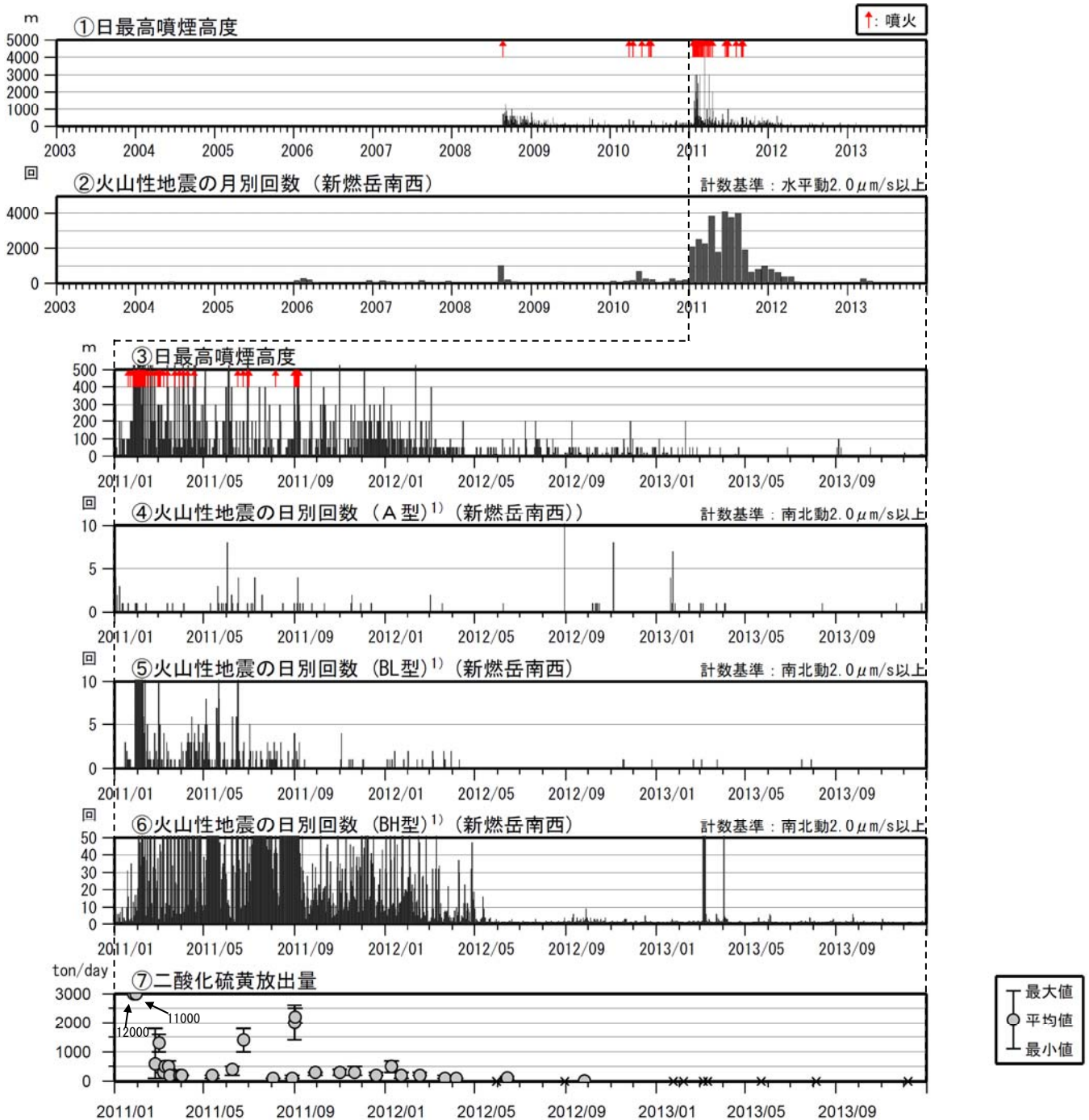
図3 霧島山（新燃岳） 火山活動経過図（2003年1月～2013年12月）
