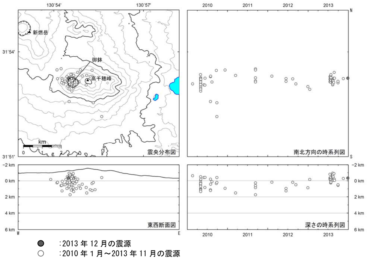
図 13 霧島山（御鉢） 震源分布図（2010 年 1 月～2013 年 12 月）
