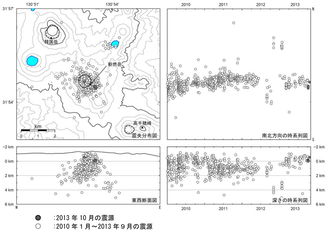
図 2 霧島山（新燃岳） 震源分布図（2010 年 1 月～2013 年 10 月）
