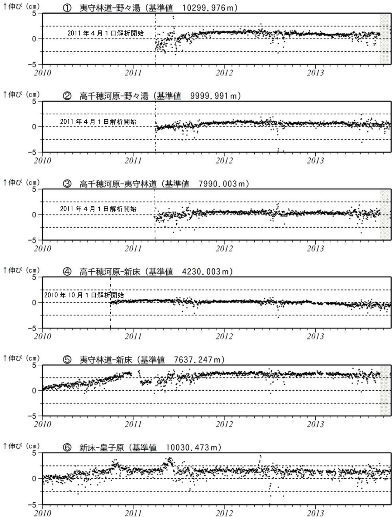
図 6-1 霧島山 GPS 連続観測による長期の基線長変化 (2010 年 1 月～2013 年 10 月)
