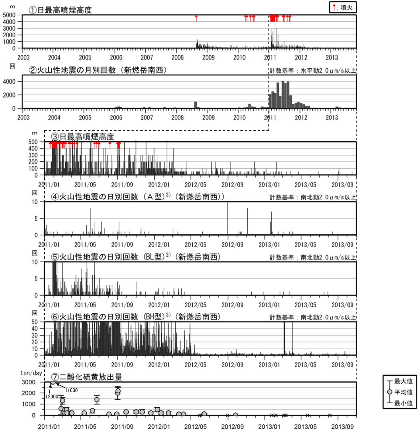
図3 霧島山（新燃岳） 火山活動経過図（2003年1月～2013年10月）
