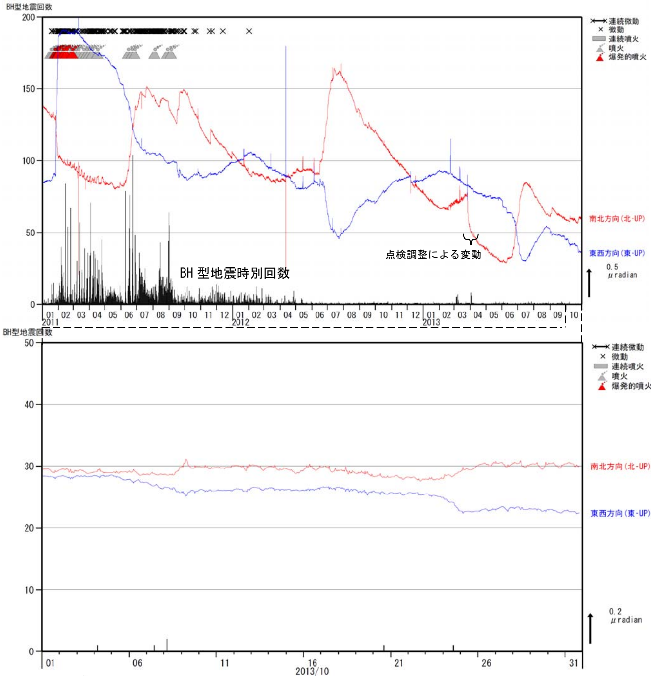
図 4-1 霧島山（新燃岳） BH 型地震の時間別回数と高千穂河原傾斜計の傾斜変動 (2011 年 1 月～2013 年 10 月)
