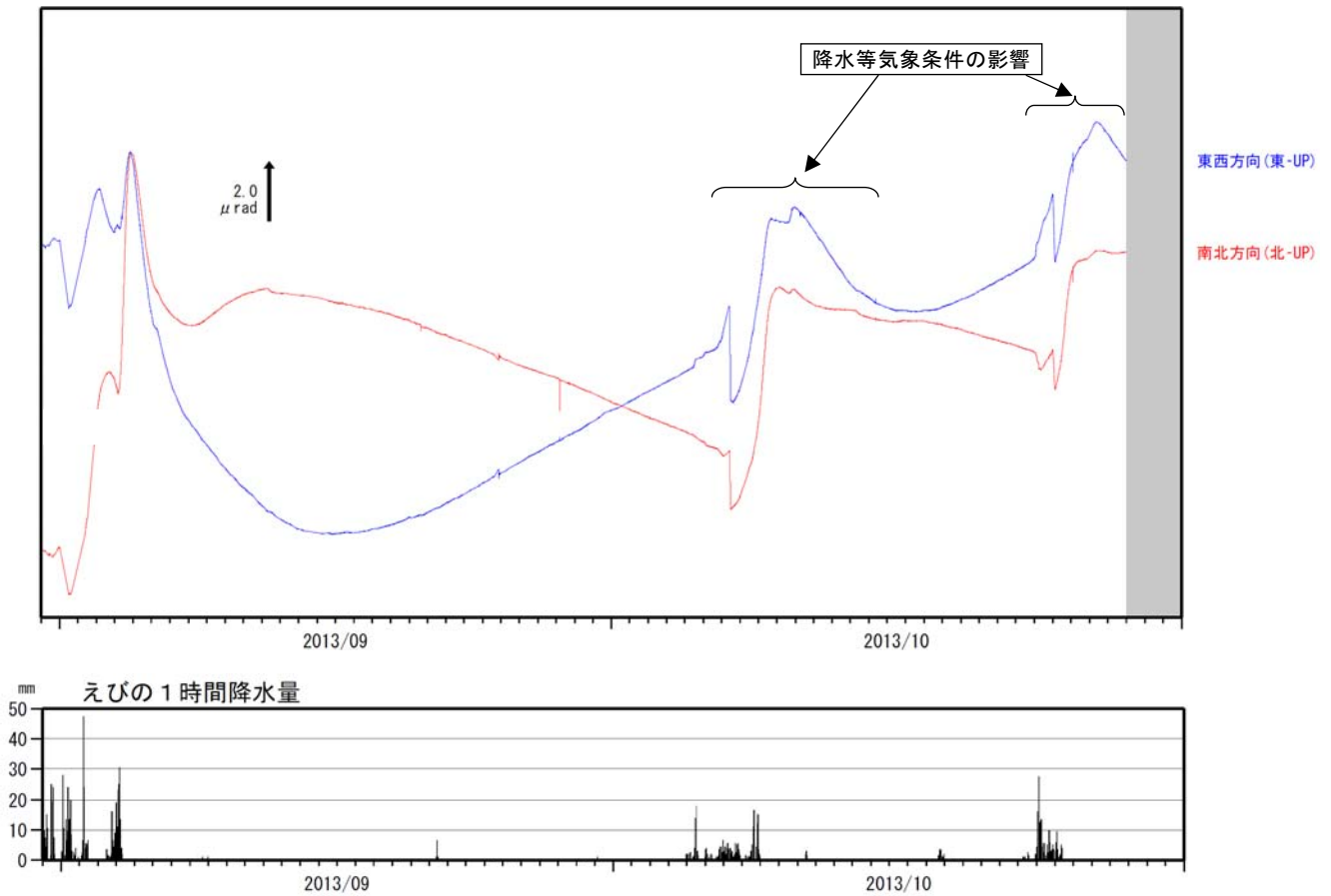
図 4-2 霧島山（新燃岳） 新燃岳北東傾斜計の傾斜変動とえびのの 1 時間降水量 （2013 年 8 月 31 日～10 月）
