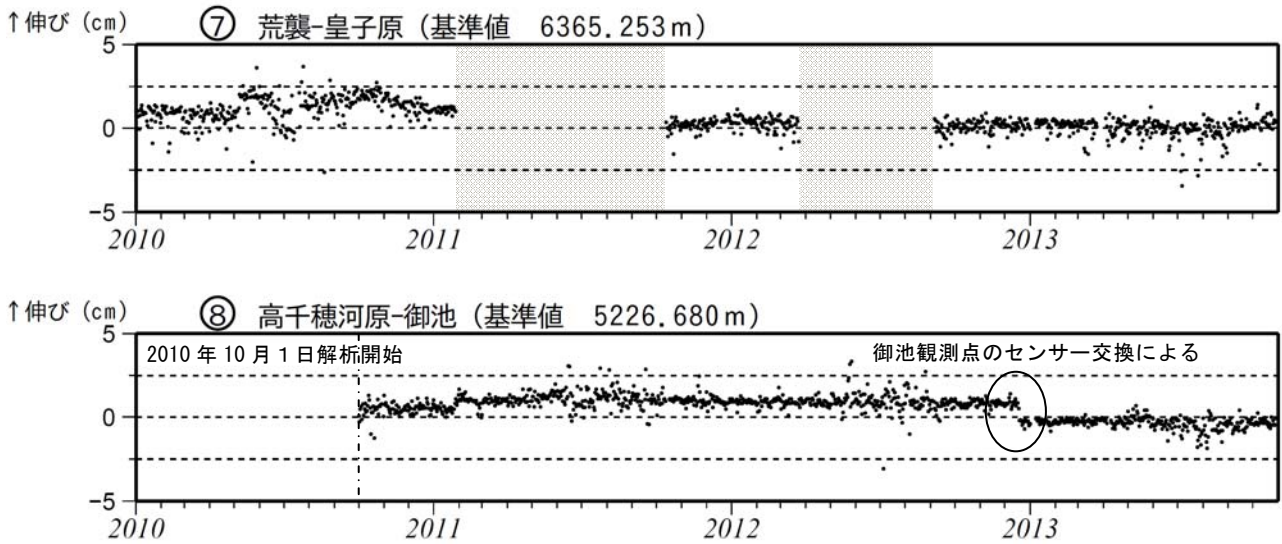
図 6-2 霧島山 GPS 連続観測による長期の基線長変化 (2010 年 1 月～2013 年 10 月)
