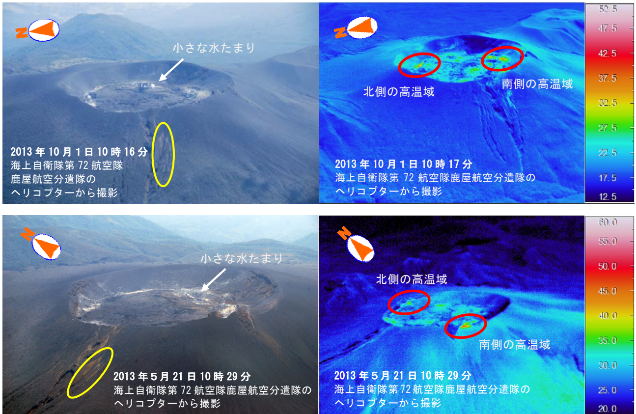
図9 霧島山（新燃岳）火口内の状況（左）および赤外熱映像装置による火口付近の地表面温度分布（右）
