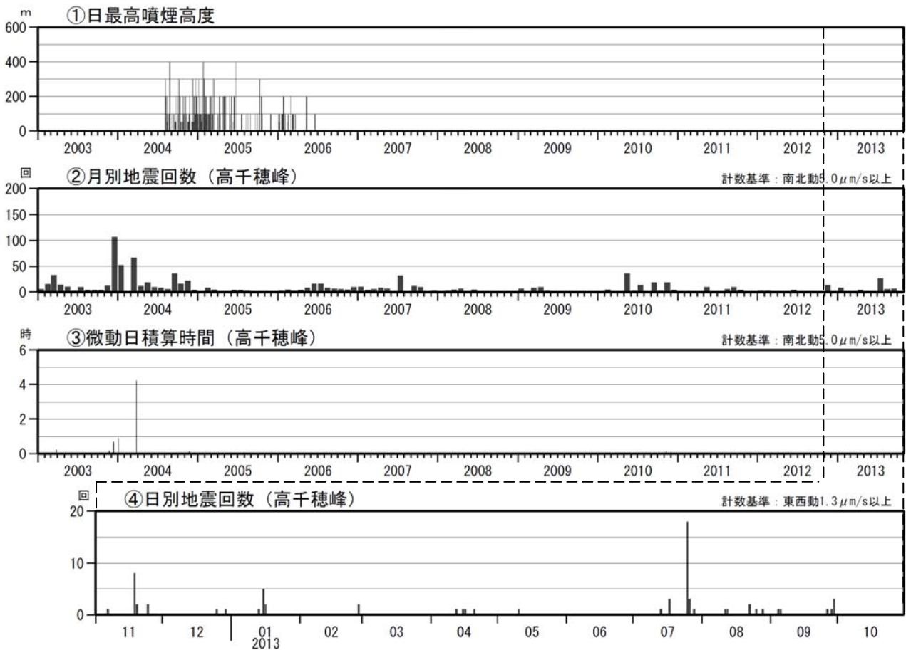
図 11 霧島山（御鉢） 火山活動経過図（2003 年 1 月～2013 年 10 月） <10 月の状況>
