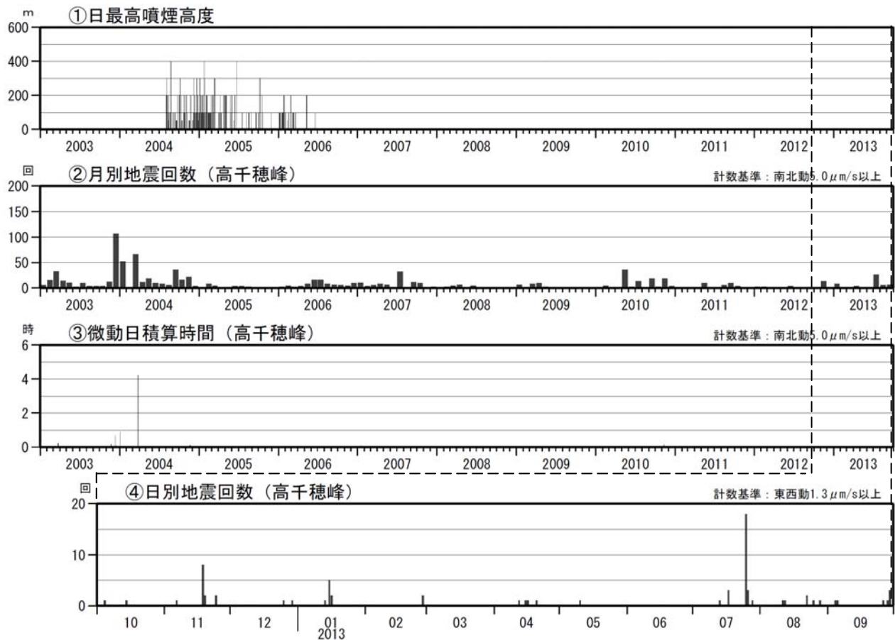
図 11 霧島山（御鉢） 火山活動経過図（2003 年 1 月～2013 年 9 月）
