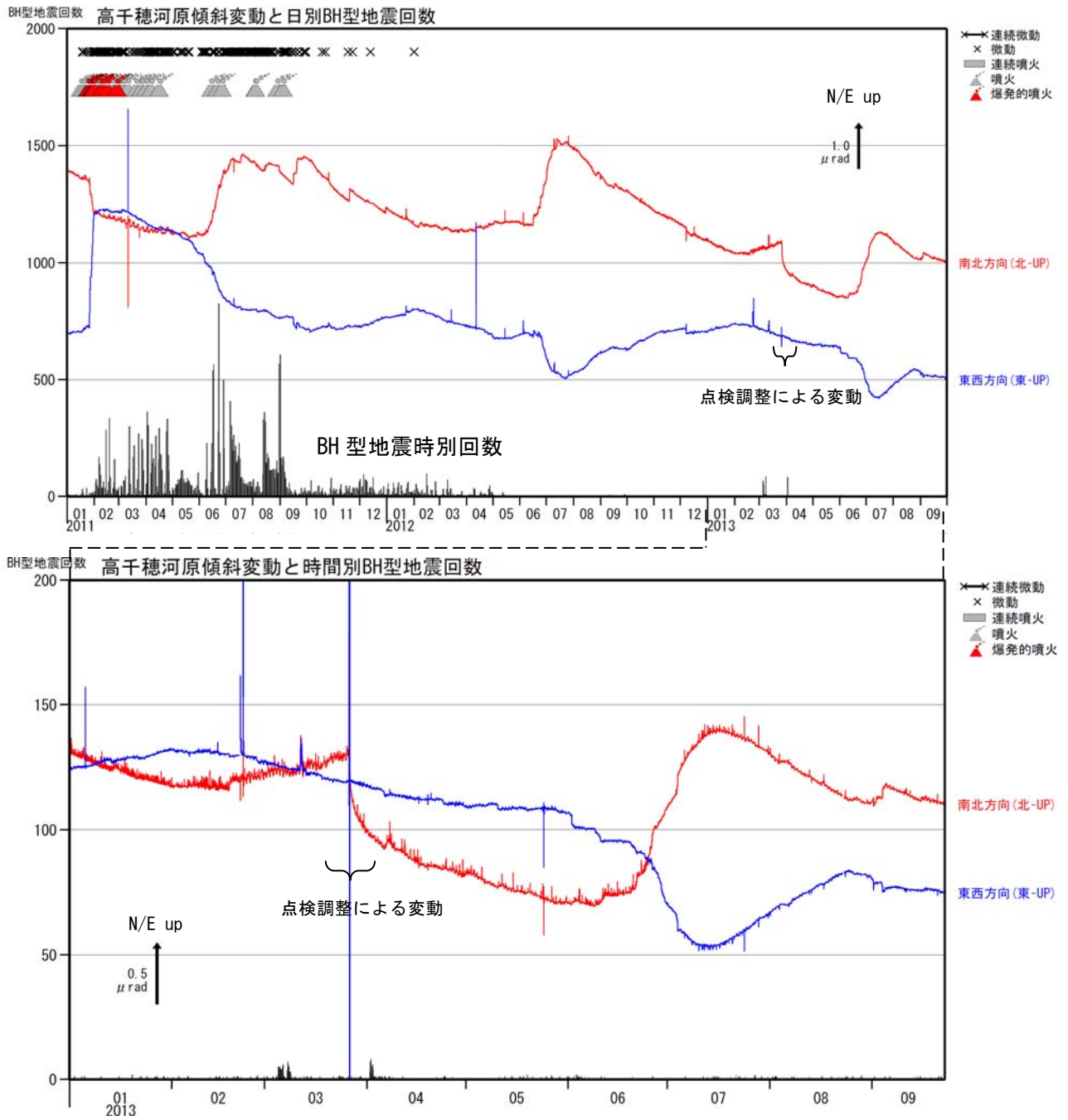
図 4-1 霧島山（新燃岳） BH 型地震の時間別回数と高千穂河原傾斜計の傾斜変動 （2011 年 1 月～2013 年 9 月）
