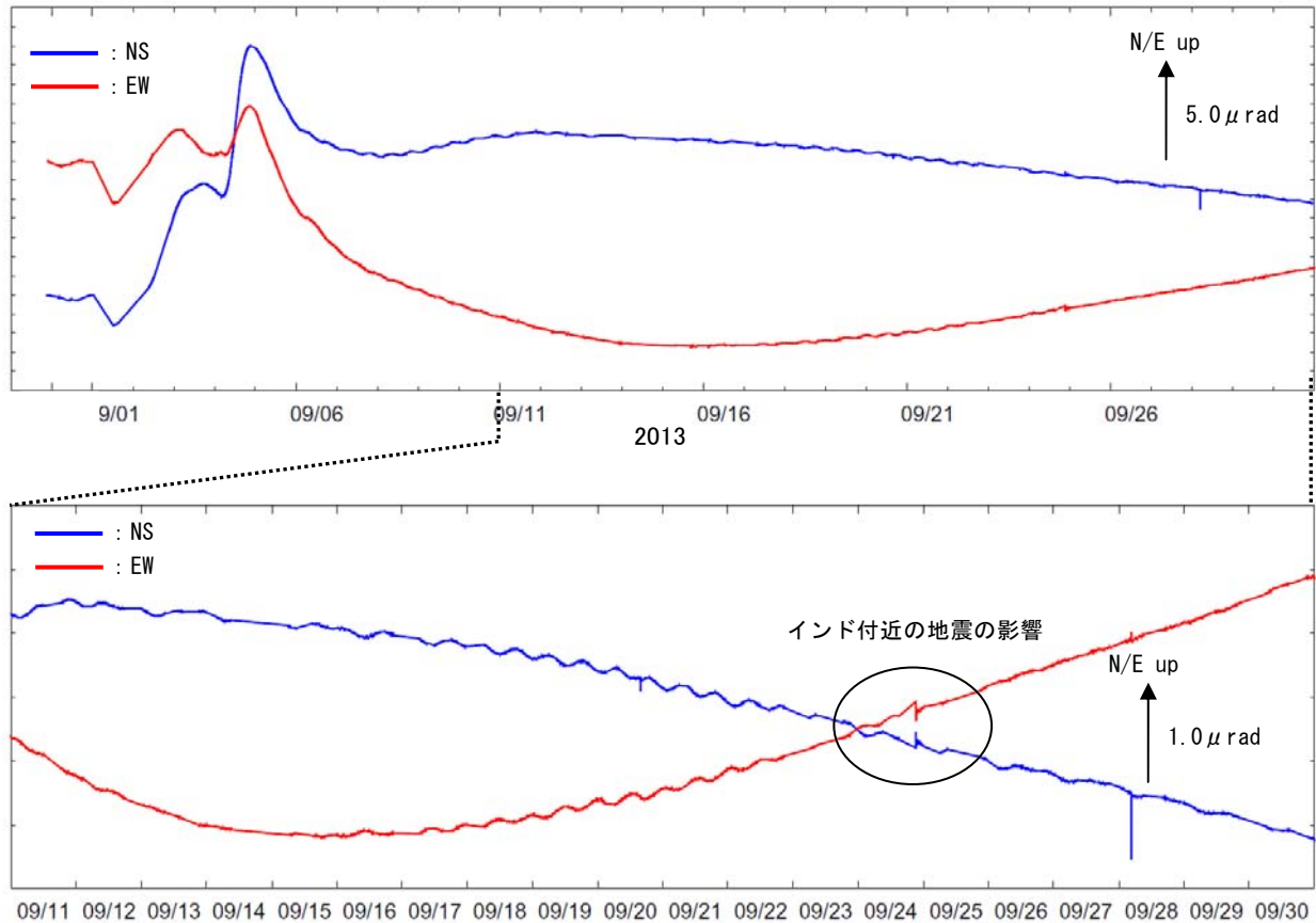
図 4-2 霧島山（新燃岳） 新燃北東傾斜計の傾斜変動（2013 年 8 月 31 日～9 月 30 日）
