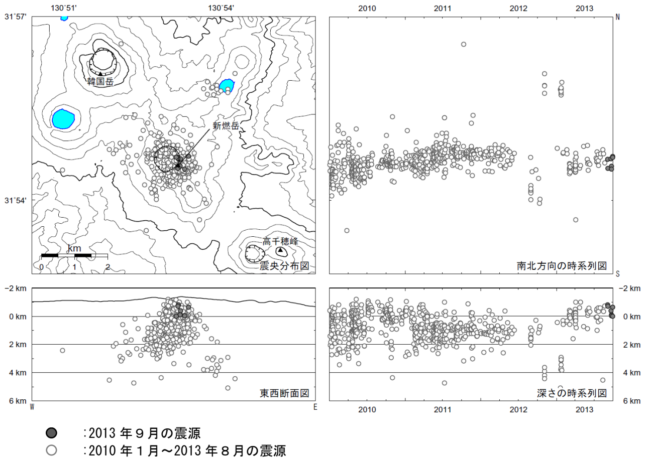
図 2 霧島山（新燃岳） 震源分布図（2010 年 1 月～2013 年 9 月）
