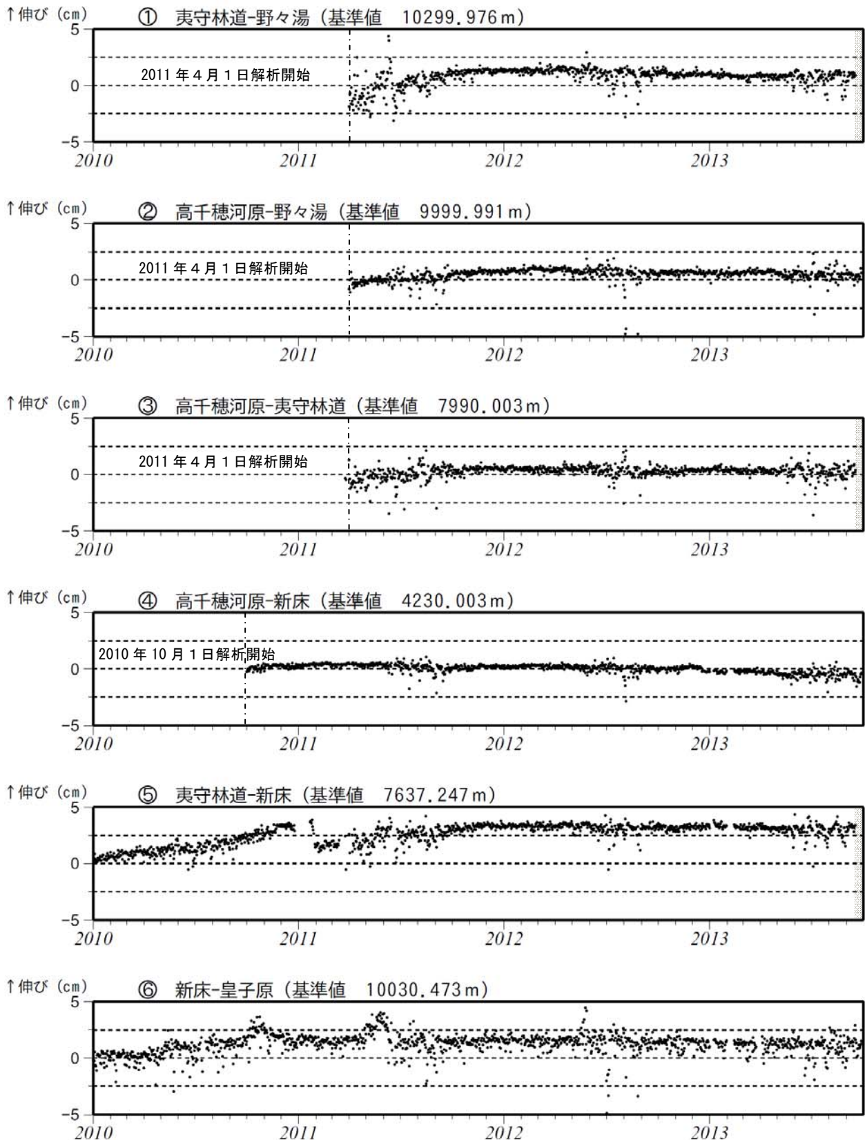
図 6-1 霧島山 GPS 連続観測による長期の基線長変化 (2010 年 1 月～2013 年 9 月)
