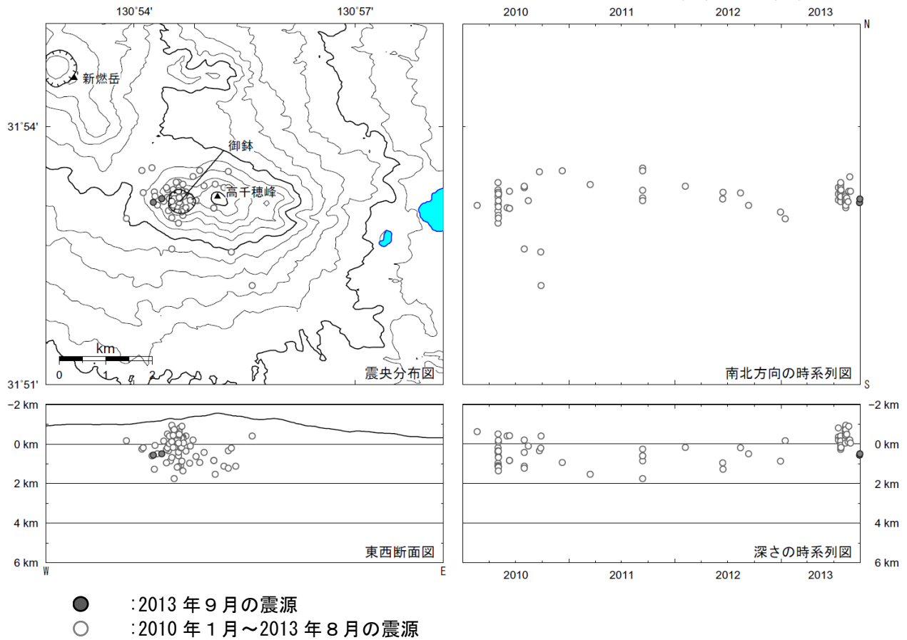
図 10 霧島山（御鉢） 震源分布図（2010 年 1 月～2013 年 9 月）
