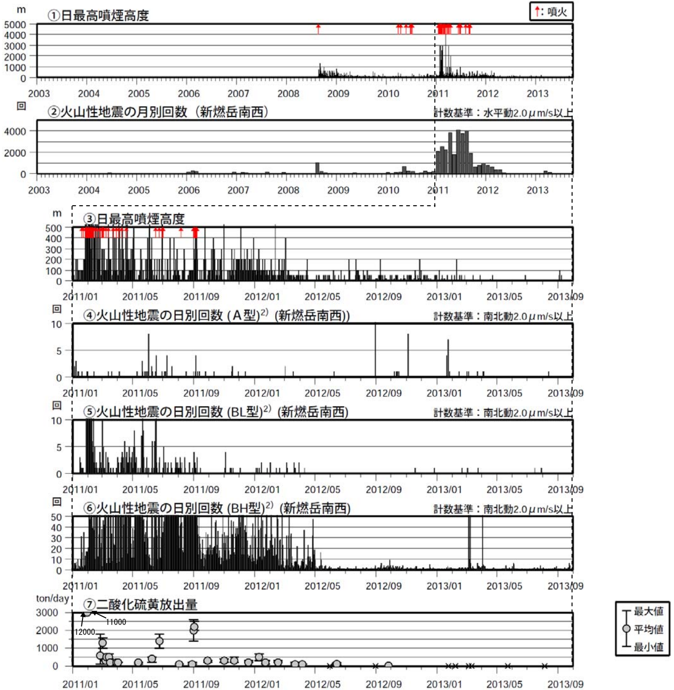
図3 霧島山（新燃岳） 火山活動経過図（2003年1月～2013年9月）
