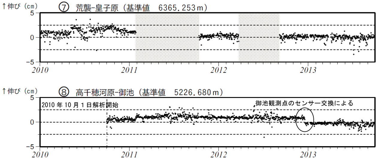
図 6-2 霧島山 GPS 連続観測による長期の基線長変化（2010 年 1 月～2013 年 9 月）
