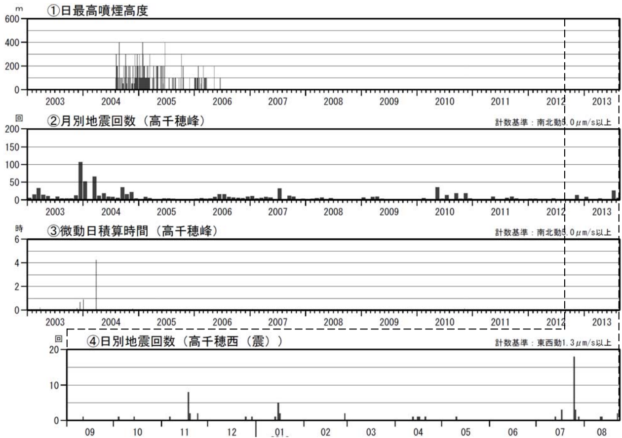
図 11 霧島山（御鉢） 火山活動経過図（2003 年 1 月～2013 年 8 月）
