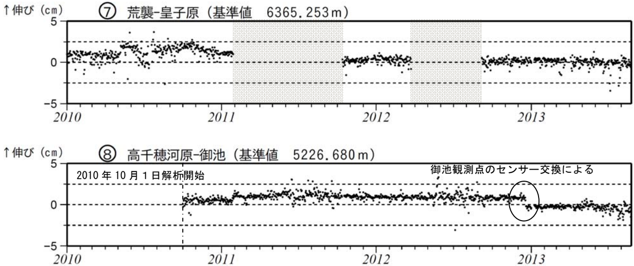
図 6-2 霧島山 GPS 連続観測による長期の基線長変化（2010 年 1 月～2013 年 8 月）
