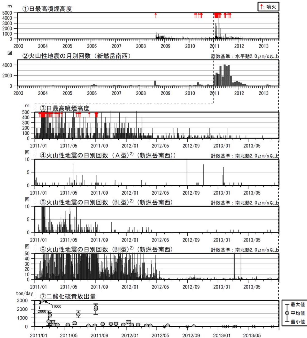
図3 霧島山（新燃岳） 火山活動経過図（2003年1月～2013年8月）
