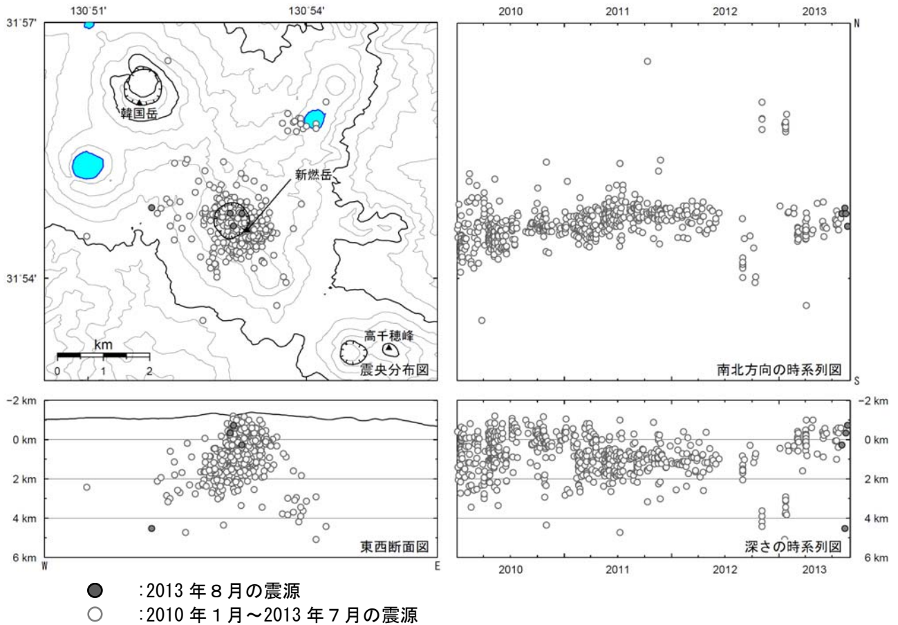
図 2 霧島山（新燃岳） 震源分布図（2010 年 1 月～2013 年 8 月）
