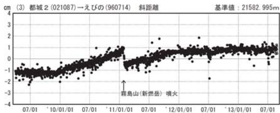
図 5 霧島山（新燃岳） 国土地理院による広域的な地殻変動観測結果*
