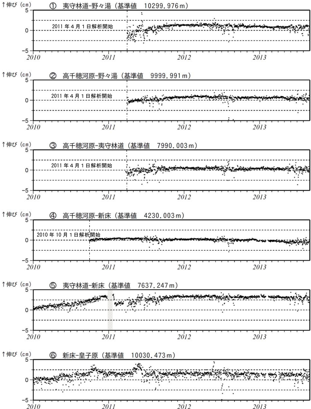
図 6-1 霧島山 GPS 連続観測による長期の基線長変化 (2010 年 1 月～2013 年 8 月)
