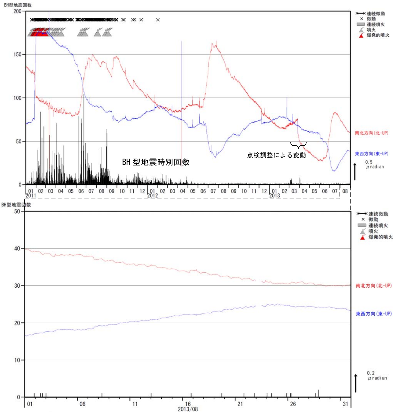
図4 霧島山（新燃岳） BH型地震の時間別回数と高千穂河原傾斜計の変化 (2011年1月～2013年8月)
