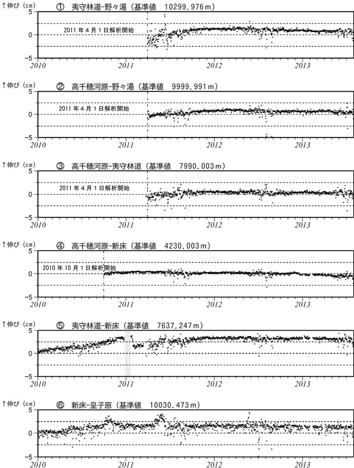
図 6-1 霧島山 GPS 連続観測による長期の基線長変化 (2010 年 1 月～2013 年 7 月)
