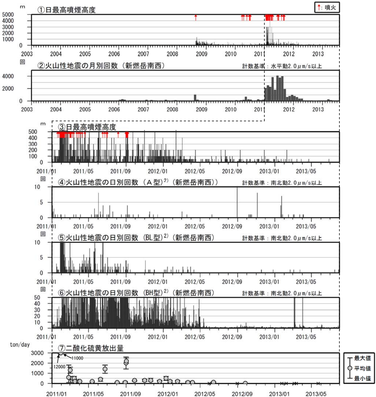
図3 霧島山（新燃岳）火山活動経過図（2003年1月～2013年7月）
