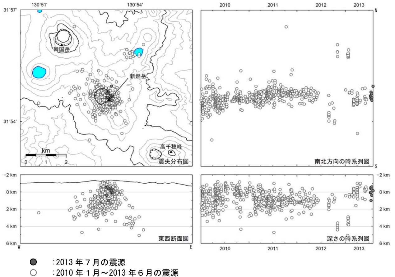
図 2 霧島山（新燃岳） 震源分布図（2010 年 1 月～2013 年 7 月）
