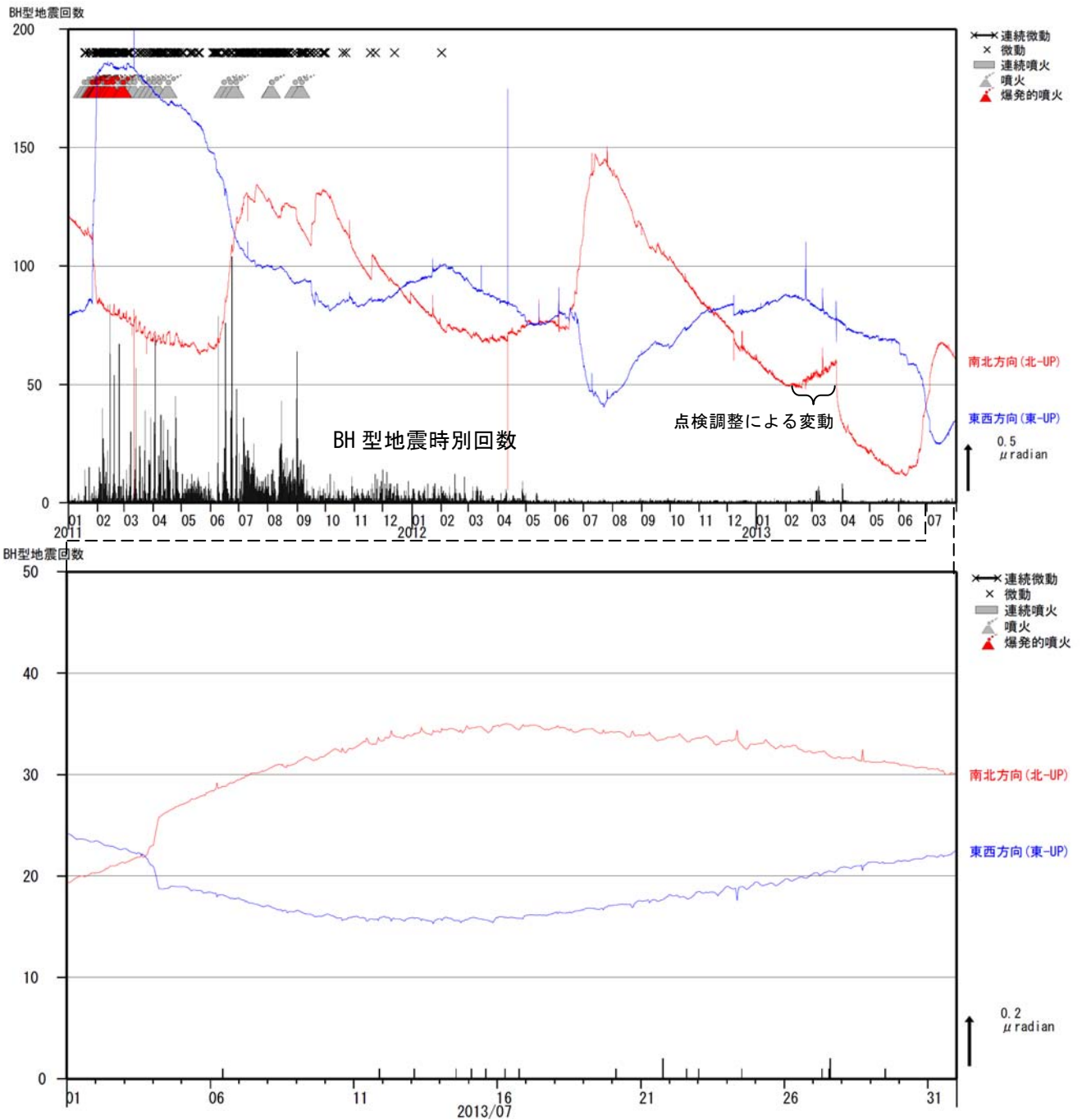
図4 霧島山（新燃岳） BH型地震の時間別回数と高千穂河原傾斜計の変化 （2011年1月～2013年7月）
