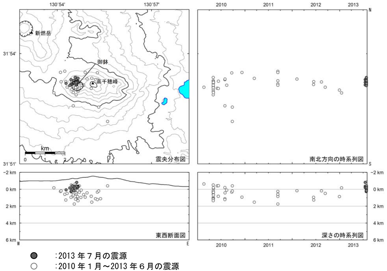
図 10 霧島山（御鉢） 震源分布図（2010 年 1 月～2013 年 7 月）
