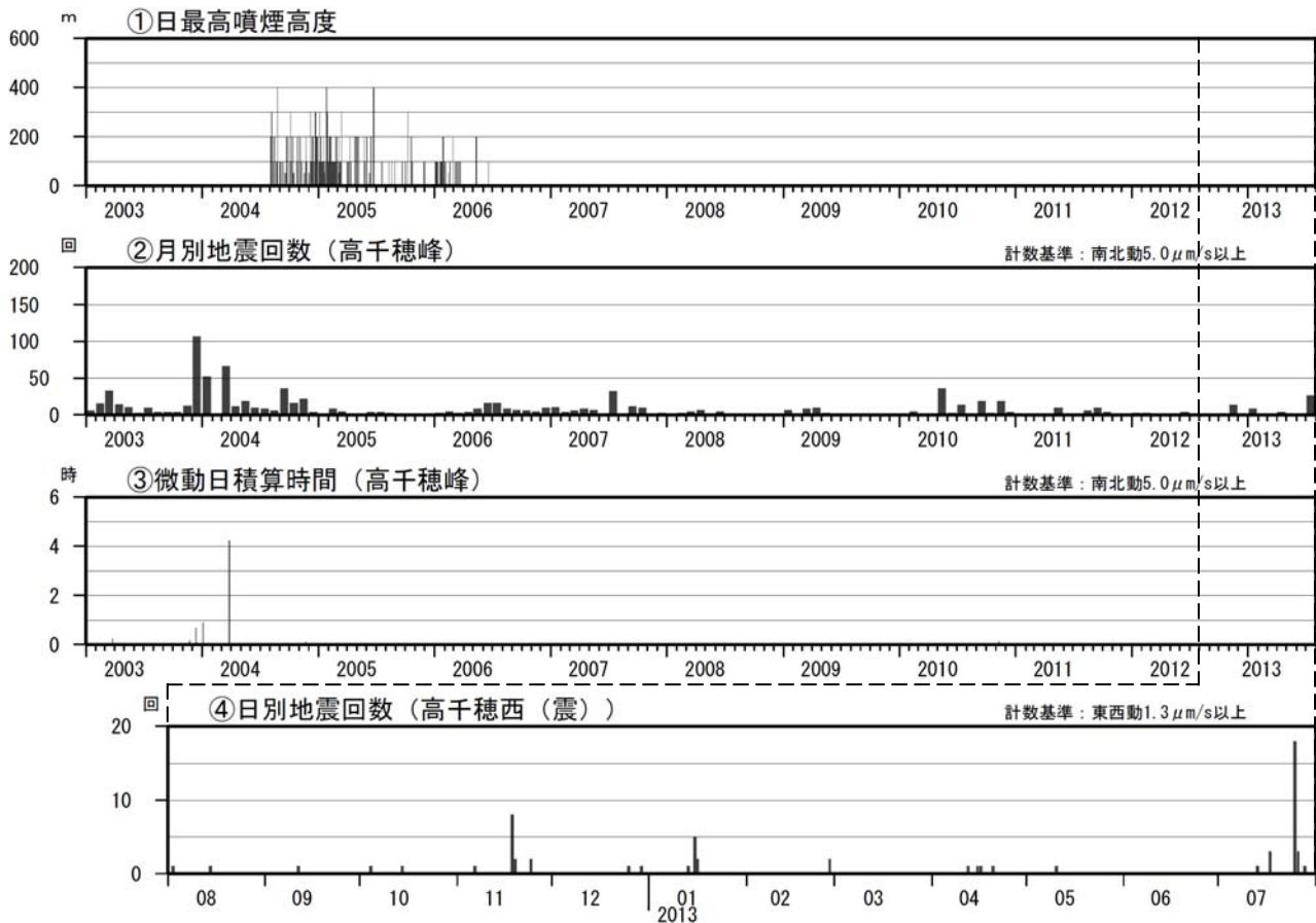
図 11 霧島山（御鉢） 火山活動経過図（2003 年 1 月～2013 年 7 月）
