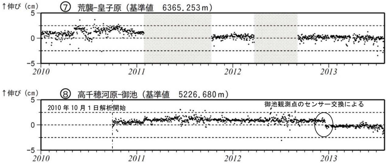
図 6-2 霧島山 GPS 連続観測による長期の基線長変化（2010 年 1 月～2013 年 7 月）
