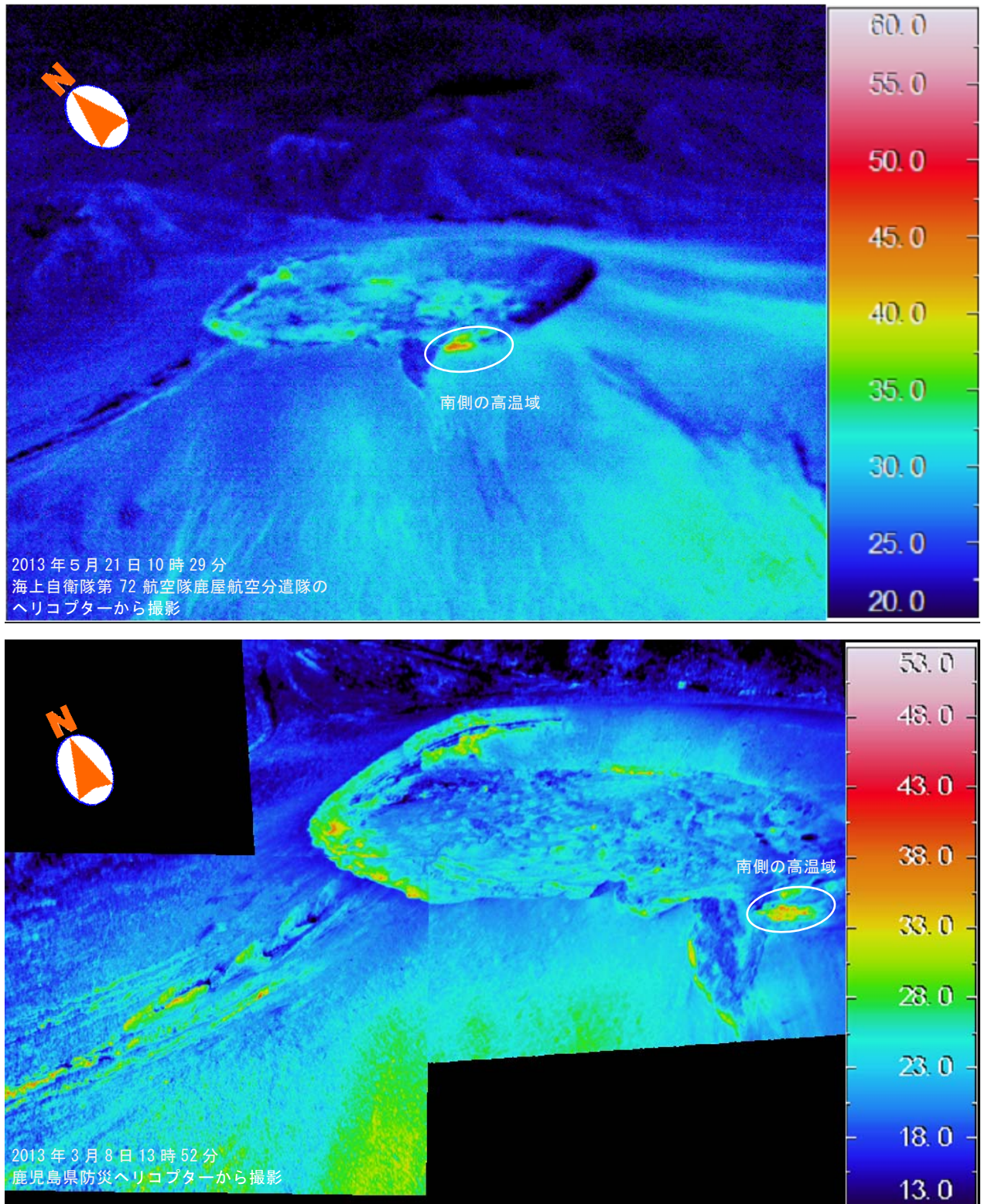
図 2 霧島山（新燃岳） 赤外熱映像装置による火口付近の地表面温度分布 火口の南側（白丸）を中心にやや温度の高い部分が認められました。
