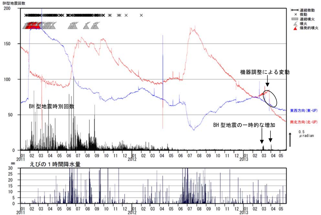
図3 霧島山（新燃岳） BH型地震 2) の時間別回数と高千穂河原傾斜計（新燃岳の南東約3km）の変化 (2011年1月～2013年5月20日)
