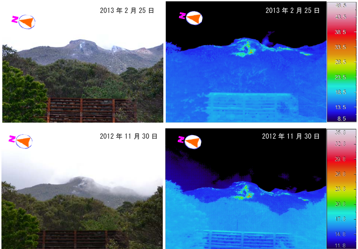
図7 口永良部島 新岳山頂及び周辺の状況
