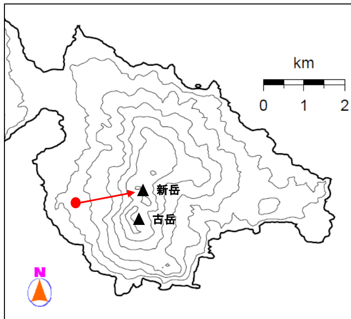
図8 口永良部島 赤外映像及び写真の撮影方向
