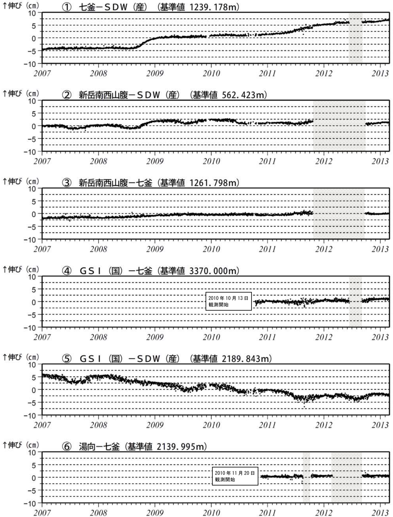
図 6-1※ 口永良部島 GPS 連続観測による基線長変化（2007 年 1 月～2013 年 2 月） GPS 連続観測では、火山活動によると考えられる変化は認められませんでした。
