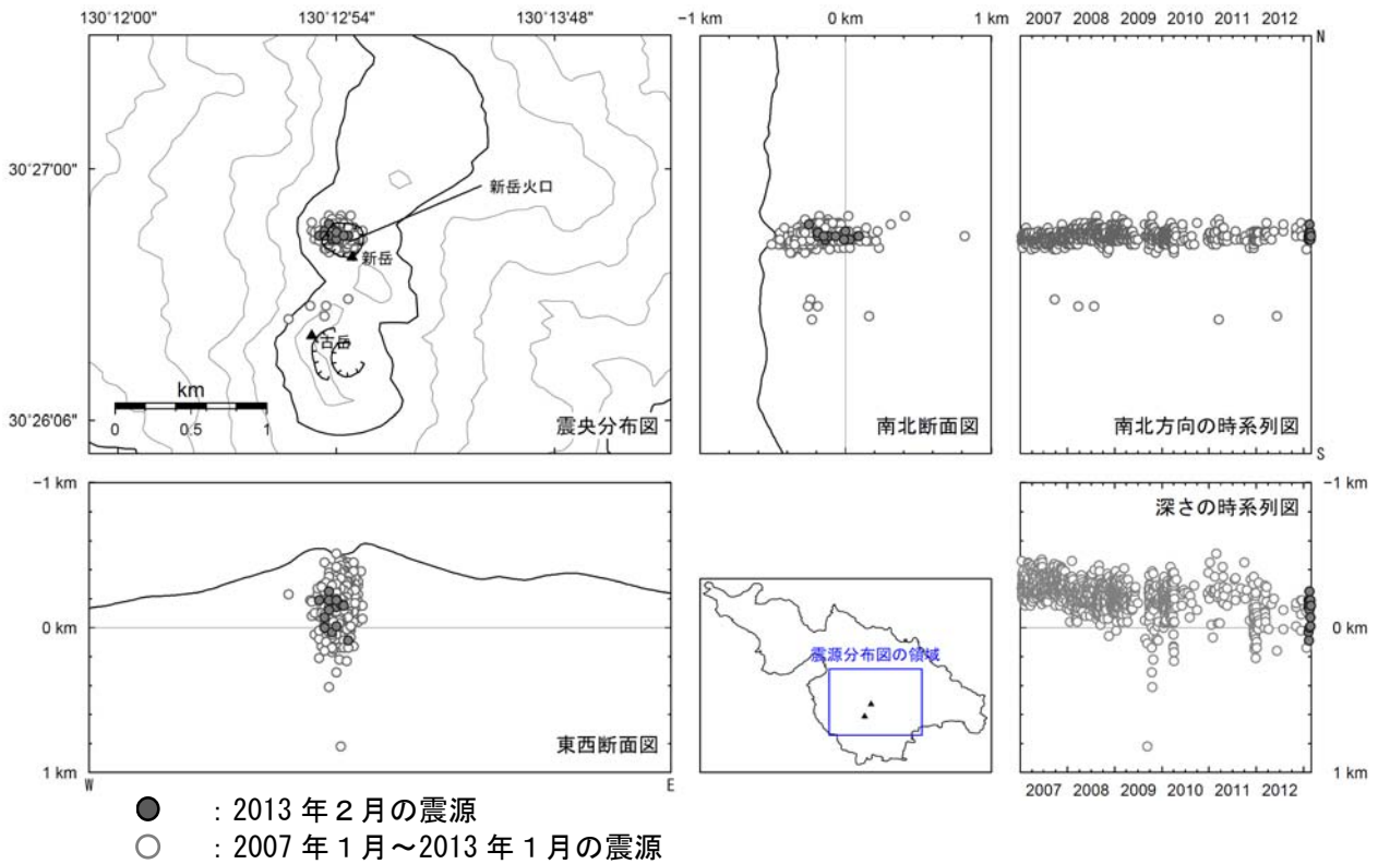
図 4※ 口永良部島 震源分布図（2007 年 1 月～2013 年 2 月） < 2 月の状況 >
