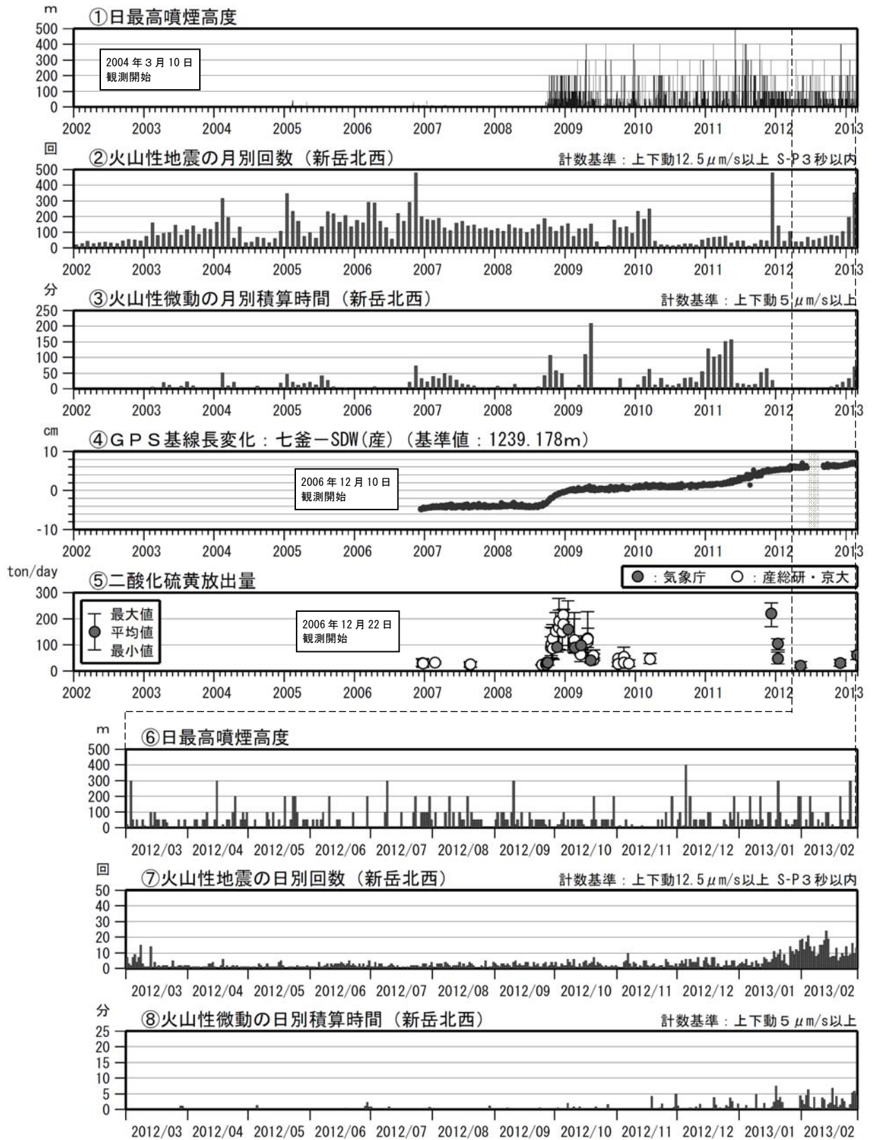
図3※ 口永良部島 火山活動経過図（2002年1月～2013年2月）
