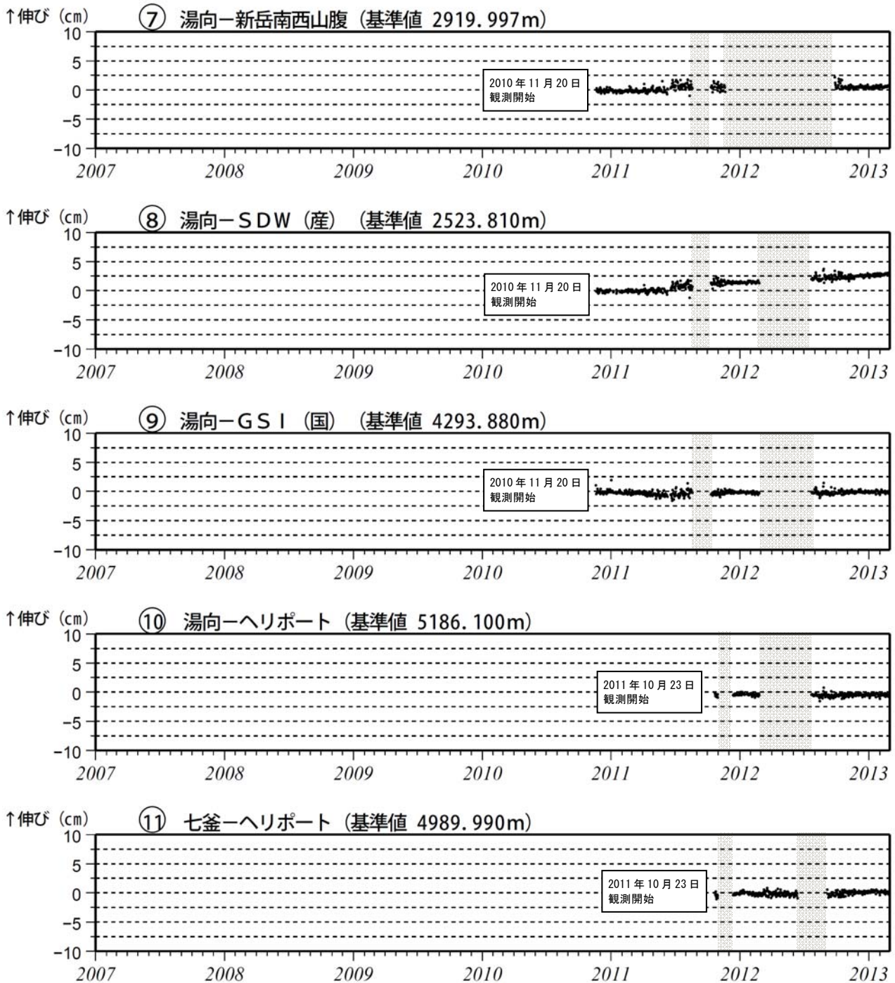
図 6-2※ 口永良部島 GPS 連続観測による基線長変化（2007 年 1 月～2013 年 2 月）
