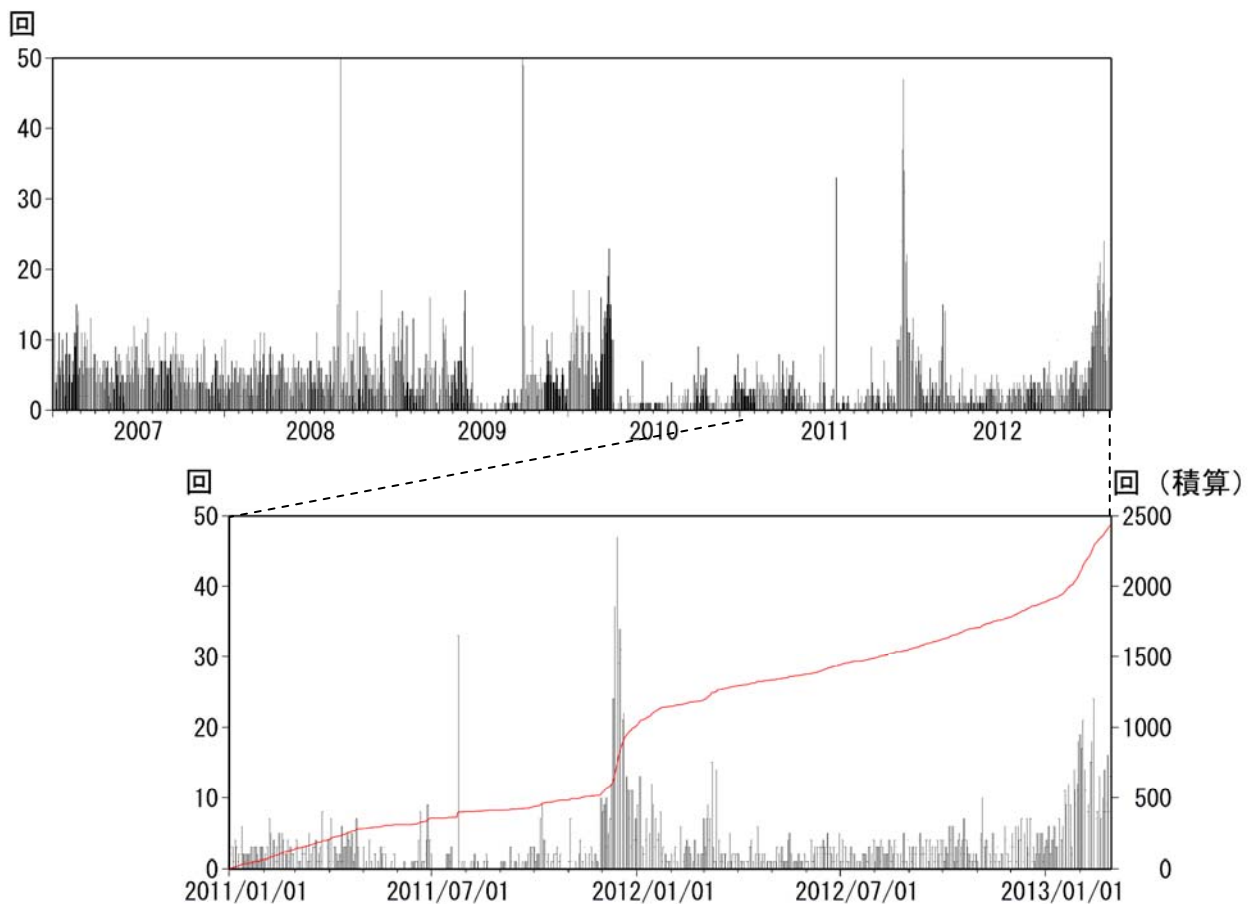
図 2 口永良部島 火山性地震の日別回数（2007年1月1日～2013年2月28日） 1月中旬頃から振幅の小さな火山性地震がやや増加しはじめ、2月中旬にやや減少したものの引き続きやや多い状態が続いています。月回数は352回（1月：277回）でした
