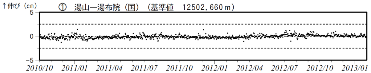
図 2※ 鶴見岳・伽藍岳 GPS連続観測による基線長変化（2010 年 10 月～2013 年 1 月） 火山活動によると考えられる変化は認められませんでした。
