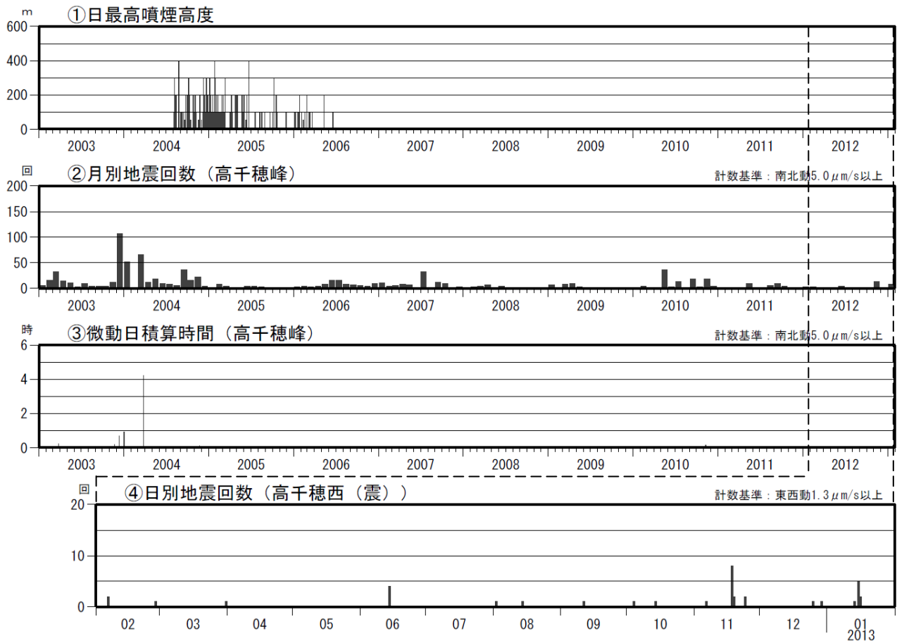
図 10※ 霧島山（御鉢） 火山活動経過図（2003 年 1 月～2013 年 1 月）
