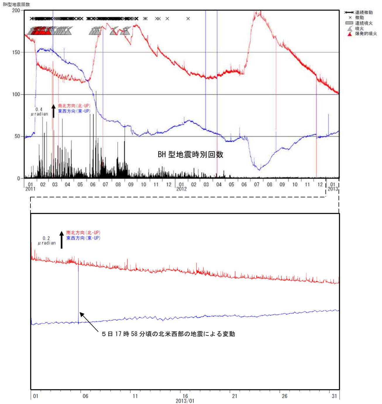
図4 霧島山（新燃岳） BH型地震の時間別回数と高千穂河原傾斜計の変化 （2011年1月～2013年1月）
