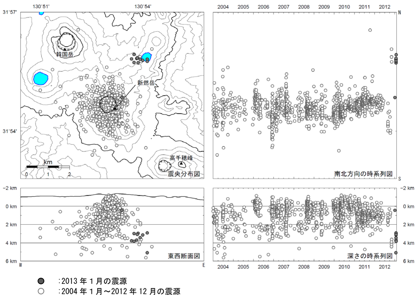
図 2※ 霧島山（新燃岳） 震源分布図（2004 年 1 月～2013 年 1 月）
