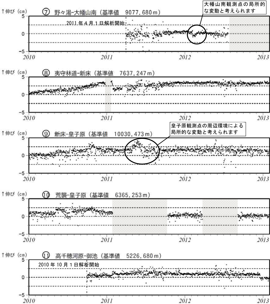
図 6-2 霧島山 GPS 連続観測による長期の基線長変化（2010 年 1 月～2013 年 1 月）
