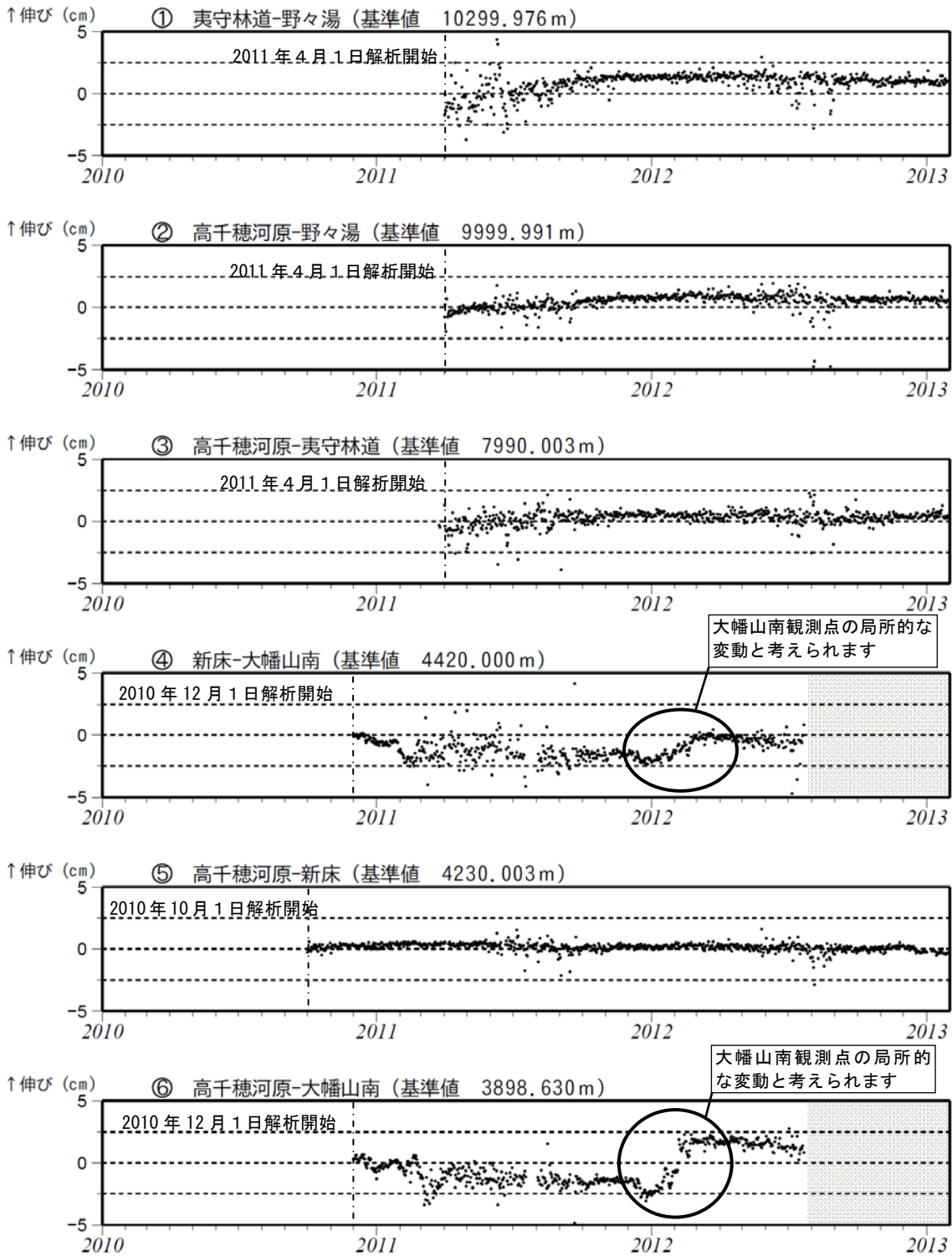
図 6-1 霧島山 GPS 連続観測による長期の基線長変化 (2010 年 1 月～2013 年 1 月)
