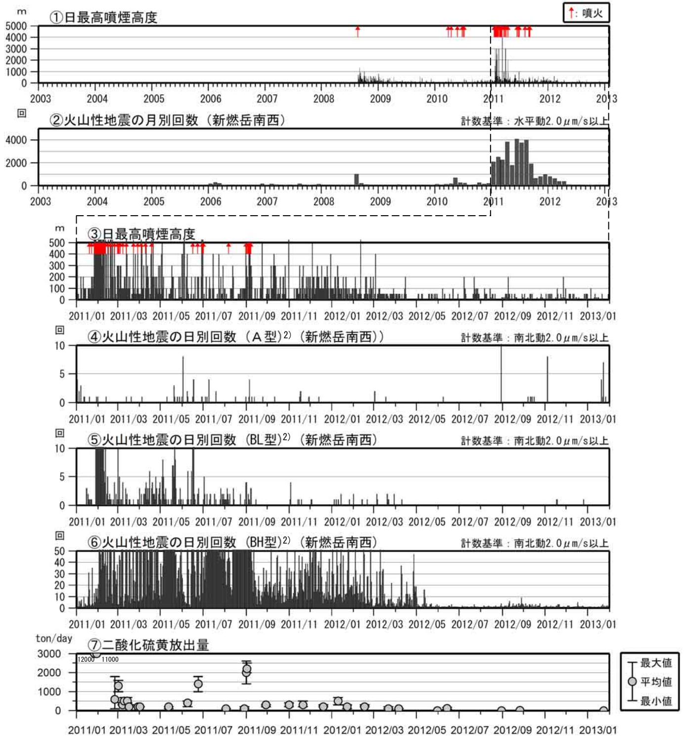
図 3※ 霧島山（新燃岳） 火山活動経過図（2003 年 1 月～2013 年 1 月）
