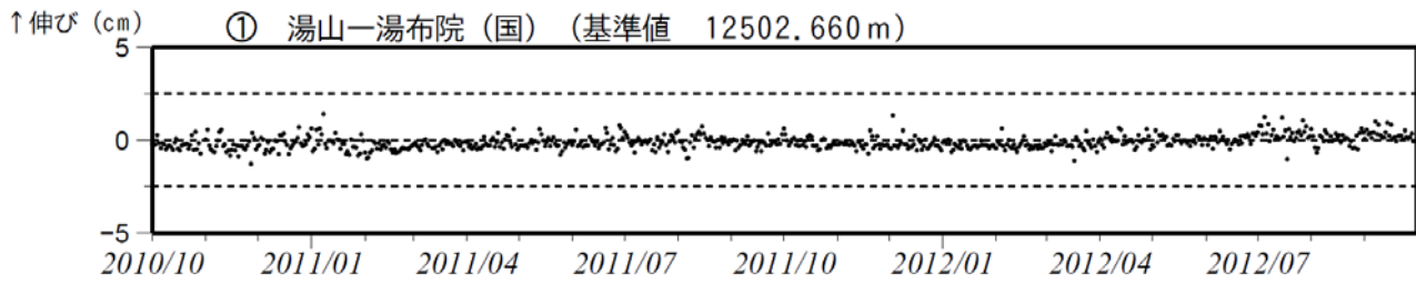
図2※ 鶴見岳・伽藍岳 GPS連続観測による基線長変化（2010年10月～2012年9月） 火山活動によると考えられる変化は認められませんでした。 この基線は図3の①に対応しています。
