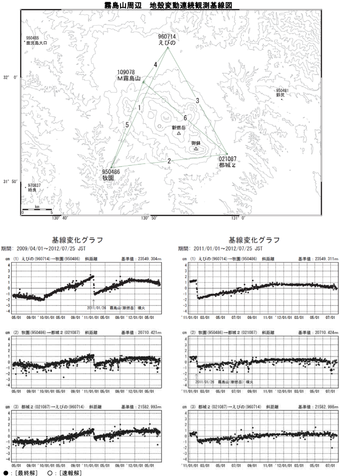
図 4 ※ 霧島山（新燃岳） 国土地理院による広域的な地殻変動観測結果*
