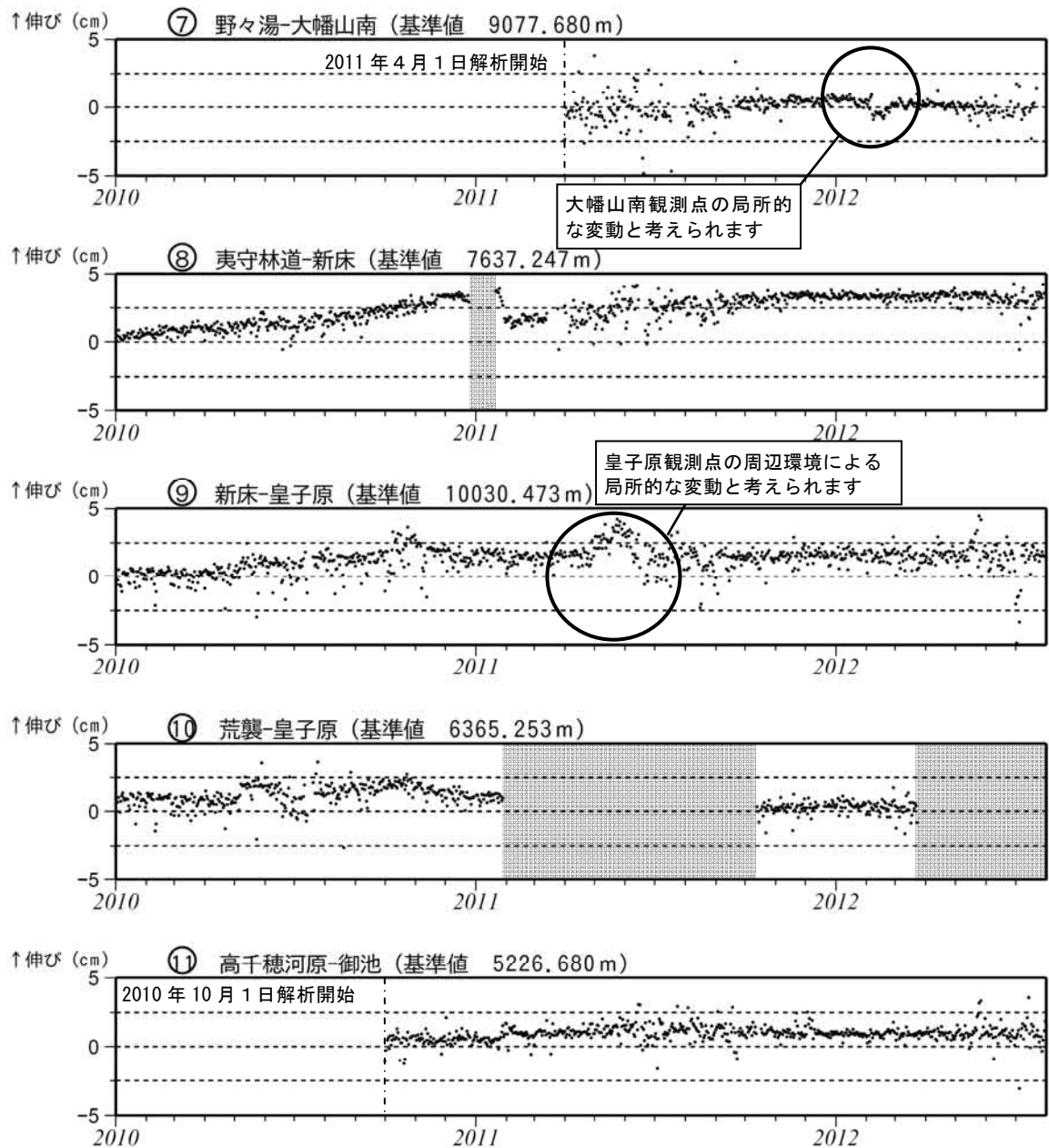
図 5-2 霧島山 GPS 連続観測による長期の基線長変化 (2010 年 1 月～2012 年 7 月)
