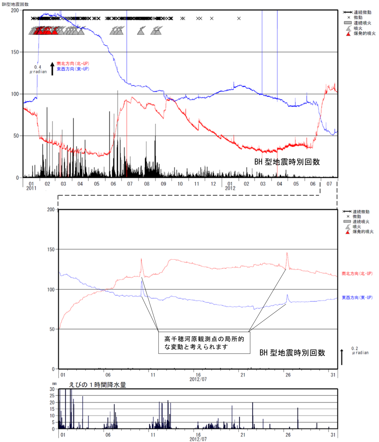
図3 霧島山（新燃岳） BH型地震の時間別回数と高千穂河原傾斜計の変化 (2011年1月～2012年7月)
