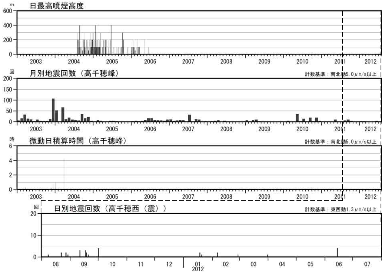
図9※ 霧島山（御鉢） 火山活動経過図（2003年1月～2012年7月） <7月の状況>
