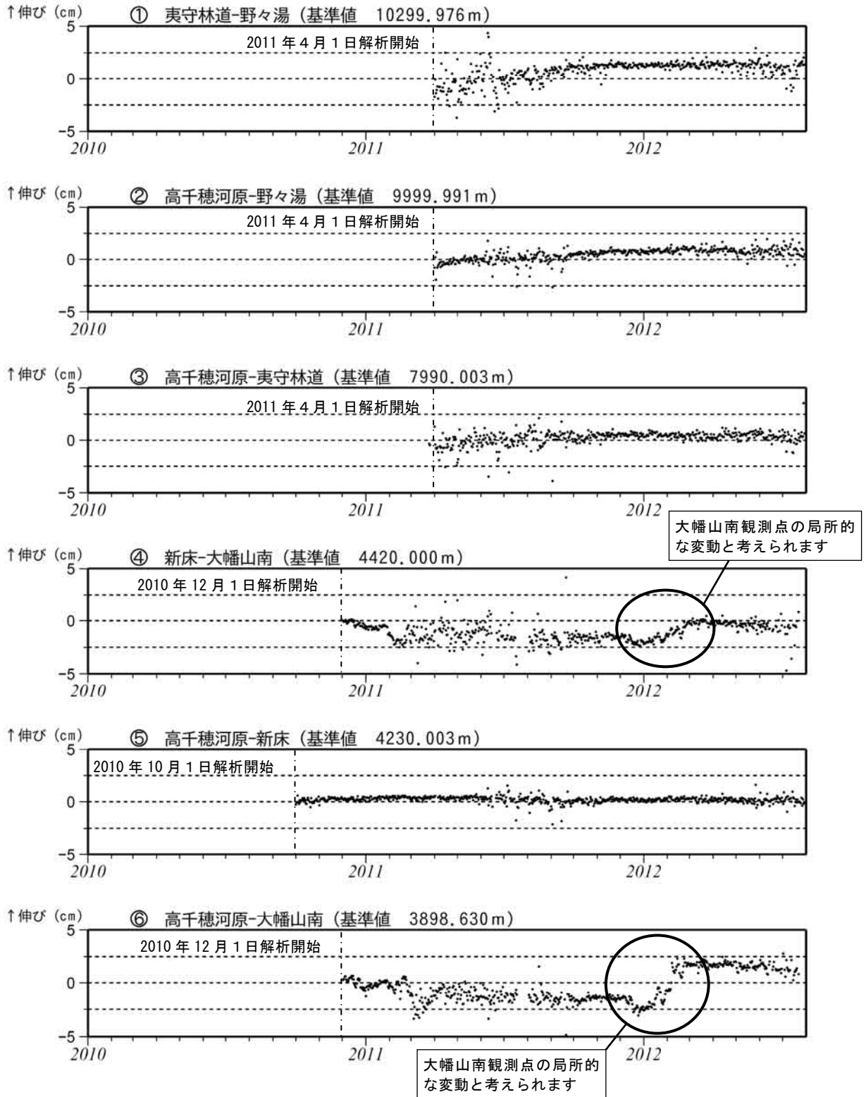
図 5-1 霧島山 GPS 連続観測による長期の基線長変化 (2010 年 1 月～2012 年 7 月) GPS 連続観測では、新燃岳周辺の基線で火山活動によると思われる変化は認められませんでした。
