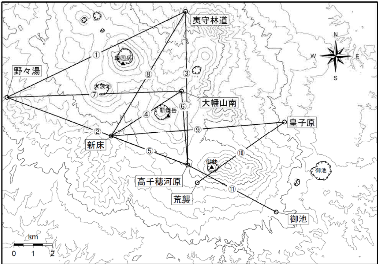
図 6 霧島山 GPS 連続観測点と基線番号
