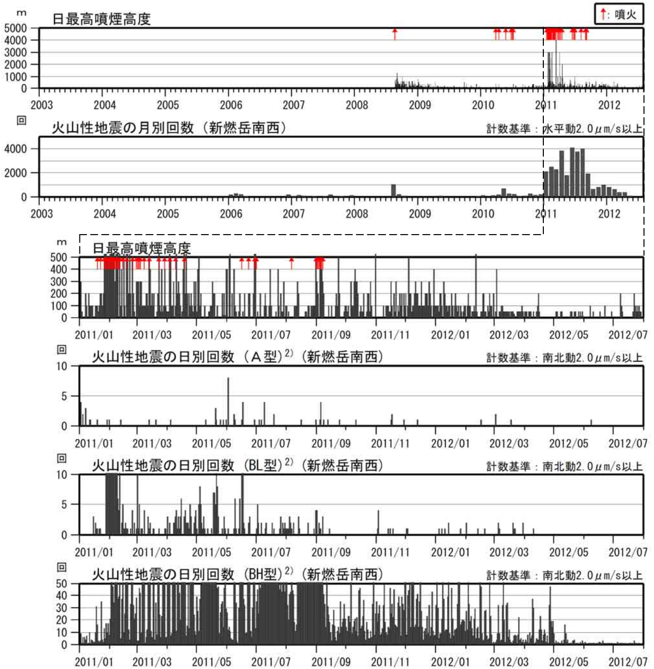
図 2※ 霧島山（新燃岳） 火山活動経過図（2003 年 1 月～2012 年 7 月）
