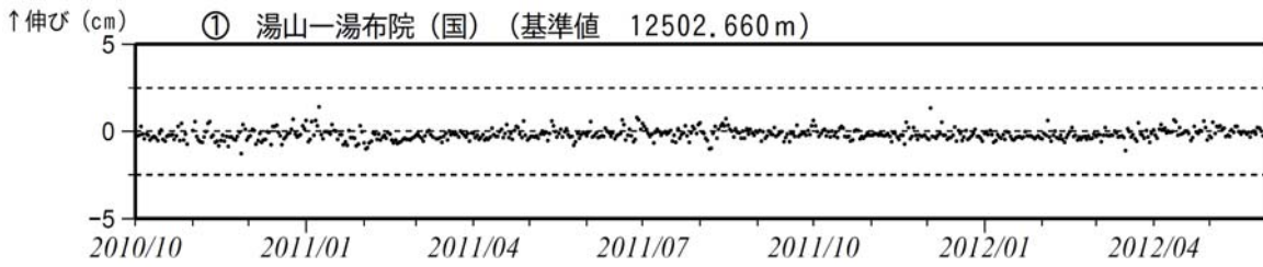
図 2※ 鶴見岳・伽藍岳 GPS連続観測による基線長変化（2010年10月～2012年5月） < 5月の状況 > 火山活動によると考えられる変化は認められませんでした。 この基線は図3の①に対応しています。
