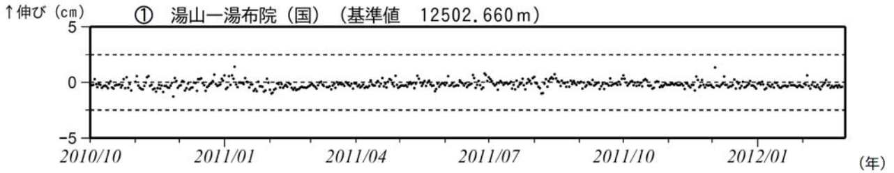
図 2※ 鶴見岳・伽藍岳 GPS連続観測による基線長変化（2010 年 10 月～2012 年 2 月） < 2 月の状況 > 火山活動によると考えられる変化は認められませんでした。 この基線は図 3 の①に対応しています。
